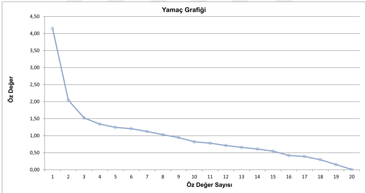
Şekil 4.3: Türkçe Form-I'e Ait Yamaç Grafiği
