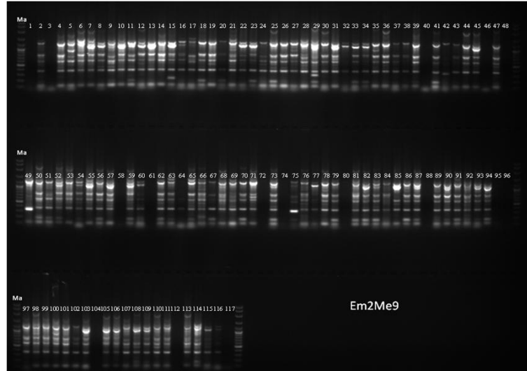
Şekil 4.7. Venturia inaequalis izolatlarının SRAP primer kombinasyonundan elde edilen jel görüntüsü, Ma:100bp DNA ladder
