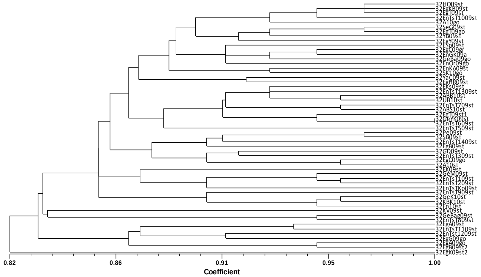
Şekil 4.11. Isparta ili Venturia inaequalis izolatlarının ISSR markırlarının analizi ile oluşturulan filogenetik soy ağacı.
