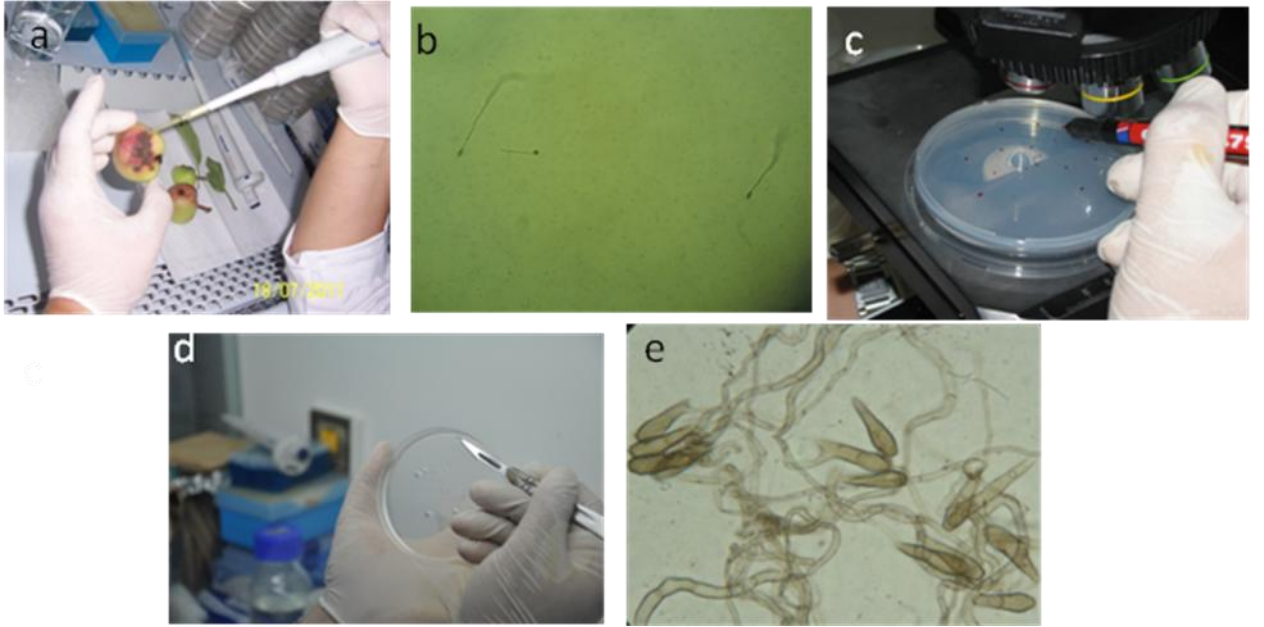
Şekil 3.1. Venturia inaequalis izolatlarından tek spor izolasyonu işlemi; a) primer lezyonlardan steril distile su ile spor süspansiyonun hazırlanışı, b-c) çimlenen konidisporların mikroskopta tespiti ve işaretlenmesi d) PDA ortamına aktarılması e) gelişen misel ve konidisporlar
