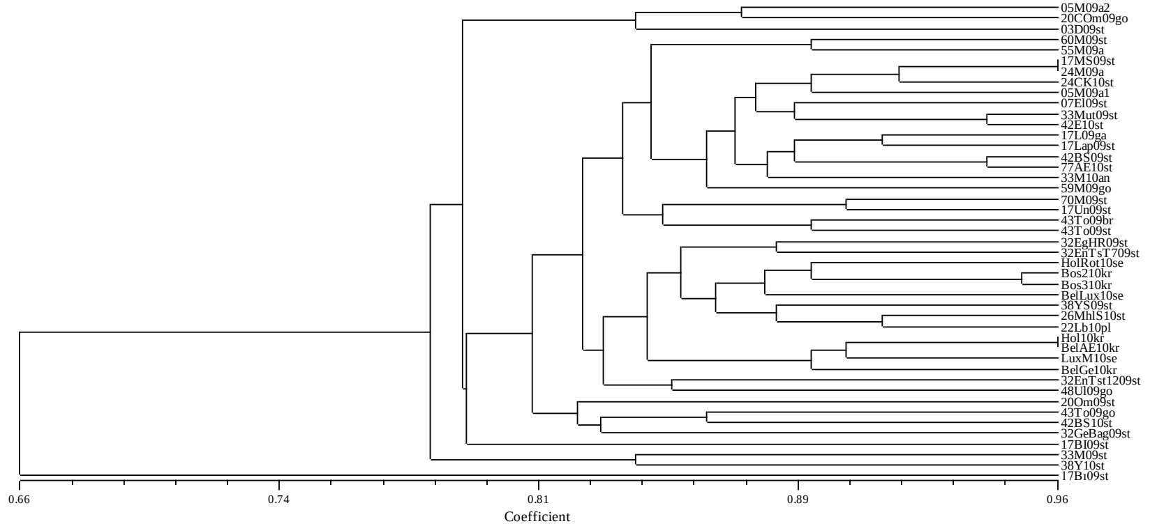
Şekil 4.19. Türkiye grubu Venturia inaequalis izolatlarının SRAP markırlarının analizi ile oluşturulan filogenetik soy ağacı.
