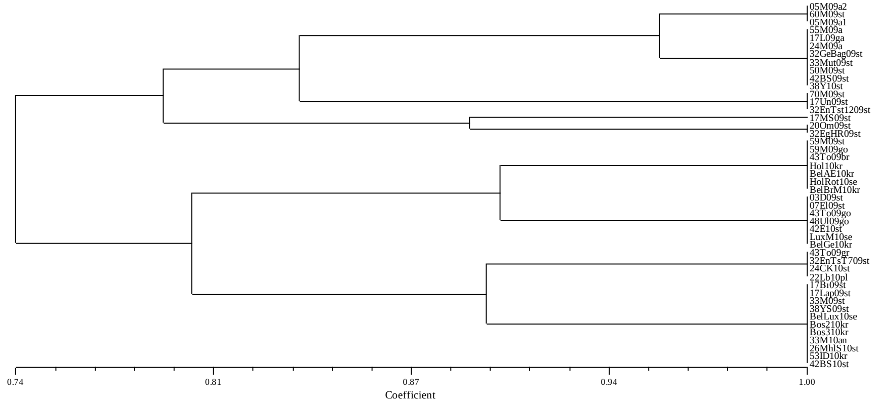
Şekil 4.18. Türkiye grubu Venturia inaequalis izolatlarının SSR markırlarının analizi ile oluşturulan filogenetik soy ağacı.
