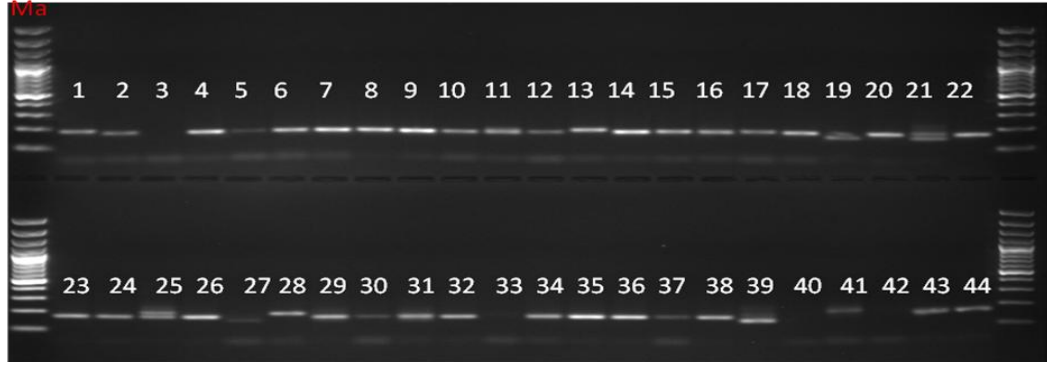
Şekil 4.6. Venturia inaequalis izolatlarının 1tc1b SSR primer çiftinden elde edilen jel görüntüsü, Ma:100bp DNA ladder
