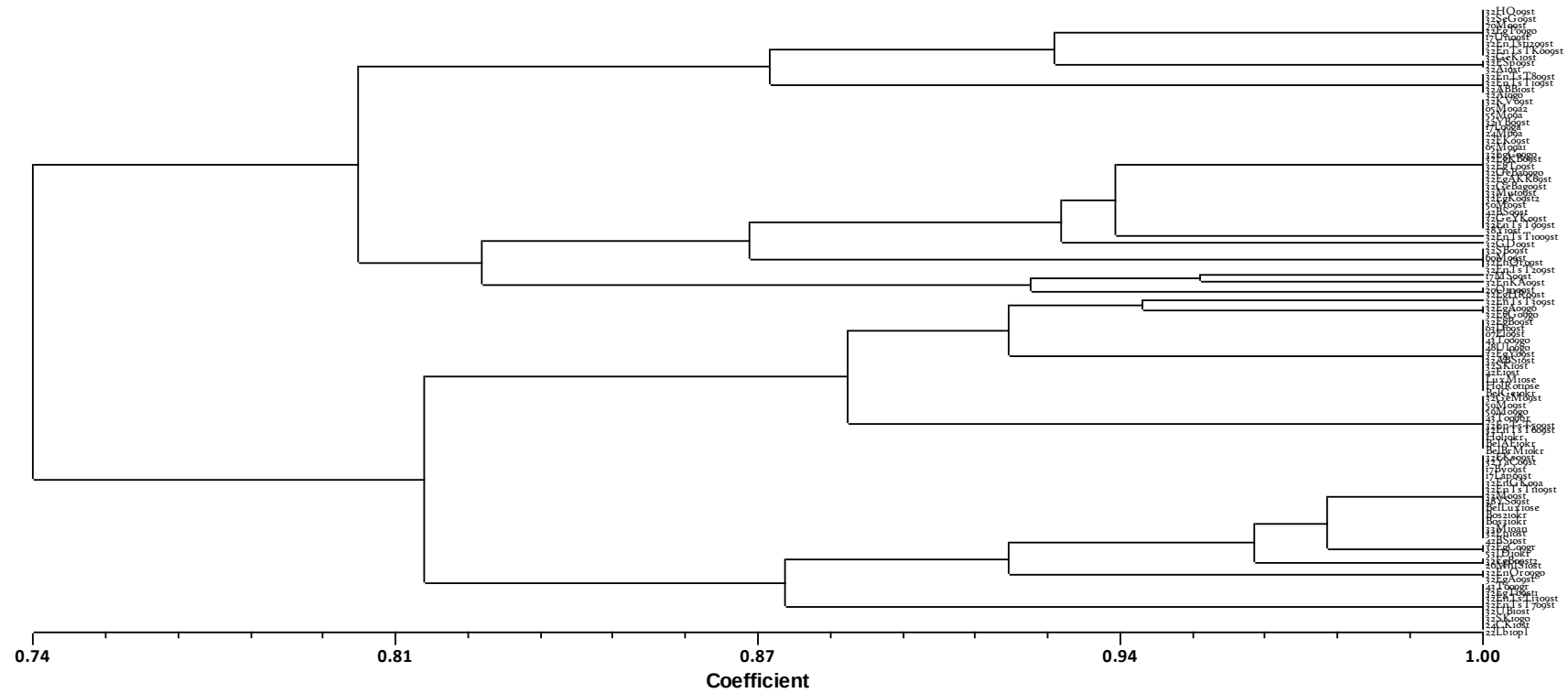
Ek. 12. Tüm Venturia inaequalis Örneklerinin SSR Markırı Kullanılarak UPGMA Metodu ile Elde Edilen ve Genetik Benzerlikleri Gösteren Dendrogram
