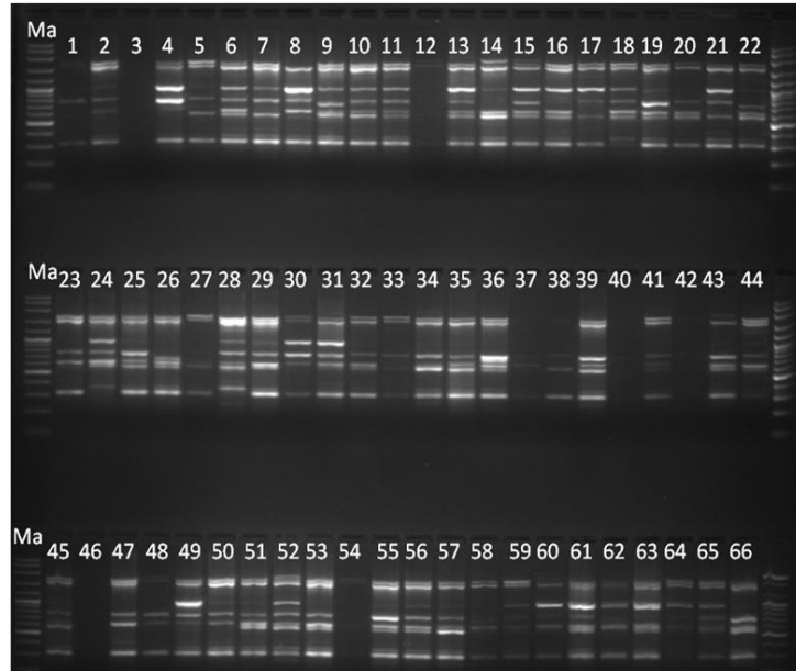
Şekil 4.4. Venturia inaequalis izolatlarının UBC 888 ISSR primerinden elde edilen jel görüntüsü Ma:100bp DNA ladder
