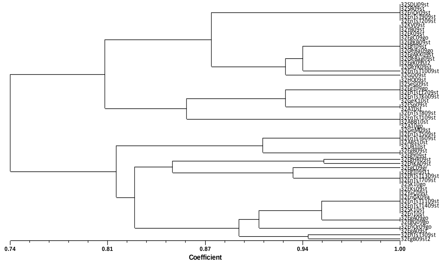
Şekil 4.12. Isparta ili Venturia inaequalis izolatlarının SSR markırlarının analizi ile oluşturulan filogenetik soy ağacı.
