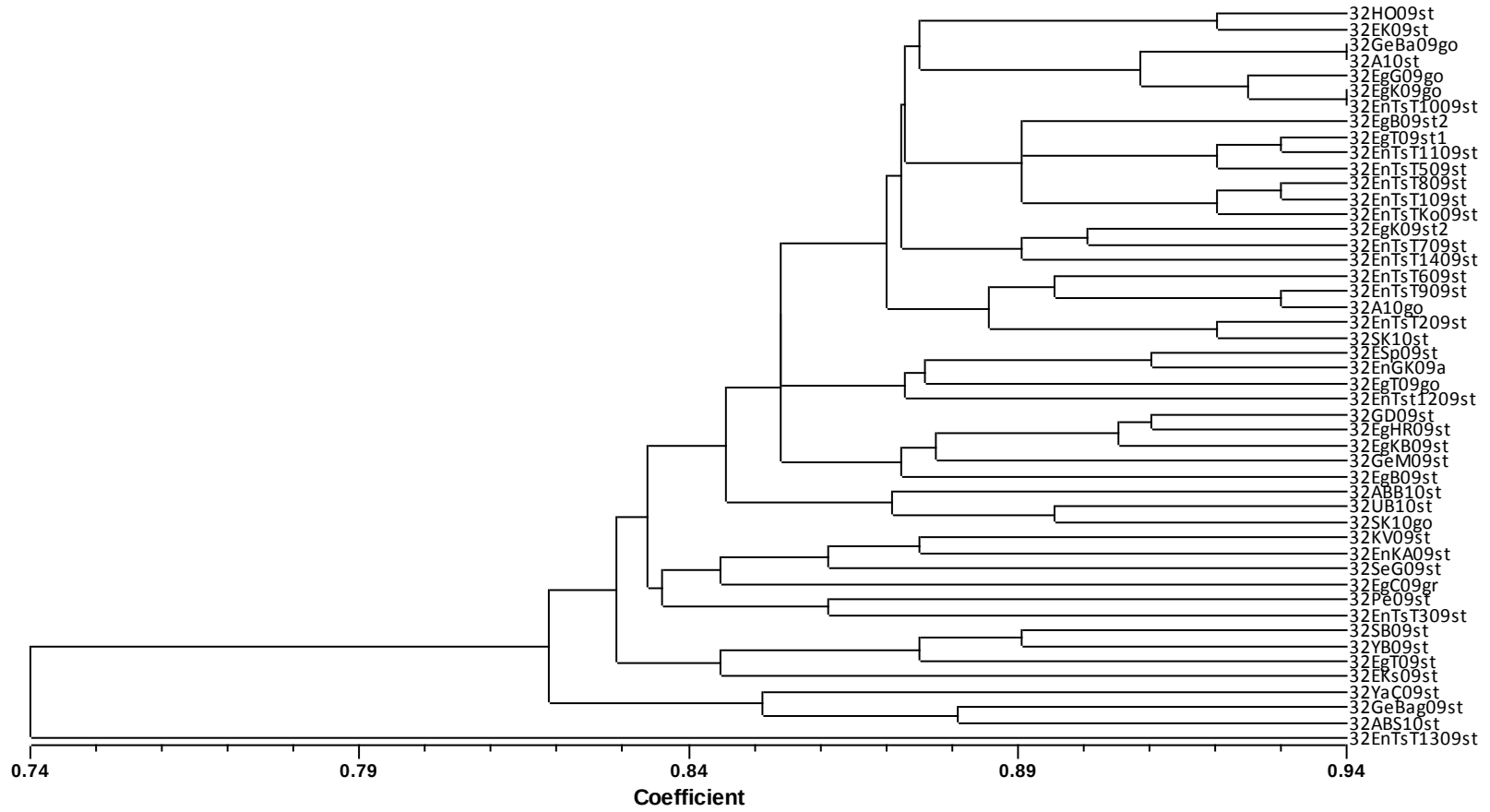
Şekil 4.13. Isparta ili Venturia inaequalis izolatlarının SRAP markırlarının analizi ile oluşturulan filogenetik soy ağacı.
