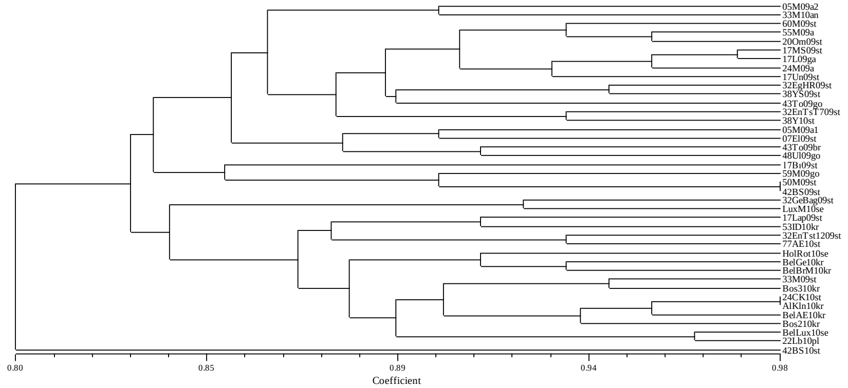
Şekil 4.17. Türkiye grubu Venturia inaequalis izolatlarının ISSR markırlarının analizi ile oluşturulan filogenetik soy ağacı.
