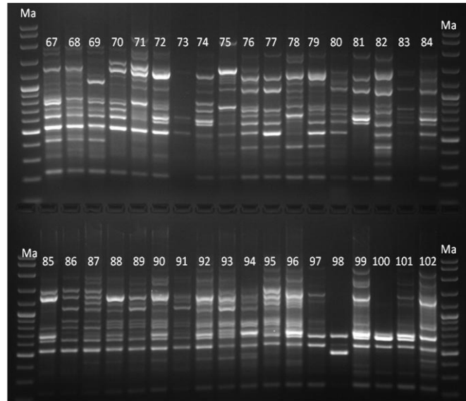
Şekil 4.1. Venturia inaequalis izolatlarının M2 RAPD primerinden elde edilen jel görüntüsü, Ma:100bp DNA ladder
