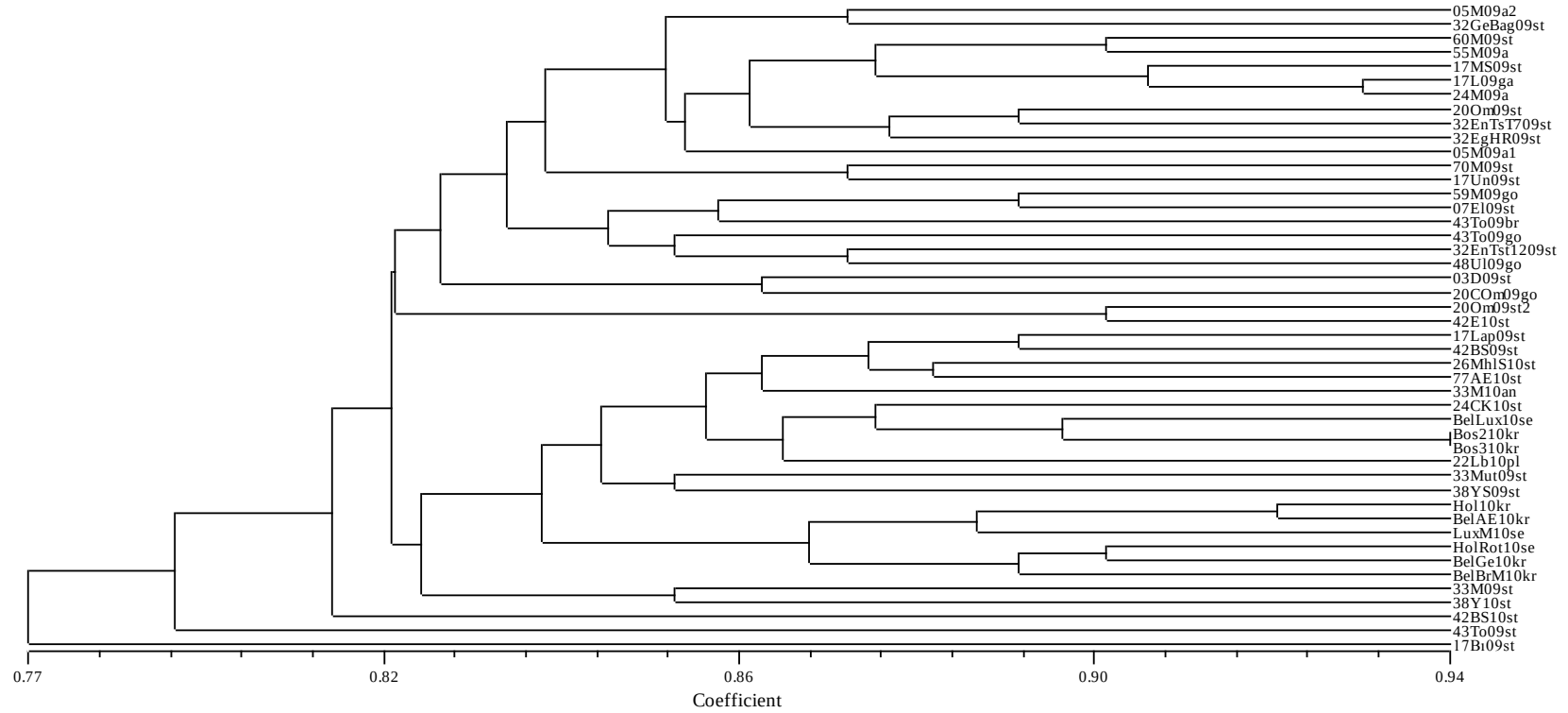
Şekil 4.20. Türkiye grubu Venturia inaequalis izolatlarının RAPD, ISSR, SSR ve SRAP markırlarının tümü kullanılarak oluşturulan filogenetik soy ağacı.
