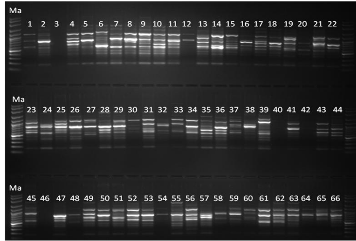
Şekil 4.3. Venturia inaequalis izolatlarının UBC 880 ISSR primerinden elde edilen jel görüntüsü Ma:100bp DNA ladder
