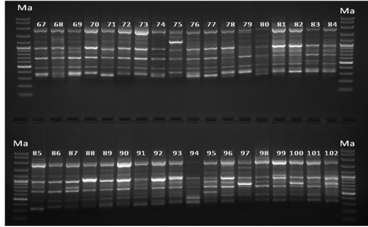
Şekil 4.2. Venturia inaequalis izolatlarının OPG05 RAPD primerinden elde edilen jel görüntüsü Ma:100bp DNA ladder
