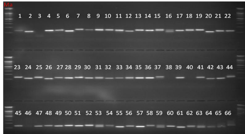
Şekil 4.5. Venturia inaequalis izolatlarının 1tc1a SSR primer çiftinden elde edilen jel görüntüsü, Ma:100bp DNA ladder
