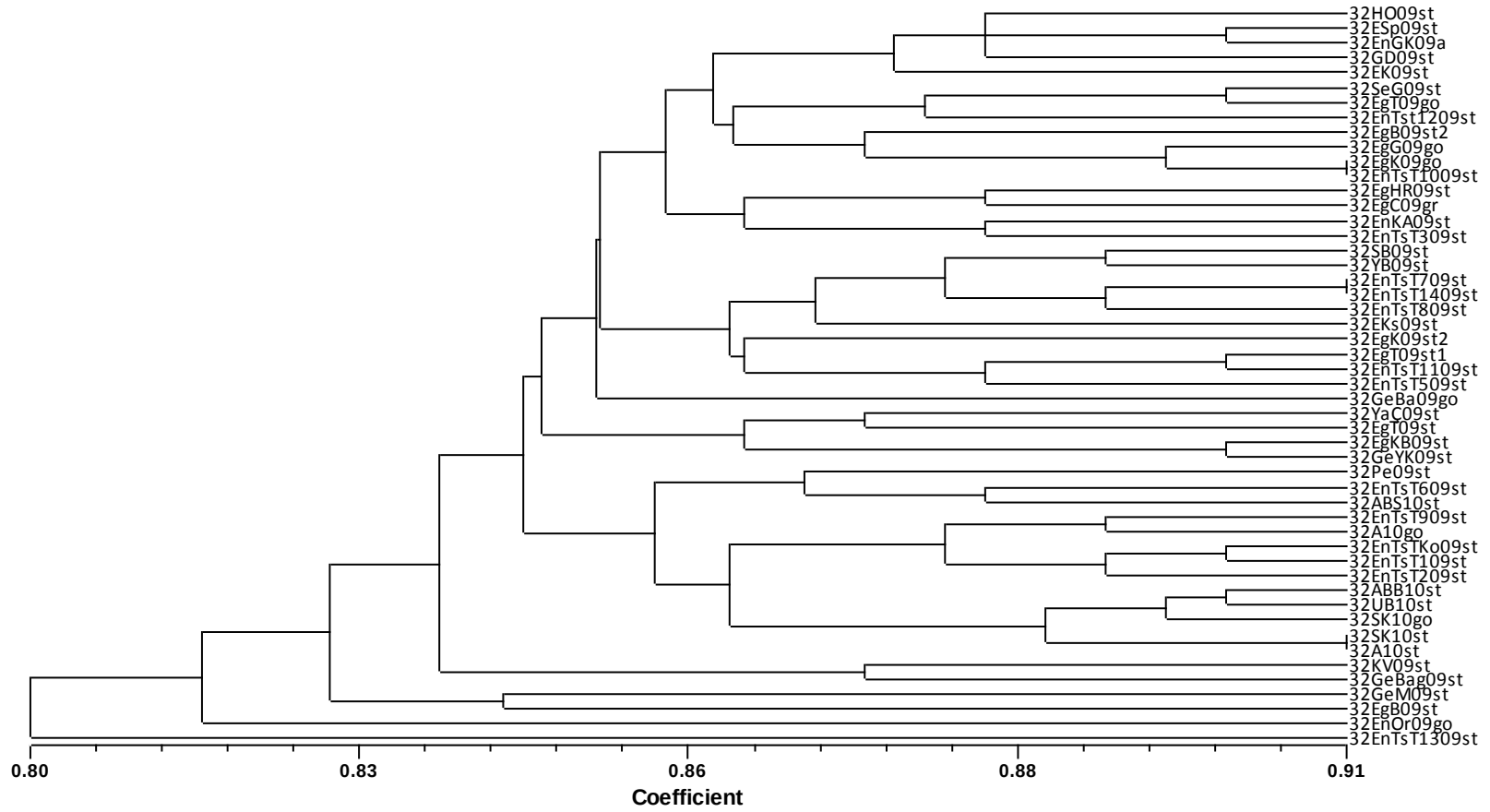
Şekil 4.14. Isparta ili Venturia inaequalis izolatlarının RAPD, ISSR, SSR ve SRAP markırlarının tümü kullanılarak oluşturulan filogenetik soy ağacı.
