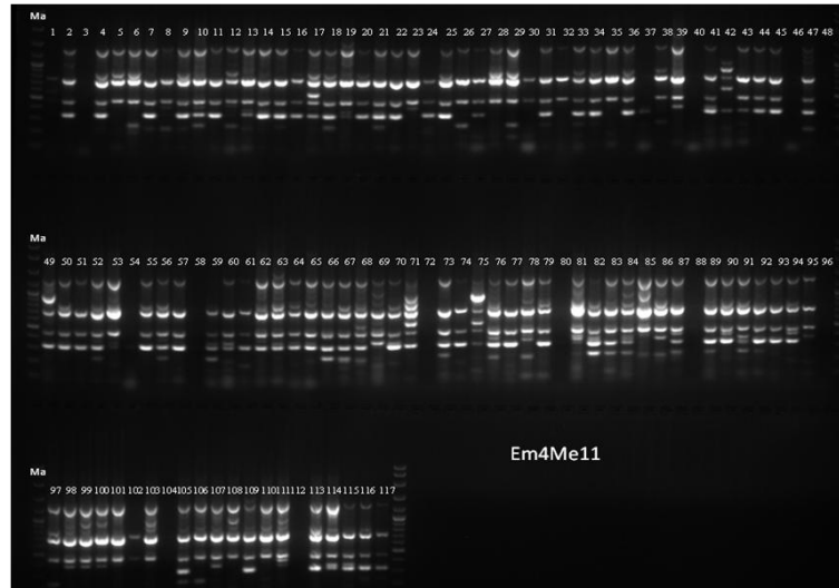
Şekil4.8. Venturia inaequalis izolatlarının SRAP primer kombinasyonundan elde edilen jel görüntüsü, Ma:100bp DNA ladder
