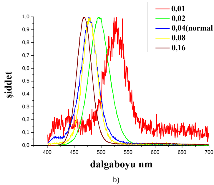
Şekil 3.5. Farklı Se/S oranlarına sahip CdSeS nanokristallerinin (a) absorpsiyon (b) flüoresans spektrumları
