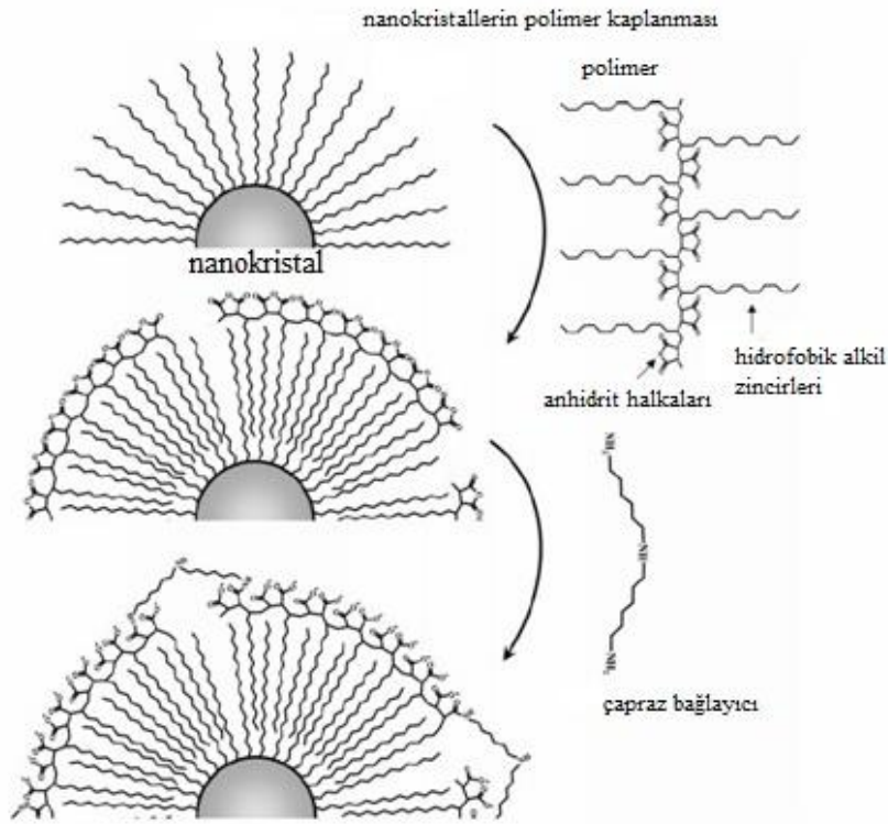
Şekil 1.17. Hidrofobik bir nanokristalin yüzeyinin polimaleik anhidrit türevi ile korumaya alınması (Parak ve ark. 2004)
