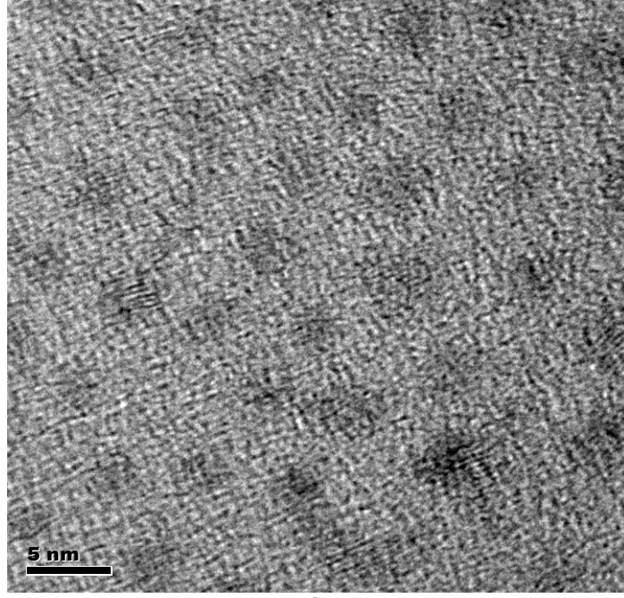
Şekil 3.9. CdSeS alaşım nanokristallerin TEM görüntüleri.
