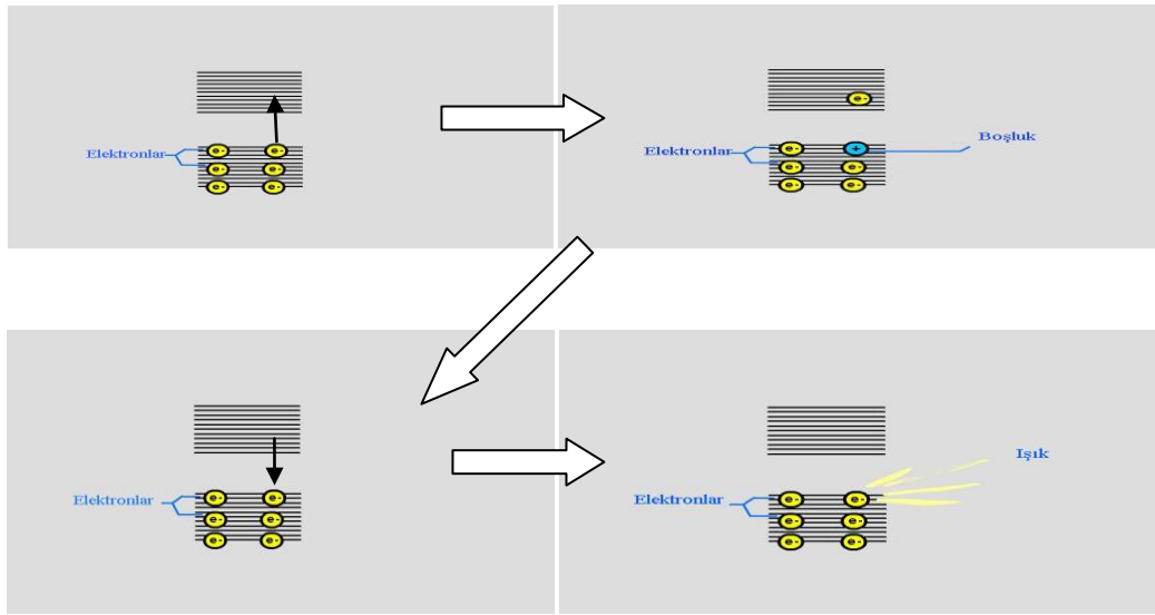
Şekil 1.24. Elektrolüminesans olayı
