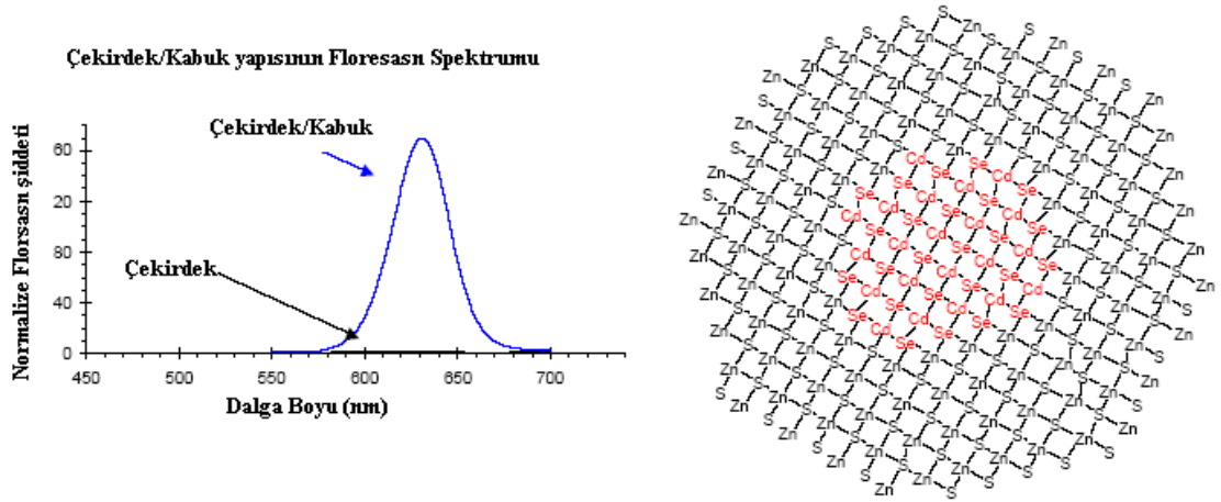
Şekil 1.6. CdSe/ZnS yapısına ait kristal şekli ve bunların flüoresans spektrumları (Quantum dot corp.2003)
