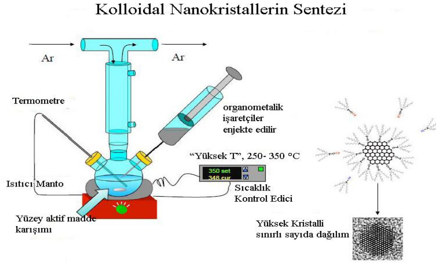
Şekil1.13. Kolloidal nanokristallerin sentezi
