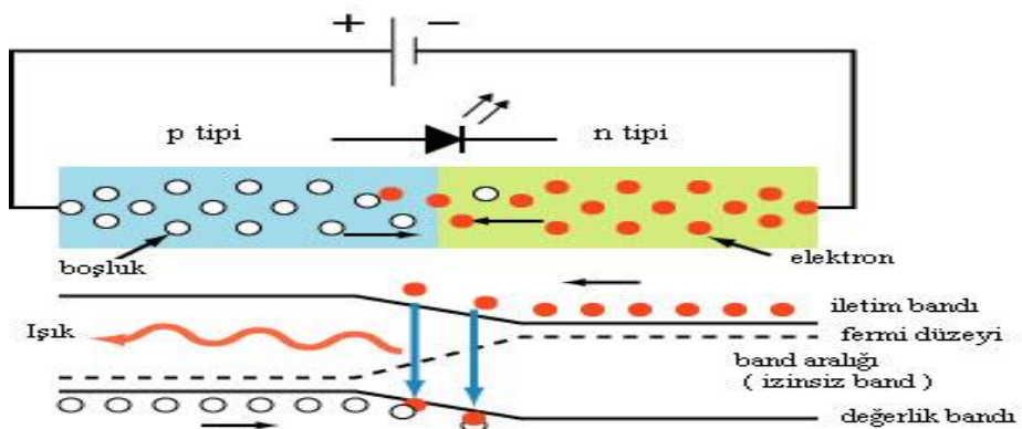
Şekil 1.23. LED'in çalışma mekanizması
