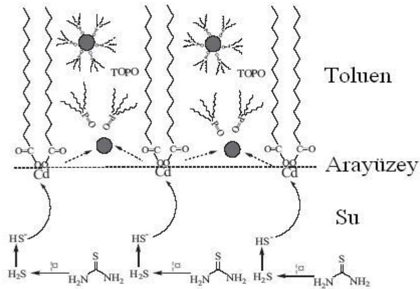
Şekil 2.3. Çift faz metodunda arayüzeyde kristal oluşumu (Pan ve ark., 2005)
