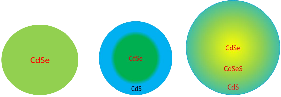
Şekil 3.8. Çekirdek, Çekirdek/kabuk, ve dereceli alaşım nanokristal yapılar
