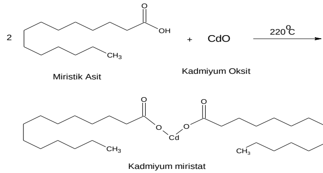
Şekil 2.1. Kadmiyum miristat sentezi
