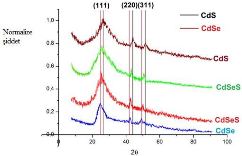
Şekil 3.7. CdS, CdSeS ve CdSe nanokristallerinin XRD spektrumu.
