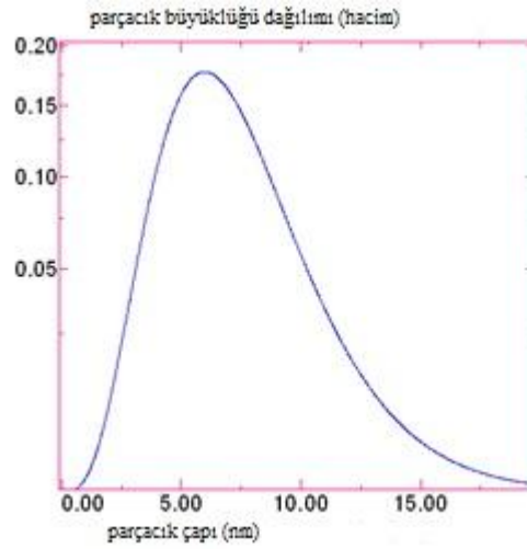
Şekil 3.6. SAXS ölçümlerine göre parçacık boyutu dağılımı (a, b, c) (sırasıyla 3, 5 ve 6.5 nm)
