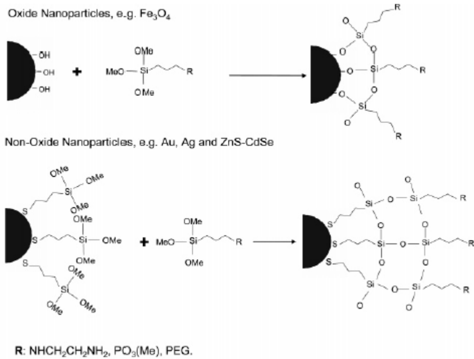
Şekil 1.16. Nanoparçacık yüzeyinin silan ile kaplanması (ying ve ark. 2007)
