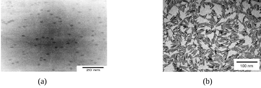
Şekil 1.9. a: Murray ve ark. (1993) tarafından sentezlenen CdSe küresel parçacıkları, b: Alivizatos ve ark. (2000) tarafından sentezlenen çubuk şeklindeki nanoparçacıkların TEM görüntüleri
