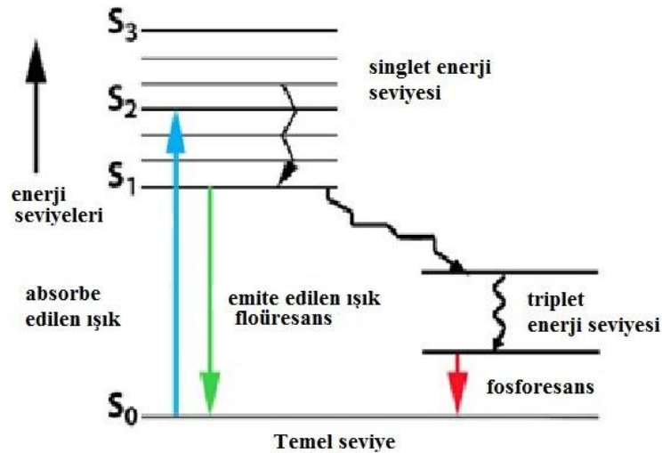
Şekil 1.7. Absorpsiyon ve flüoresansın şematik gösterimi (anonim university of Victoria 2005)
