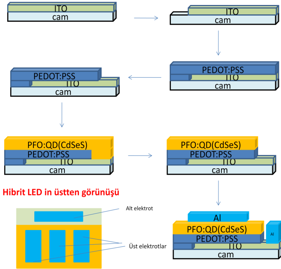
Şekil 3.6. Hibrit led hazırlanışı
