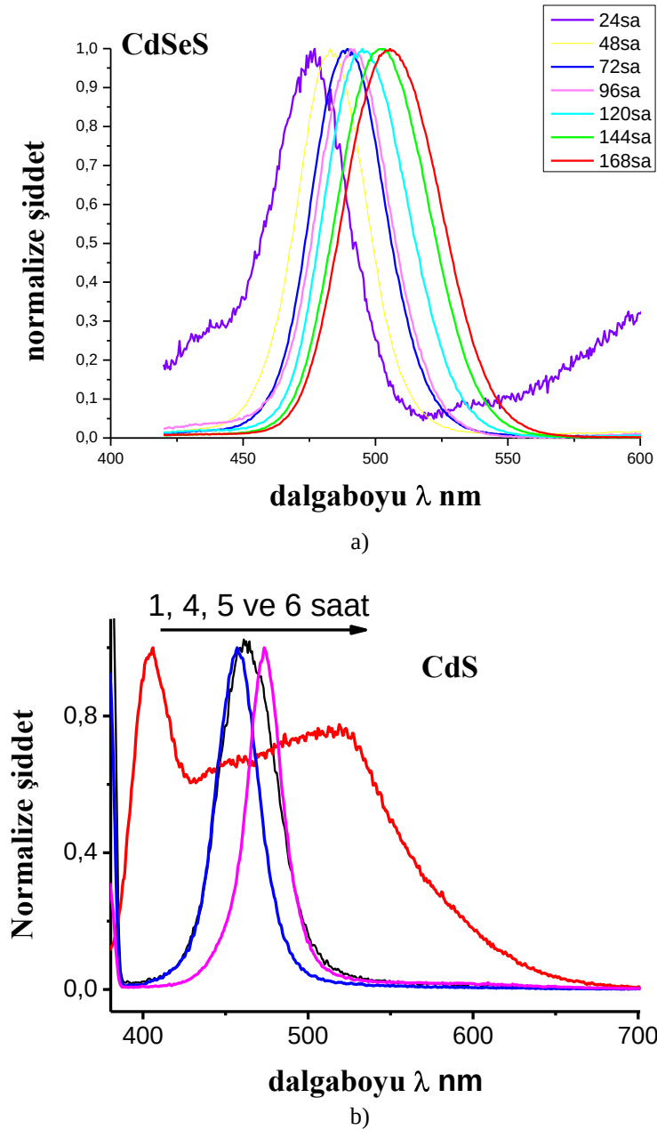
Şekil 3.2. CdSeS (a), CdS (b), , nanokristallerinin flüoresans spektrumları
