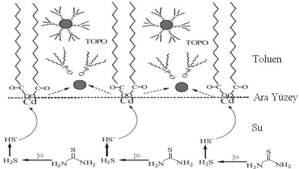
Şekil 1.14. Toluen-Su Ara yüzeyinde CdS Nanokristallerinin Oluşma Mekanizması (Pan ve ark 2005)
