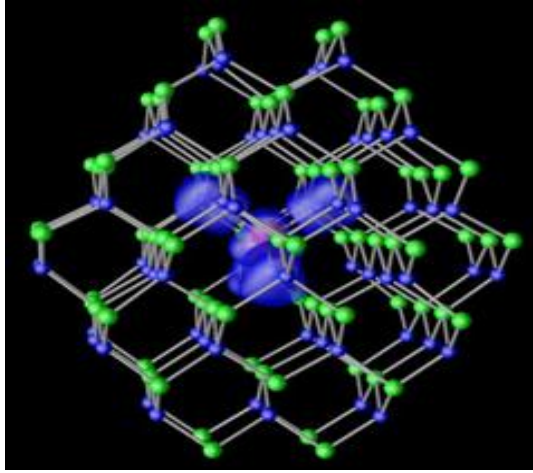
Şekil 1.2. Mangan'ın bir atomu ile CdSe'in 1.7 nm çaplı nanokristalinin görüntüsü (Yeşil: Cd, Mavi: Se) (Quantum dot corp.2003)
