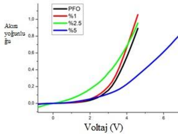
Şekil 3.11. PFO-CdSeS hibrid LED lerin Akım-Voltaj (I-V) karakteristikleri
