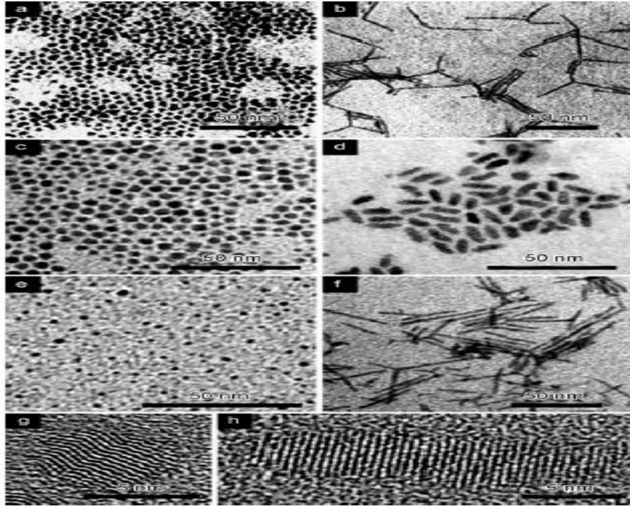
Şekil 1.12. Kalkojenitin değişik injeksiyon hızına bağlı parçacık büyüklüğü ve şekline dair TEM sonuçları (Shieh ve ark. 2005)
