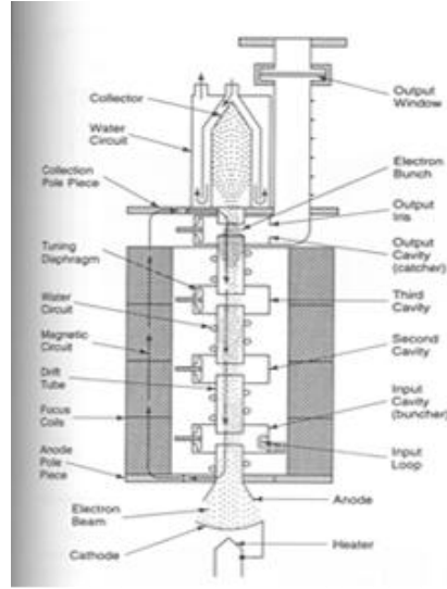
Şekil 2.12. : Klystron diyagramı
