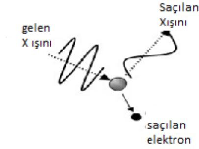
Şekil 2.6. Compton saçılmasının şematik gösterimi
