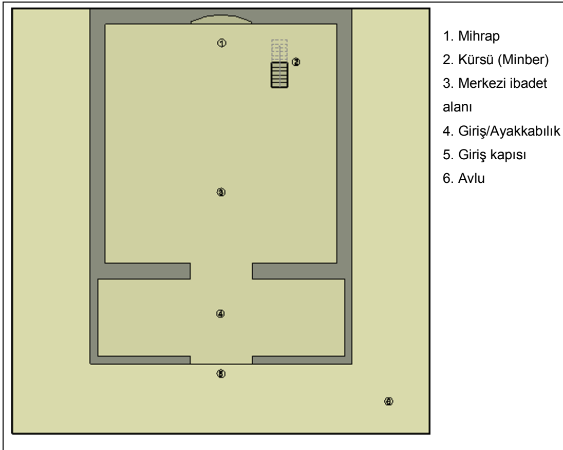
Görsel 25. Cami İç Mekân Plan Şeması
