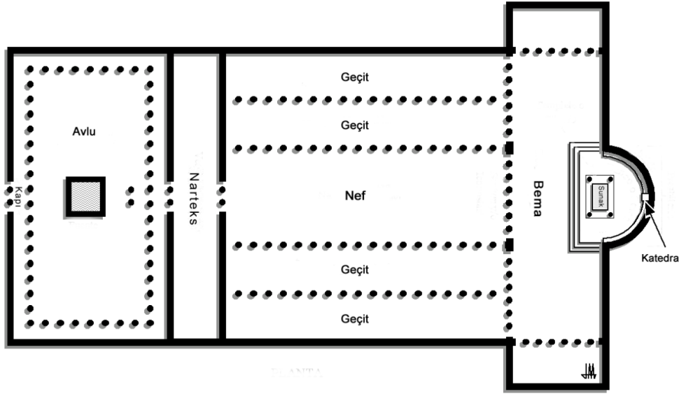
Görsel 14. Tarihi St Peter's Bazilikasının Planı
