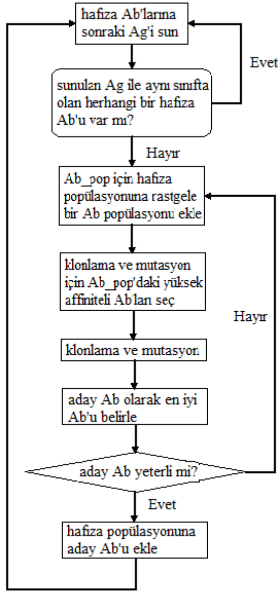
Şekil 5.2. Geliştirilen klonsal seçme tabanlı AIS' in akış diagramı
