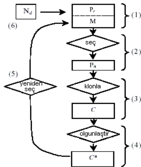
Şekil 4.4. Klonsal seçme algoritmasının blok diyagramı
