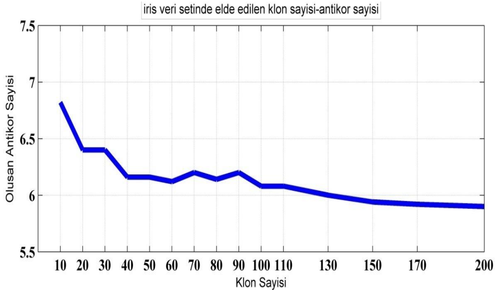
Şekil 6.5. İRİS veri setinden elde edilen klon sayısı- oluşan antikor sayısı ilişkisi
