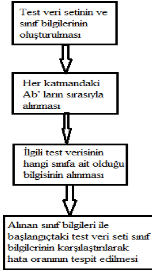
Şekil 5.7. Geliştirilen elipsoid şekilli katmanlı-YBS sisteminin test edilmesi için oluşturulan akış şeması
