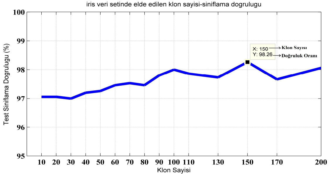
Şekil 6.1. İRIS veri setinden elde edilen klon sayısı- test sınıflama doğruluğu ilişkisi
