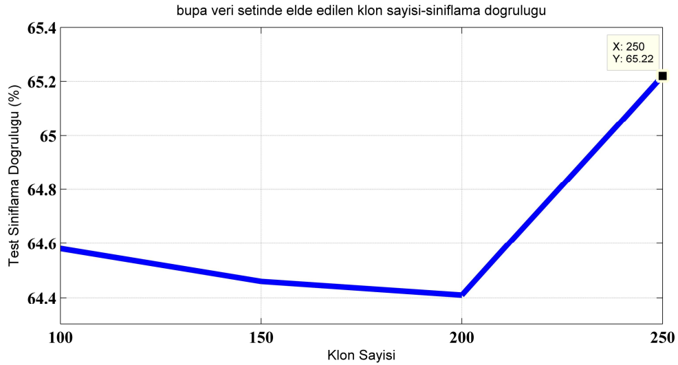
Şekil 6.6. BUPA liver disorders veri setinden elde edilen klon sayısı- test sınıflama doğruluğu ilişkisi
