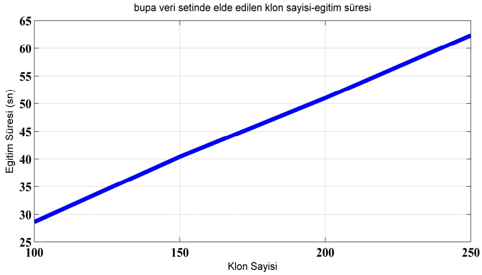
Şekil 6.8. BUPA liver disorders veri setinden elde edilen klon sayısı- eğitime süresi ilişkisi
