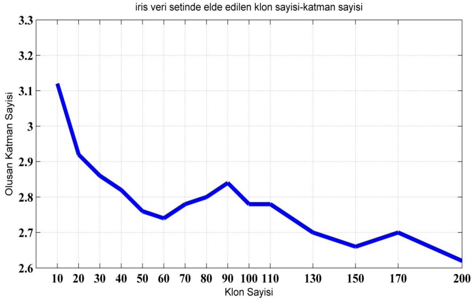
Şekil 6.4. İRİS veri setinden elde edilen klon sayısı- oluşan katman sayısı ilişkisi
