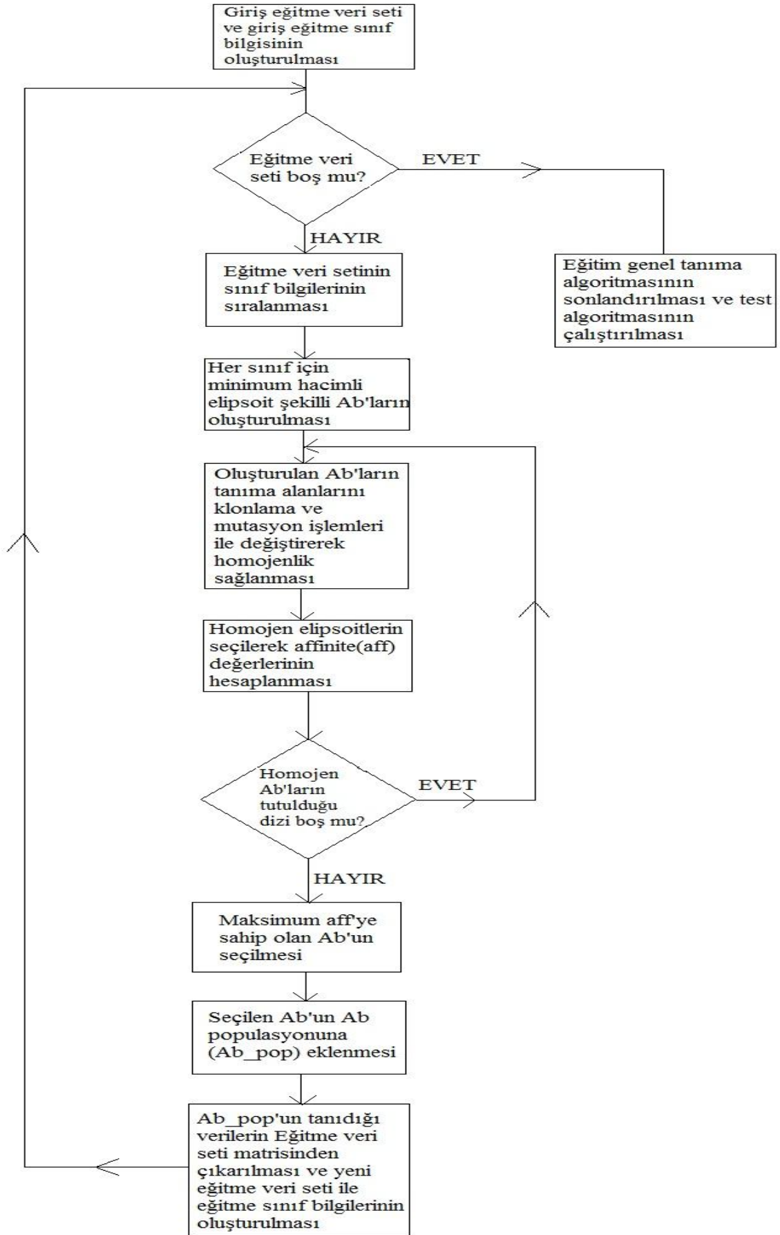
Şekil 5.6. Geliştirilen elipsoid şekilli katmanlı-YBS sisteminin akış şeması
