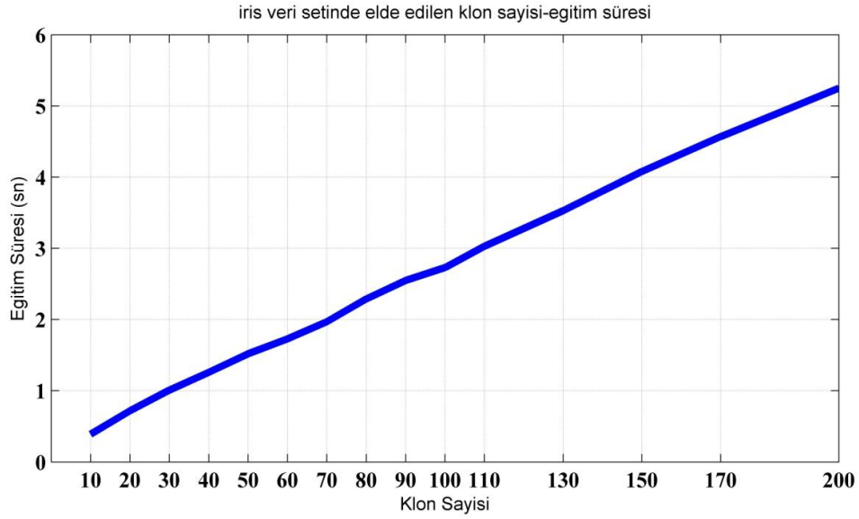
Şekil 6.3. İRİS veri setinden elde edilen klon sayısı- eğitim süresi ilişkisi
