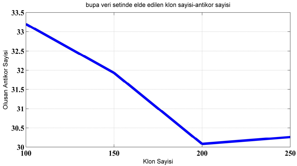
Şekil 6.10. BUPA liver disorders veri setinden elde edilen klon sayısı- oluşan antikor sayısı ilişkisi
