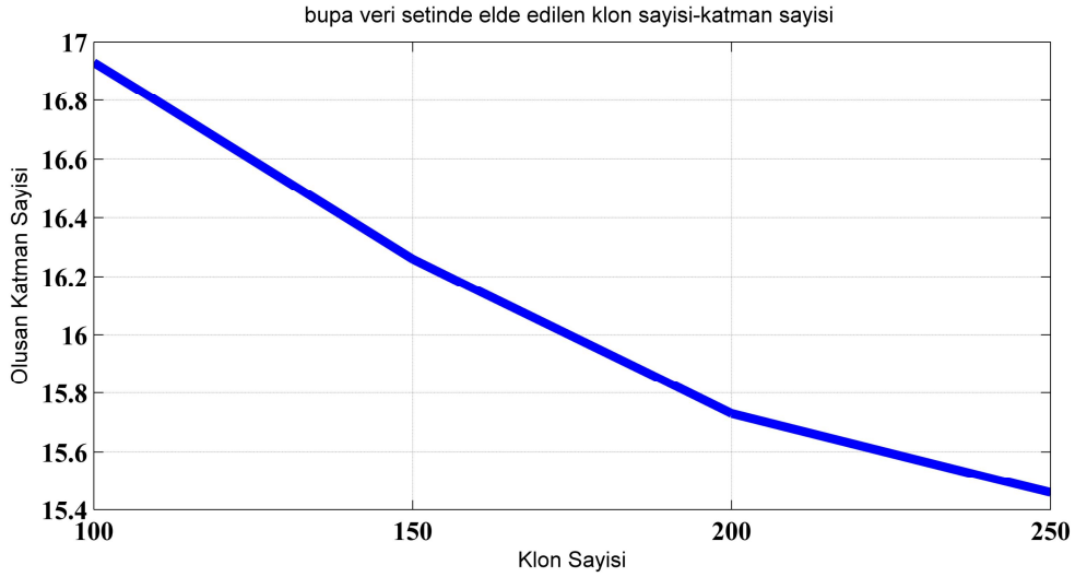
Şekil 6.9. BUPA liver disorders veri setinden elde edilen klon sayısı- oluşan katman sayısı ilişkisi
