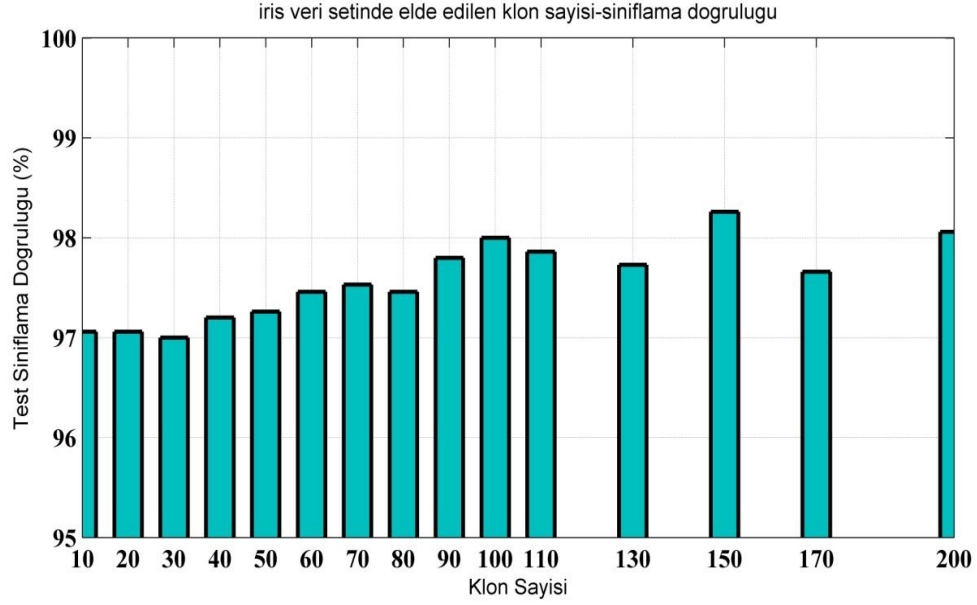
Şekil 6.2. İRİS veri setinden elde edilen klon sayısı- test sınıflama doğruluğu ilişkisi
