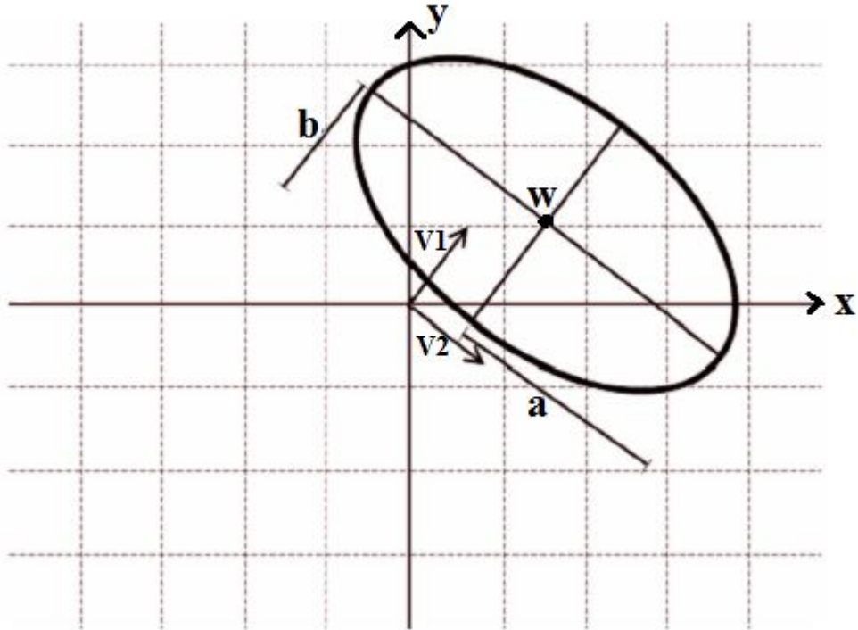
Şekil 5.1. Tanımlanan değişkenler ile döndürülmüş bir elipsin grafiksel gösterimi
