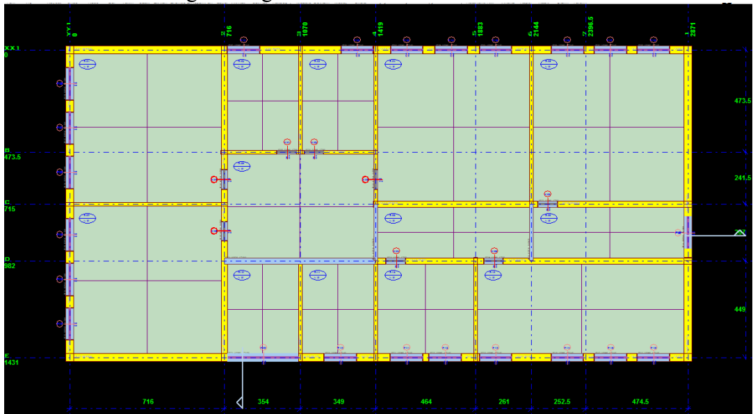
EK-11 StatiCAD-Y1gma Programında Birinci Kat Planı
