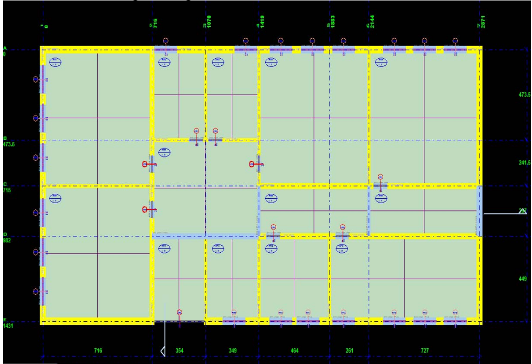
EK-10 StatiCAD-Y1gma Programında Zemin Kat Planı
