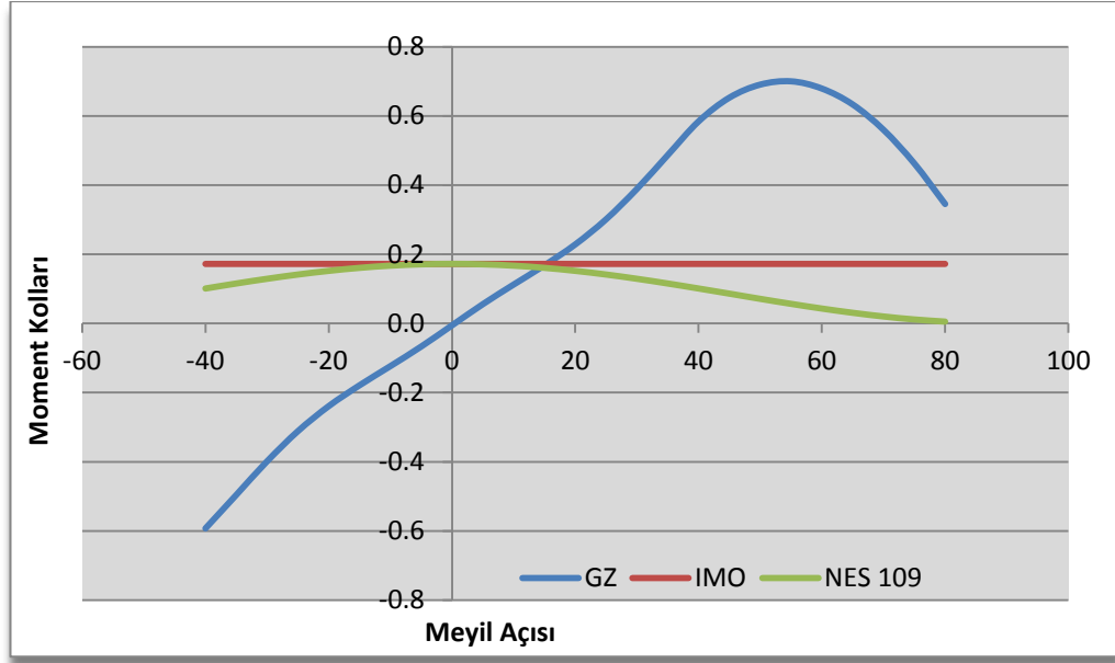
Şekil 9.7: Yatırıci moment kolunun NES 109'a göre meyil açısıyla değişimi.
