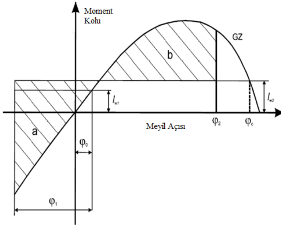
Şekil 7.1: Rus hava kriterinde kullanılan değerler [4].
