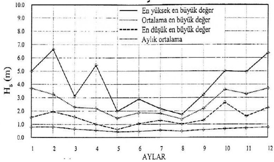
Şekil 9.2: Aylık ortalama ve en uç değer belirgin dalga yükseklikleri [14].
