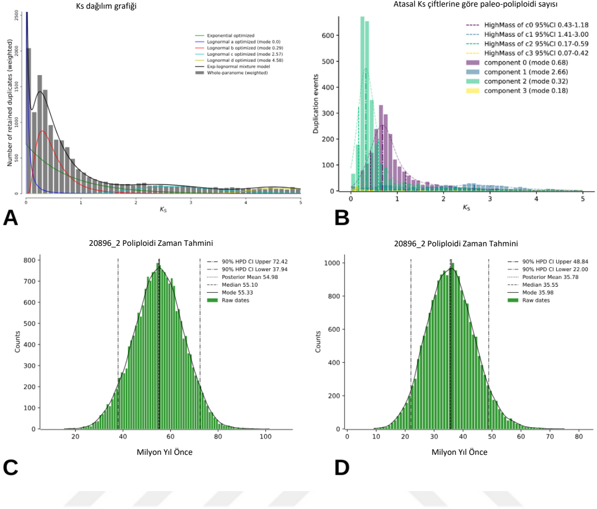
Şekil 3.11. AAD20896_2 numaralı bireye ait poliploidi analizleri. A. Ks değerini gösteren grafik. B. İki adet paleo-poliploidinin gerçekleştiğini gösteren grafik. C. İlk paleo-poliploidinin gerçekleşme zamanı. D. Son poliploidinin gerçekleşme zamanı.
