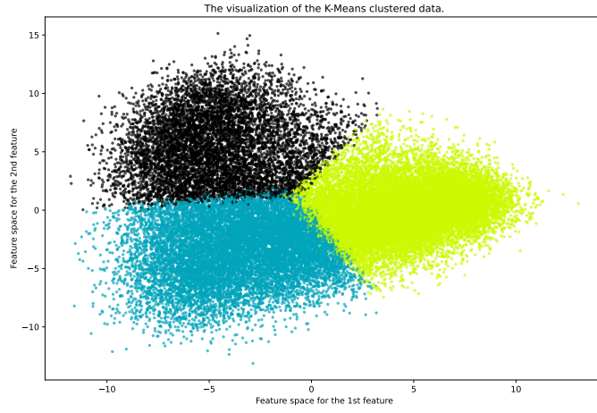
(a) PCA
