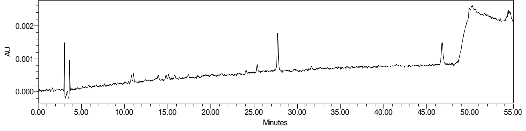
Şekil A.23 505I kodlu sosun 312 nm'deki kromatogramı
