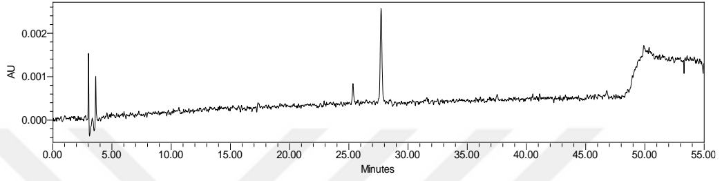
Şekil A.24 505I kodlu sosun 360 nm'deki kromatogramı
