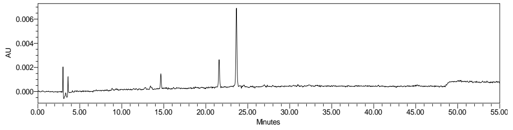
Şekil A.57 B5O5I kodlu sosun 360 nm'deki kromatogramı
