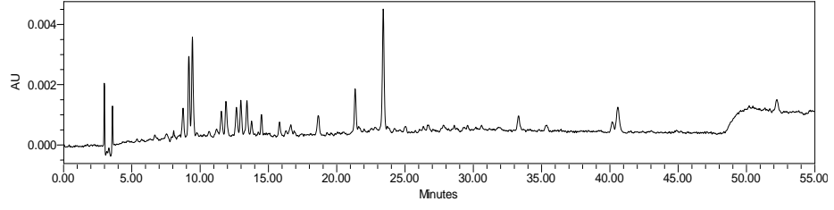
Şekil A.62 B10O5I kodlu sosun 312 nm'deki kromatogramı
