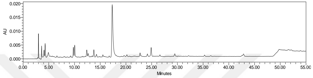
Şekil A.37 BIS kodlu sosun 280 nm'deki kromatogramı
