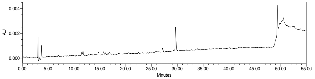
Şekil A.14 100 kodlu sosun 312 nm'deki kromatogramı
