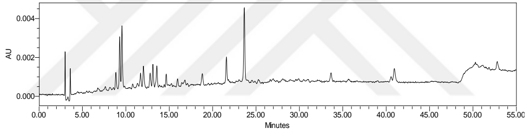
Şekil A. 56 B5O5I kodlu sosun 312 nm'deki kromatogramı
