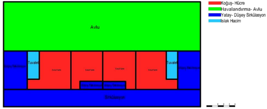
Şekil 3.9 Oda sistemine dönüştürülmüş E Tipi Kapalı Ceza İnfaz Kurumu kısmi 1. kat planı [118]
