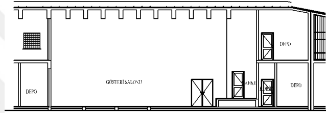
Şekil 5.6 Ceza infaz kurumu çok amaçlı salon kesiti
