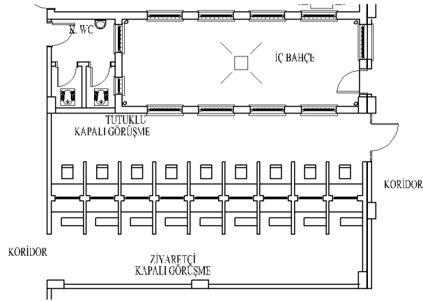
Şekil 5.10 Kapalı görüş alanı planı
