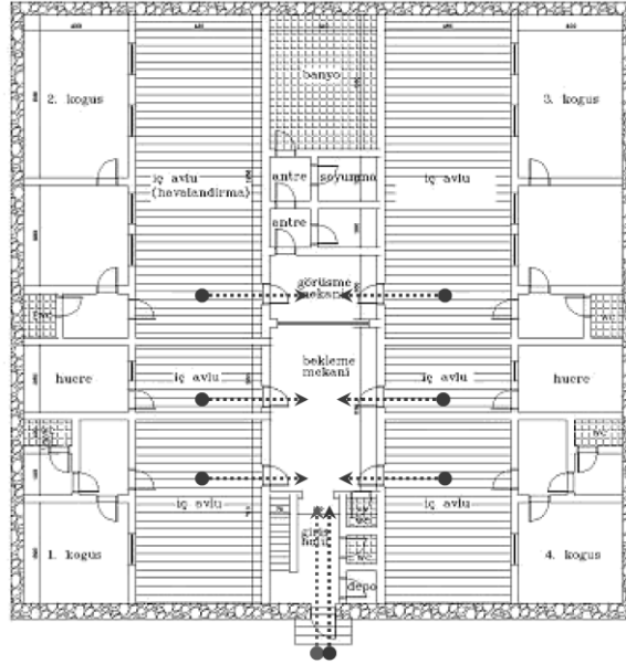
Şekil 2. 56 A2 Tipi Kapalı Ceza İnfaz Kurumu planı [118]
