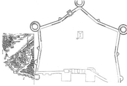
Şekil 2. 44 Yedikule Zindanları plan ve görünüşleri [103]
