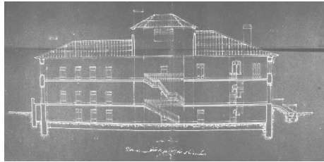
Şekil 2. 51 Üsküdar Paşakapısı Tevkifhanesi'ni gösteren bir kesit [112]
