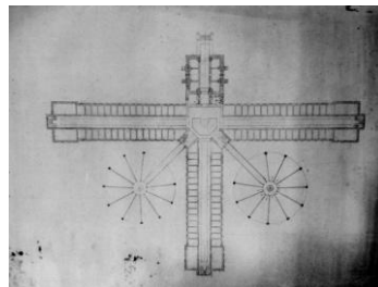
Şekil 2. 53 Mimar Kemaleddin ve Mimar Jasmund'un modern cezaevi tasarımı [115]
