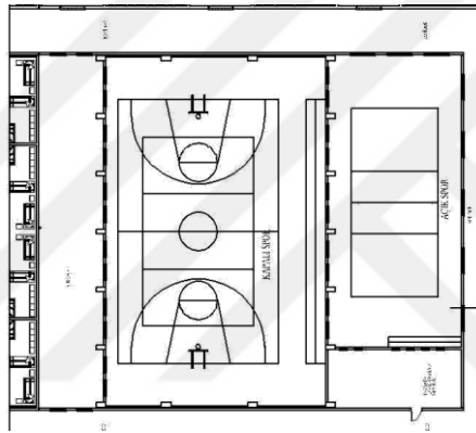
Şekil 5.5 Açık ve kapalı spor alanı planı
