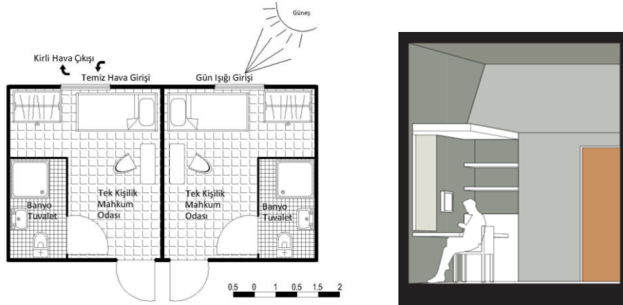
Şekil 4.11 Mahpus odası örneđi
