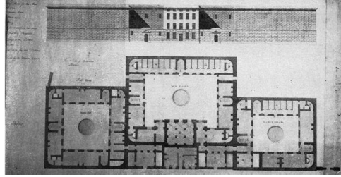
Şekil 2. 15 George Dance tasarımı Newgate Hapishanesi planı, 1768 [53]
