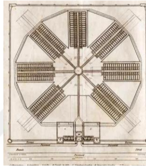
Şekil 2. 34 Merkezden dağılım, Pensilvanya Sistemi [84]
