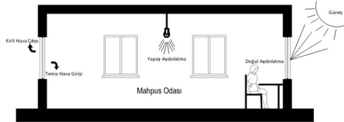
Şekil 5.1 Tek kişilik hükümlü odası
