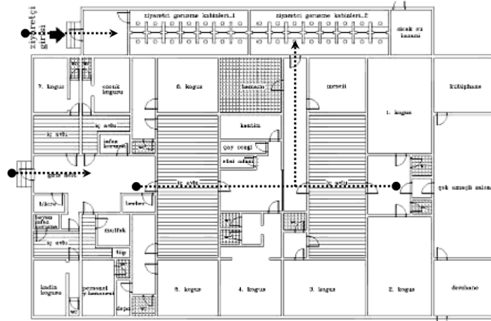
Şekil 2. 58 B Tipi Kapalı Ceza İnfaz Kurumu planı [118]
