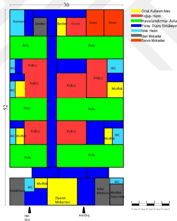
Şekil 3.12 K2 Tipi Kapalı Ceza İnfaz Kurumu krokisi [121]
