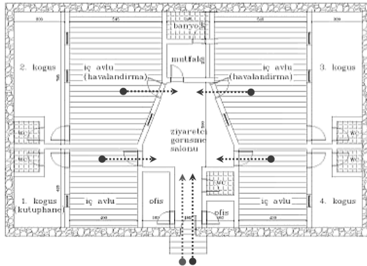
Şekil 2. 54 A Tipi Kapalı Ceza İnfaz Kurumu planı [118]
