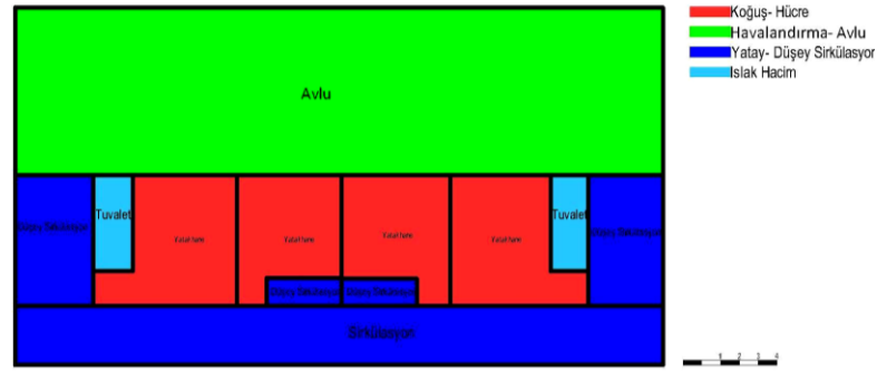
Şekil 2. 65 E Tipi Ceza İnfaz Kurumu kısmi birinci kat planı (oda sistemine dönüştürülmüş hali) [121]
