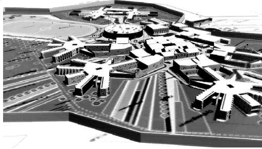
Şekil 2. 37 Vridsløsselille'de Danimarka Devlet Hapishanesi yıldız sistemi tasarımı [87]
