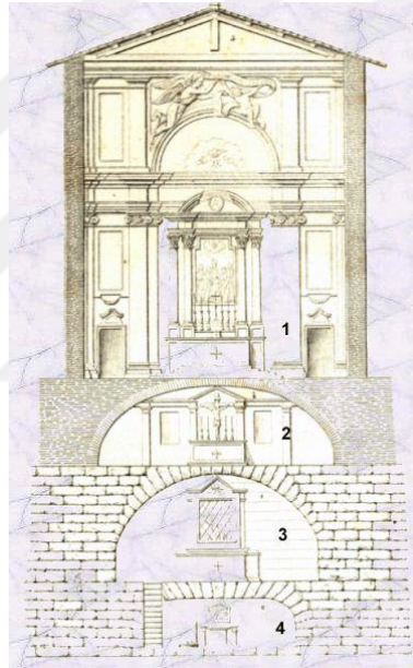
Şekil 2. 2 Antik Roma Mamertime Cezaevi kesiti [29]
