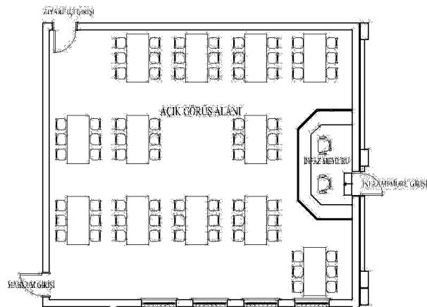
Şekil 5.11 Açık görüş alanı planı
