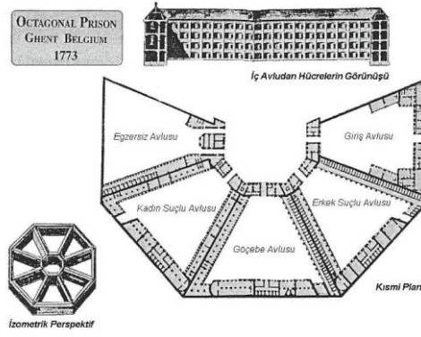
Şekil 2. 12 Belçika Gand (Ghent) Cezaevi kısmi plan ve görünüşü, 1773 [16]
