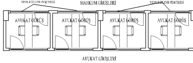
Şekil 5.12 Avukat görüşme mekânları
