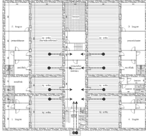
Şekil 2. 57 A3 Tipi Kapalı Ceza İnfaz Kurumu planı [118]
