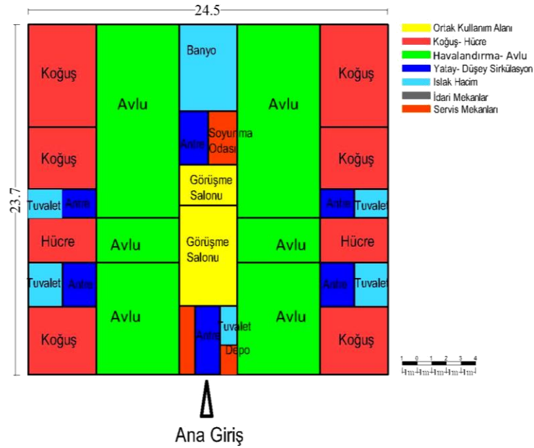
Şekil 3.4 A2 Tipi Ceza İnfaz Kurumu şematik gösterimi [121]
