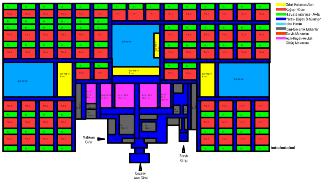
Şekil 3.15 L Tipi Kapalı Ceza İnfaz Kurumu şematik gösterimi [121]
