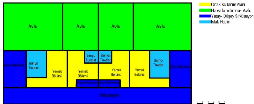
Şekil 3. 8 Oda sistemine dönüştürülmüş E Tipi Kapalı Ceza İnfaz Kurumu kısmi zemin kat planı [32]
