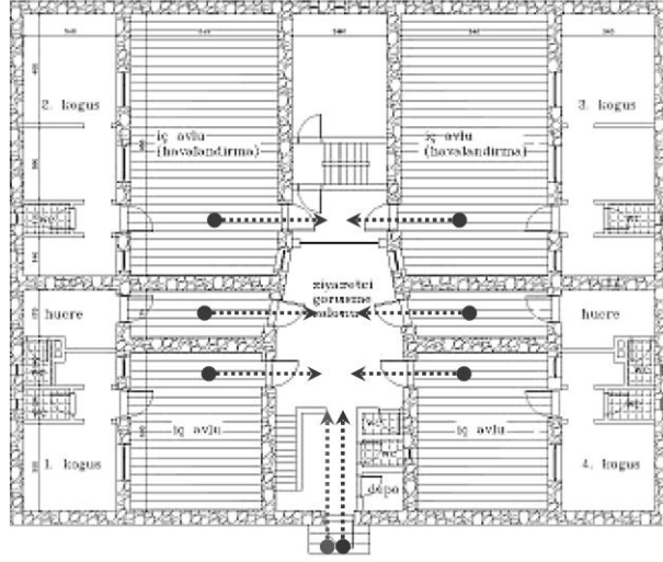
Şekil 2. 55 A1 Tipi Kapalı Ceza İnfaz Kurumu planı [118]
