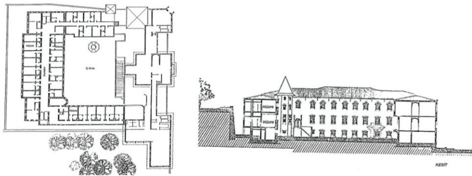
Şekil 2. 52 Sultanahmet Cezaevi plan ve görünüşü [114]
