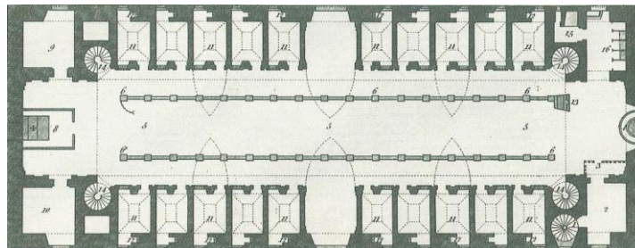
Şekil 2. 10 St. Michael's Hapishanesi planı [28]
