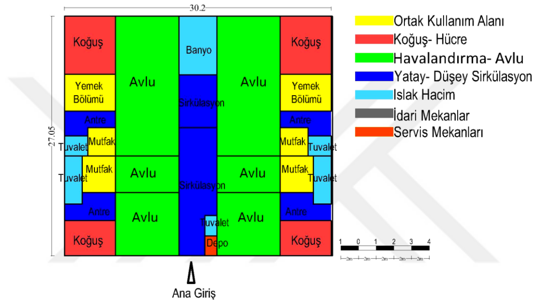
Şekil 3.5 A3 Tipi Ceza İnfaz Kurumu kat planı [121]
