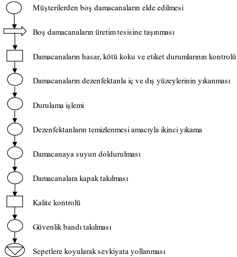
Şekil 2.5. Damacana Su Üretim Süreci Kaynak: Kutlu ve Kağncioğlu, 2015, s.1281
