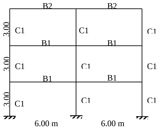
Figure D.1 Frame F1-3S2B
