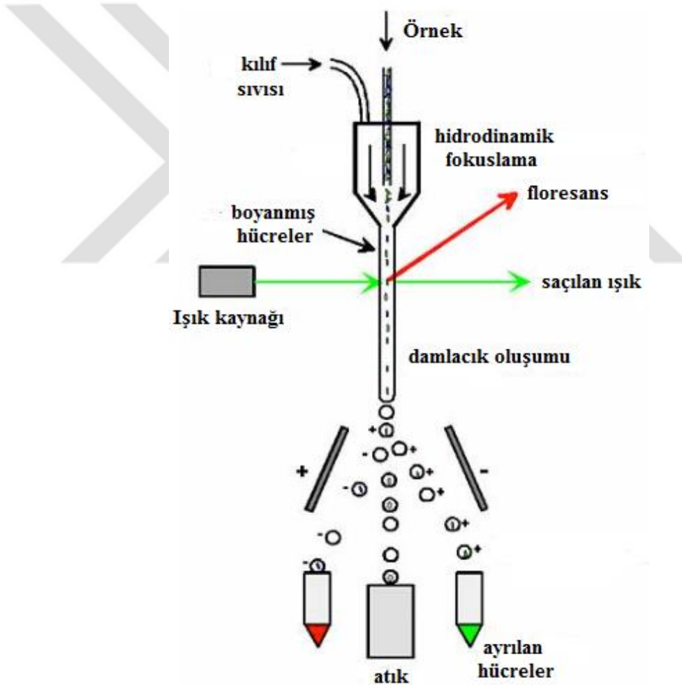
Şekil 2.12. Akan hücre ölçer çalışma prensibi (83).
