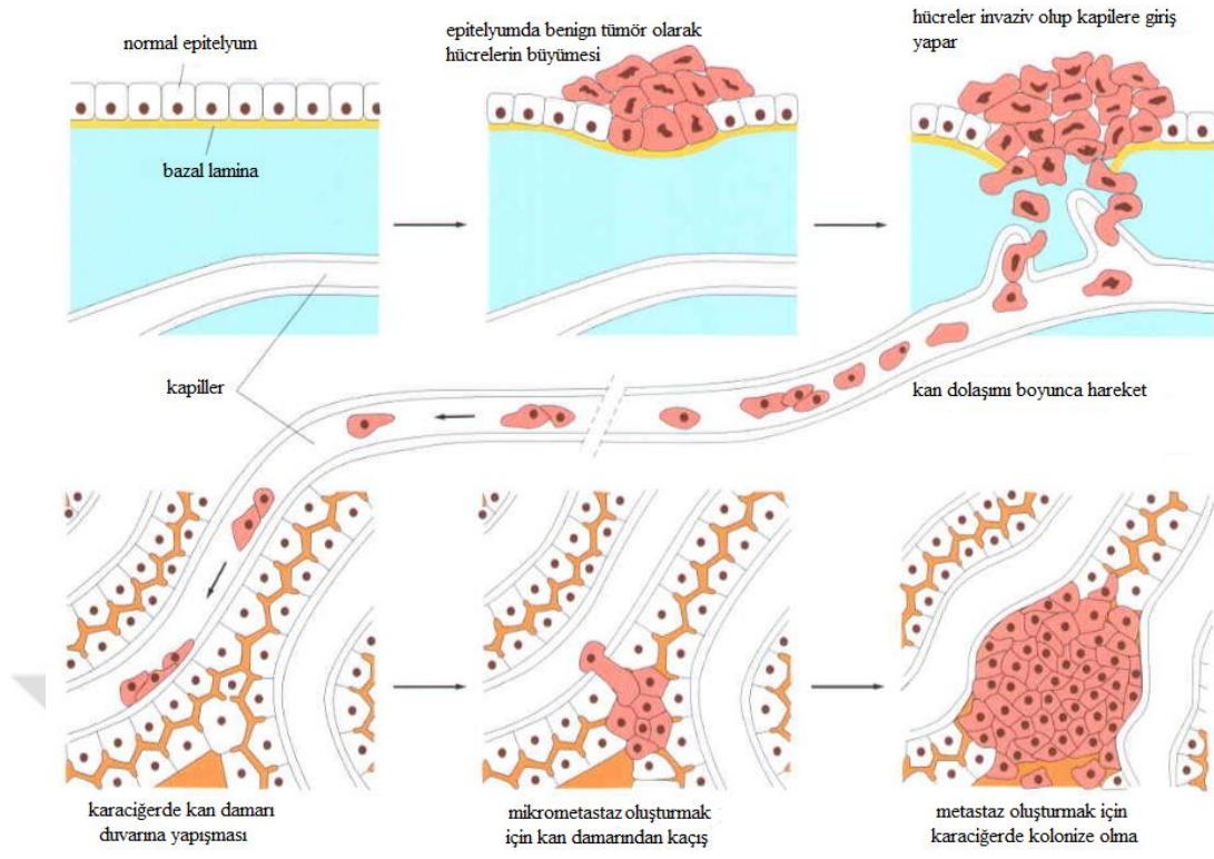
Şekil 2.7. Metastaz basamakları (19).
