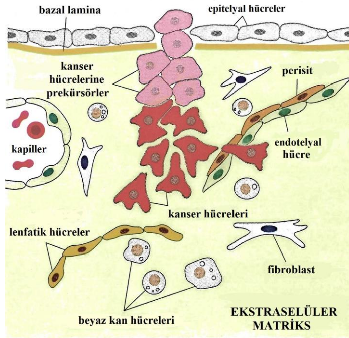
Şekil 2.4. Mikroçevre elemanları (19).
