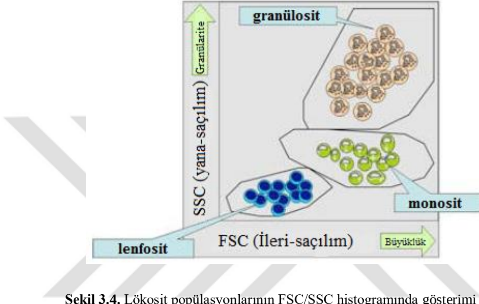
Şekil 3.4. Lökosit popülasyonlarının FSC/SSC histogramında gösterimi (87).
