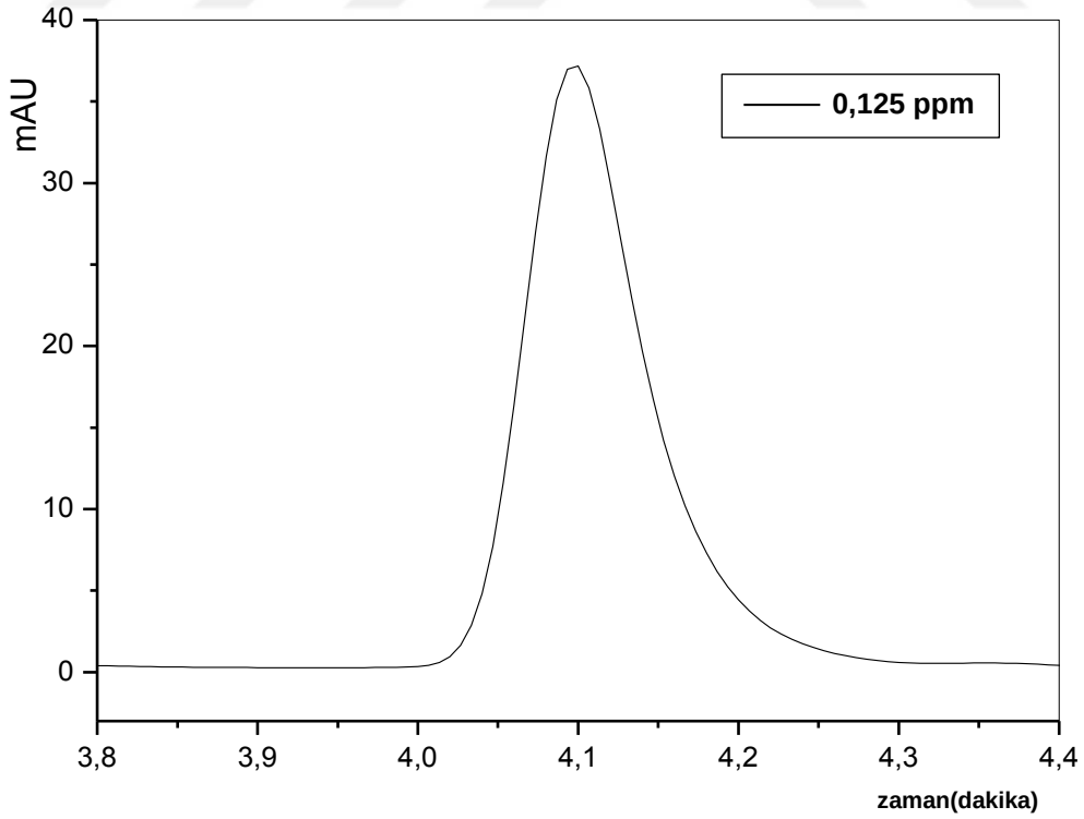
Şekil 4.11. 0,125 ppm NDPhA için HPLC kromatogramı (500 mL NDPhA standardı AT 280 oto deriştirici ile 5 mL'ye deriştirilmiştir, 100 kat deriştirme).
