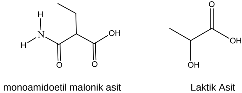
Şekil 4.51. 2 ppm NDPhA’nın 2,21 kGy ışınlanması sonucu gözlenen ara ürünler. (Ara ürünler TMS esteri olarak gözlenmiştir.)
