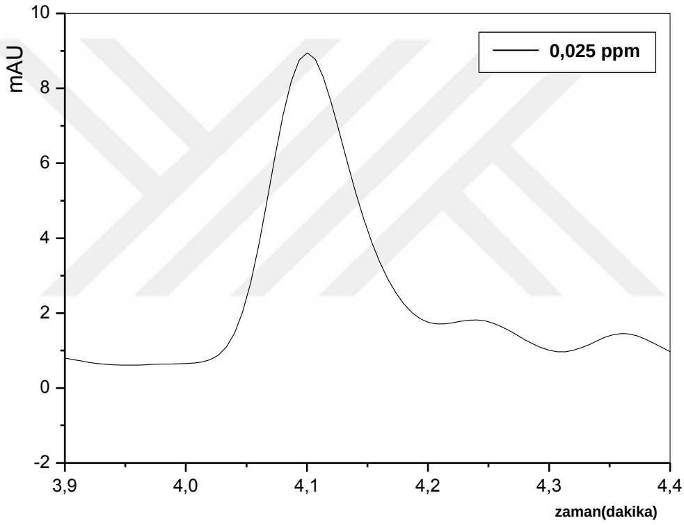
Şekil 4.9. 0,025 ppm NDPhA için HPLC kromatogramı (500 mL NDPhA standartı AT 280 oto deriştirici ile 5 mL'ye deriştirilmiştir, 100 kat deriştirme).
