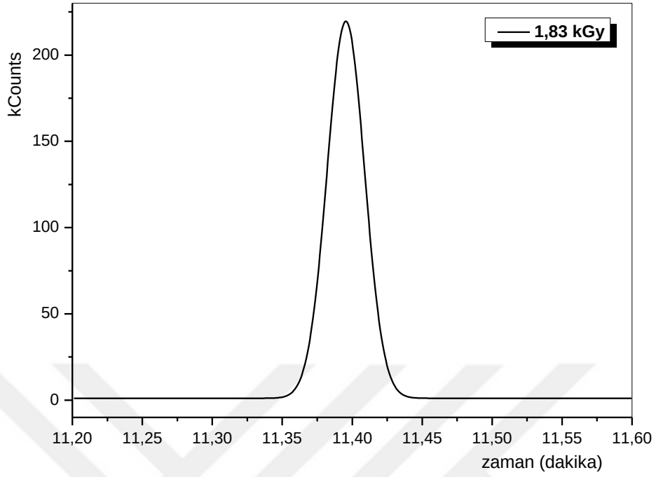
Şekil 4.45. 2 ppm sulu NDPhA'nın 1,83 kGy ışınlaması sonucu gözlenen ara ürün gaz kromatogramı (11,38 ve 11,40 dakika).
