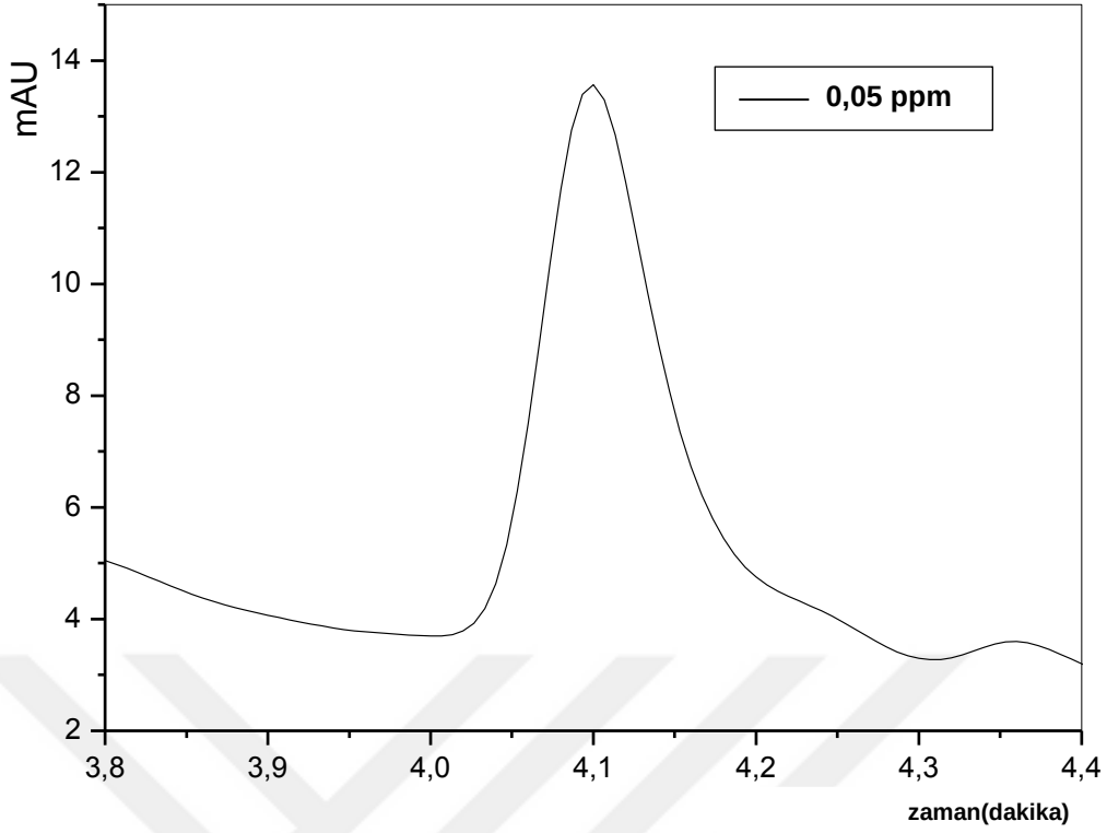
Şekil 4.10. 0,05 ppm NDPhA için HPLC kromatogramı (500 mL NDPhA standardı AT 280 oto deriştirici ile 5 mL'ye deriştirilmiştir, 100 kat deriştirme).
