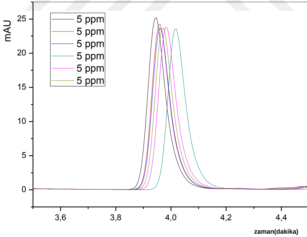
Şekil 4.8. 5 ppm NDPhA için HPLC kromatogramları (Mobil faz ACN/Su oranı (%v/v) %80/%20 ve metil alkol içinde hazırlanmış standartlar).
