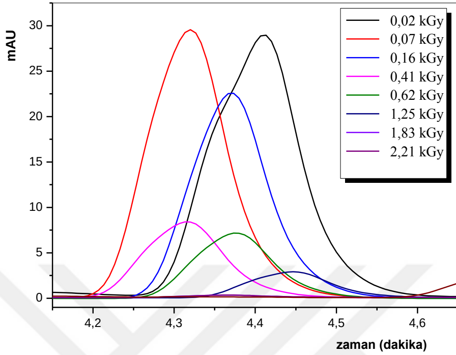
Şekil 4.36. 2 ppm sulu NDPhA için HPLC kromatogramlarının ışınlama dozu ile değişimi (7,5 kat deriştirme).
