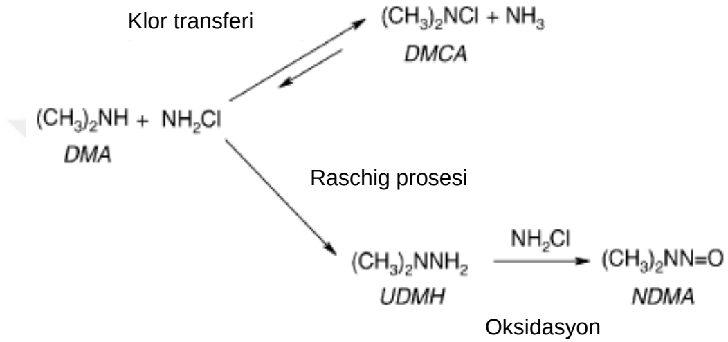
Şekil 2.8. DMA ve monokloramin varlığında NDMA için önerilen oluşum reaksiyonu [30].
