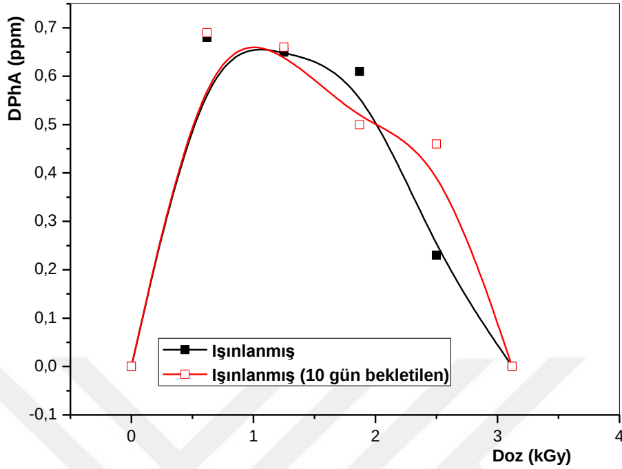
Şekil 4.34. 2 ppm NDPhA çözeltilerinin ışınlaması sonucu oluşan ara ürün DPhA miktarının ışınlama dozu ile değişimi.
