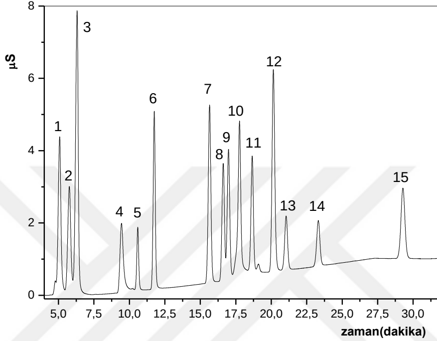
Şekil 4.54. NDPhA'nın ışınlama ile bozunma sonrası oluşabilecek olası ara ürünler için iyon kromatogramı; 1: asetik asit, 2: formik asit, 3: propiyonik asit 4: valerik asit, 5: c,t-mukonik asit: 6: nitrit, 7: nitrat, 8: glutarik asit 9: süksinik asit, 10: malonik asit, 11: maleik asit, 12: okzalik asit, 13: c,c-mukonik asit, 14: t,t-mukonik asit, 15: sitrik asit. (Bütün bileşiklerin derişimi 3 ppm).
