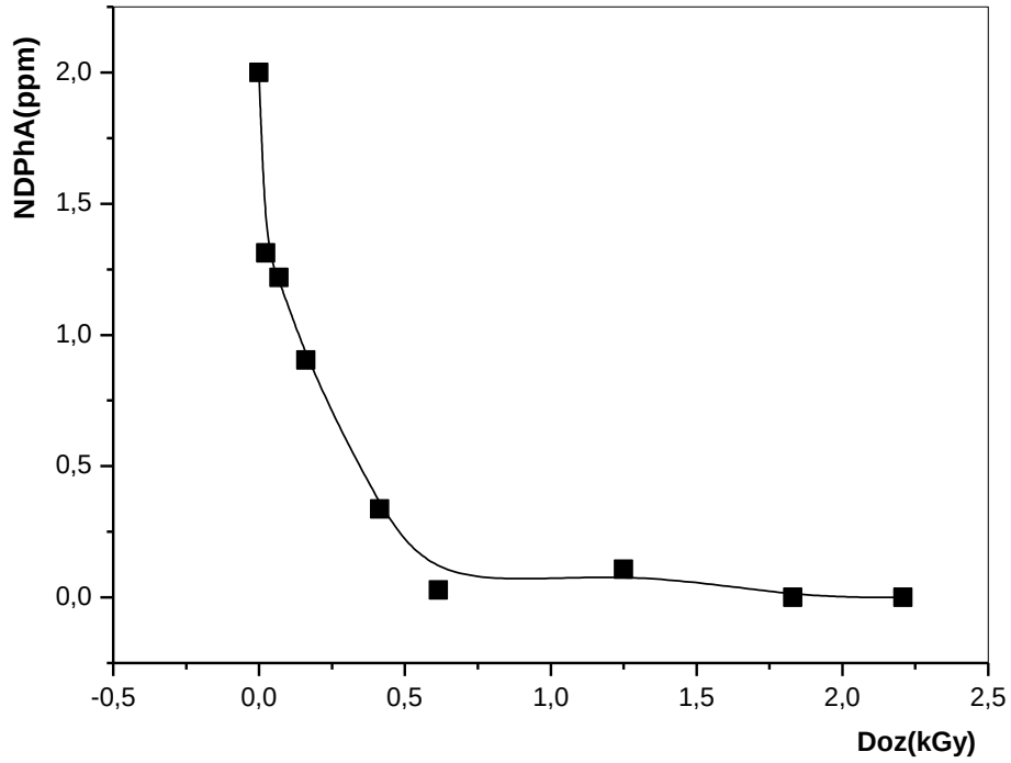
Şekil 4.37. 2 ppm sulu NDPhA miktarının ışınlama dozu ile değişimi.
