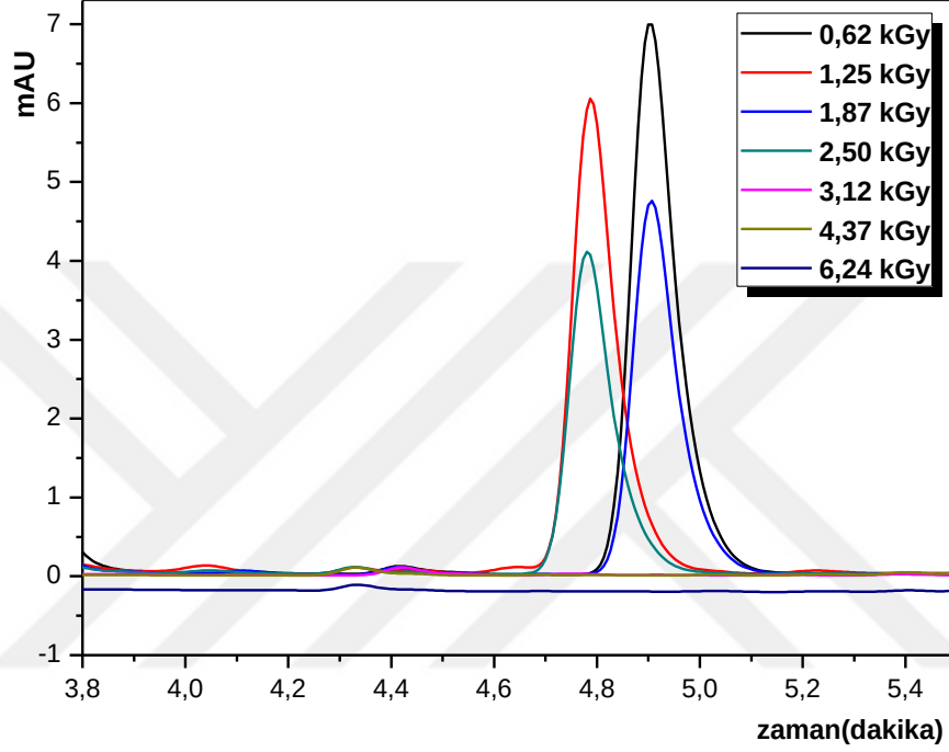
Şekil 4.33. C18 kartuşundan geçirilen ışınlanmış sulu 2 ppm NDPhA (ışınlandıktan sonra 10 gün kapalı bir şişede ve karanlık ortamda bekletilmiş) için HPLC kromatogramı (50 kat deriştirme, Mobil faz: ACN/Su oranı (%v/v) %80/%20).
