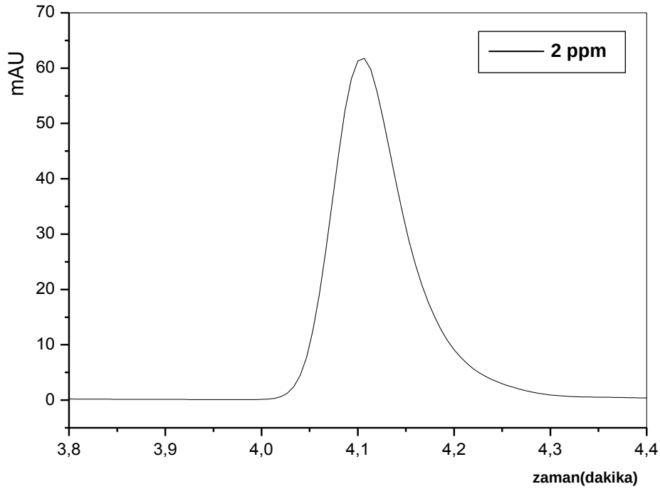
Şekil 4.15. 2 ppm NDPhA için HPLC kromatogramı (500 mL NDPhA standartı AT 280 oto deriştirici ile 5 mL'ye deriştirilmiştir, 100 kat deriştirme. NDPhA bu durumda çok derişik olduđu için metil alkol ile deriştirme oranı 10 kata düşürölmüşür.).
