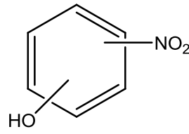
Şekil 4.47. 2 ppm NDPhA'nın 1,83 kGy ışınlanması sonucu gözlenen ara ürünler. (Ara ürünler TMS esteri olarak ve verilen bileşiklerin izomerleri olarak gözlenmiştir.)
