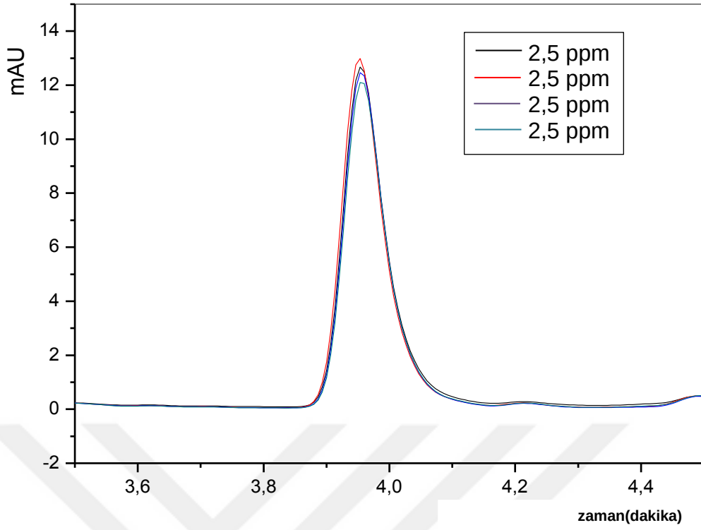
Şekil 4.7. 2,5 ppm NDPhA için HPLC kromatogramları (Mobil faz ACN/Su oranı (%v/v) %80/%20 ve metil alkol içinde hazırlanmış standartlar).
