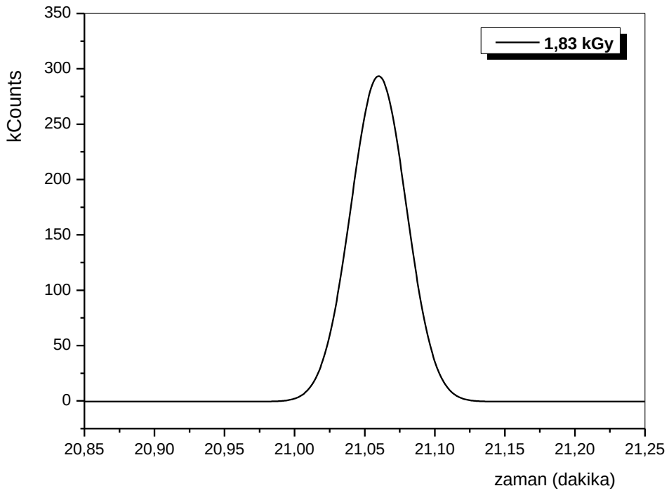
Şekil 4.46. 2 ppm sulu NDPhA'nın 1,83 kGy ışınlaması sonucu gözlenen ara ürün gaz kromatogramı (21,05 ve 21,08 dakika).
