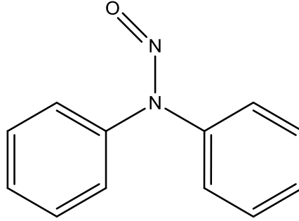
Şekil 2.9. N-nitrozodifenilamin kimyasal yapısı.
