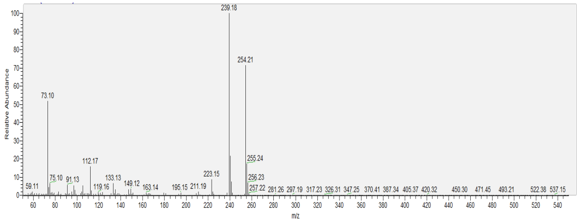
Şekil 4.48. 2 ppm NDPhA'nın 1,83 kGy ışınlanması sonucu gözlenen ara ürüne ait kütle spektrumu. (Alıkonma süresi: 11,38, Resorsinol).
