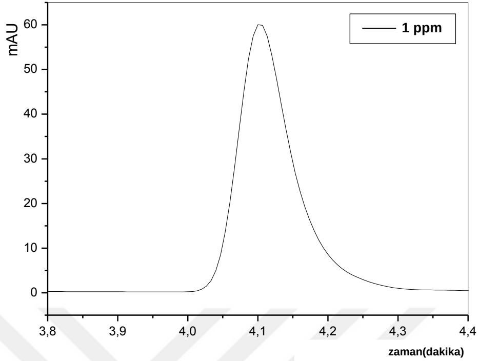
Şekil 4.14. 1 ppm NDPhA için HPLC kromatogramı (500 mL NDPhA standartı AT 280 oto deriştirici ile 5 mL'ye deriştirilmiştir, 100 kat deriştirme. NDPhA bu durumda çok derişik olduđu için metil alkol ile deriştirme oranı 20 kata düşürölmüşür.).
