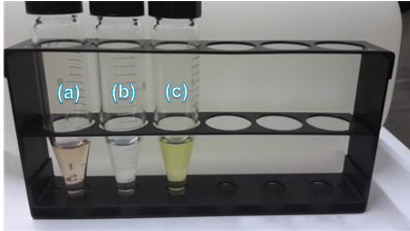
Şekil 4.31. C18 kartuş ile sudan diklorometan fazına geçirilmiş (a) 1,74 kGy ışınlanmış NDPhA (10 gün karanlıkta ve ağzı kapalı bekletilen), (b) 1,74 kGy ışınlanmış NDPhA (bekletilmeyen), (c) ışınlanmamış NDPhA örneklerinin görüntüsü.
