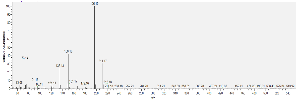
Şekil 4.49. 2 ppm NDPhA'nın 1,83 kGy ışınlanması sonucu gözlenen ara ürüne ait kütle spektrumu (Alıkonma süresi: 21,05, p-nitro fenol).
