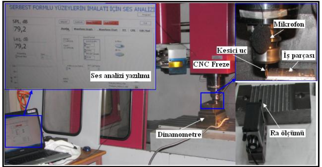
Şekil III.1 Deney düzeneęi
