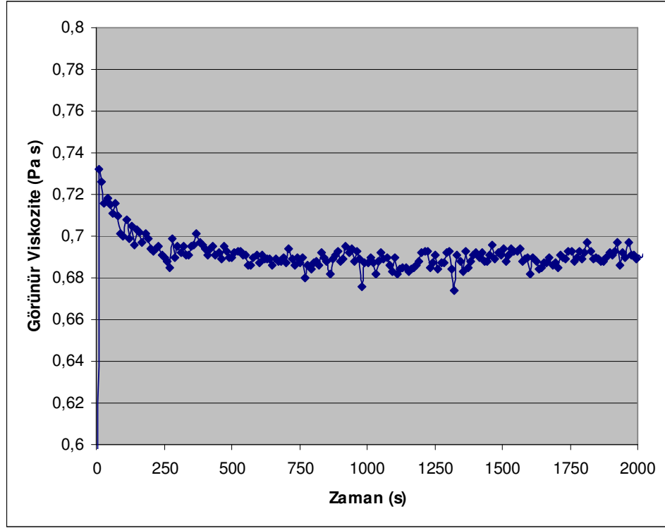
Şekil 5.16: Ayva püresinin %14 konsantrasyon, pH 3,5, 25 °C ve 100 \text{ s}^{-1} sabit kayma hızında görünür viskozite eğrisi
