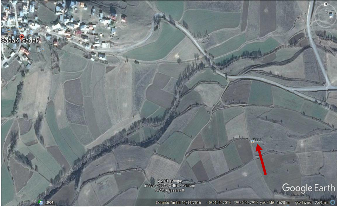
Fig.280 Satala kenti (Google earth görünümü).
