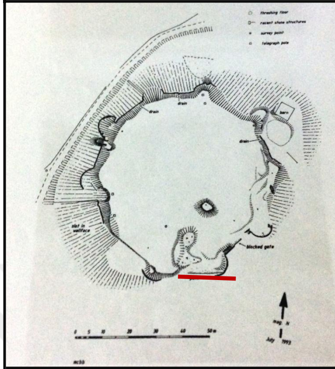
Fig.270 Hortokop Kalesi'nin planı.
