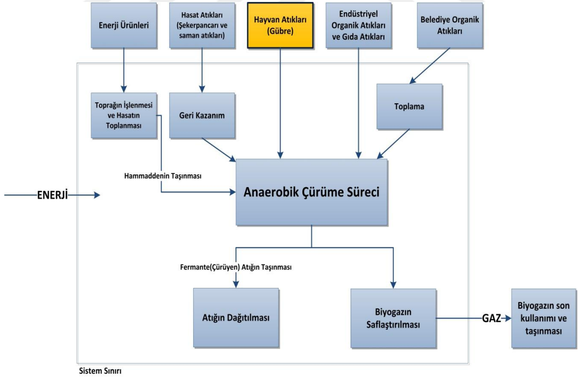
Şekil 2. 1: Biyogaz Üretim Sisteminde Hammadde ve Enerji Akışları Diyagramı (Berglund ve Börjesson 2006)
