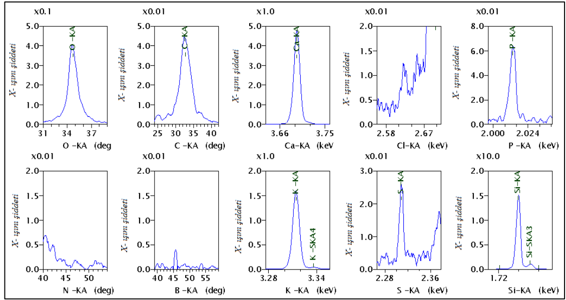
A8 numunesi için XRF analizi sonucu elde edilen X-ışını spektrumu.
