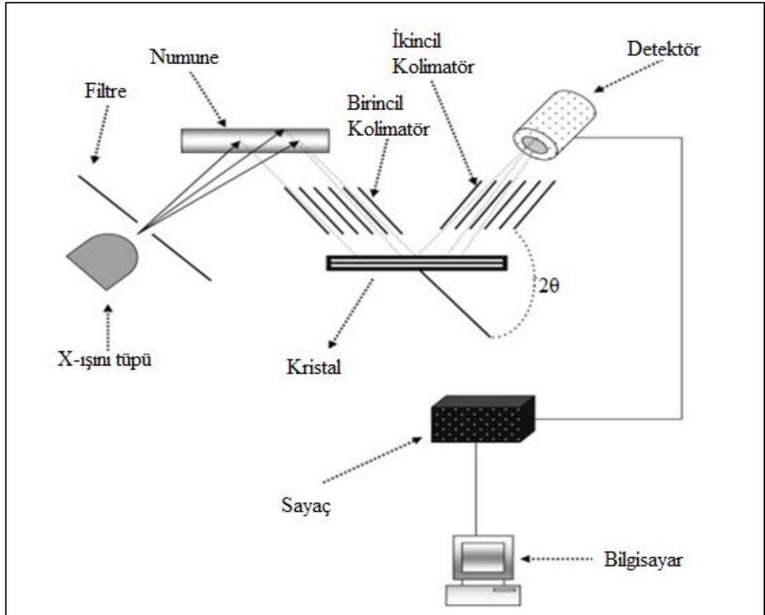
Şekil 1. WDXRF cihazı ve sistemin şematik gösterimi
