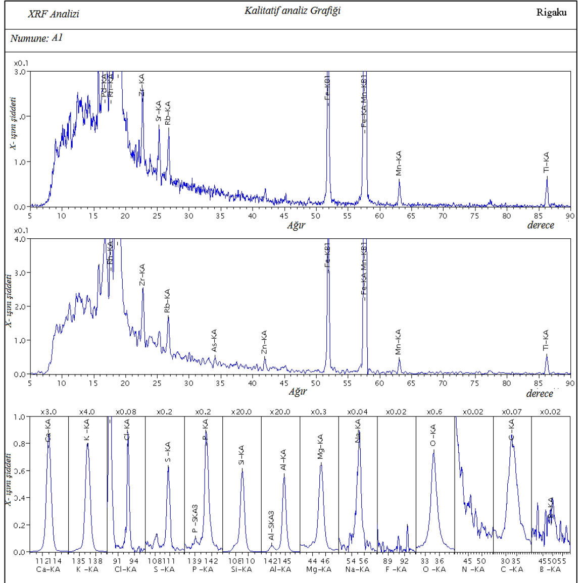
A1 numunesi için XRF analizi sonucu elde edilen X-ışını spektrumu.
