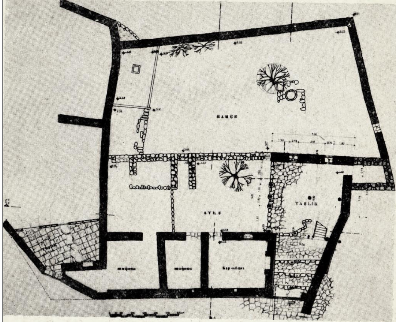
2 — Konağın rölöve plânı (Zemin Kat).
