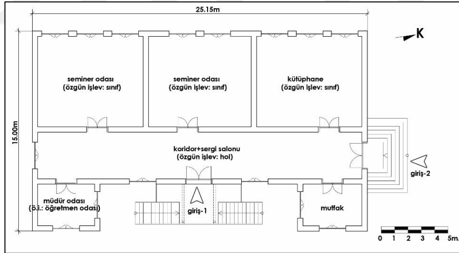
Şekil 3. 34 Taş Mektep, plan krokisi [E. Alyakut, 2017]
