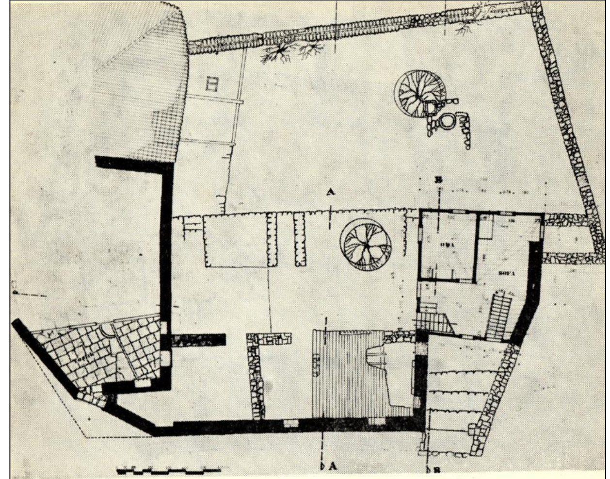
3 — Konağın rölöve plânı (Birinci kat).
