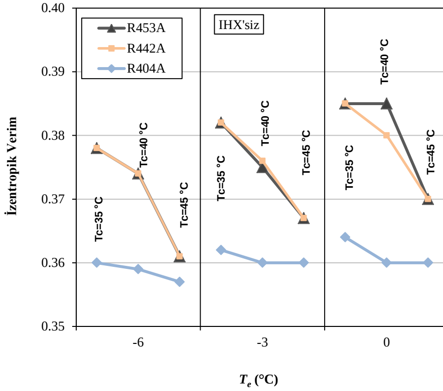
Şekil 4.19. IHX'siz sistemde izentropik verimin T_e ve T_c sıcaklıkları ile değişimi
