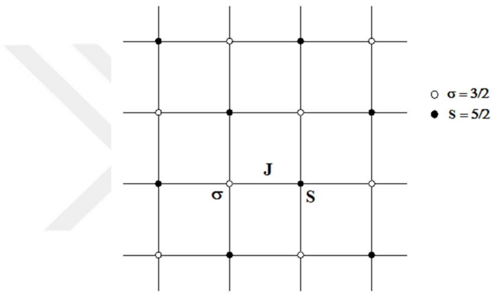
Şekil 1.1 İki iç içe geçmiş kare örgü üzerindeki spin düzenlemesinin taslağı. Örgü A (içi boş daireler) ve B ( içi dolu daireler) spinlerin örgüleri tarafından oluşturulmuştur.
