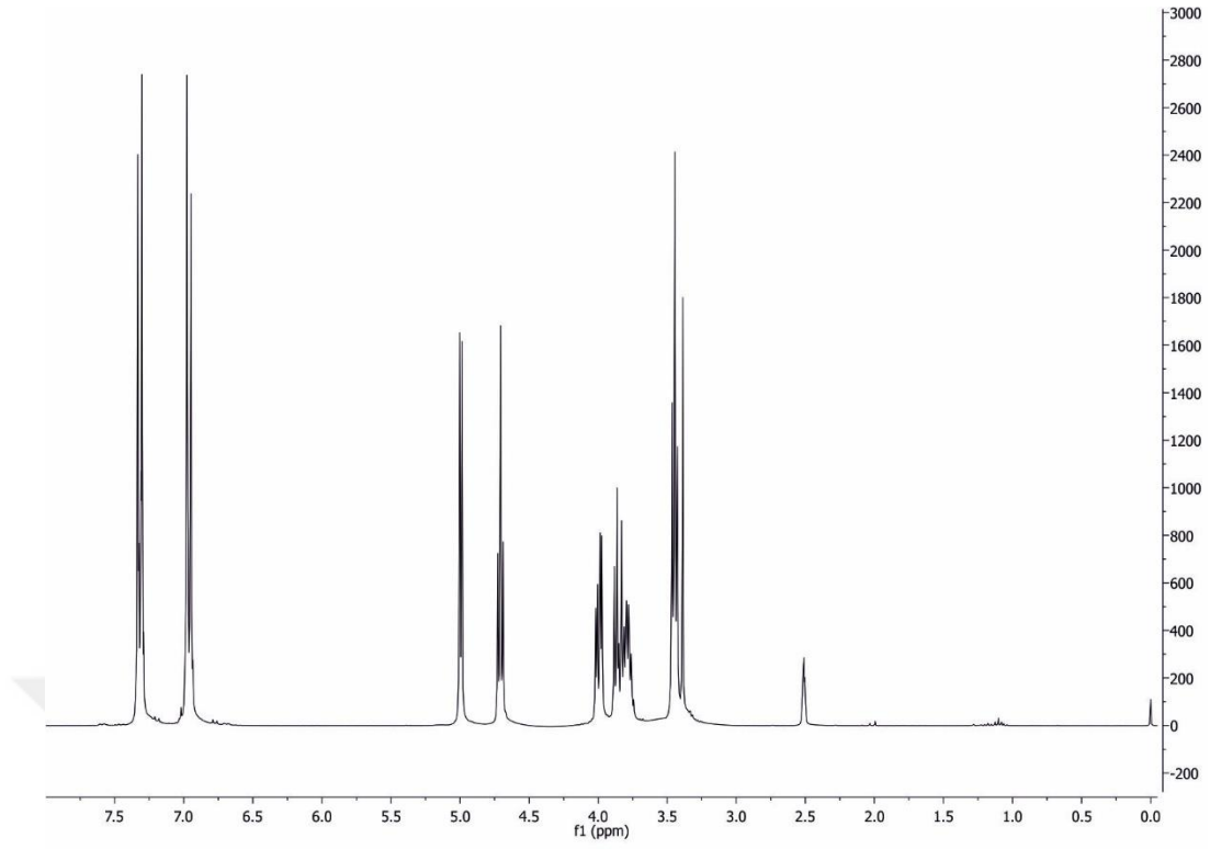
Şekil 4.1.7.a. 3-(4-klorfenoksi)propan-1,2-diolün ^1\text{H} NMR spektrumu
