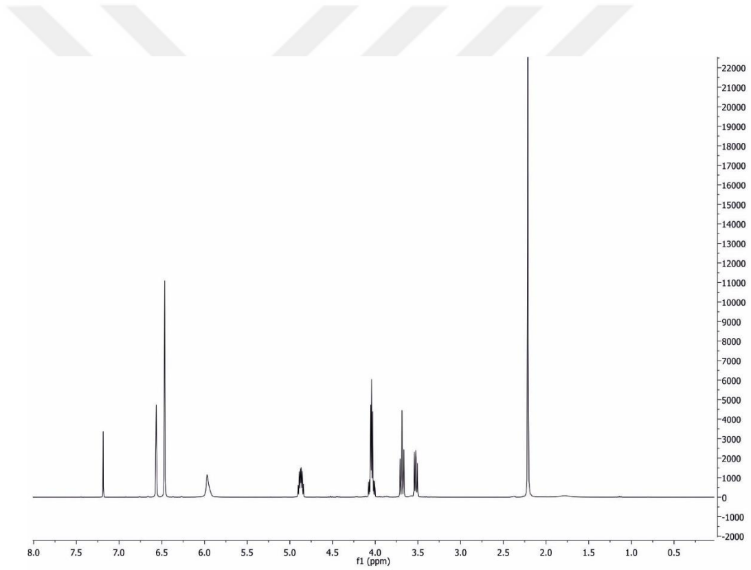
Şekil 4.2.1.a. 5-((3,5-dimetilfenoksi)metil)oksazolidin-2-onun ^1\text{H} NMR spektrumu
