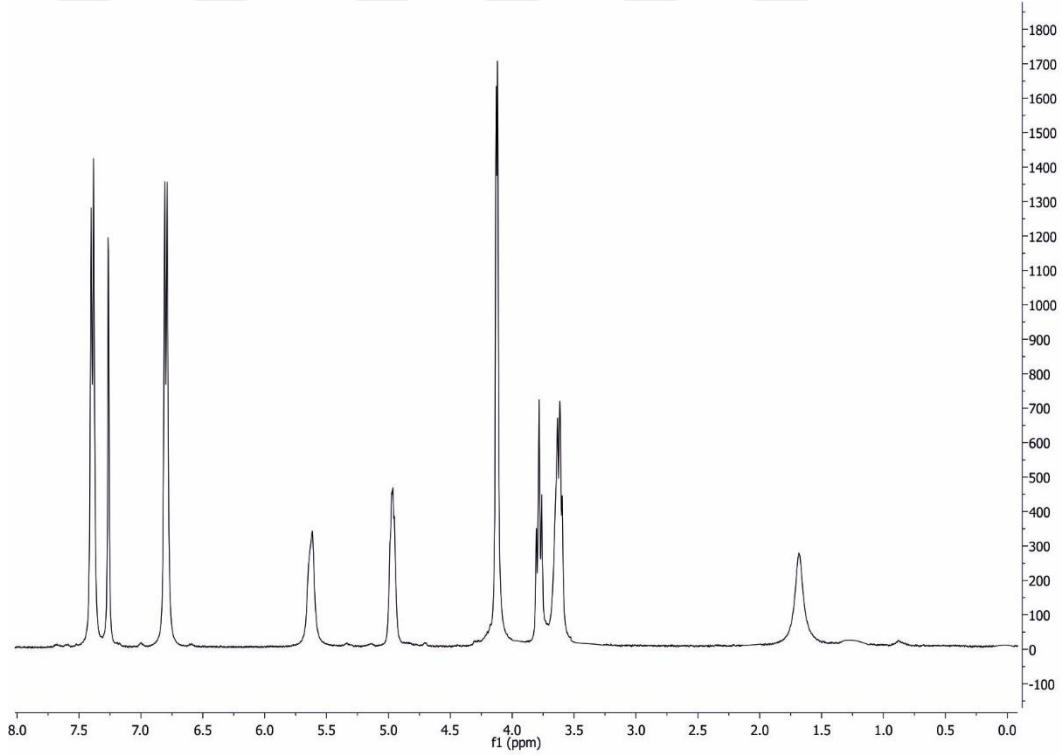
Şekil 4.2.10.a. 5-((4-bromfenoksi)metil)oksazolidin-2-onun 1 H NMR spektrumu
