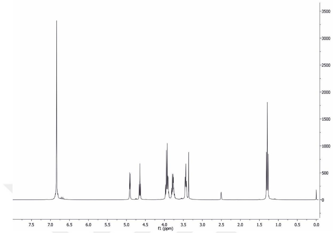
Şekil 4.1.15.a. 3-(4-etoksifenoksi)propan-1,2-diolün ^1\text{H} NMR spektrumu
