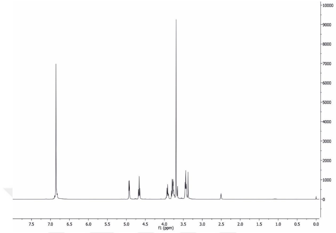
Şekil 4.1.11.a. 3-(4-metoksifenoksi)propan-1,2-diolün ^1\text{H} NMR spektrumu
