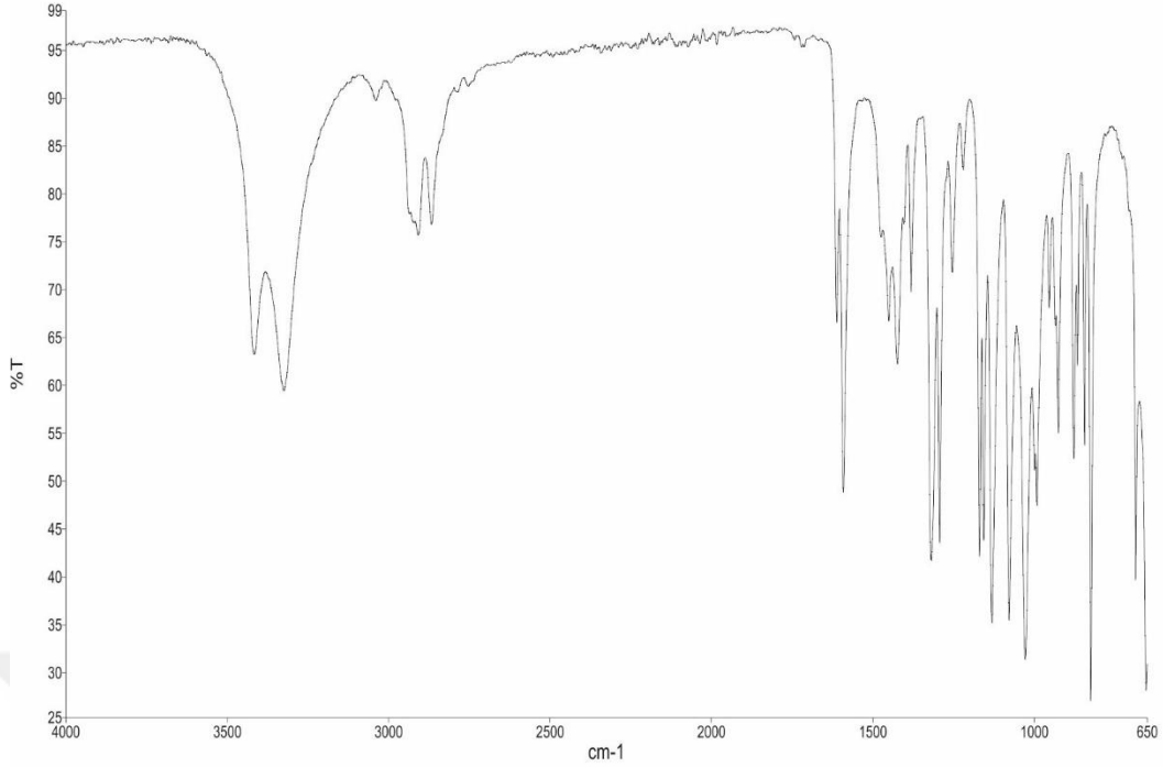
Şekil 4.1.1.c. 3-(3,5-dimetilfenoksi)propan-1,2-diolün IR spektrumu
