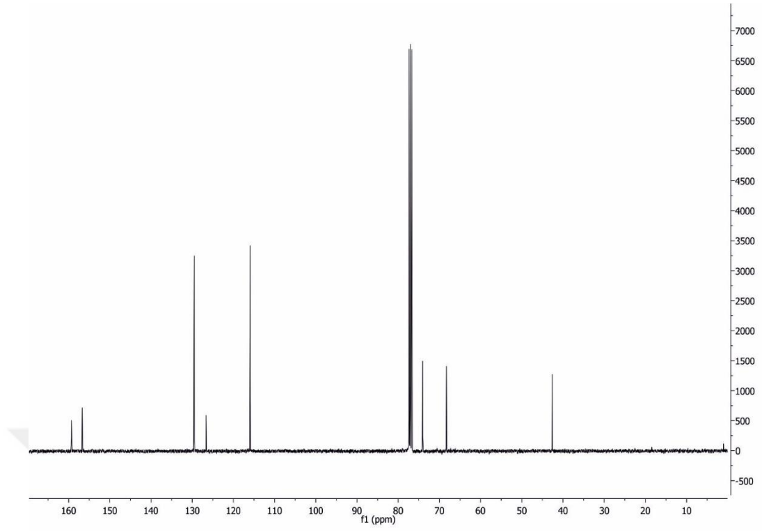
Şekil 4.2.7.b. 5-((4-klorfenoksi)metil)oksazolidin-2-onun ^{13}\text{C} NMR spektrumu
