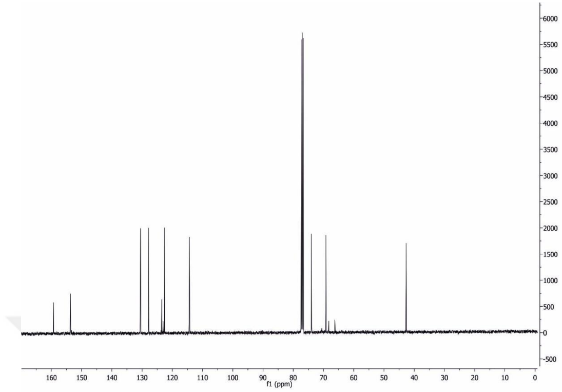
Şekil 4.2.5.b. 5-((2-klorfenoksi)metil)oksazolidin-2-onun ^{13}\text{C} NMR spektrumu
