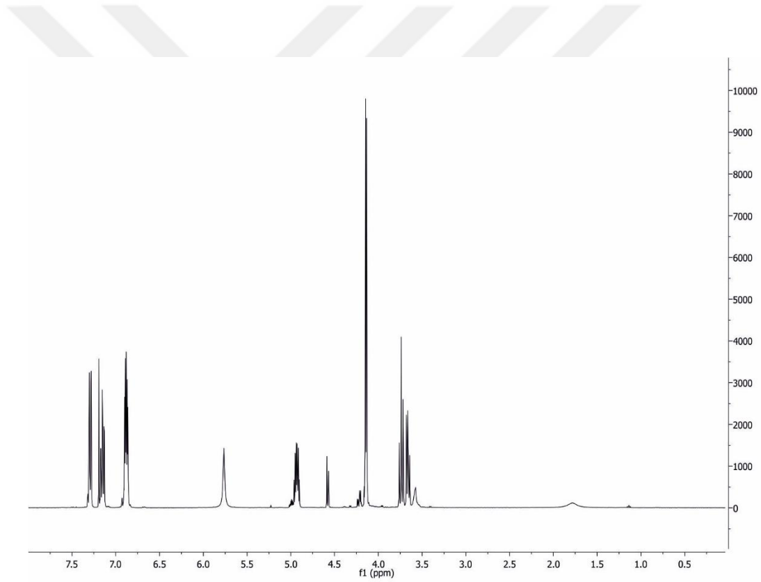
Şekil 4.2.5.a. 5-((2-klorfenoksi)metil)oksazolidin-2-onun 1 H NMR spektrumu
