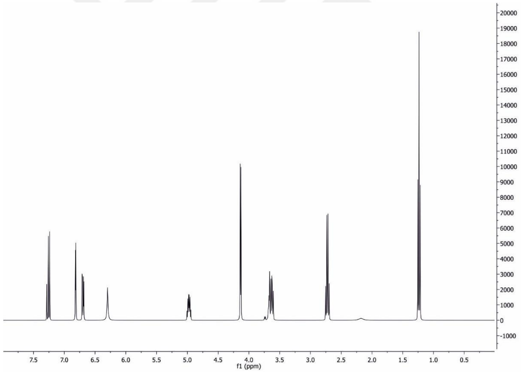
Şekil 4.2.14.a. 5-((3-etil-4-klorfenoksi)metil)oksazolidin-2-onun 1 H NMR spektrumu
