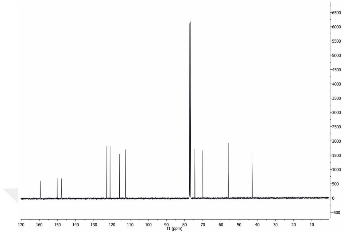
Şekil 4.2.18.b. 5-((2-metoksifenoksi)metil)oksazolidin-2-onun ^{13}\text{C} NMR spektrumu
