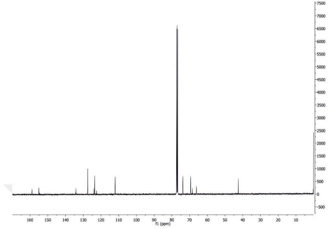
Şekil 4.2.8.b. 5-((2,3-diklorfenoksi)metil)oksazolidin-2-onun ^{13}\text{C} NMR spektrumu
