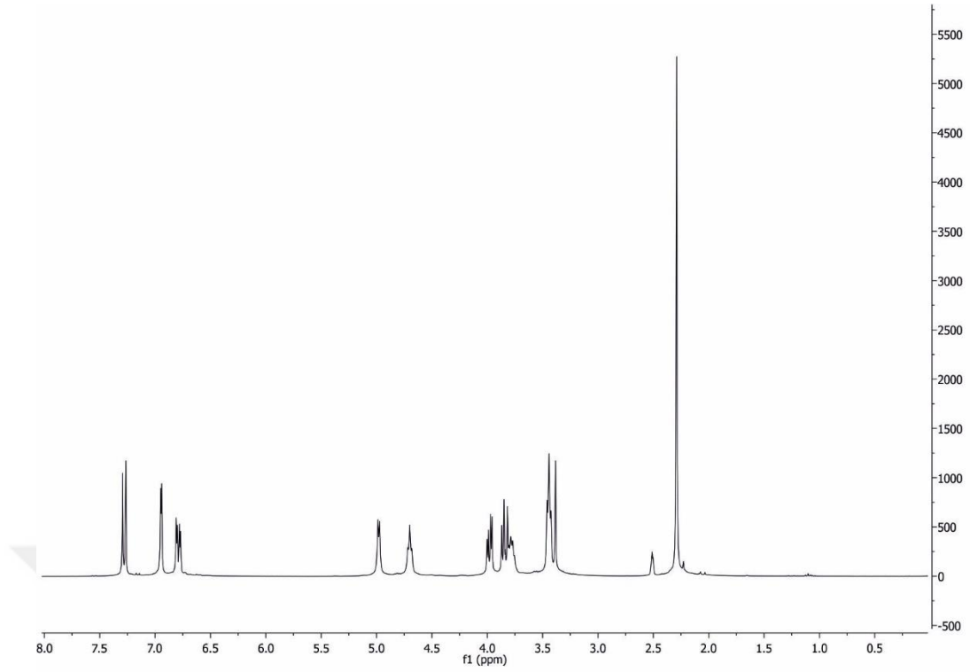
Şekil 4.1.13.a. 3-(4-klor-3-metilfenoksi)propan-1,2-diolün ^1\text{H} NMR spektrumu
