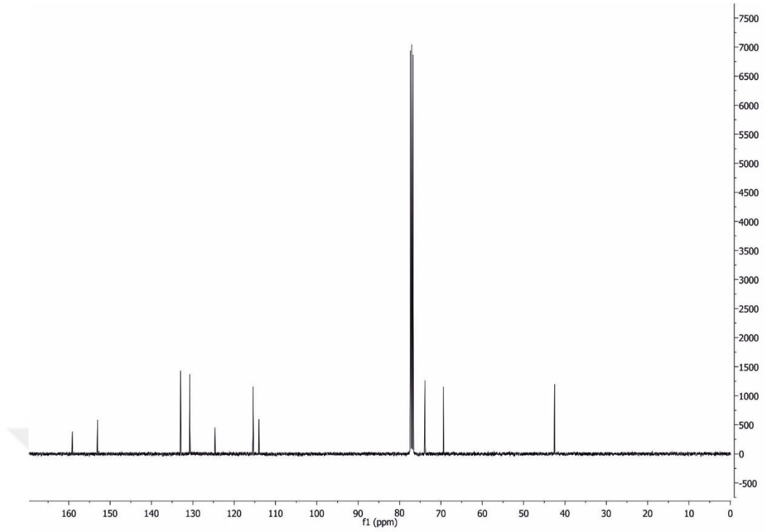
Şekil 4.2.4.b. 5-((4-brom-2-klorfenoksi)metil)oksazolidin-2-onun ^{13}\text{C} NMR spektrumu
