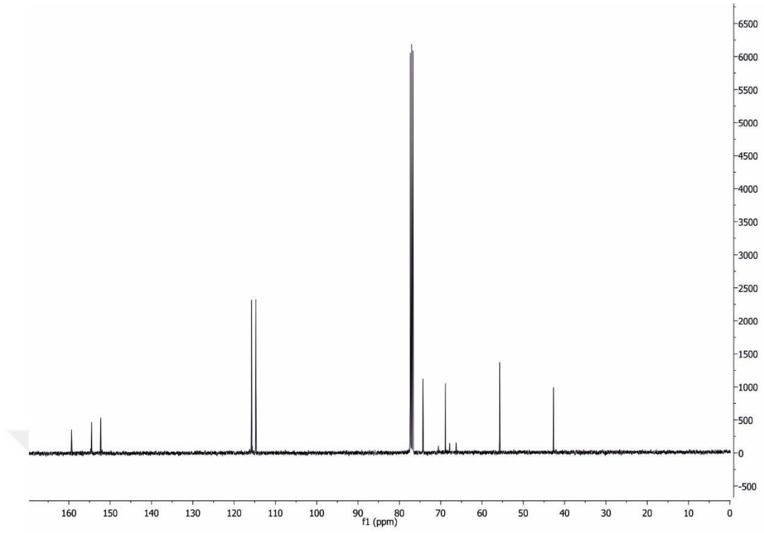
Şekil 4.2.11.b. 5-((4-metoksifenoksi)metil)oksazolidin-2-onun ^{13}\text{C} NMR spektrumu
