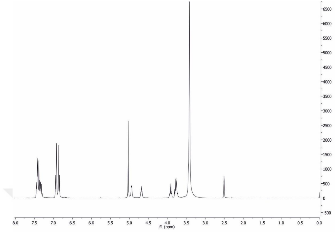
Şekil 4.1.16.a. 3-(4-benziloksifenoksi)propan-1,2-diolün ^1\text{H} NMR spektrumu
