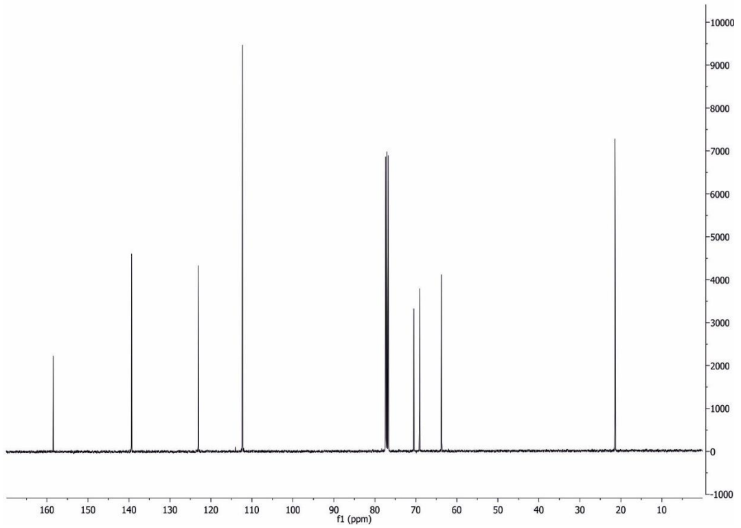
Şekil 4.1.1.b. 3-(3,5-dimetilfenoksi)propan-1,2-diolün ^{13}\text{C} NMR spektrumu
