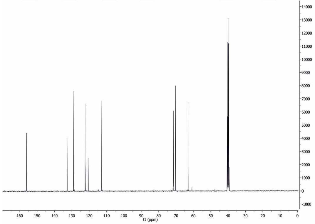
Şekil 4.1.8.b. 3-(2,3-diklorfenoksi)propan-1,2-diolün ^{13}\text{C} NMR spektrumu
