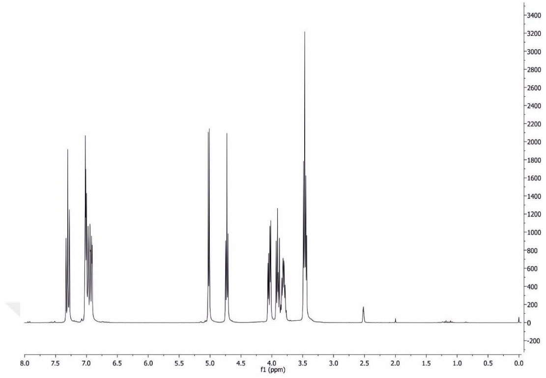
Şekil 4.1.6.a. 3-(3-klorfenoksi)propan-1,2-diolün ^1\text{H} NMR spektrumu
