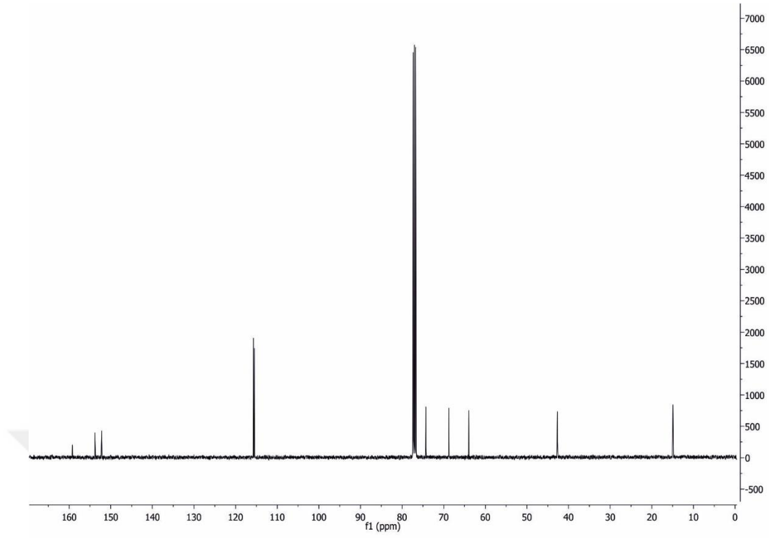
Şekil 4.2.15.b. 5-((4-etoksifenoksi)metil)oksazolidin-2-onun ^{13}\text{C} NMR spektrumu
