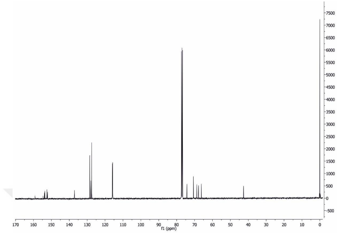
Şekil 4.2.16.b. 5-((4-(benziloxy)fenoksi)metil)oksazolidin-2-onun ^{13}\text{C} NMR spektrumu
