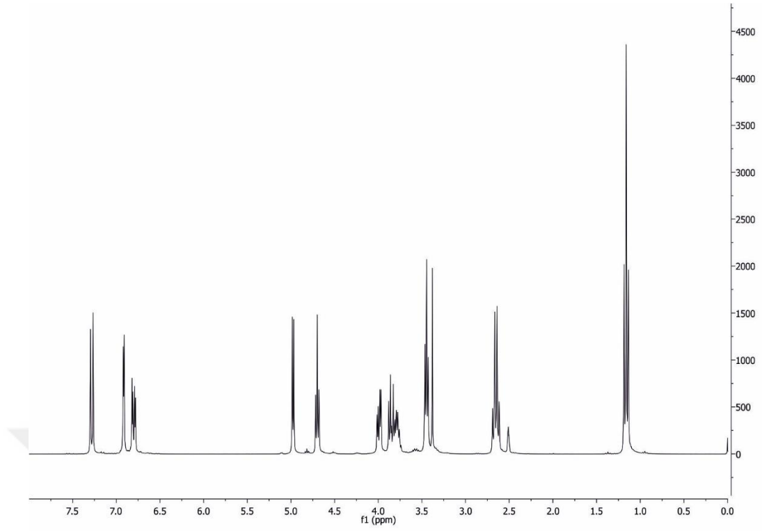
Şekil 4.1.14.a. 3-(3-etil-4-klorfenoksi)propan-1,2-diolün ^1\text{H} NMR spektrumu
