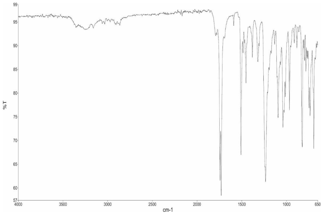
Şekil 4.2.16.c. 5-((4-(benziloxy)fenoksi)metil)oksazolidin-2-onun IR spektrumu
