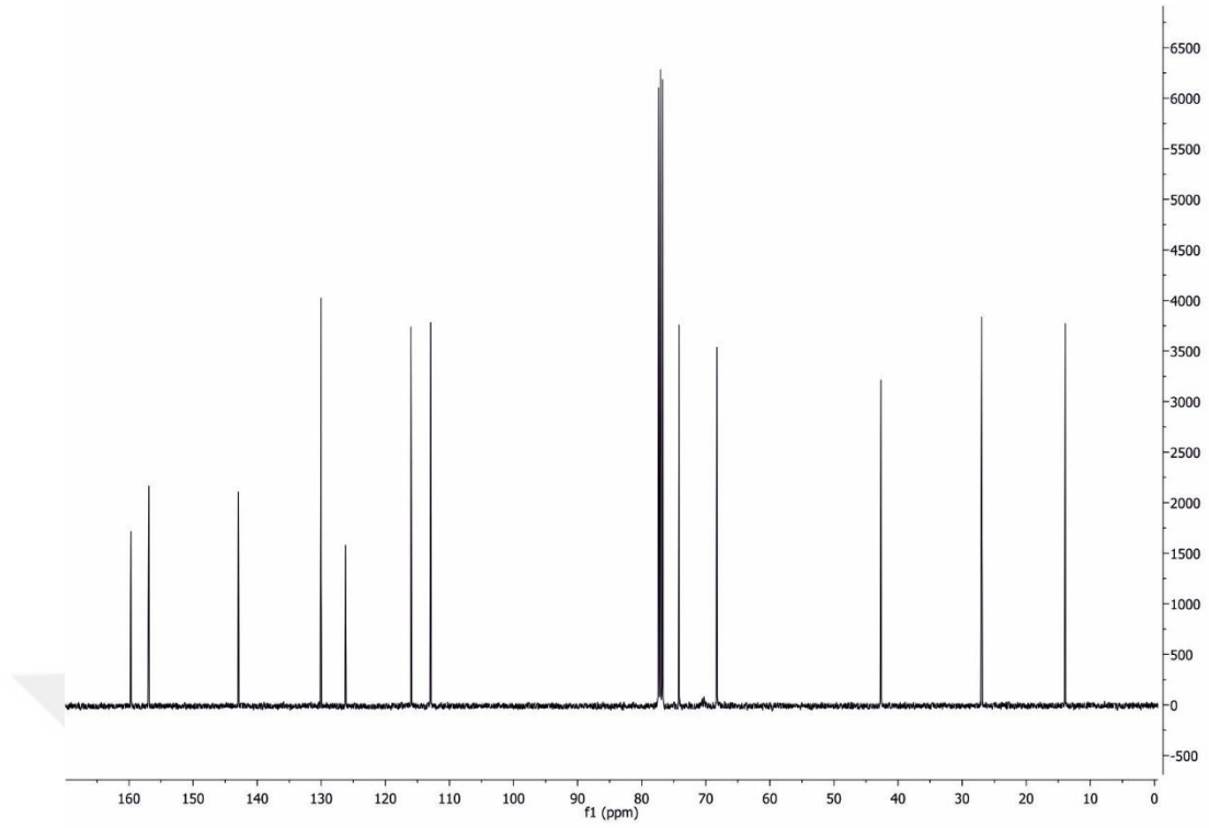
Şekil 4.2.14.b. 5-((3-etil-4-klorfenoksi)metil)oksazolidin-2-onun ^{13}\text{C} NMR spektrumu
