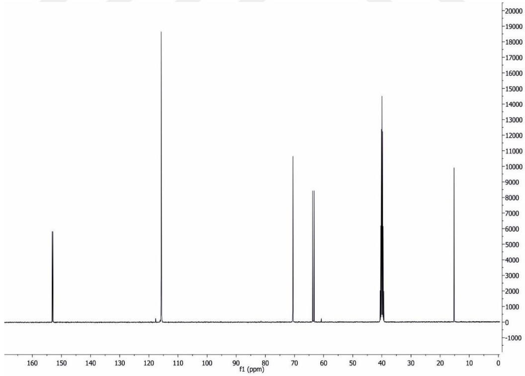
Şekil 4.1.15.b. 3-(4-etoksifenoksi)propan-1,2-diolün ^{13}\text{C} NMR spektrumu
