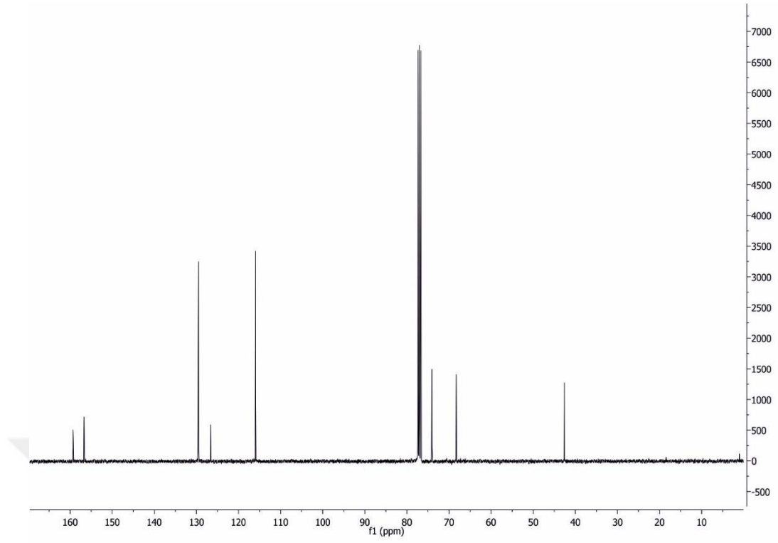
Şekil 4.2.12.b. 5-((4-izopropilfenoksi)metil)oksazolidin-2-onun ^{13}\text{C} NMR spektrumu
