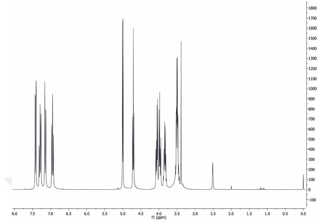
Şekil 4.1.5.a. 3-(2-klorfenoksi)propan-1,2-diolün ^1\text{H} NMR spektrumu
