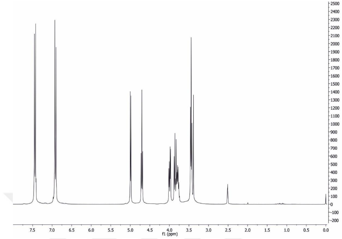
Şekil 4.1.10.a. 3-(4-bromfenoksi)propan-1,2-diolün ^1\text{H} NMR spektrumu
