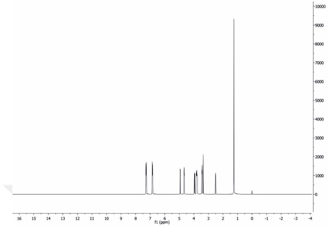
Şekil 4.1.17.a. 3-(4-ter-bütilfenoksi)propan-1,2-diolün 1 H NMR spektrumu
