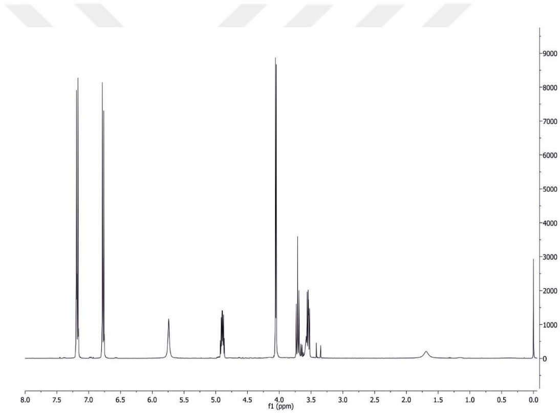
Şekil 4.2.7.a. 5-((4-klorfenoksi)metil)oksazolidin-2-onun 1 H NMR spektrumu
