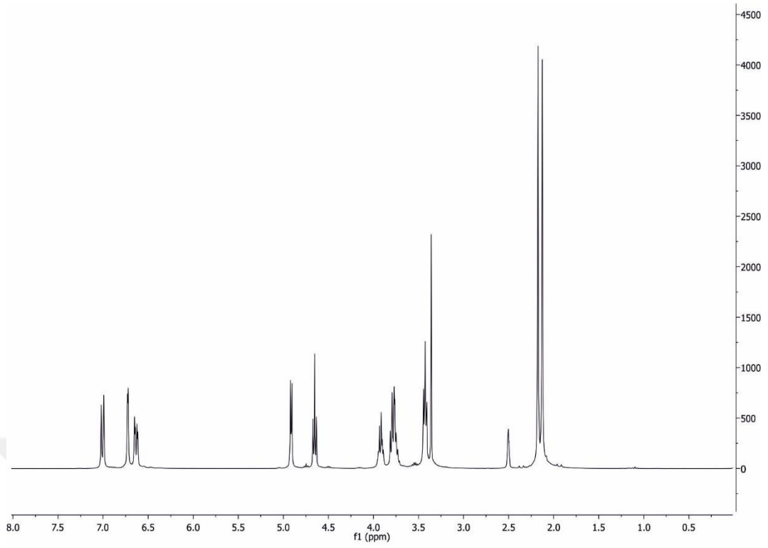
Şekil 4.1.2.a. 3-(3,4-dimetilfenoksi)propan-1,2-diolün ^1\text{H} NMR spektrumu
