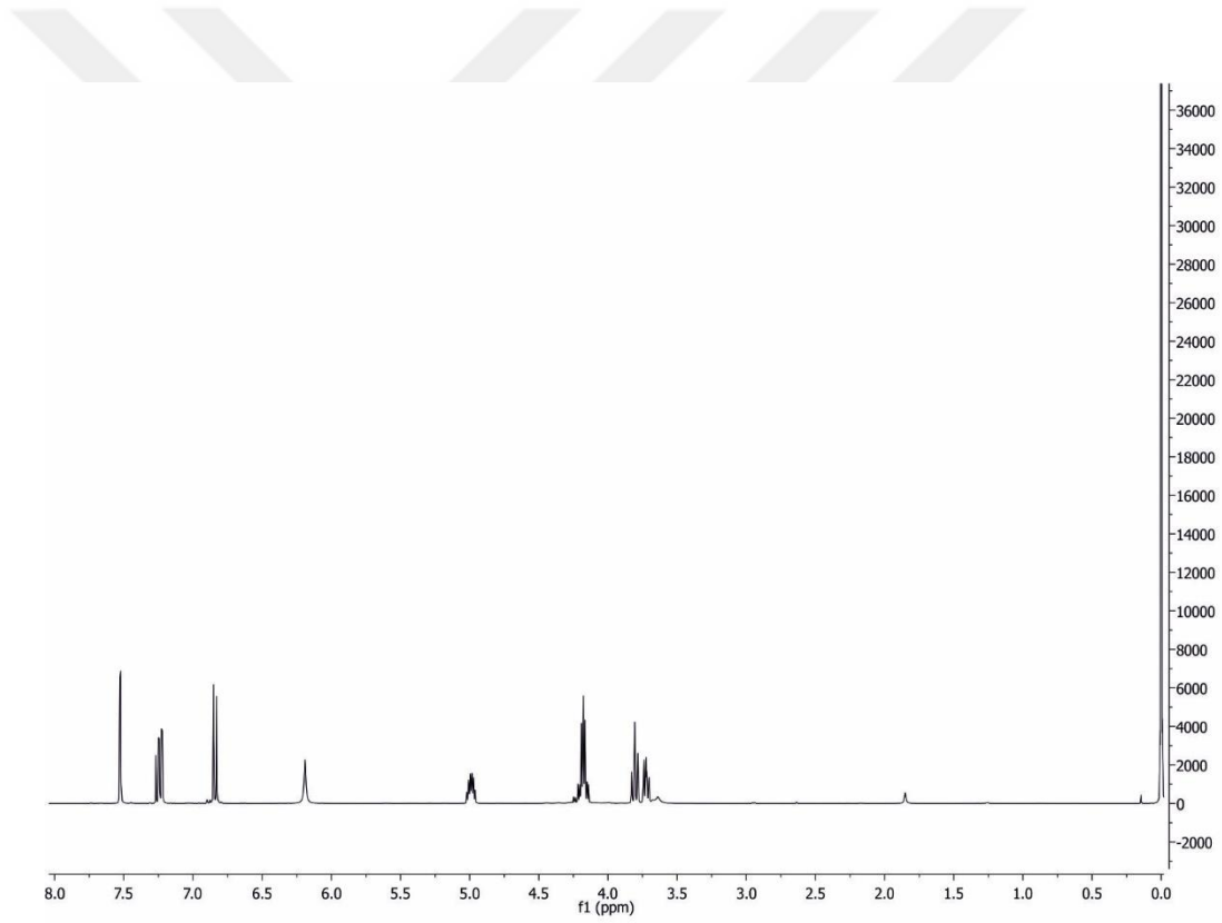
Şekil 4.2.3.a. 5-((2-brom-4-klorfenoksi)metil)oksazolidin-2-onun 1 H NMR spektrumu
