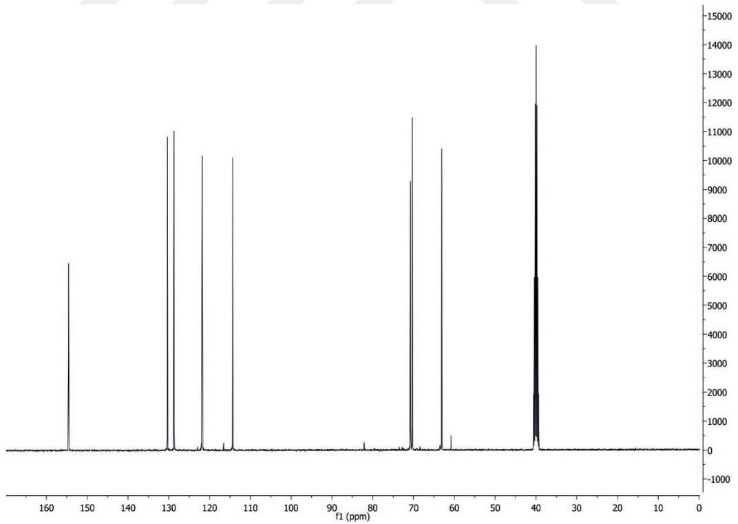
Şekil 4.1.5.b. 3-(2-klorfenoksi)propan-1,2-diolün ^{13}\text{C} NMR spektrumu
