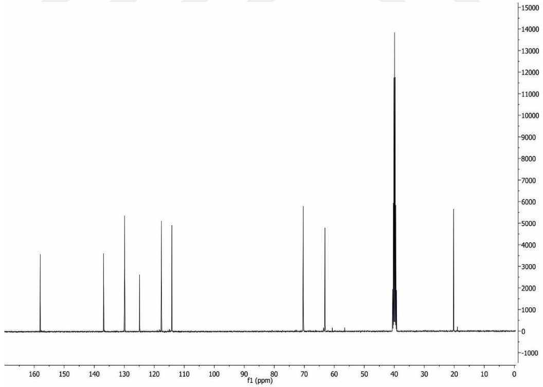
Şekil 4.1.13.b. 3-(4-klor-3-metilfenoksi)propan-1,2-diolün ^{13}\text{C} NMR spektrumu
