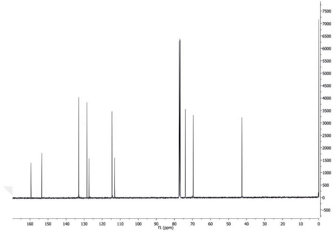
Şekil 4.2.3.b. 5-((2-brom-4-klorfenoksi)metil)oksazolidin-2-onun ^{13}\text{C} NMR spektrumu
