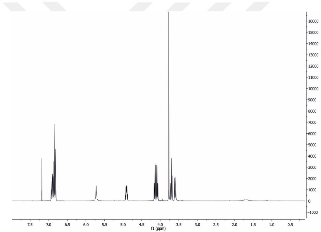
Şekil 4.2.18.a. 5-((2-metoksifenoksi)metil)oksazolidin-2-onun 1 H NMR spektrumu
