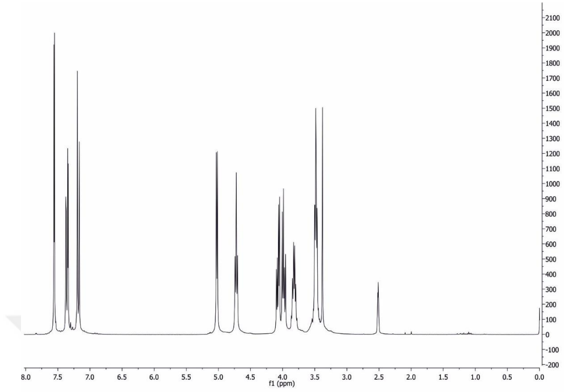
Şekil 4.1.9.a. 3-(2,4-diklorfenoksi)propan-1,2-diolün ^1\text{H} NMR spektrumu
