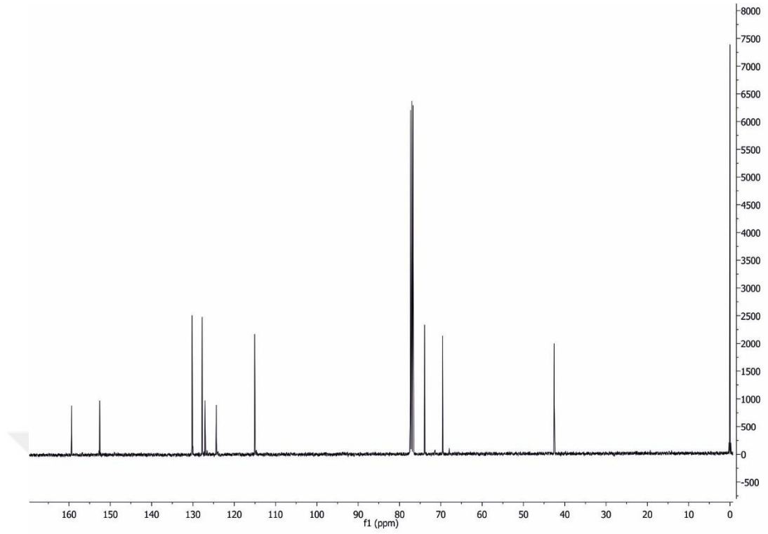
Şekil 4.2.9.b. 5-((2,4-diklorfenoksi)metil)oksazolidin-2-onun ^{13}\text{C} NMR spektrumu
