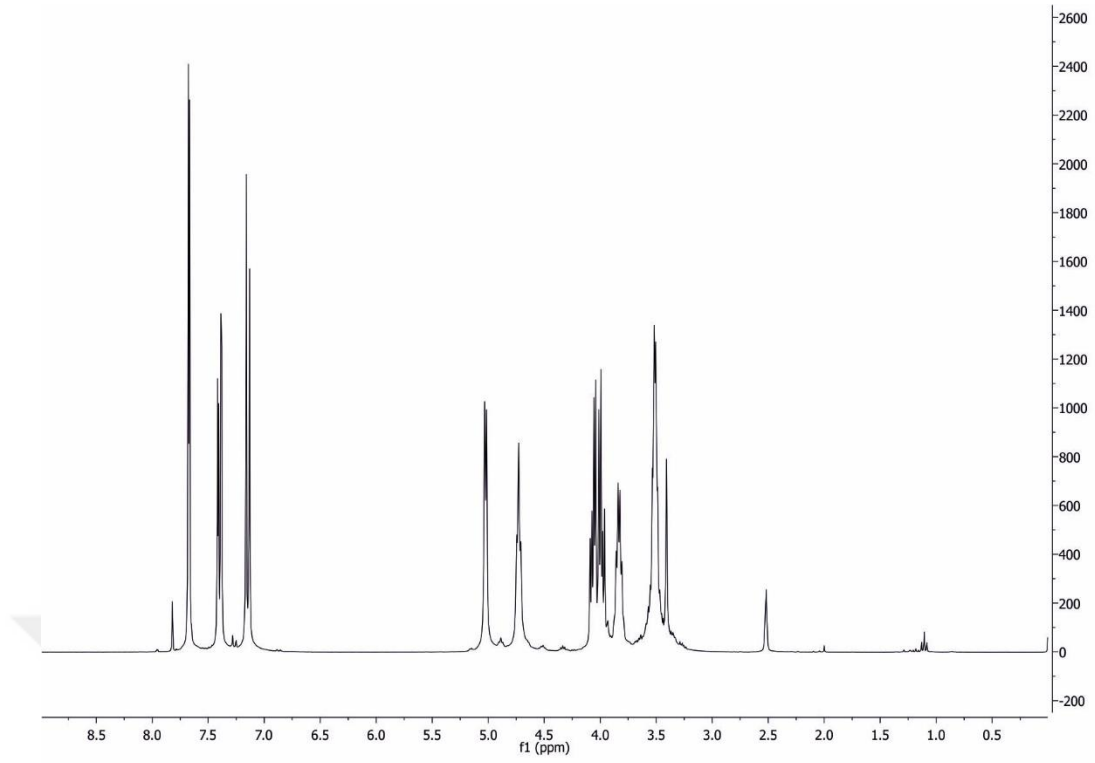
Şekil 4.1.3.a. 3-(2-brom-4-klorfenoksi)propan-1,2-diolün ^1\text{H} NMR spektrumu
