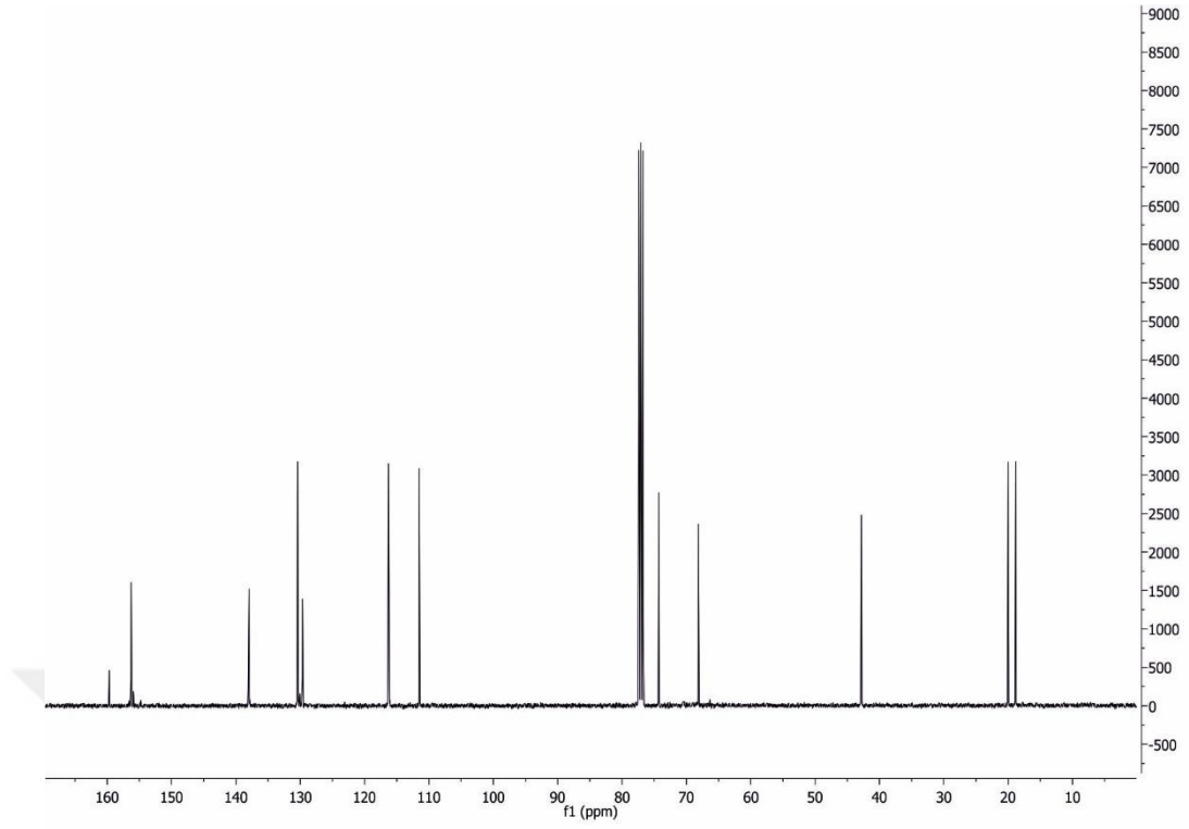
Şekil 4.2.2.b. 5-((3,4-dimetilfenoksi)metil)oksazolidin-2-onun ^{13}\text{C} NMR spektrumu
