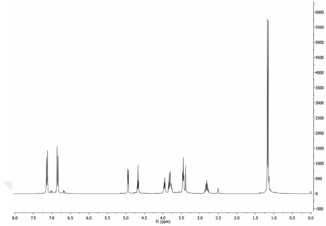
Şekil 4.1.12.a. 3-(4-izopropilfenoksi)propan-1,2-diolün ^1\text{H} NMR spektrumu
