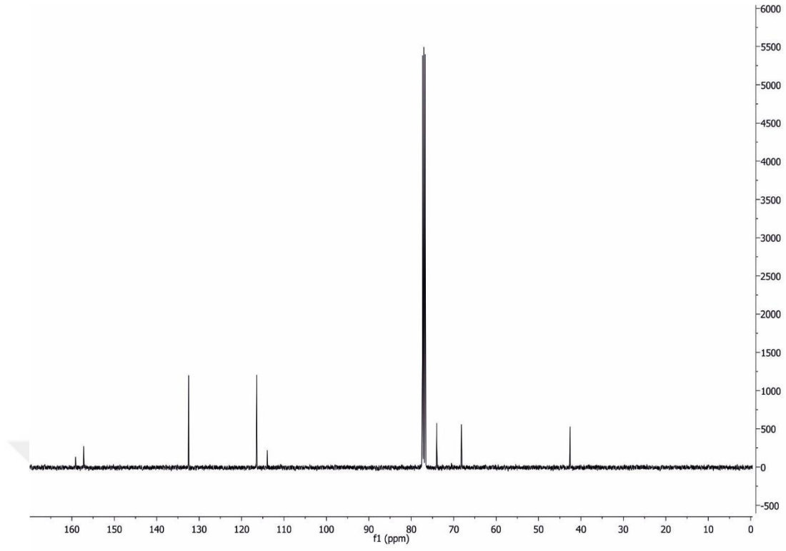
Şekil 4.2.10.b. 5-((4-bromfenoksi)metil)oksazolidin-2-onun ^{13}\text{C} NMR spektrumu
