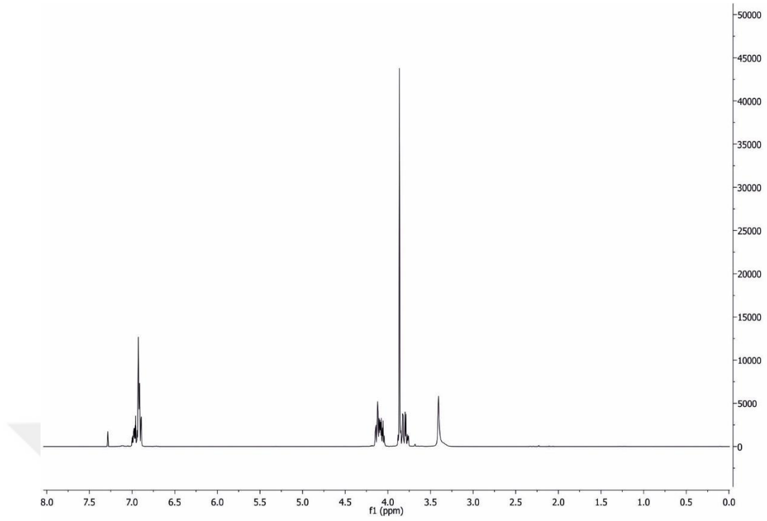
Şekil 4.1.18.a. 3-(2-metoksifenoksi)propan-1,2-diolün ^1\text{H} NMR spektrumu
