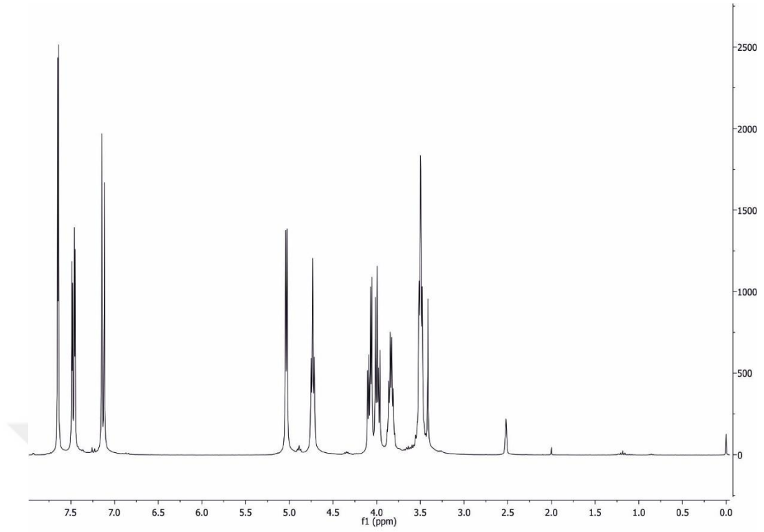
Şekil 4.1.4.a. 3-(4-brom-2-klorfenoksi)propan-1,2-diolün ^1\text{H} NMR spektrumu
