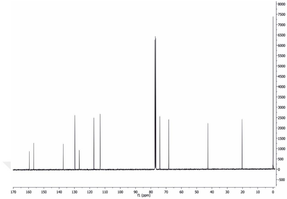
Şekil 4.2.13.b. 5-((4-klor-3-metilfenoksi)metil)oksazolidin-2-onun ^{13}\text{C} NMR spektrumu
