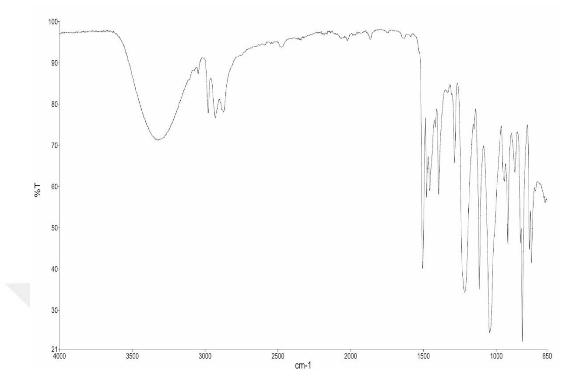
Şekil 4.1.15.c. 3-(4-etoksifenoksi)propan-1,2-diolün IR spektrumu
