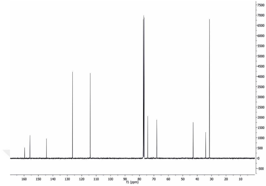
Şekil 4.2.17.b. 5-((4-(ter-bütıl)fenoksi)metil)oksazolidin-2-onun ^{13}\text{C} NMR spektrumu
