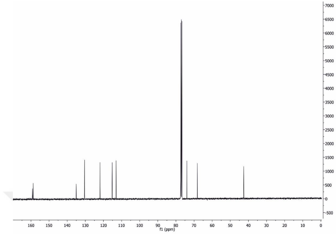
Şekil 4.2.6.b. 5-((3-klorfenoksi)metil)oksazolidin-2-onun ^{13}\text{C} NMR spektrumu
