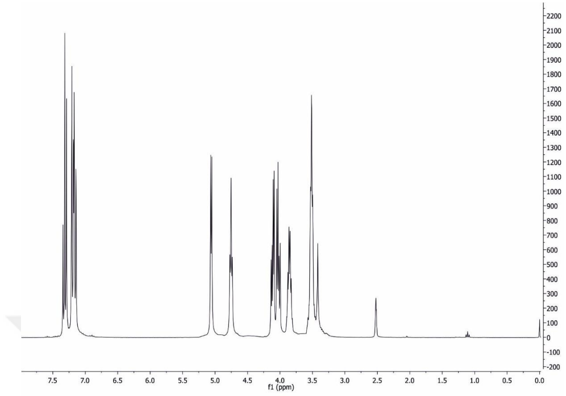
Şekil 4.1.8.a. 3-(2,3-diklorfenoksi)propan-1,2-diolün ^1\text{H} NMR spektrumu
