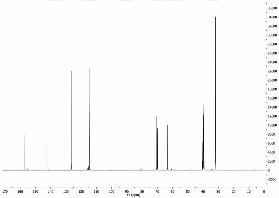
Şekil 4.1.17.b. 3-(4-ter-bütilfenoksi)propan-1,2-diolün 13 C NMR spektrumu
