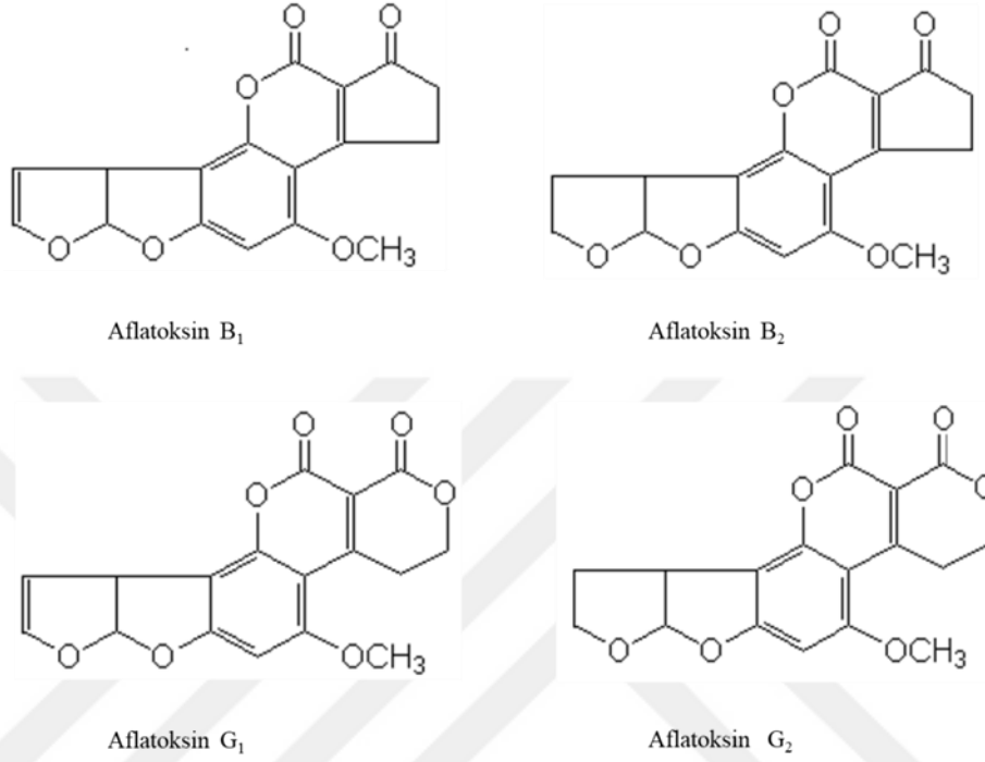
Şekil 1.2: Aflatoksin B 1 , B 2 , G 1 ve G 2 'nin kimyasal yapısı
