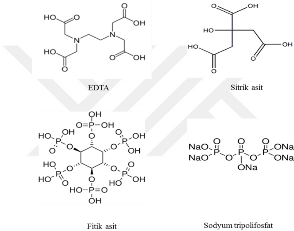
Şekil 1.4: Şelat ajanlarının kimyasal yapıları
