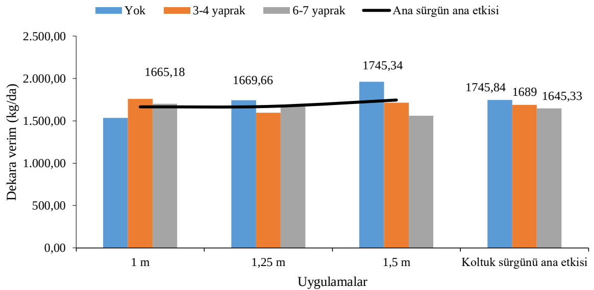
řekil 4.196. 2013 yılı dekara verim (kg/da)
