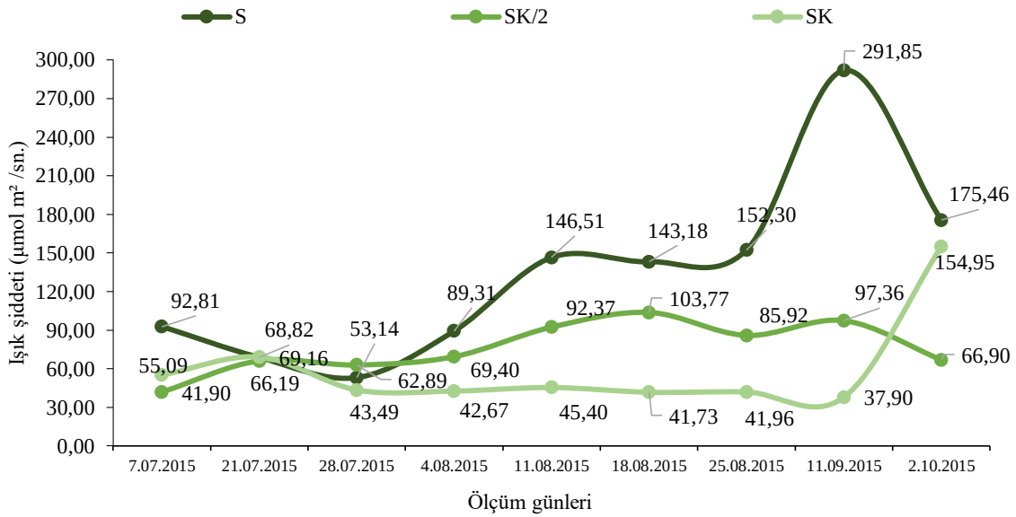
Şekil 4.38. 2015 yılı fizyolojik aktivite ölçümü yapılan günlerde taç içi mikroklimalarının ışık şiddeti verileri
