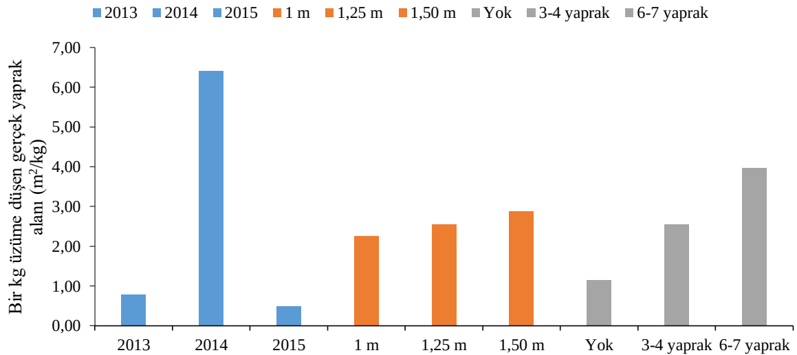
Şekil 4.128. Bir kg üzüme düşen gerçek yaprak alanı yıl birleştirmesi ( m^2/kg )
