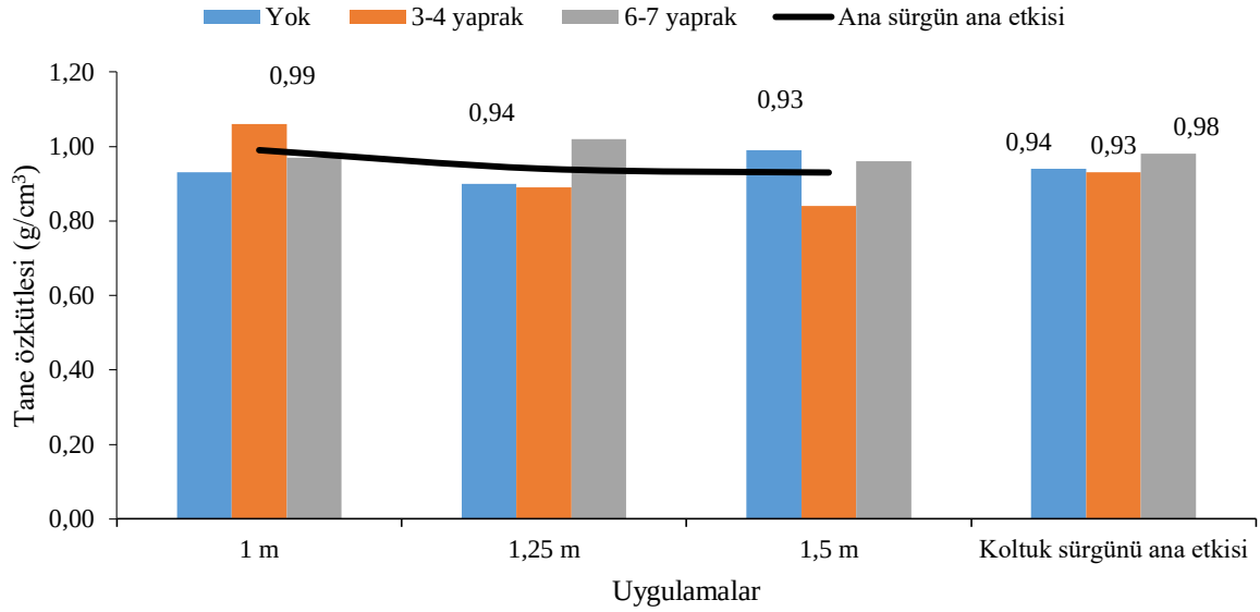
Şekil 4.157. 2013 yılı tane özkütlesi (g/cm 3 )
