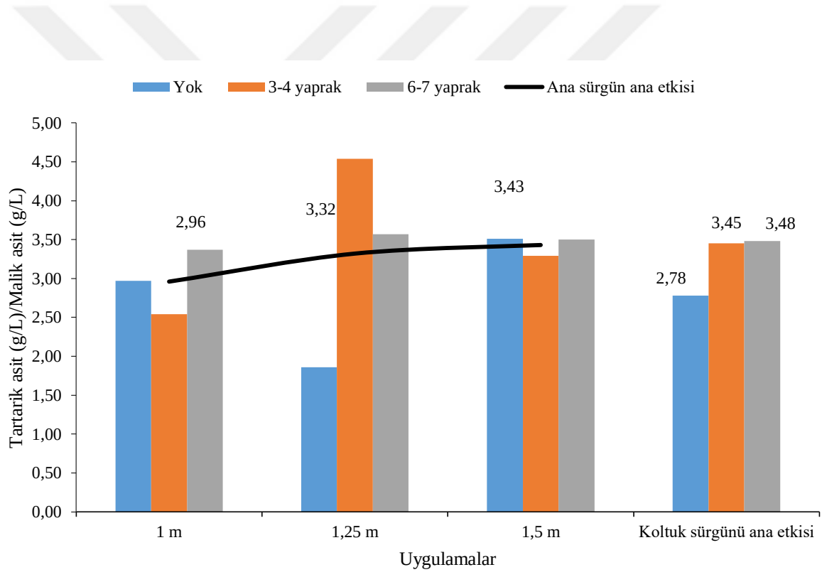
Şekil 4.283. 2015 yılı Tartarik asit (g/L)/Malik asit (g/L)
