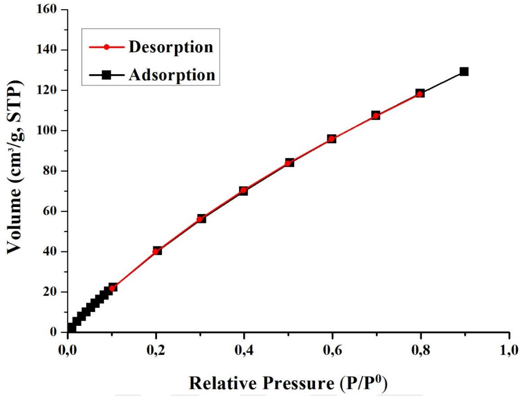
Şekil 4.113: Cu-OATA-Zn (12)'nin 273 K'de deneysel \text{CO}_2 izotermi.
