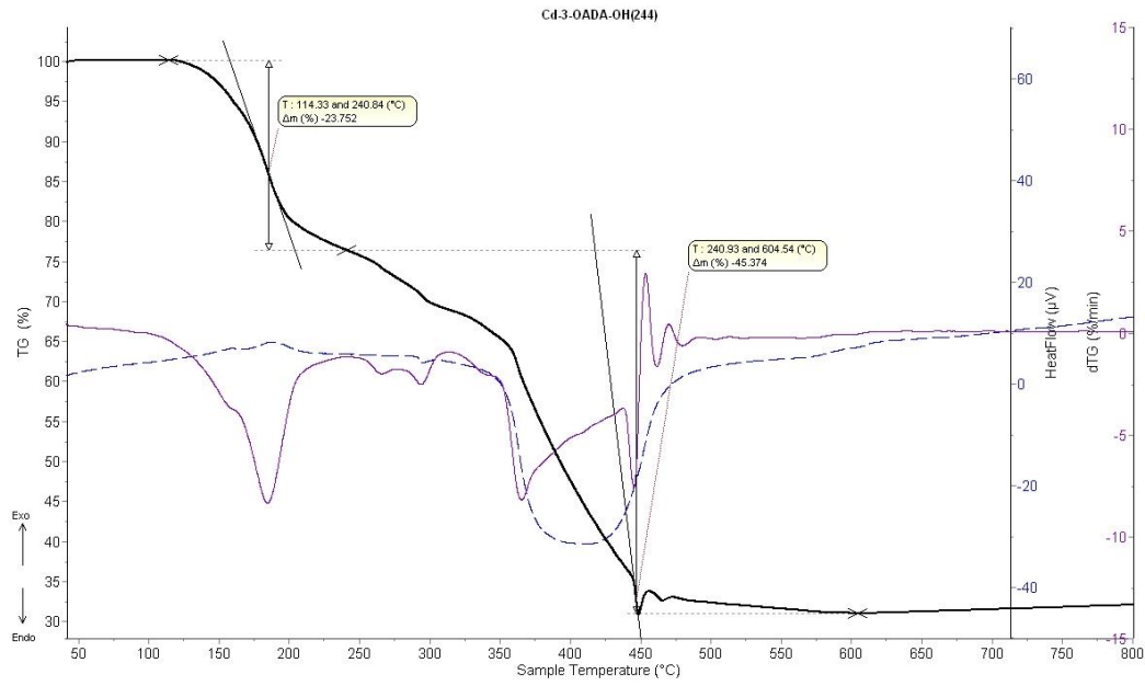
Şekil 4.32: Cd-3OADA-OH (8)’nın termal analiz eğrileri.
