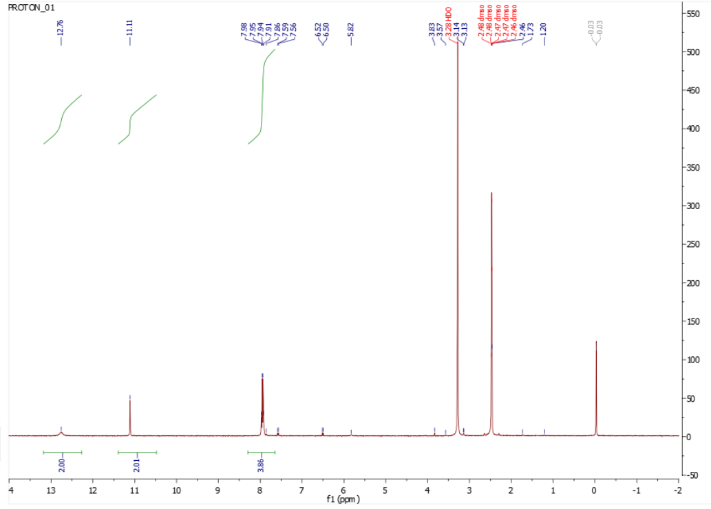
Şekil 4.9: 4-OADAH 2 'nin 1 H NMR spektrumu .
