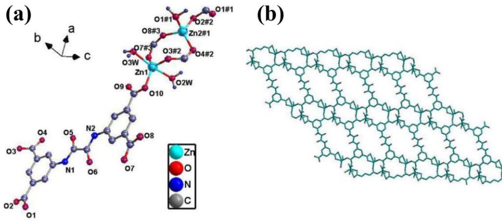
Şekil 2.7: \{[(Zn_2(BDPO) \cdot 3H_2O) \cdot H_2O]_n kompleksinin (a) asimetric birimi (b) iki boyutlu yapısı.
