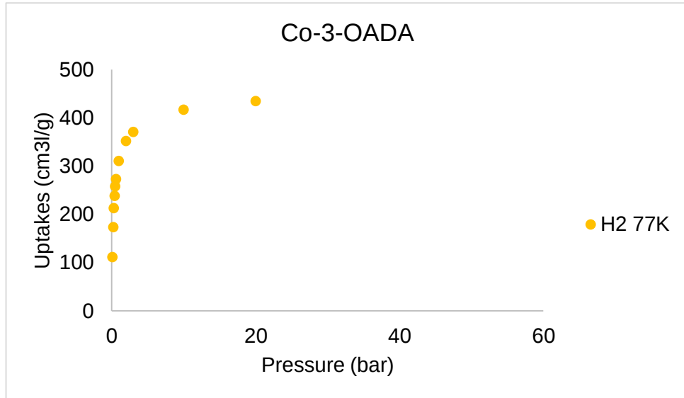
Şekil 4.90: Co-3-OADA (3)'nın 77 K'de teorik H 2 adsorpsiyon izotermi.
