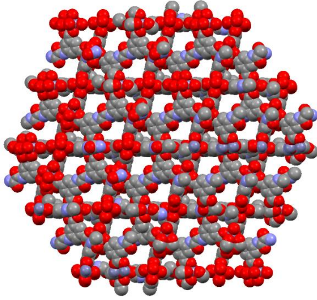
Şekil 4.39: Zn-OATA (4)'nin gözenekli yapısının uzay-dolgu modeliyle gösterimi.
