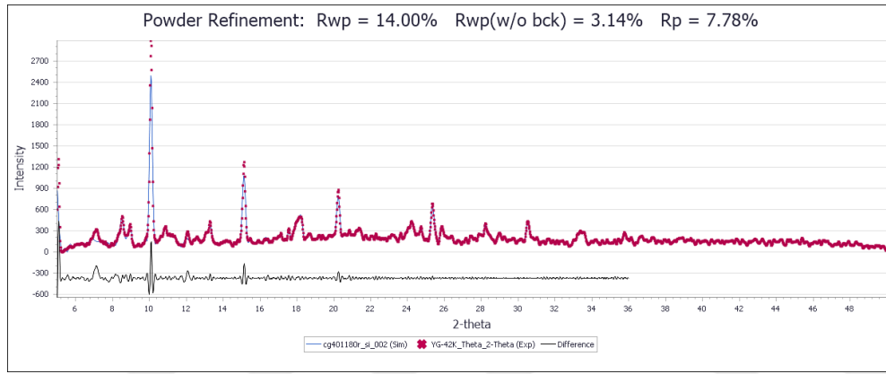
Şekil 4.46: Co-OATA (kırmızı) (7)'in modellenmesi.
