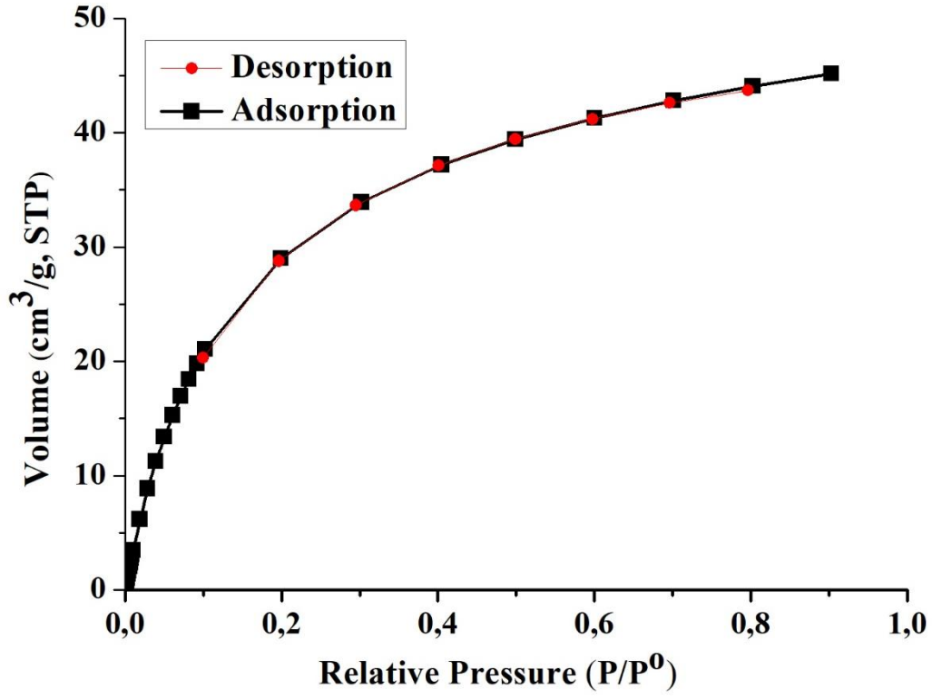
Şekil 4.109: Co-3-OADA (3)'ün 273 K'de deneysel \text{CO}_2 izoterminin.
