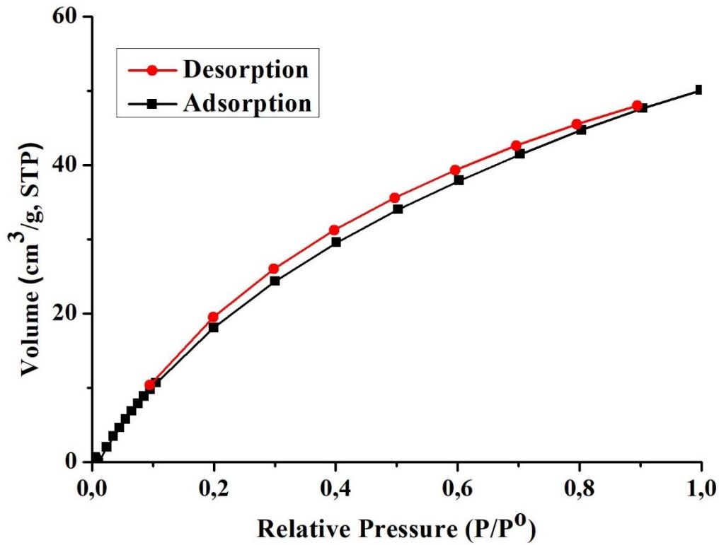
Şekil 4.114: Cu-OATA-Zn (12)'nin 298 K'de deneysel \text{CO}_2 izotermi.
