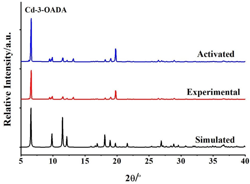
Şekil 4.57: Simüle edilen, deneysel ve aktive edilen Cd-3-OADA (2)'nın toz XRD desenleri.
