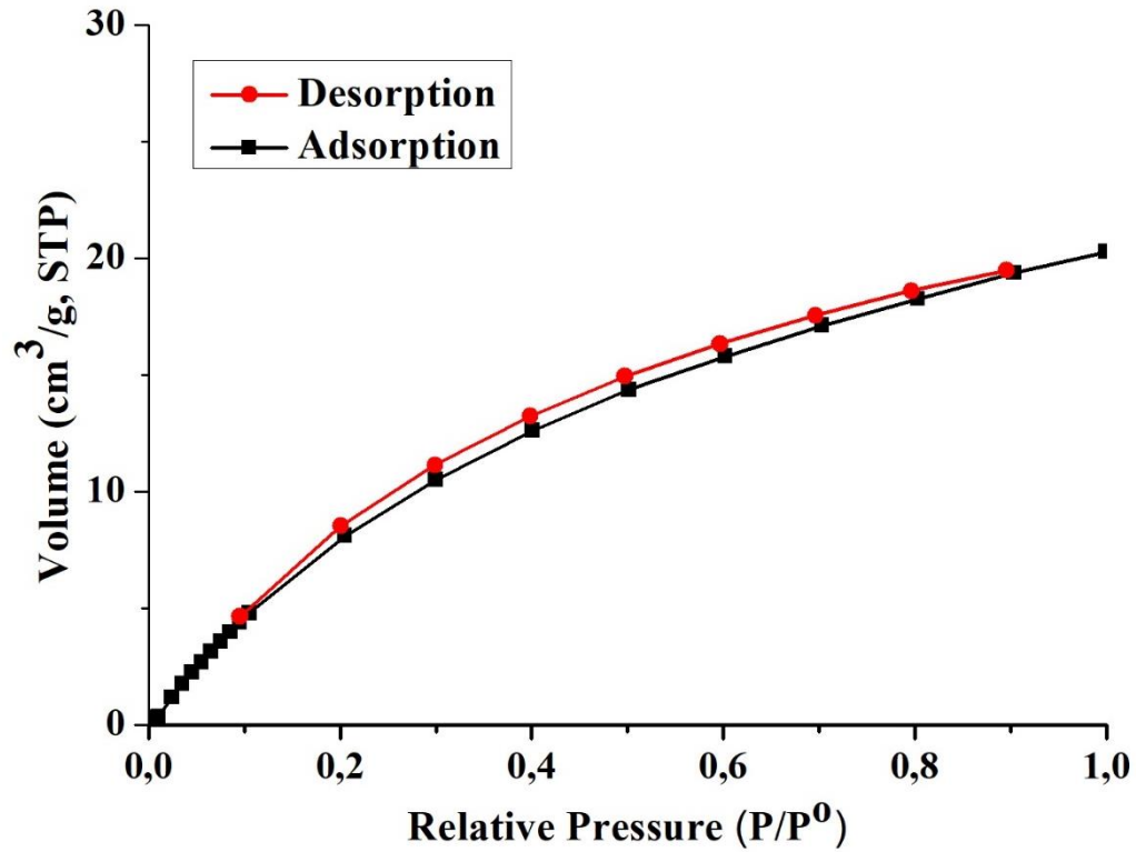
Şekil 4.110: Co-3-OADA (3)'ün 298 K'de deneysel \text{CO}_2 izoterminin.
