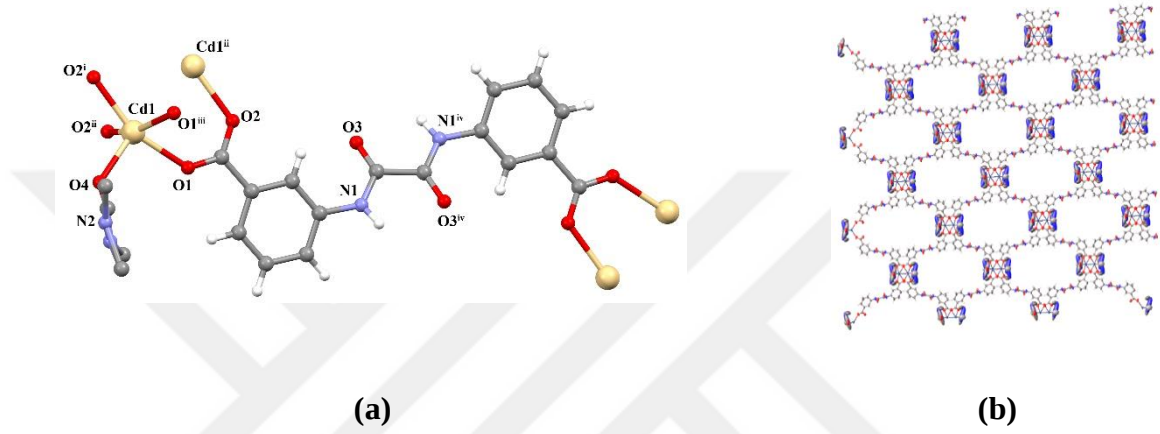
Şekil 4.33: (a) Cd-3-OADA (2)'nin molekül yapısı (b) 2D tabaka yapısı
