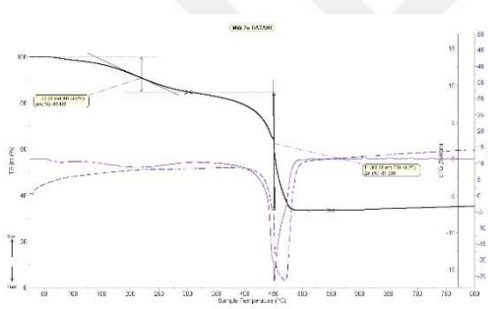
Zn-OATA-MW (10a)
