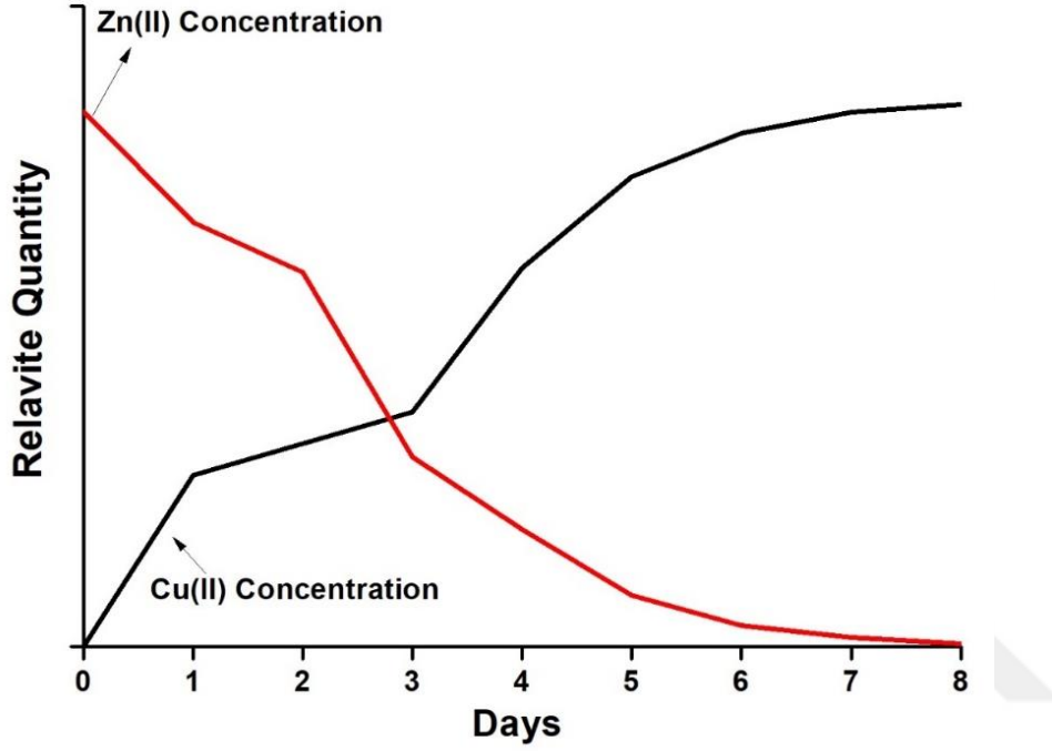
Şekil 4.77: Zn-OATA (4)'ün Cu-OATA-Zn (12)'e dönüşüm sürecinin ICP ile takip edilmesi.
