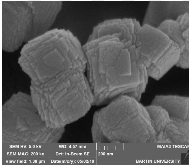
Şekil 4.75: Cd-OATA-MW (11)'in SEM görüntüsü
