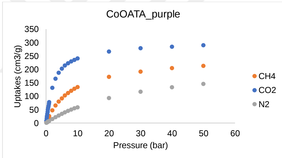
Şekil 4.85: Co-OATA (mor) (6)'un 298 K'de CH 4 , CO 2 , ve N 2 adsorpsiyon teorik izotermi.
