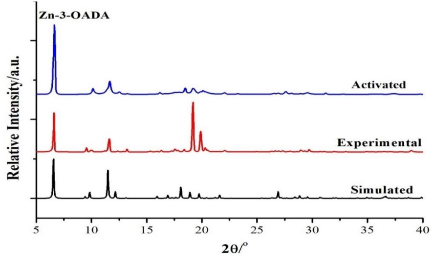
Şekil 4.55: Simüle edilen, deneysel ve aktive edilen Zn-3-OADA (1)'nın toz XRD desenleri.
