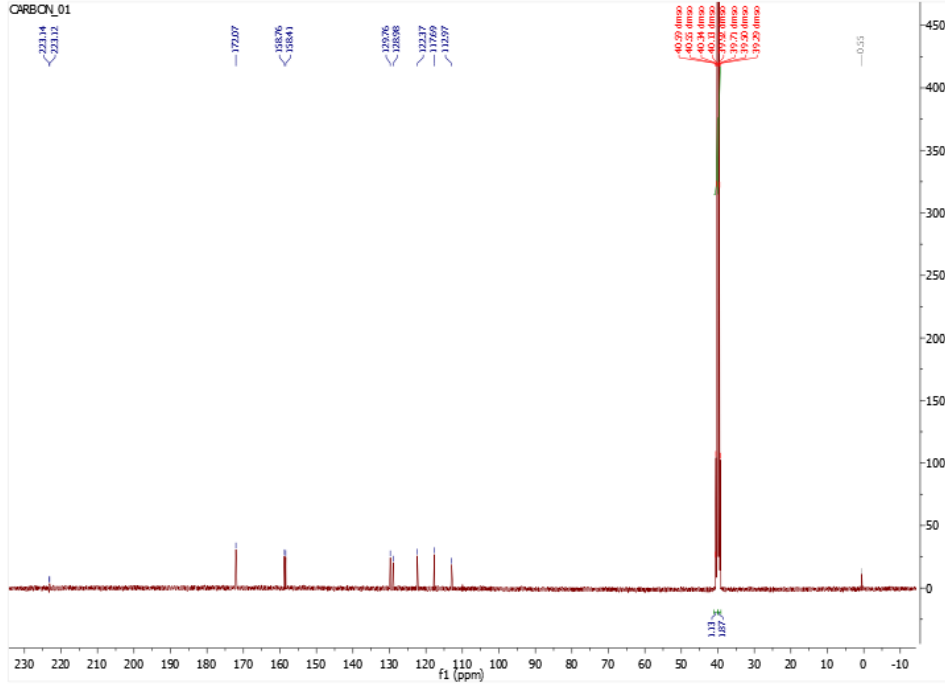
Şekil 4.8: 3-OADAH 2 -OH'nin 13 C NMR spektrumu
