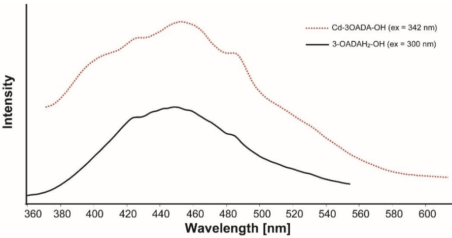
Şekil 4.54: 3-OADAH 2 -OH ve Cd-3-OADA-OH 'nın katı hal emisyon eğrileri.
