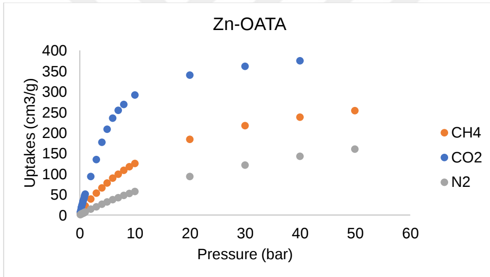
Şekil 4.83: Zn-OATA (4)'nın 298 K'de CH 4 , CO 2 , ve N 2 adsorpsiyon teorik izotermeleri.
