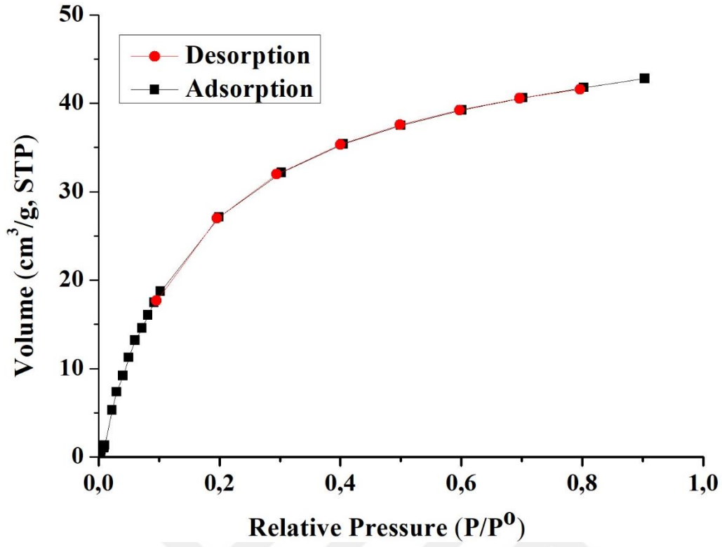
Şekil 4.105: Zn-3-OADA (1)'nin 273 K'de deneysel \text{CO}_2 izotermi.
