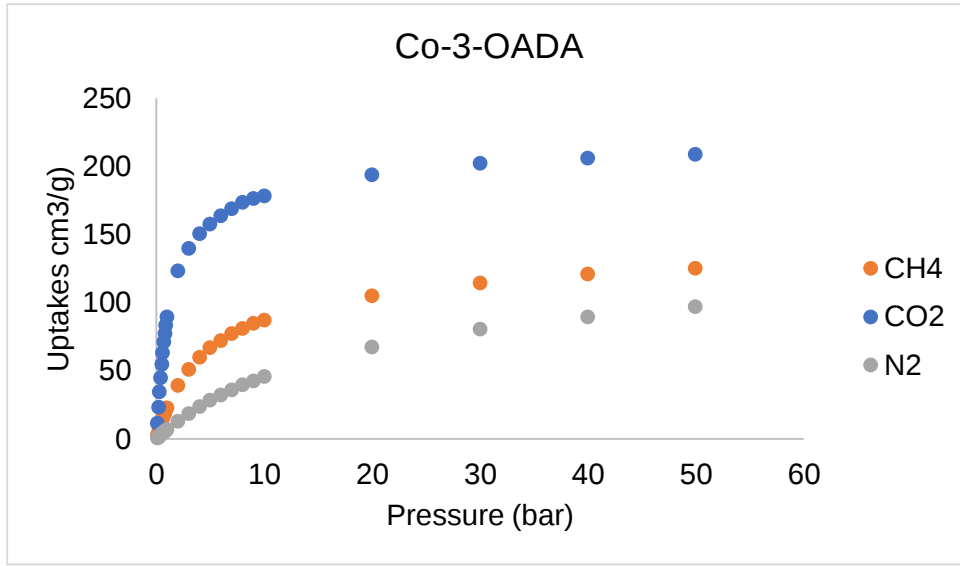
Şekil 4.82: Co-3-OADA (3)'nın 298 K'de CH 4 , CO 2 , ve N 2 adsorpsiyon teorik izotermeleri.
