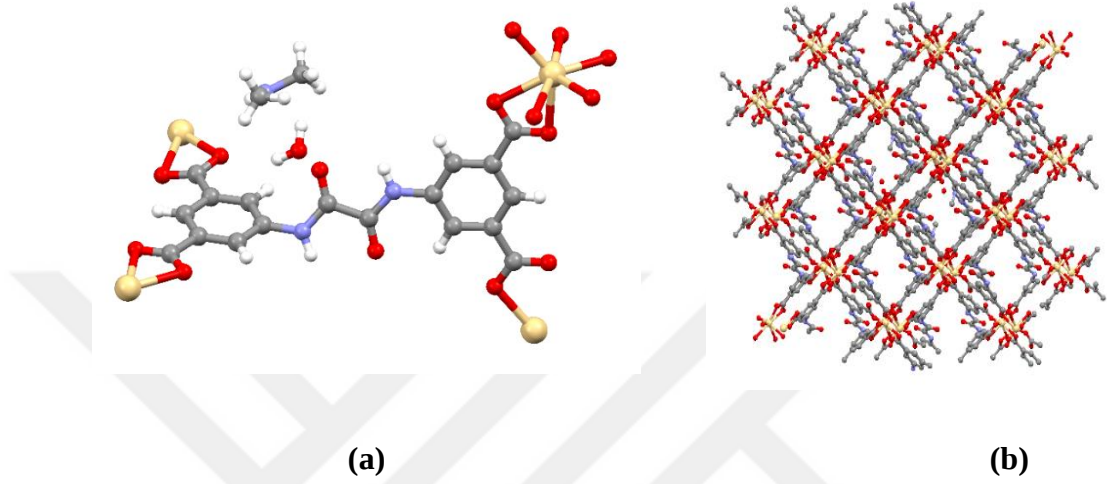
Şekil 4.41: (a) Cd-OATA (5)'in molekül yapısı (b) 3D yapısı.
