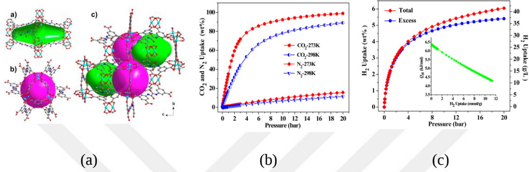
Şekil 2.2: HNUST-3’in (a) iki farklı gözenek yapısının gösterimi (b) yüksek basınçta CO 2 , N 2 (c) ve H 2 adsorpsiyon izotermi.
