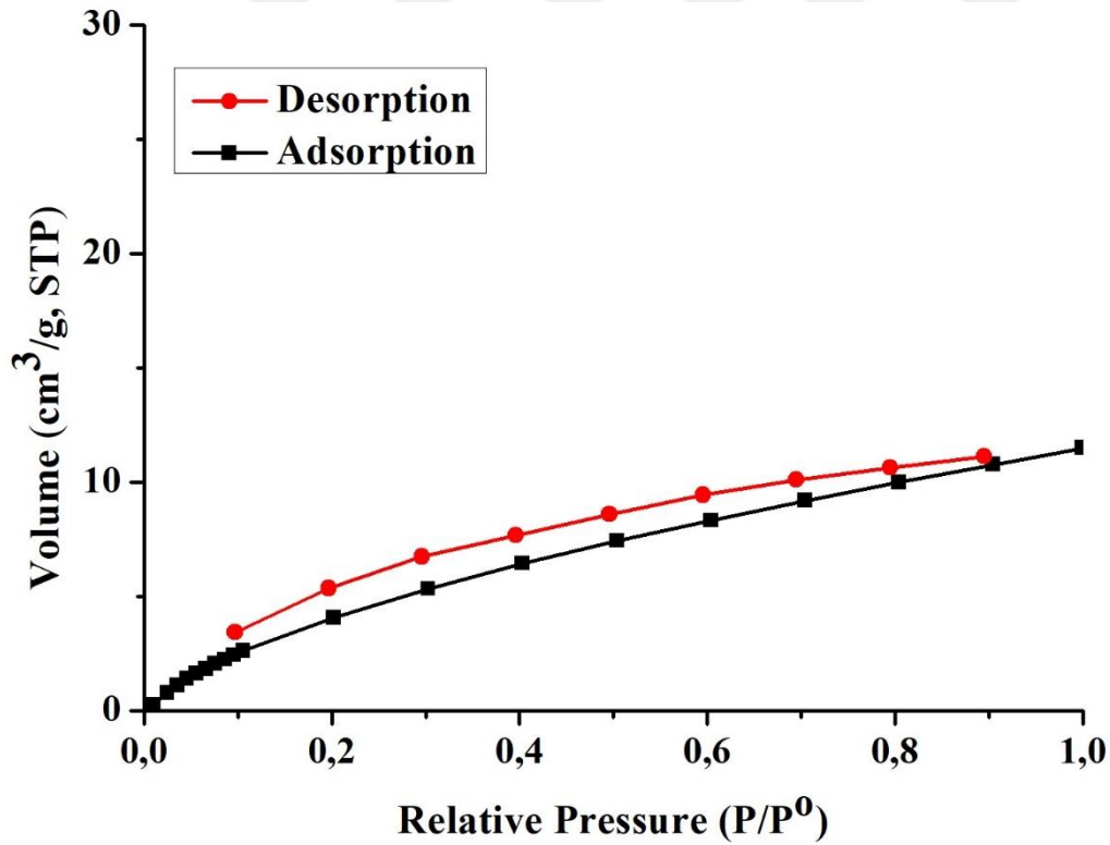
Şekil 4.112: Cd-OATA (5)'nin 298 K'de deneysel CO 2 izoterminin.
