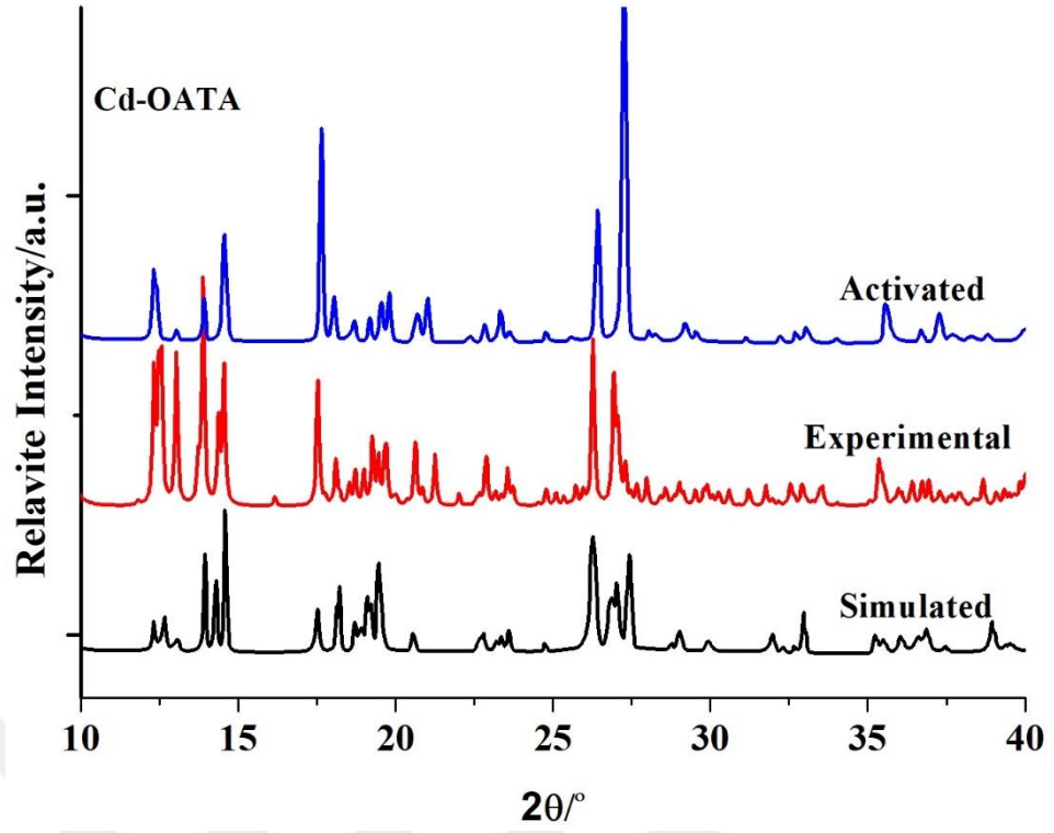
Şekil 4.63: Simüle edilen, deneysel ve aktive edilen Cd-OATA (5)'nın toz XRD desenleri.
