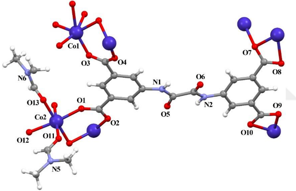
Şekil 4.43: Co-OATA (mor) (6)'un molekül yapısı.
