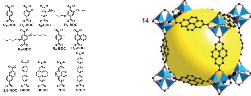
Şekil 1.9: Prototip olarak MOF-5 baz alınarak ligantların değiştirilmesiyle farklı fonksiyoneli MOF'ların hazırlanması (a) kullanılan ligantlar ve (b) MOF yapısı.
