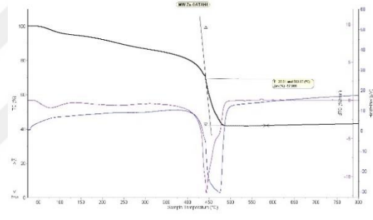
Zn-OATA-MW (10b)
