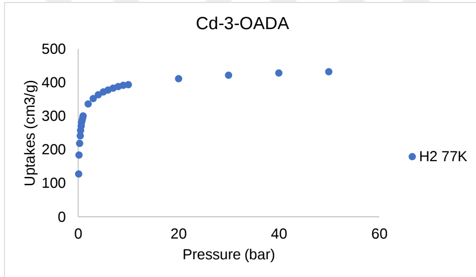
Şekil 4.89: Cd-3-OADA (2)'nin 77 K'de teorik H 2 adsorpsiyon izotermi.
