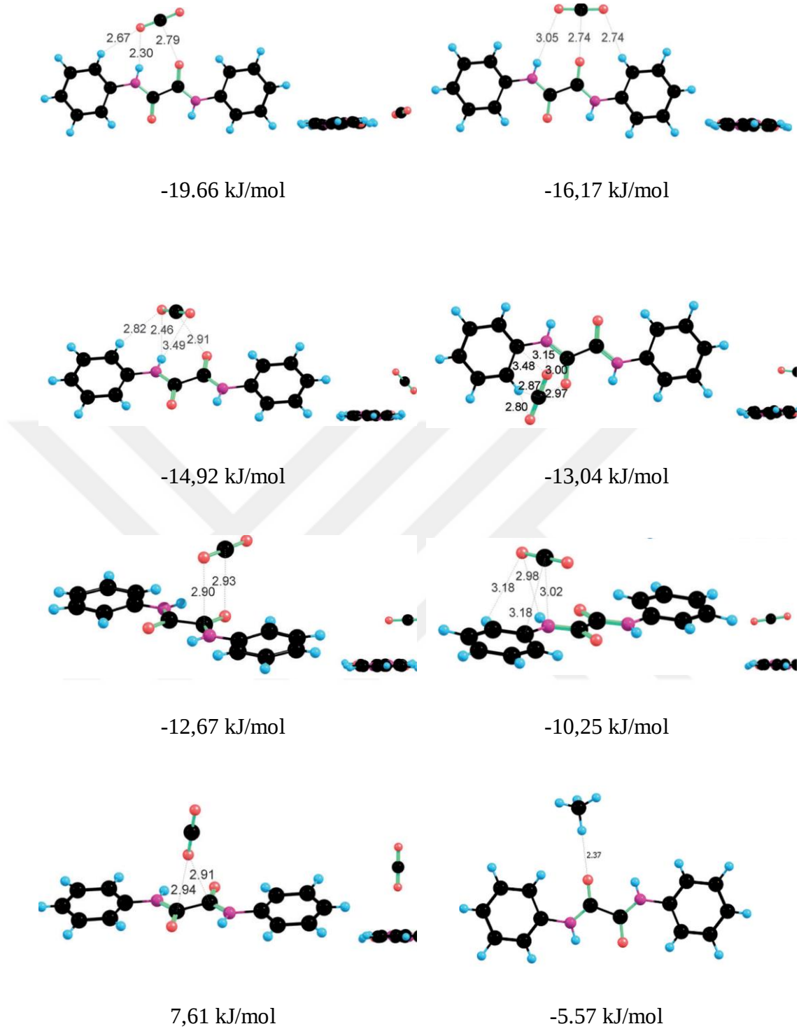
Şekil 2.3: Kafes içerisindeki okzalamit grubu ile adsorplanan CO 2 ve CH 4 arasında meydana gelen etkileşimlerin geometrisi ve bağlanma enerjileri
