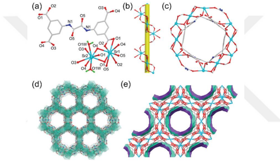
Şekil 2.5: Sr-MOF kafes yapısının gösterimi.
