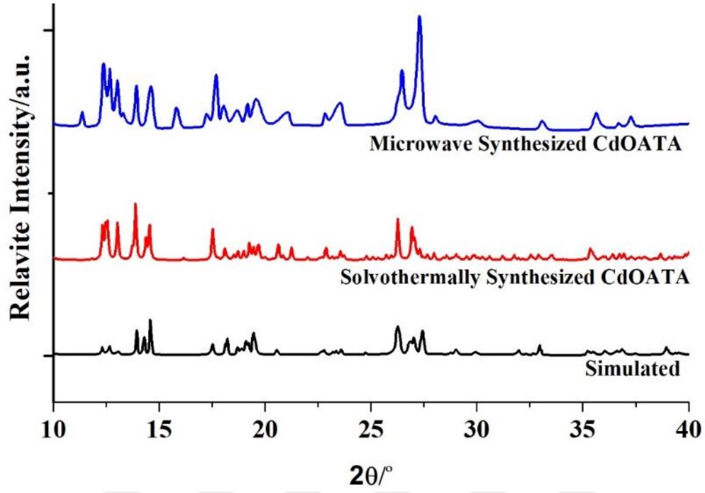
Şekil 4.74: Mikrodalga yöntemiyle sentezlenen Cd-OATA-MW (11) 'nın toz XRD desenleri.
