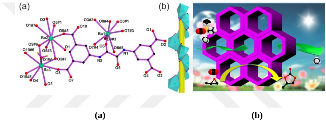
Ş ekil 2.6: Okzalamit ile dekore edilmiş (a) Ba-MOF'nun kristal yapısı ve (b) ilgili makalenin grafiksel özeti.
