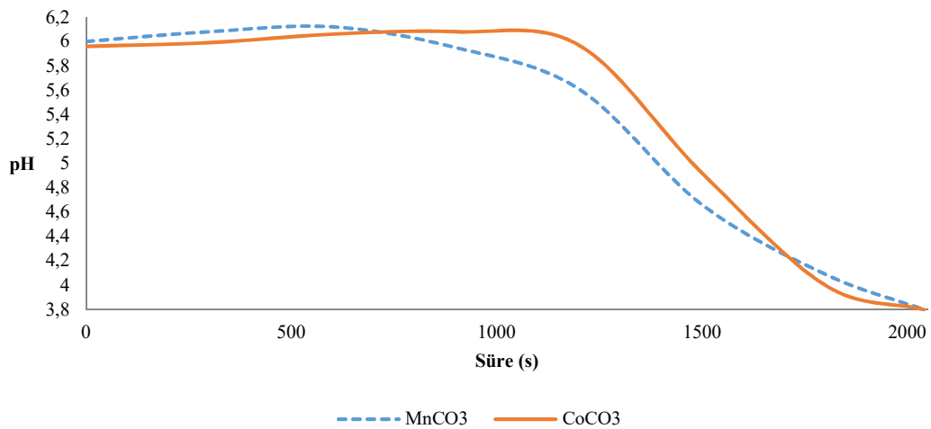
Şekil 40. \text{MnCO}_3 katkılı olan PVC hamuru ile \text{CoCO}_3 katkılı PVC hamurundan elde edilen plastik malzemelerin termostatik kararlılık eğrilerinin karşılaştırılması
