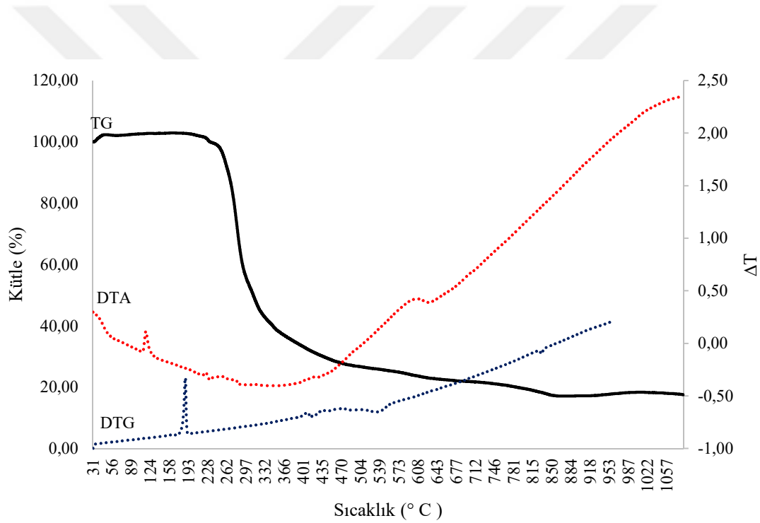
Şekil 4.32. 3.2 kompleksinin termal bozunma eğrileri
