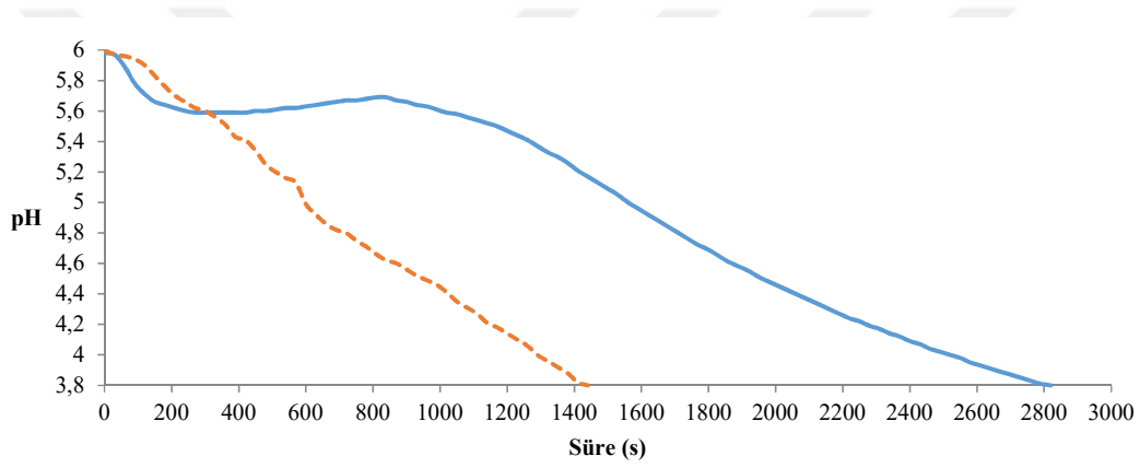
Şekil 4.39. Referans bileşik ile \text{NiCO}_3 \cdot n\text{H}_2\text{O} katkılı PVC hamurunun dehidroklorizasyon eğrileri.
