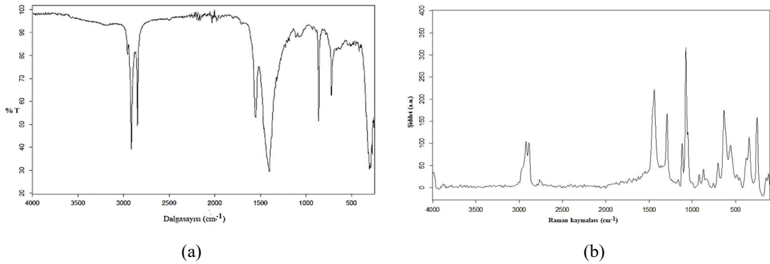
Şekil 4.18. 1.3 kompleksinin FT-IR (a) ve Raman (b) spektrumu
