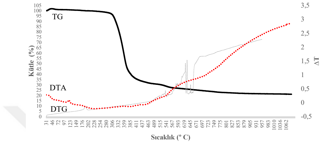
Şekil 4.25. 1.1 kompleksinin termal bozunum eğrileri
