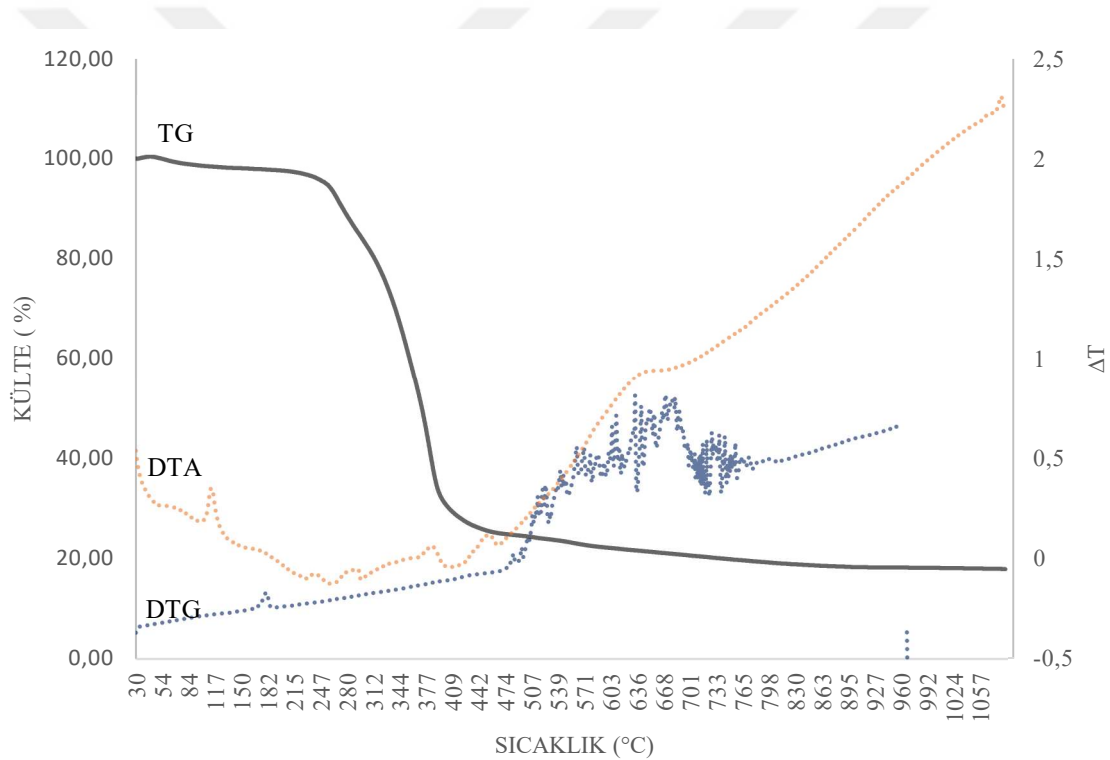
Şekil 4.27. 1.3 kompleksinin termal bozunum eğrileri
