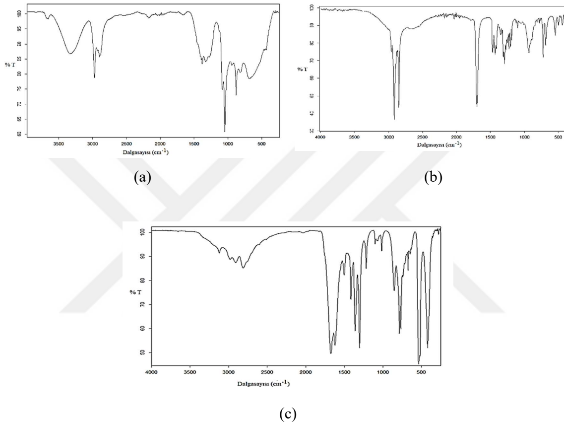
Şekil 4.15. Sodyum tetraborat ( \text{Na}_2\text{B}_4\text{O}_7 \cdot 10\text{H}_2\text{O} ) (a), Sodyum stereat (b) ve sodyum barbiturat (c) moleküllerinin FT-IR spektrumu
