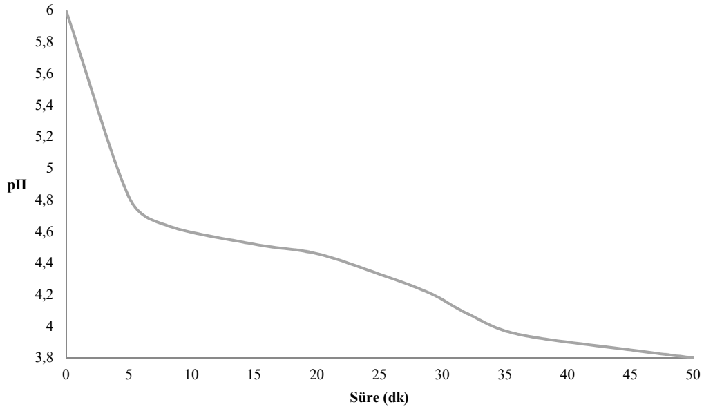
Şekil 4.44. \text{CuB}_4\text{O}_7 \cdot n\text{H}_2\text{O} katkılı PVC hamurunun termostatik kararlık analizi
