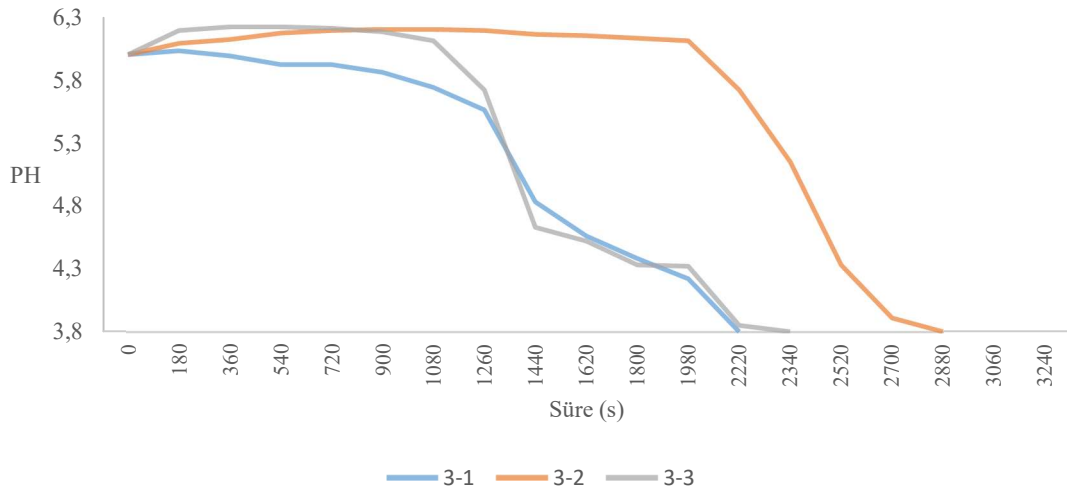
Şekil 4.47. III. Grup kompleksleri katkılı PVC hamurunun termostatik kararlık analizi
