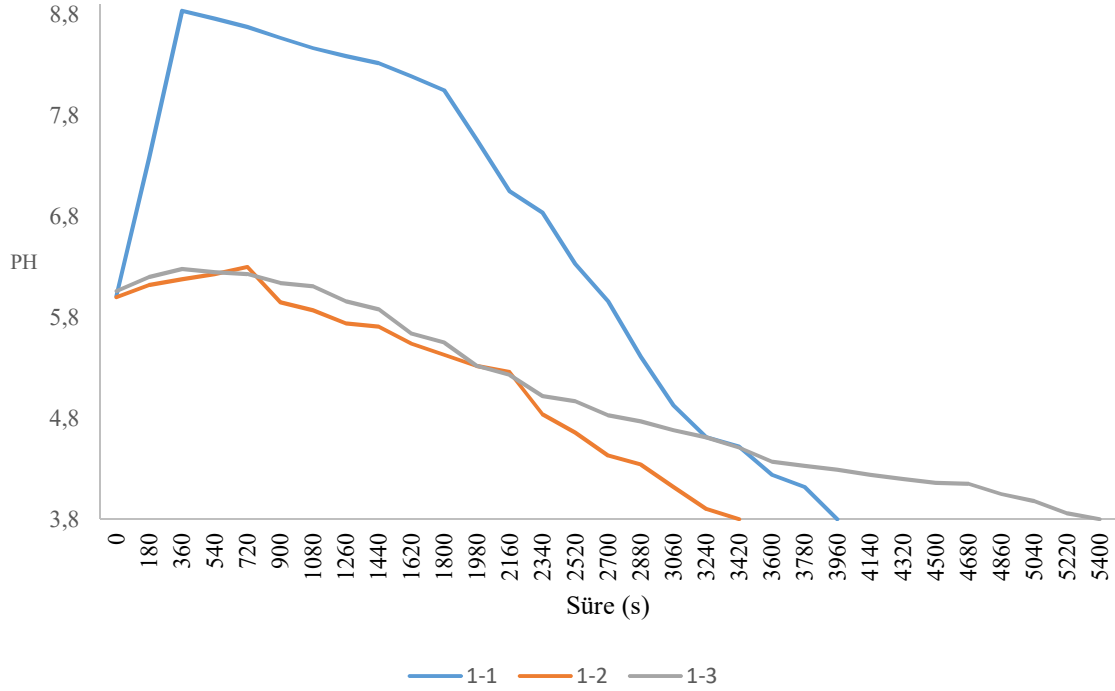
Şekil 4.45. I. Grup kompleksleri katkılı PVC hamurunun termostatik kararlılık analizi
