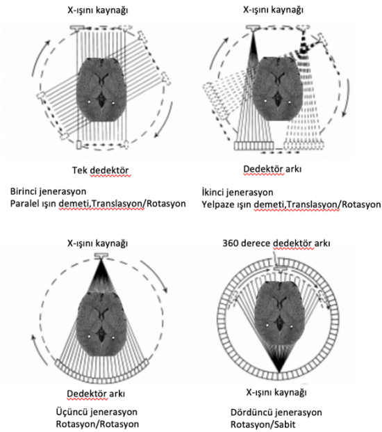
Şekil 1. BT cihazının farklı jenerasyonları
