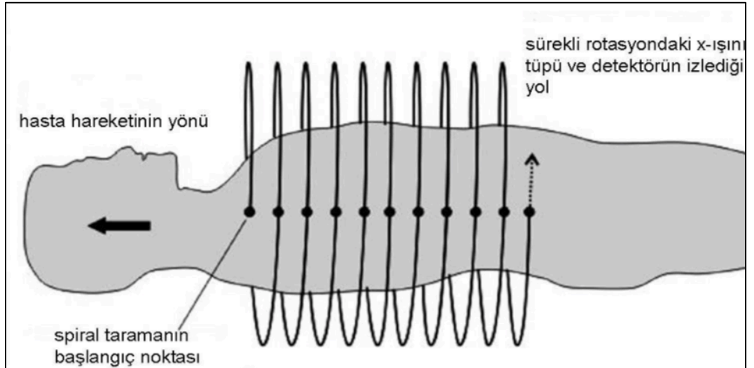
Şekil 2. Spiral BT çalışma prensibi
