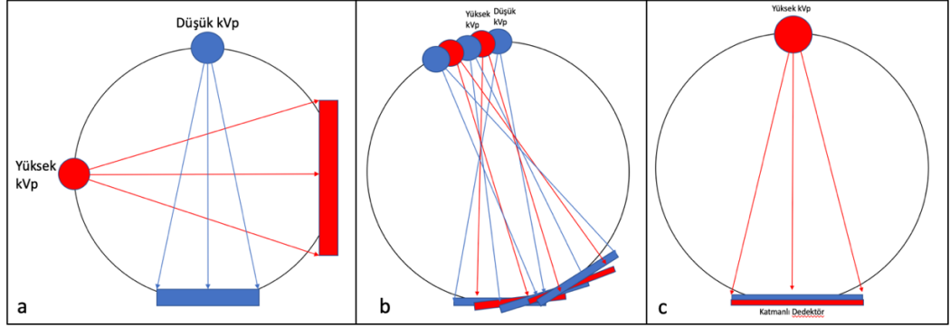
Şekil 6. Farklı çalışma prensibine sahip DEBT sistemleri şematik gösterim. a- Çift kaynaklı DEBT, b- Hızlı kVp değiştiricili DEBT, c-Katmanlı Dedektörlü DEBT
