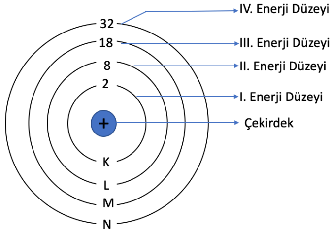
Şekil 8. Atomun enerji seviyeleri
