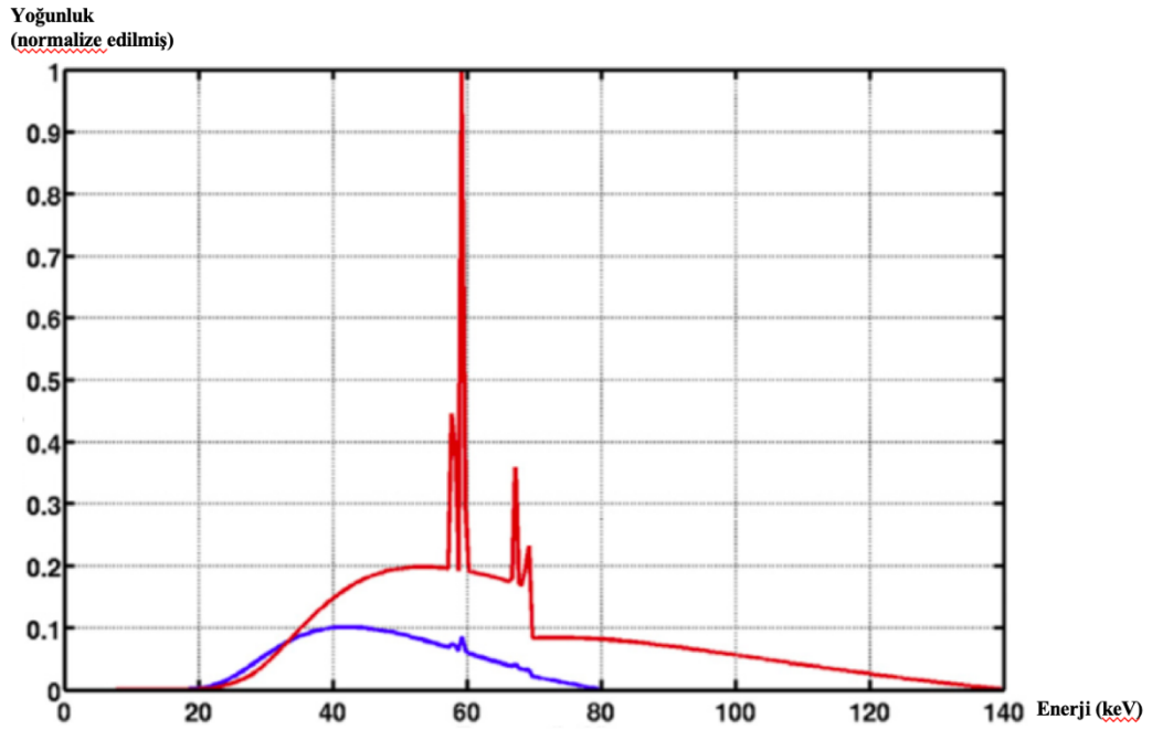
Şekil 7. 80 ve 140 kVp'de polikromatik X-ışını spektrumu
