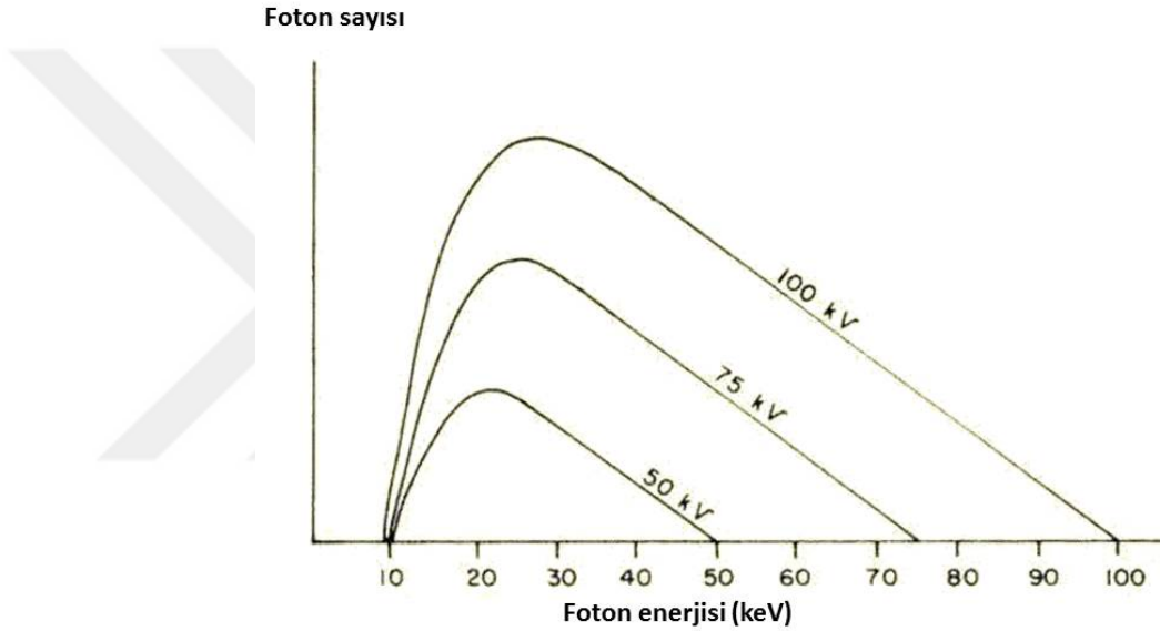
Şekil 10. Foton enerjilerinin dağılımı
