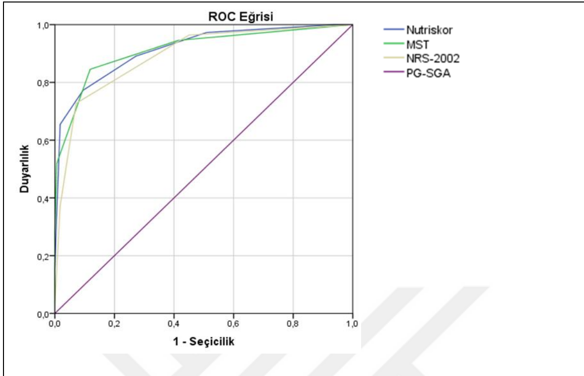
Şekil 4.4. Nutriskor, MST ve NRS-2002 sonuçlarının PG-SGA ile karşılaştırmasını gösteren ROC eğrisi
