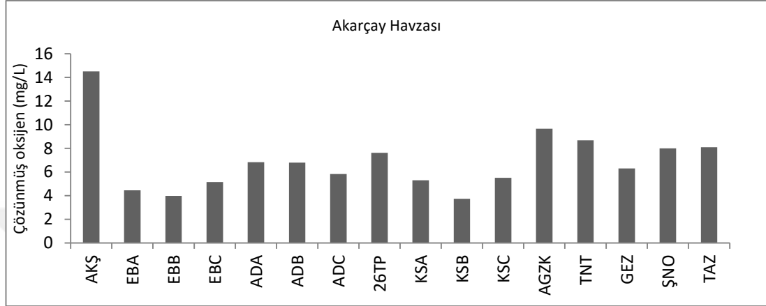
Şekil 4.4. Akarçay Havzası Gölleri'ndeki noktalarda ölçülen çözünmüş oksijen miktarı değerleri
