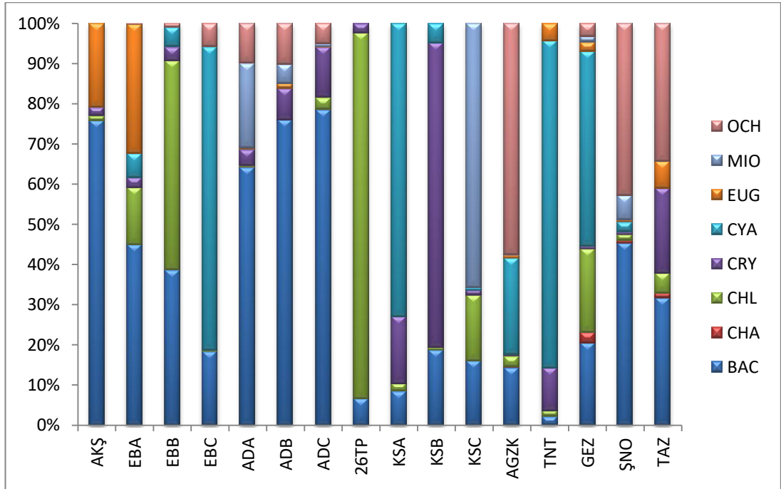
Şekil 4.20. Akarçay Havzası Gölleri’ndeki noktalarda belirlenen fitoplankton gruplarının yüzdelik dağılımı
