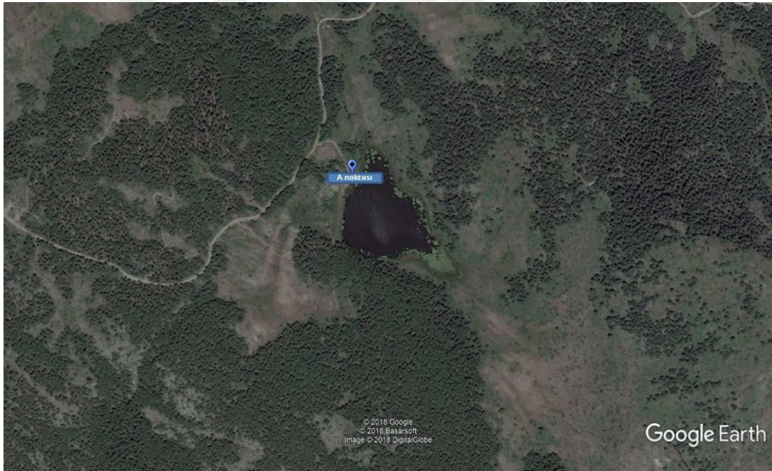
Şekil 3.17. Cüneyt Sönmez Göleti uydu görüntüsü ve A noktasının konumu
