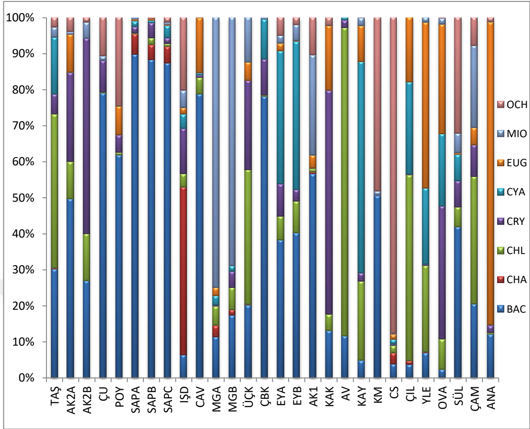
Şekil 4.19. Sakarya Havzası Gölleri’ndeki noktalarda belirlenen fitoplankton gruplarının yüzdelik dağılımı
