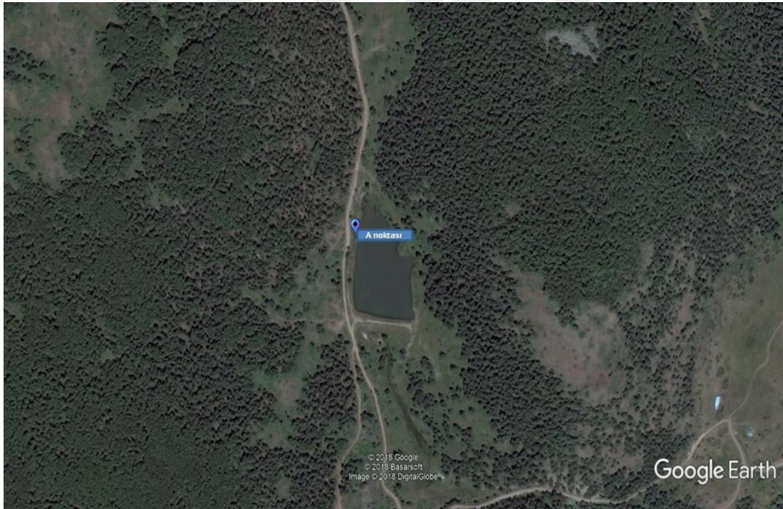
Şekil 3.18. Çılgınlar Göleti uydu görüntüsü ve A noktasının konumu
