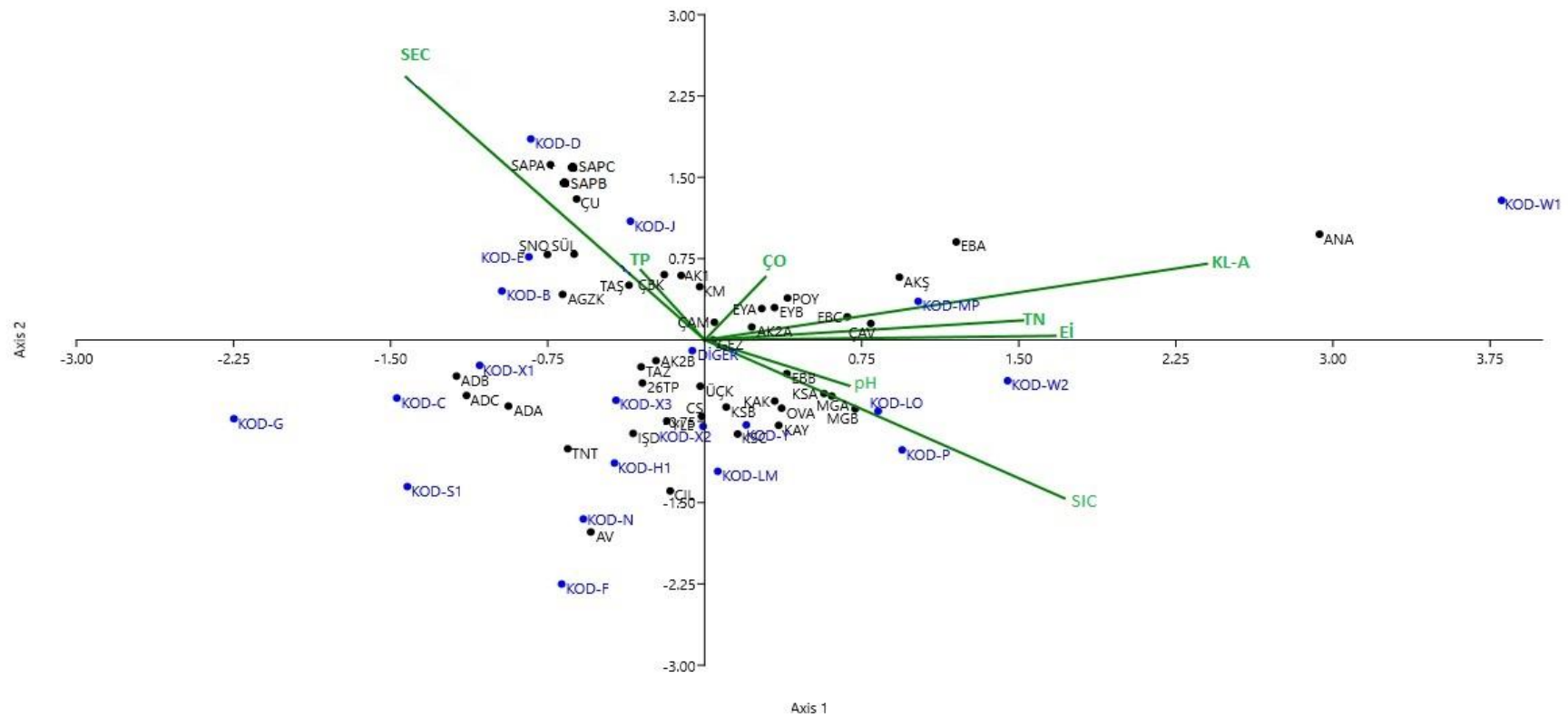
Şekil 4.26. Baskın fitoplankton kodonları ile çevresel değişkenlere uygulanan Kanonin Uyum Analizi (CCA) . Çevresel değişkenler (Eİ; elektriksel iletkenlik, KL-A; klorofil – a, ÇO; çözülmüş oksijen, TN; toplam azot, TP; toplam fosfor, SEC; secchi diski derinliği, pH, SIC; sıcaklık) yeşil renkle, Kodonlar mavi renkle ve göllere ait istasyonlar ise siyah renkle gösterilmiştir.
