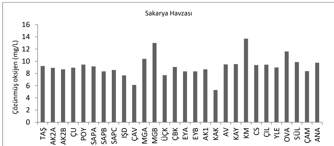
Şekil 4.3. Sakarya Havzası Gölleri'ndeki noktalarda ölçülen çözülmüş oksijen miktarı değerleri
