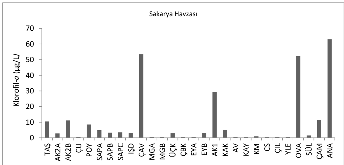
Şekil 4.15. Sakarya Havzası Gölleri'ndeki noktalarda ölçülen klorofil-a değerleri
