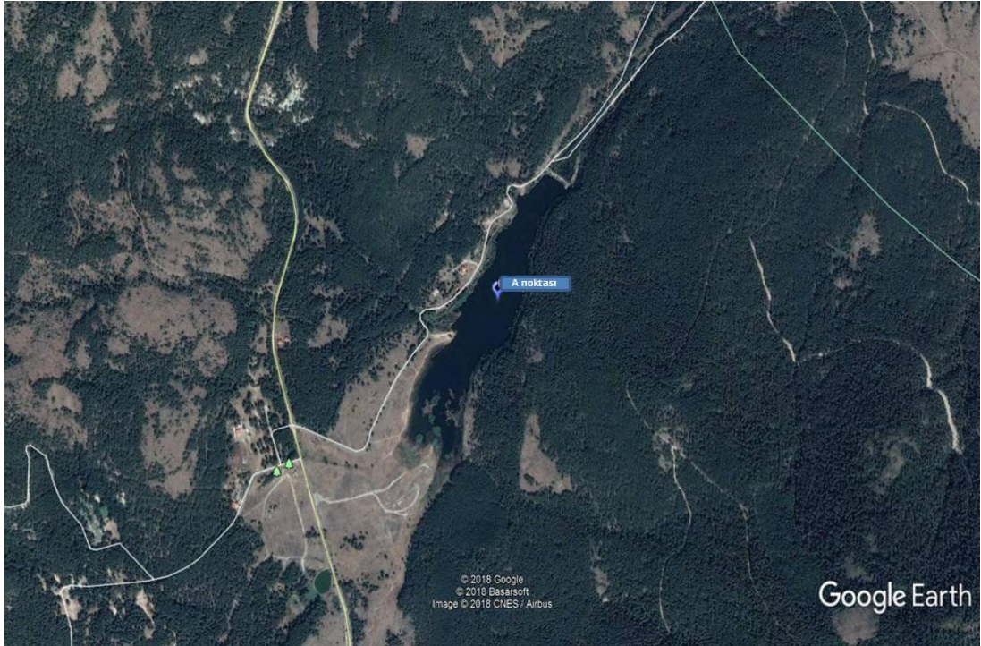
Şekil 3.22. Çamkoru Tabiat Parkı Göleti uydu görüntüsü ve A noktasının konumu
