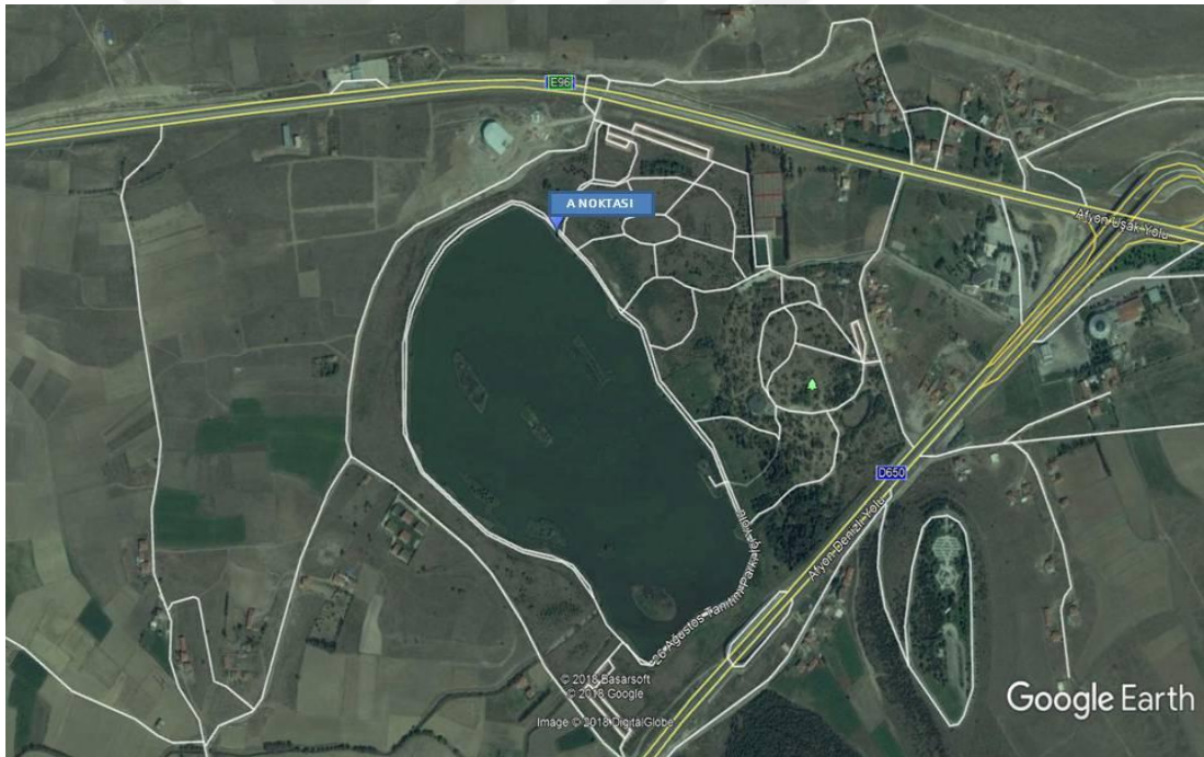
Şekil 3.27. 26 Ağustos Tabiat Parkı Göleti ve A noktasının konumu
