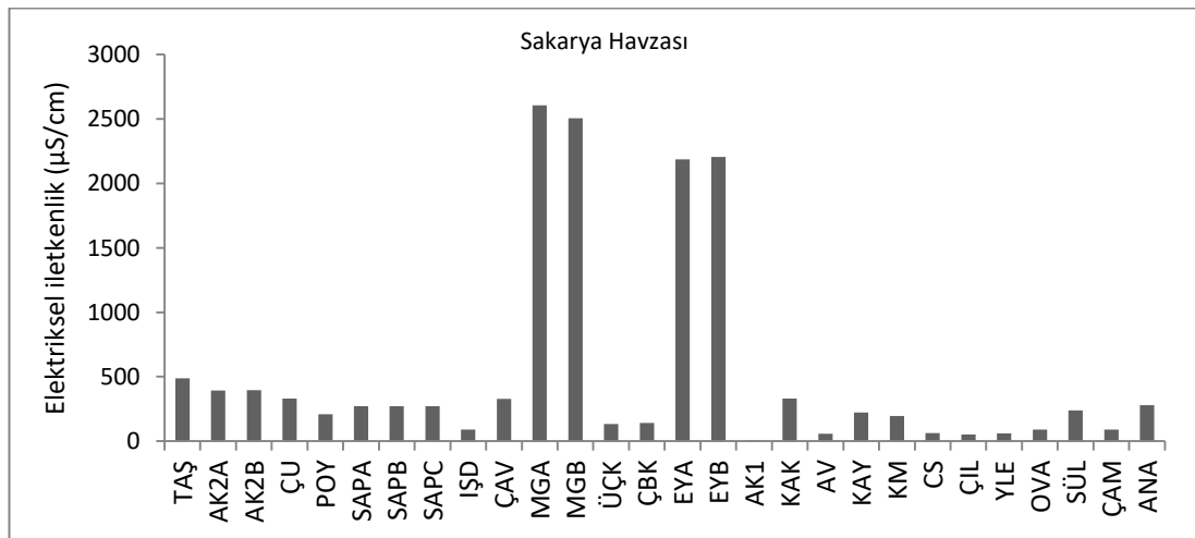
Şekil 4.5. Sakarya Havzası Gölleri'ndeki noktalarda ölçülen elektriksel iletkenlik değerleri
