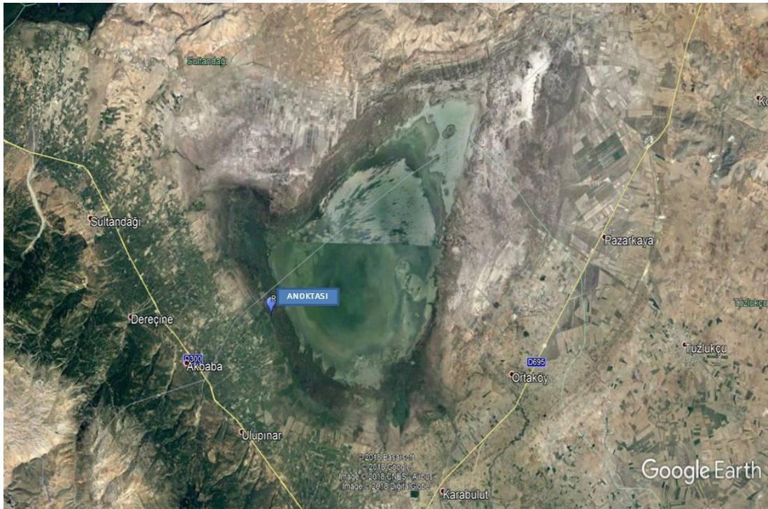
Şekil 3.24. Akşehir Gölü uydu görüntüsü ve A noktasının konumu
