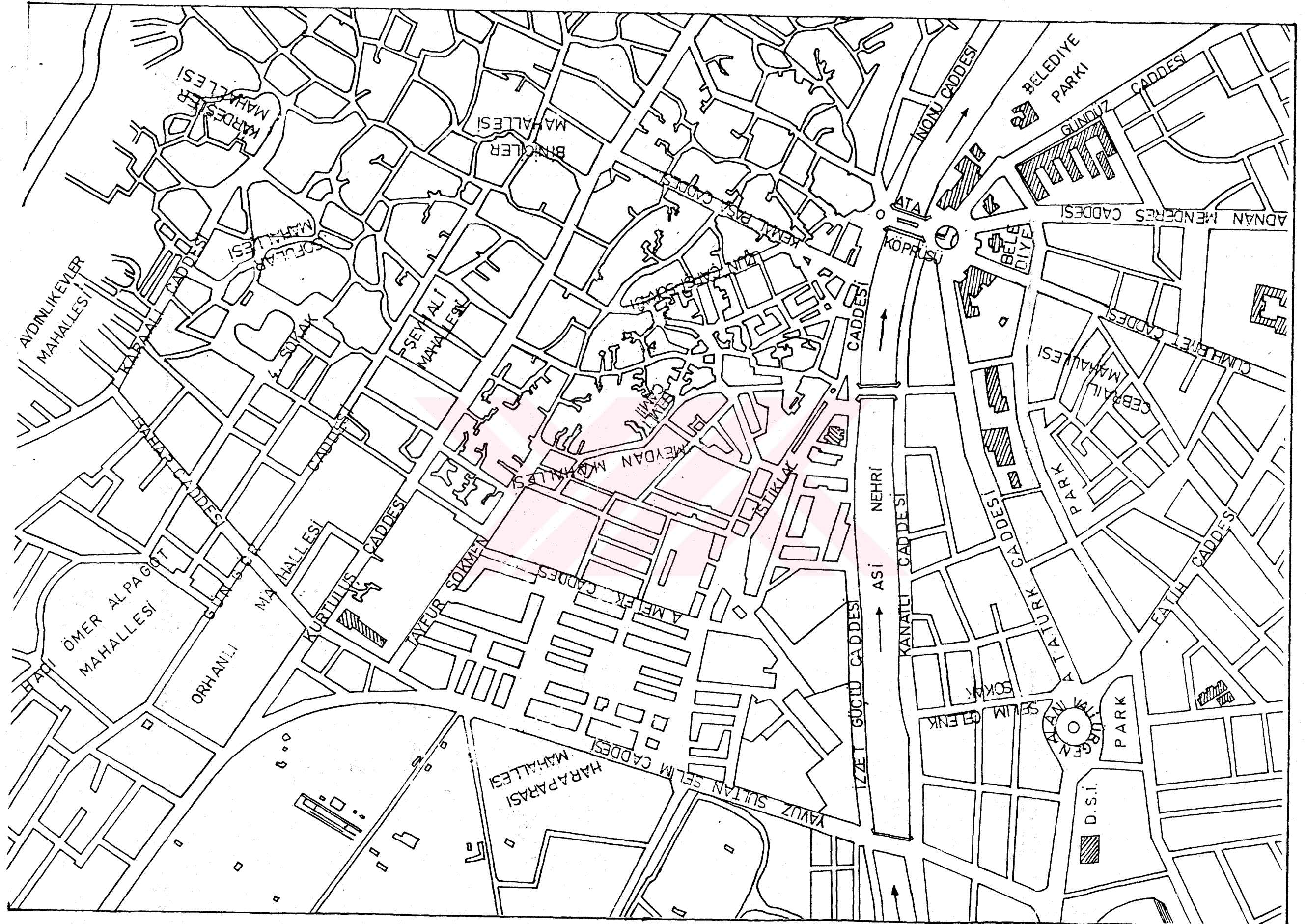
ANTAKYA'NIN KISMİ PLANI Ö:1/5000
