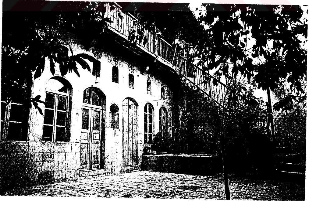
F 20. Avlu cephesi ve üst kata çıkan merdiven (1973)
