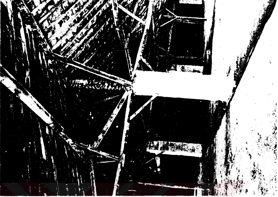
F261. Müftüoğlu Sabunhanesi asma çatı sistemi
