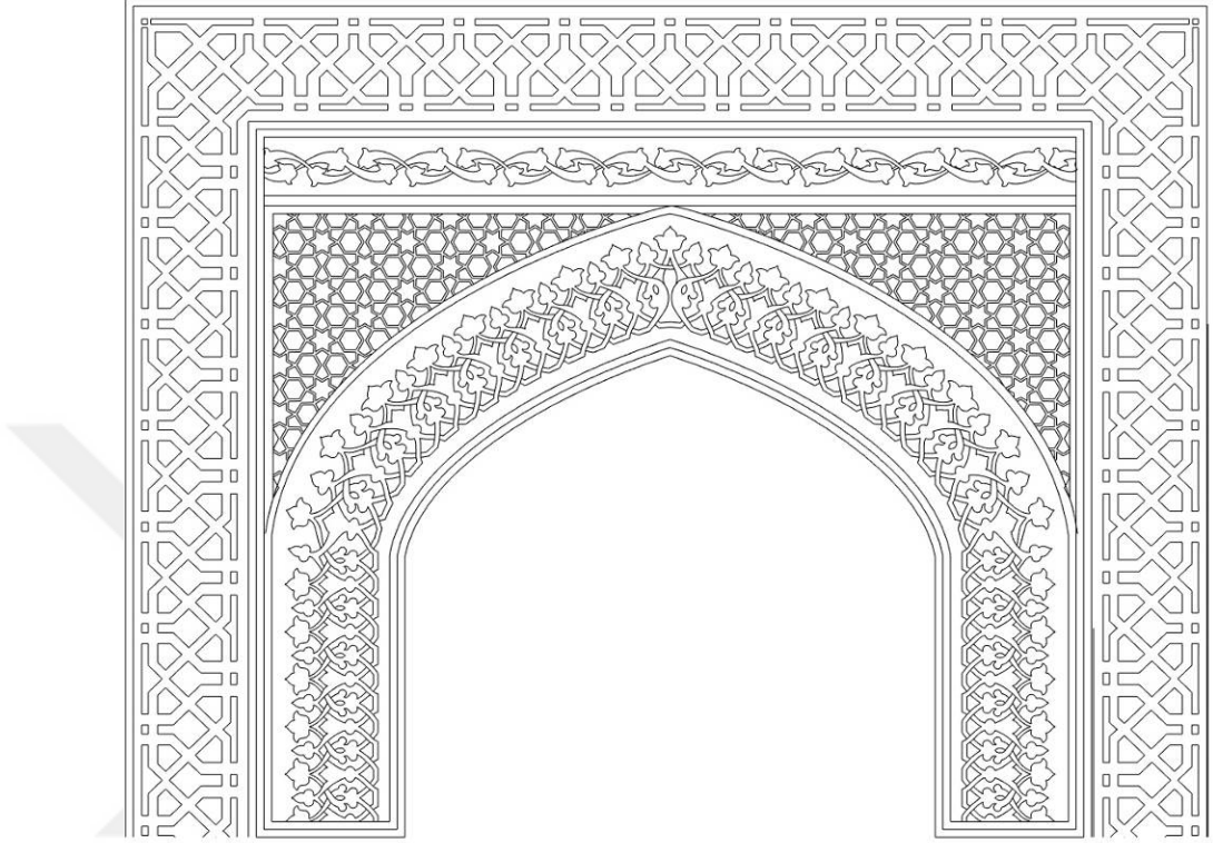
Çizim 68: Batı Duvarı 12 No'lu "Türbe Girişi" Alınlık Panosu
