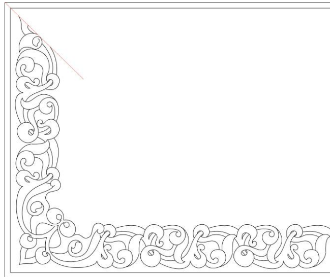
Çizim 33: Taç Kapı Pano Rumi Bordür Köşe Detay Çizimi
