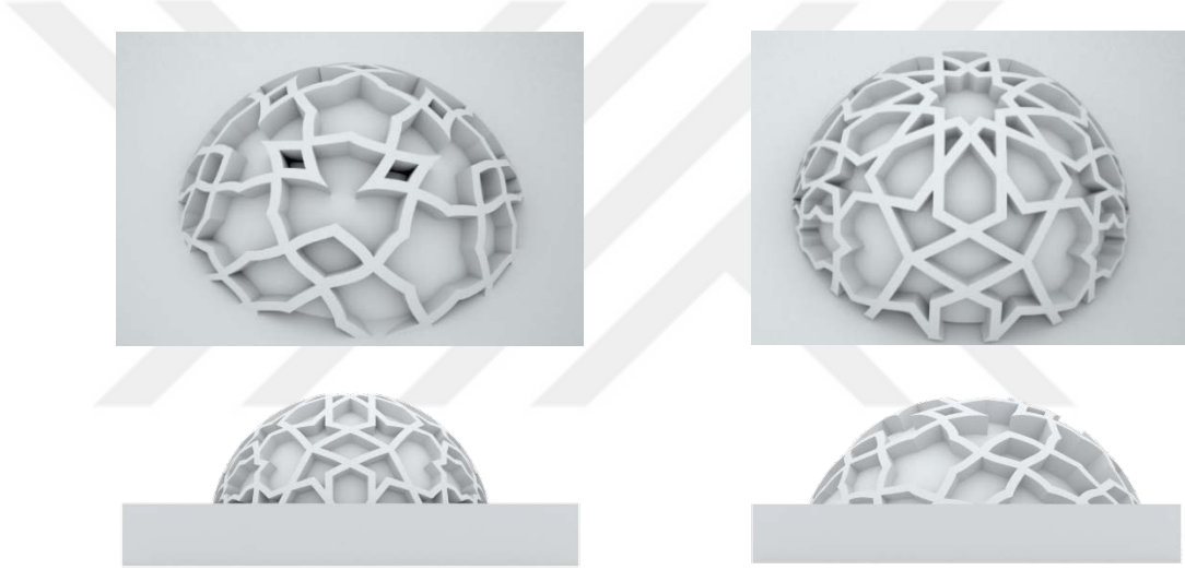
Çizim 35: Taç Kapı Üzerinde Yer Alan Kabaraların, Rhinoceros Programı ile Üç Boyutlu Görselleştirilmesi
