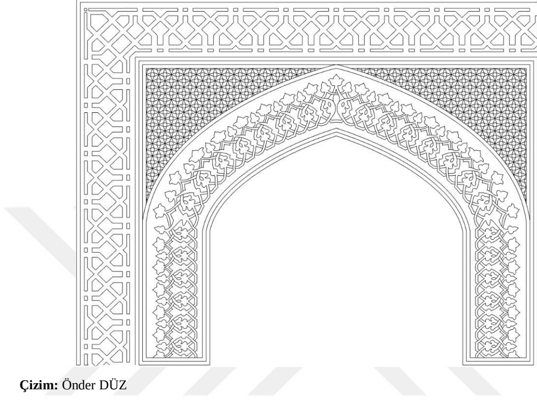
Çizim 54: Doğu Duvarı 4 No'lu İç Kapı Alınlık Panosu
