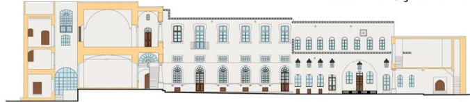
A-A KESİTİ
