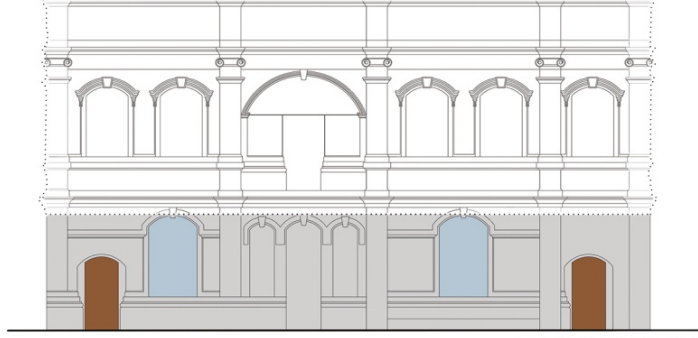
BATI GÖRÜNÜŞ
