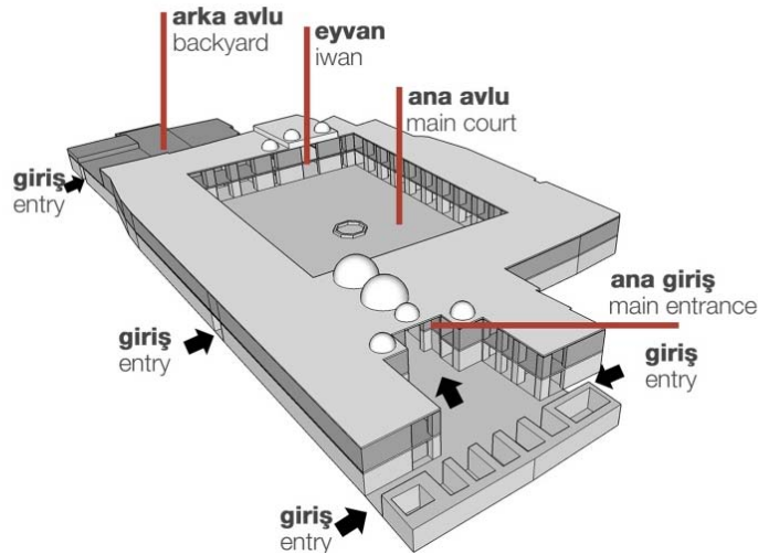
Şekil 3.7; Kortbey Hanın iç fotoğrafları ve modellemesi
