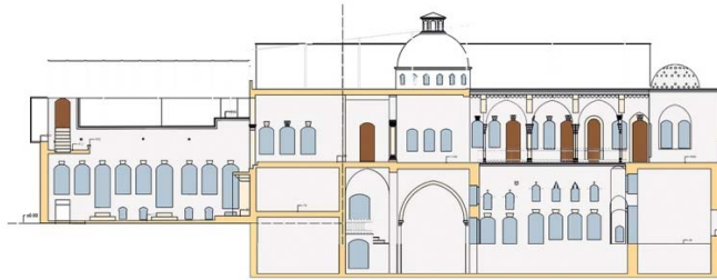
B-B KESİTİ
