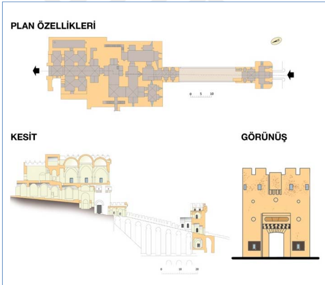
Şekil 3.3; Halep Kalesinin plan özellikleri, kesiti ve görünüşü
