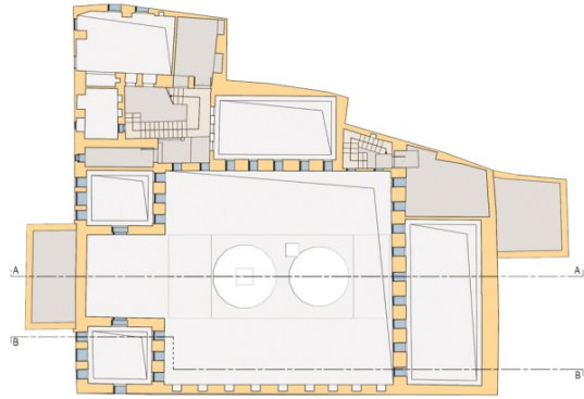
BİRİNCİ KAT PLANI
