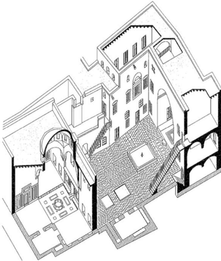
Şekil 3.45; 17. ve 18. yy.'a ait bir Halep geleneksel evin aksonometrik kesiti (Urban Form in The Arap World).
