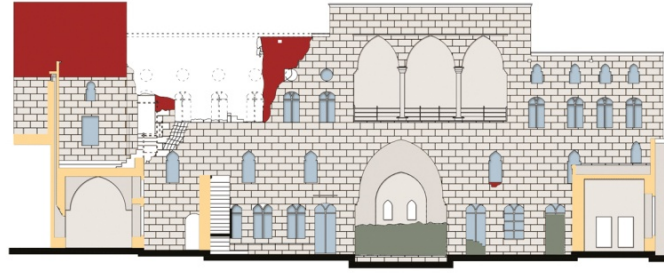
B-B KESİTİ
