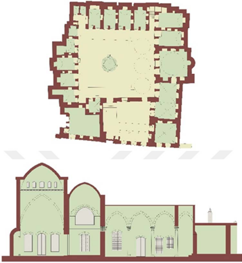
Şekil 3.21; Halep'teki Osmanlı döneminde inşa edilen Ahmediye Medresesi'nin planı ve kesiti
