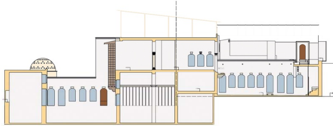
A-A KESİTİ
