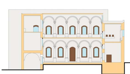
B-B KESİTİ
