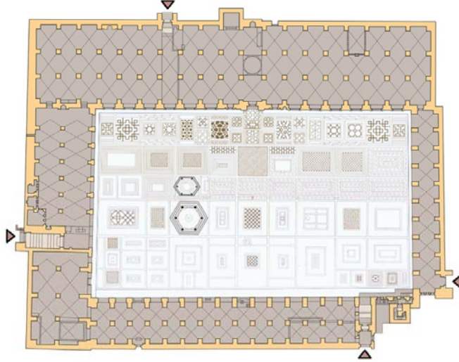
ZEMİN KAT PLANI
