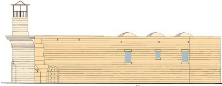
GÜNEY CEPHESİ
