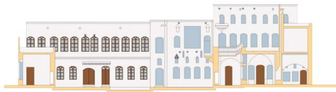
C-C KESİTİ
