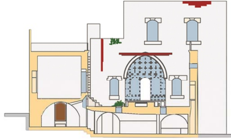
C-C KESİTİ
