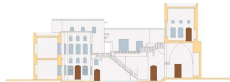
B-B KESİTİ
