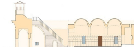
C-C KESİTİ
