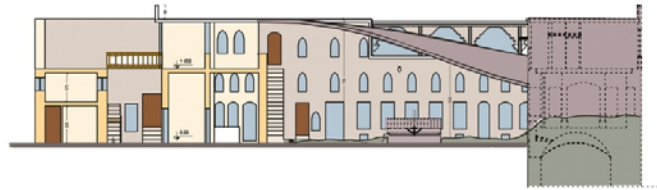
A-A KESİTİ
