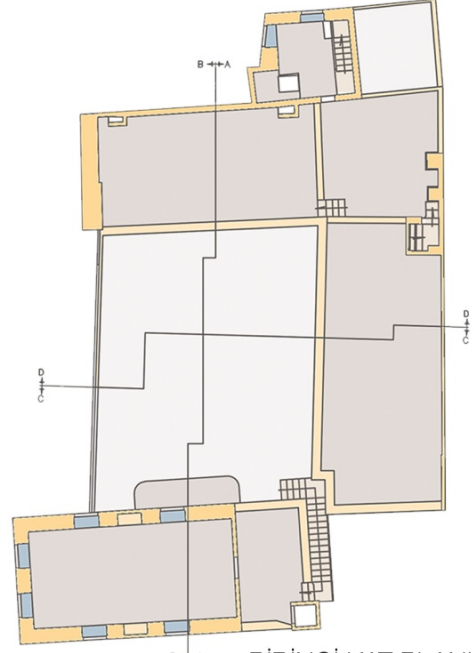
BİRİNCİ KAT PLANI
