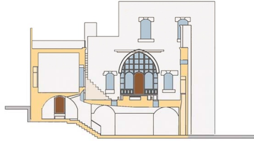
C-C KESİTİ
