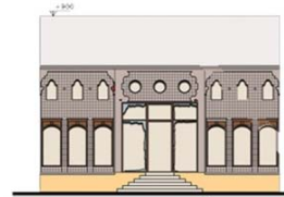
AVLU GÜNEY CEPHE
