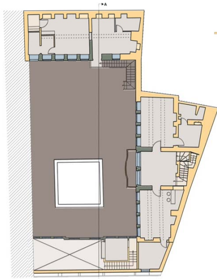
BİRİNCİ KAT PLANI
