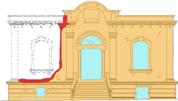
YAN CEPHE
