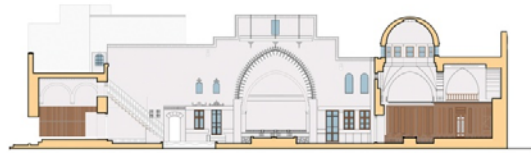
A-A KESİTİ
