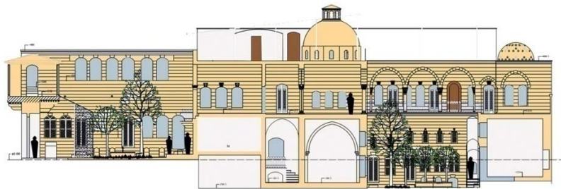
B-B KESİTİ
