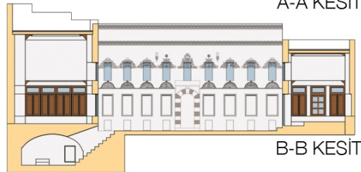
A-A KESİTİ
