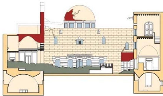
B-B KESİTİ
