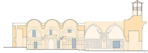
A-A KESİTİ
