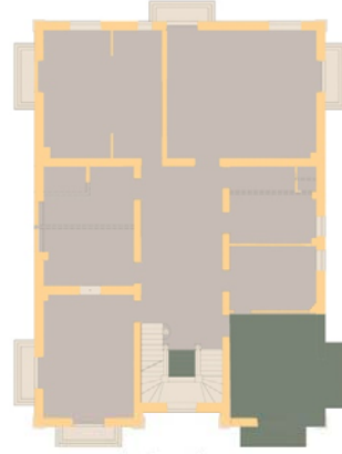
BİRİNCİ KAT PLANI
