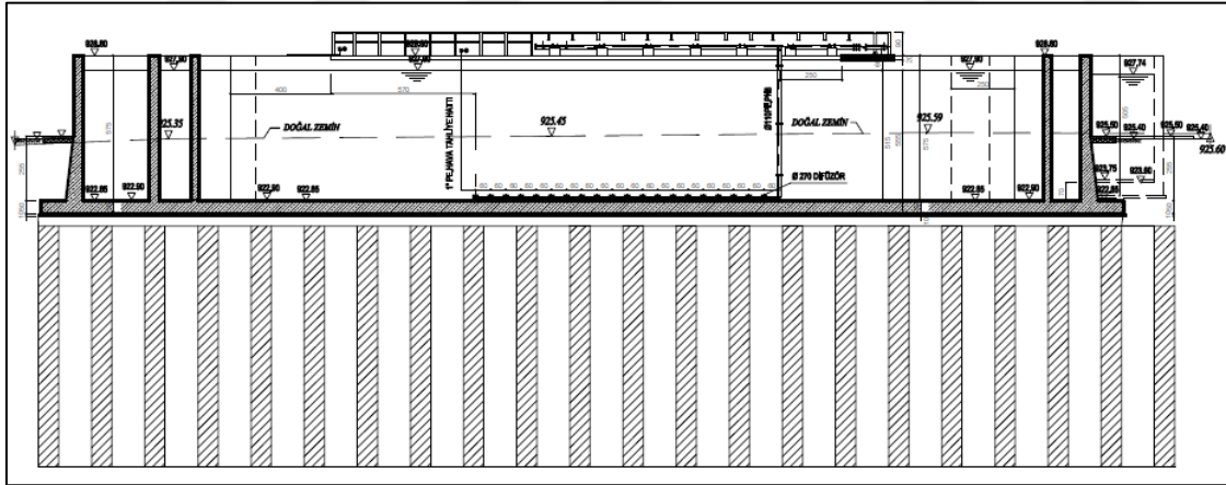
Şekil 6.2. A ve B yapıları altındaki jet grout profili
