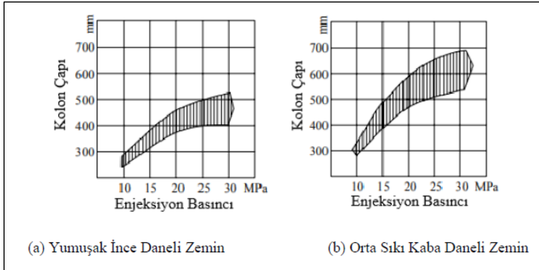
Şekil 2.3. Enjeksiyon basıncı - kolon çapı grafiği [10]
