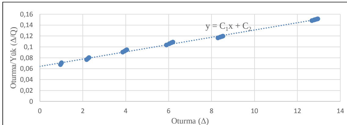
Şekil 3.3. Chin Kondner (1970) yöntemi örneği
