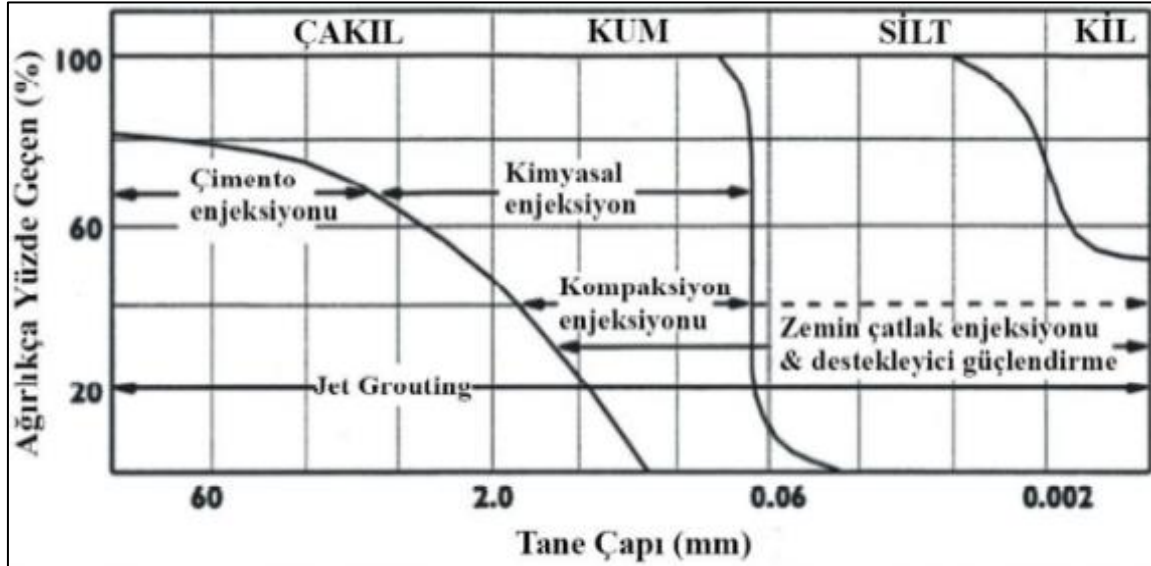
Şekil 2.1. Jet groutun uygulanabildiği zeminler [6]
