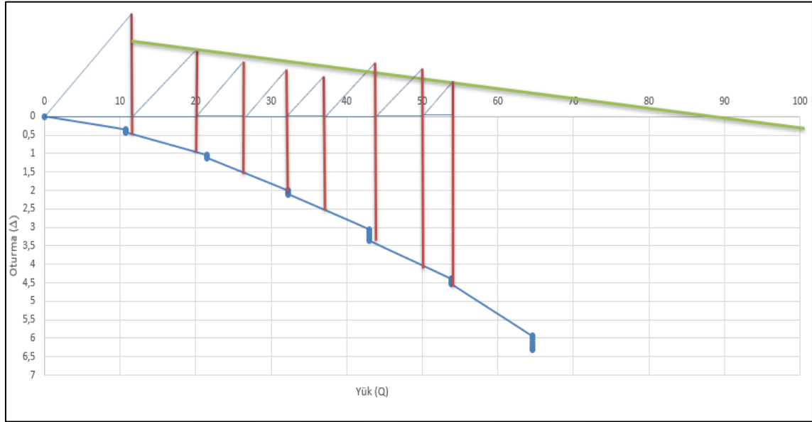
Şekil 39. G kolonu Mazurkiewicz grafiği
