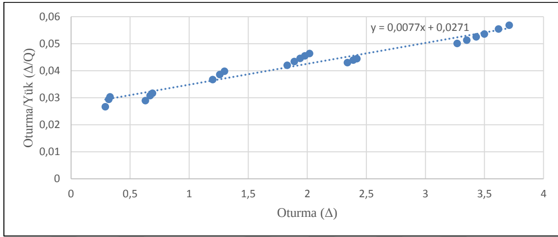
Şekil 19. E kolonu Chin Kondner grafiği
