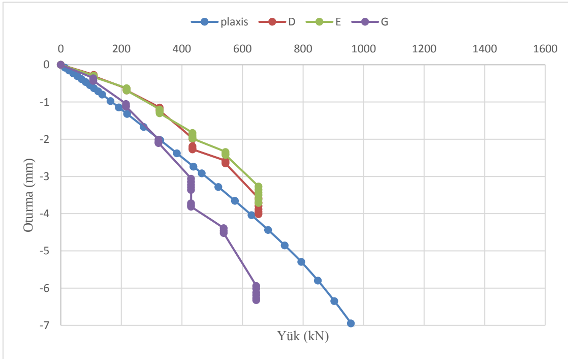
Şekil 50. D,E,G kazık yükleme deneyleri ve Plaxis 3D Foundation yük-oturma grafiklerinin karşılaştırılması
