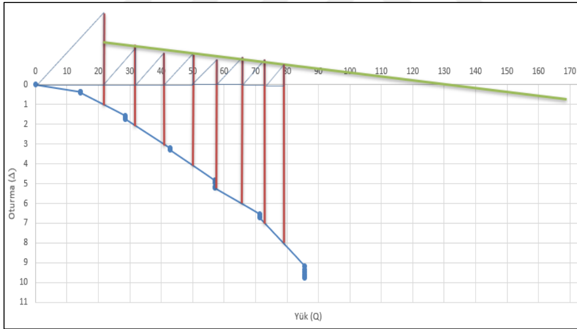
Şekil 32. A2 kolonu Mazurkiewicz grafiği
