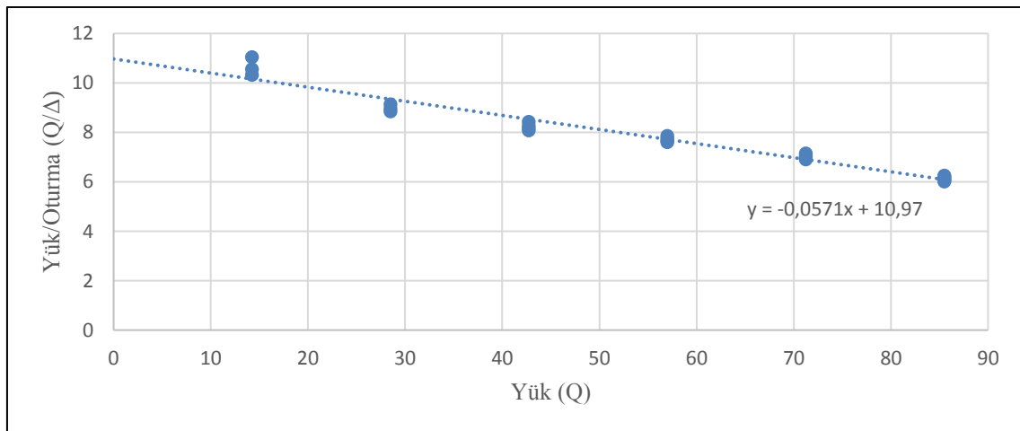
Şekil 24. B1 kolonu Decourt grafiği
