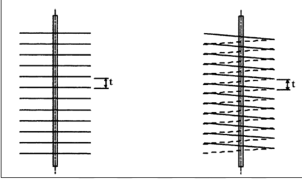
Şekil 2.5. Kademeli çekme (a) - sürekli çekme (b) [12]
