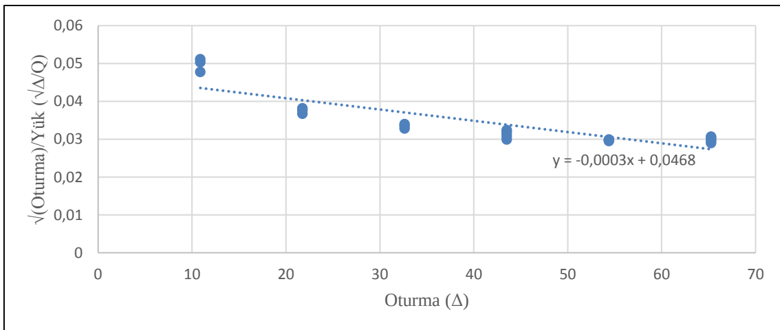
Şekil 9. D kolonu Brinch Hansen grafiği
