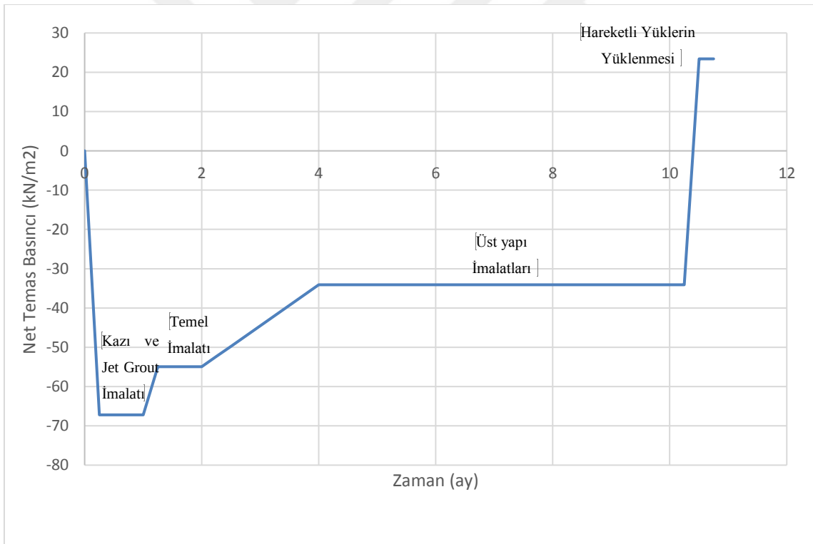
Şekil 6.16. Üst yapı yükü - zaman ilişkisi
