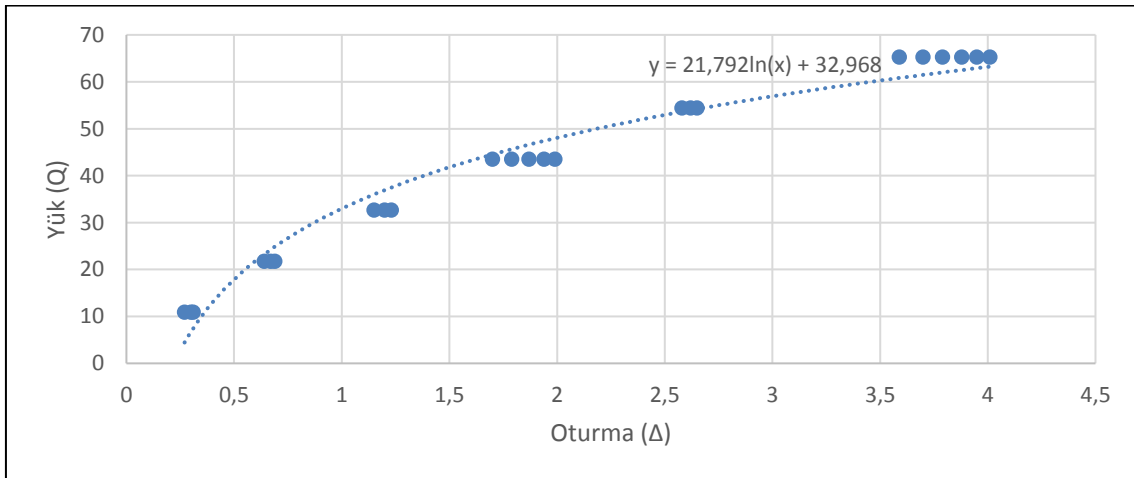
Şekil 45. D kolonu Hirany-Kulhawy grafiği
