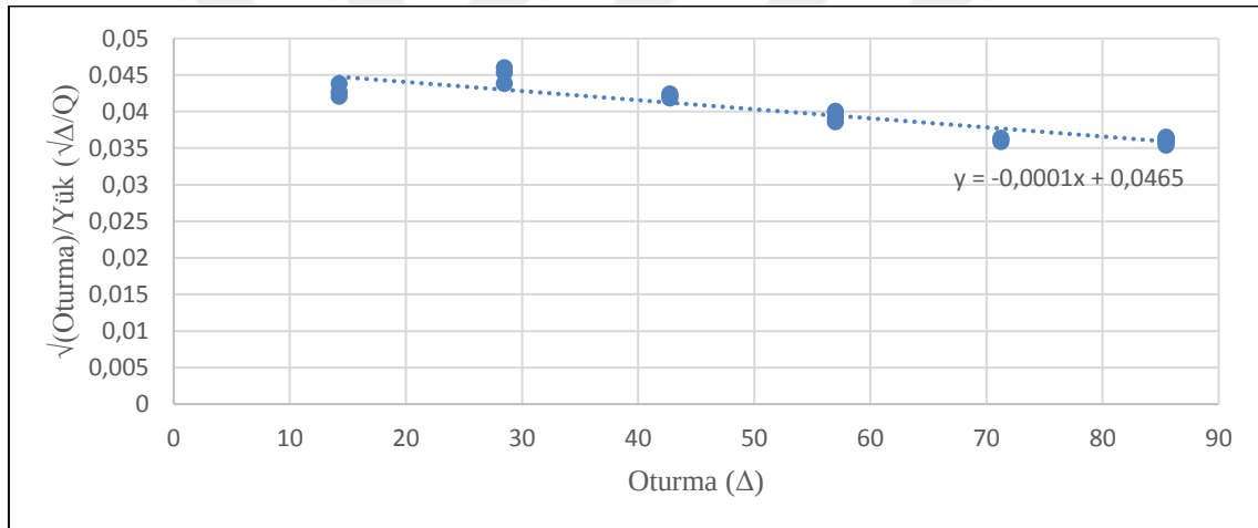
Şekil 5. A2 kolonu Brinch Hansen grafiği
