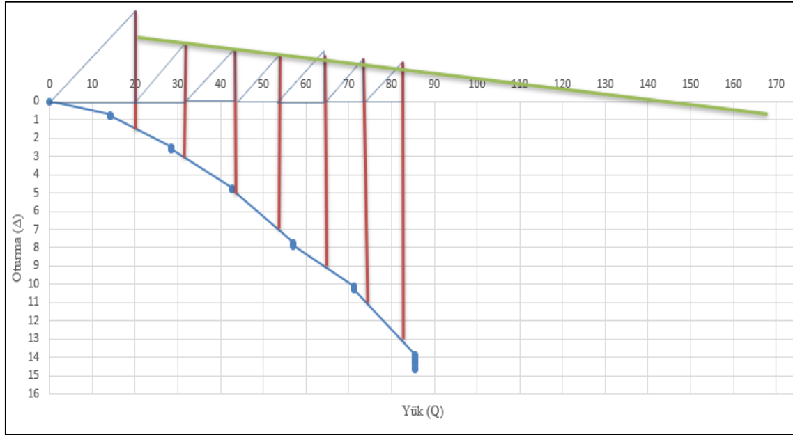
Şekil 31. A1 kolonu Mazurkiewicz grafiği
