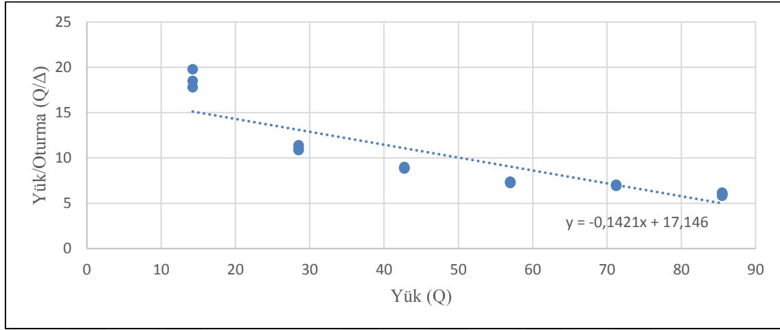
Şekil 22. A1 kolonu Decourt grafiği
