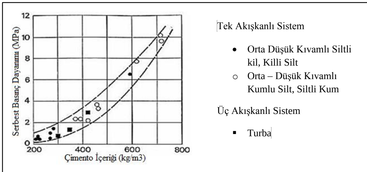
Şekil 2.12. Çimento oranının karot basınç dayanımına etkisi [11]
