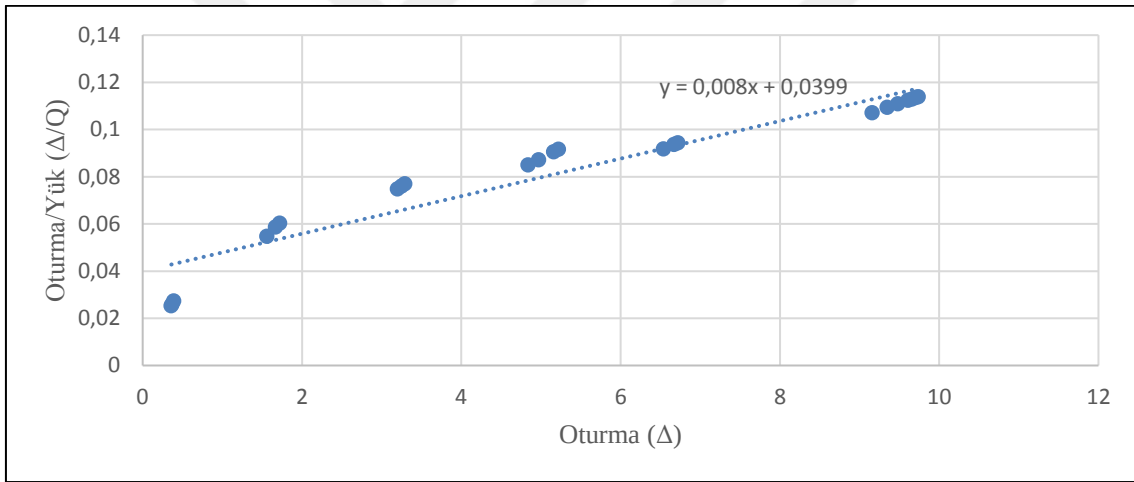
Şekil 14. A2 kolonu Chin Kondner grafiği
