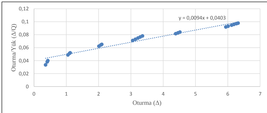
Şekil 21. G kolonu Chin Kondner grafiği
