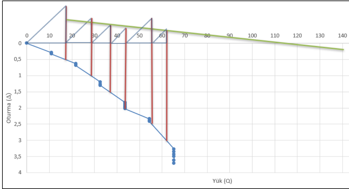
Şekil 37. E kolonu Mazurkiewicz grafiği
