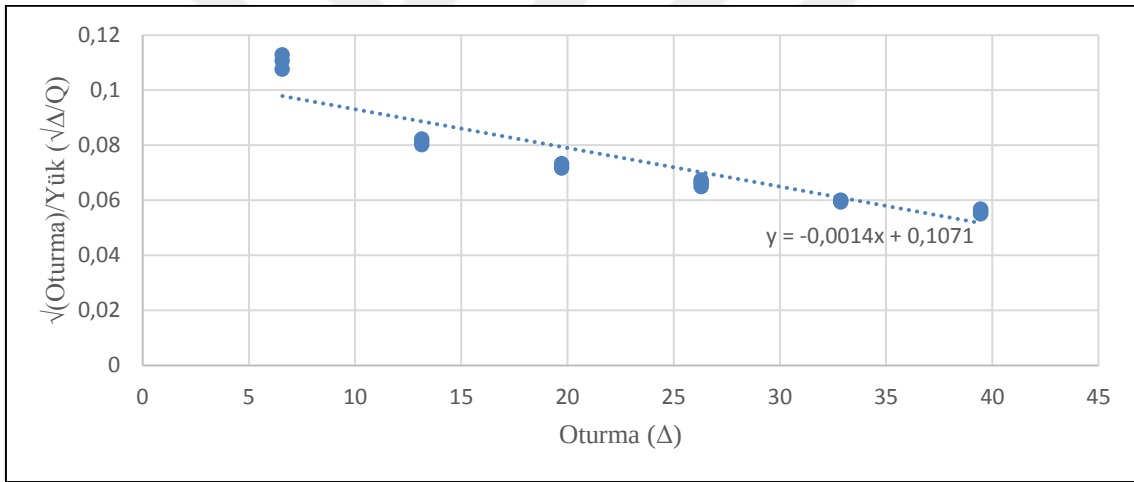
Şekil 11. F kolonu Brinch Hansen grafiği
