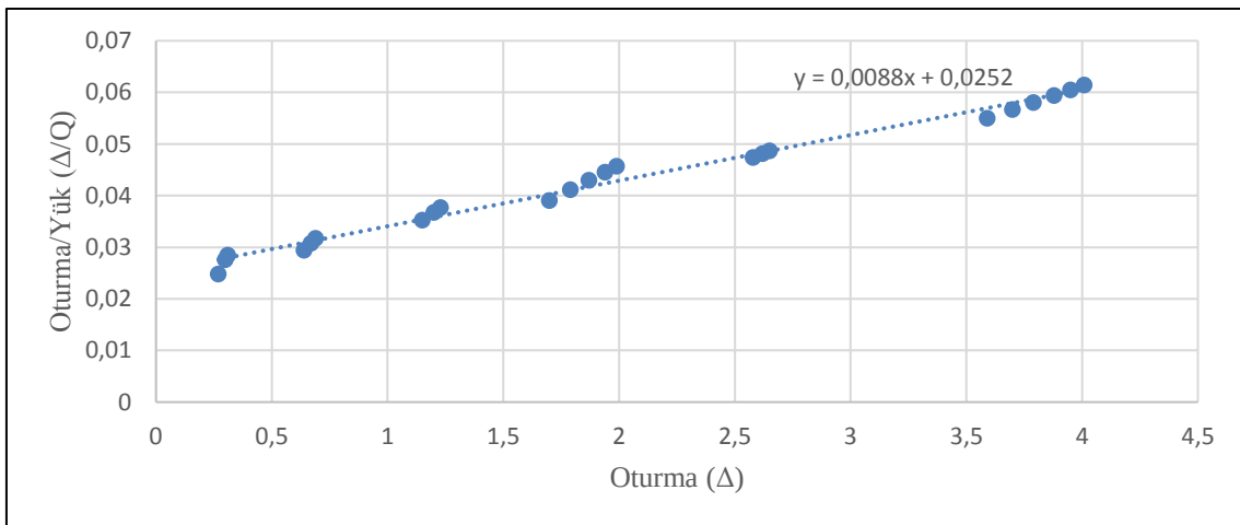
Şekil 18. D kolonu Chin Kondner grafiği
