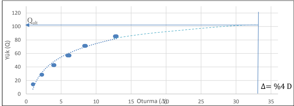
Şekil 3.5. Hirany-Kulhawy (2002) yöntemi örneği
