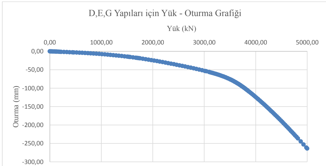
Şekil 6.5. D,E,G yapıları altındaki jet grout modeli için yük-oturma ilişkisi
