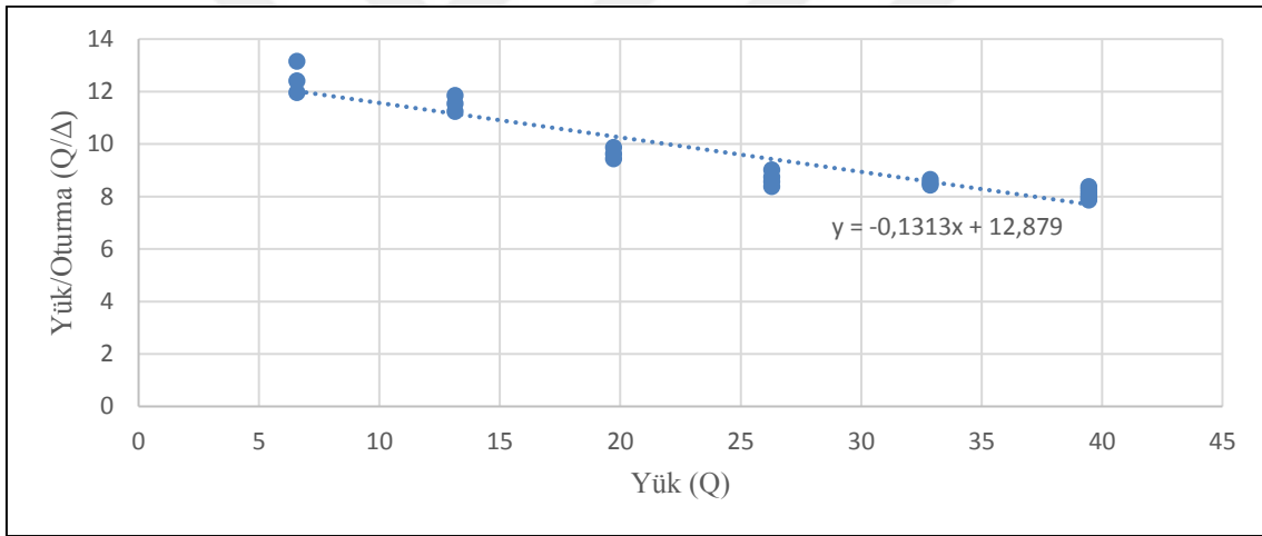
Şekil 29. F kolonu Decourt grafiği
