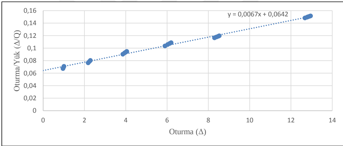
Şekil 17. C kolonu Chin Kondner grafiği
