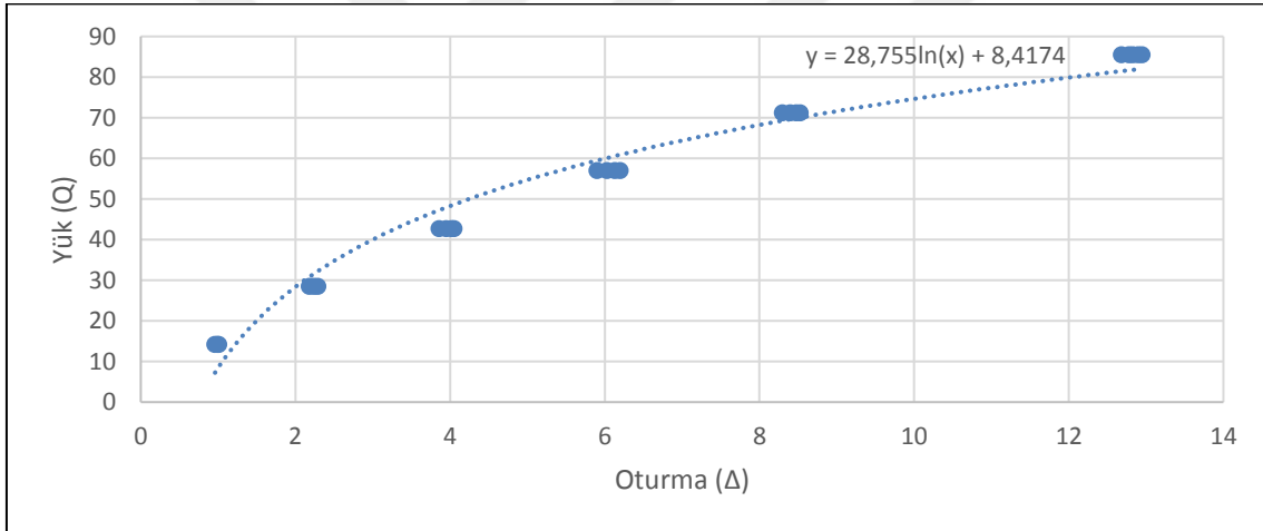
Şekil 44. C kolonu Hirany-Kulhawy grafiği
