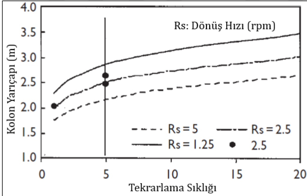
Şekil 2.6. Jet enjeksiyonu için optimum tekrarlama sıklığının deneysel sonuçları [12]
