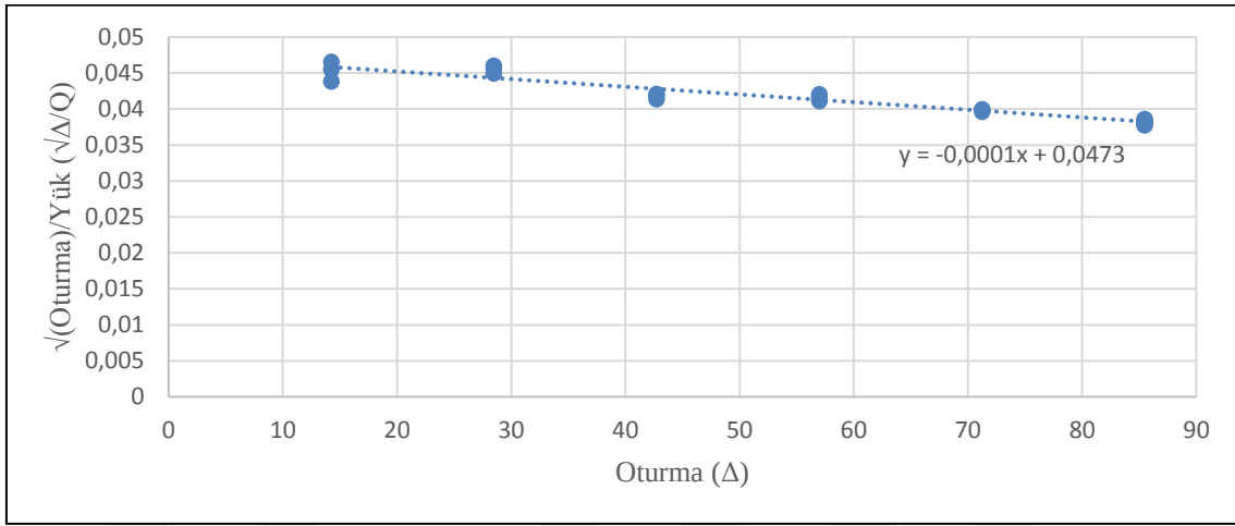
Şekil 7. B2 kolonu Brinch Hansen grafiği
