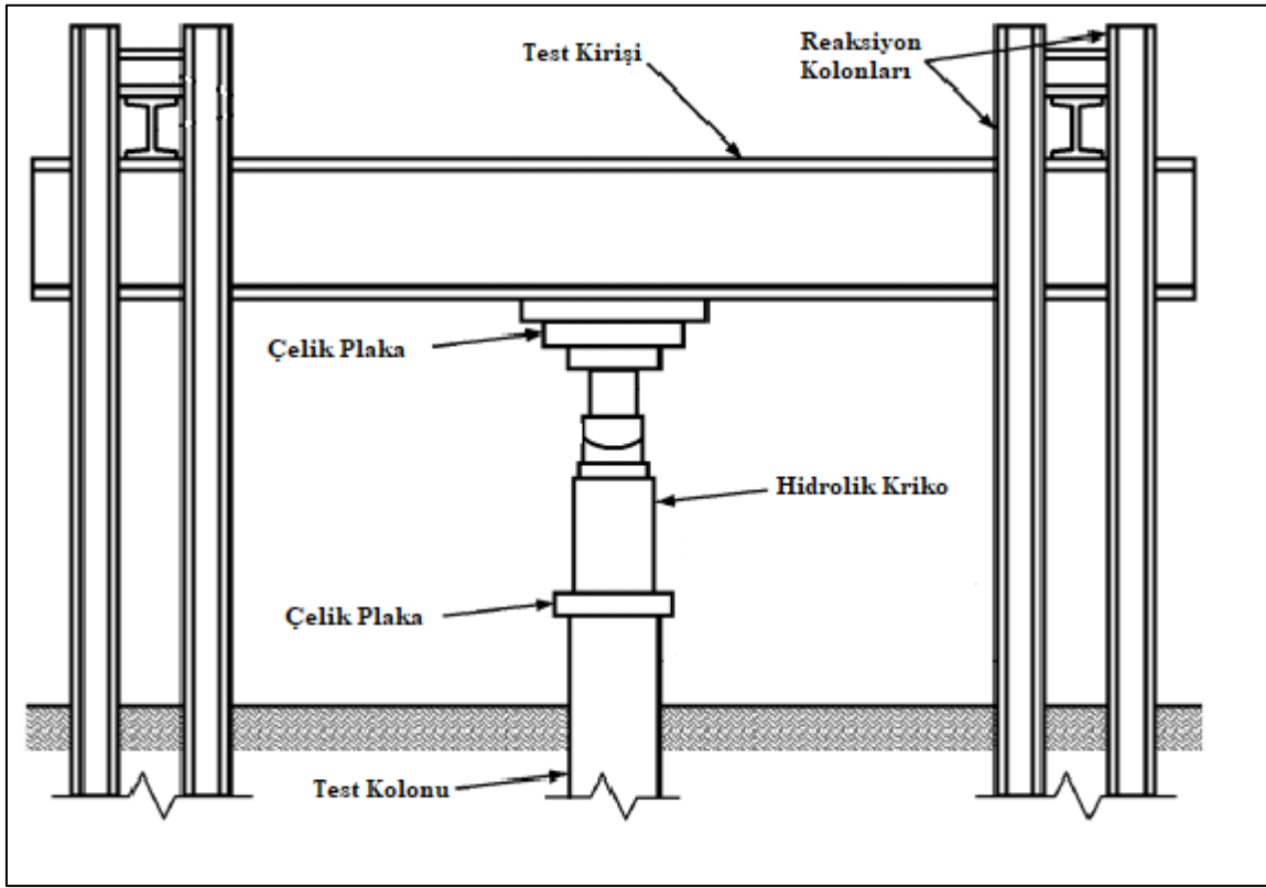
Şekil 2.9. Kazık yükleme deney düzeneği [18]
