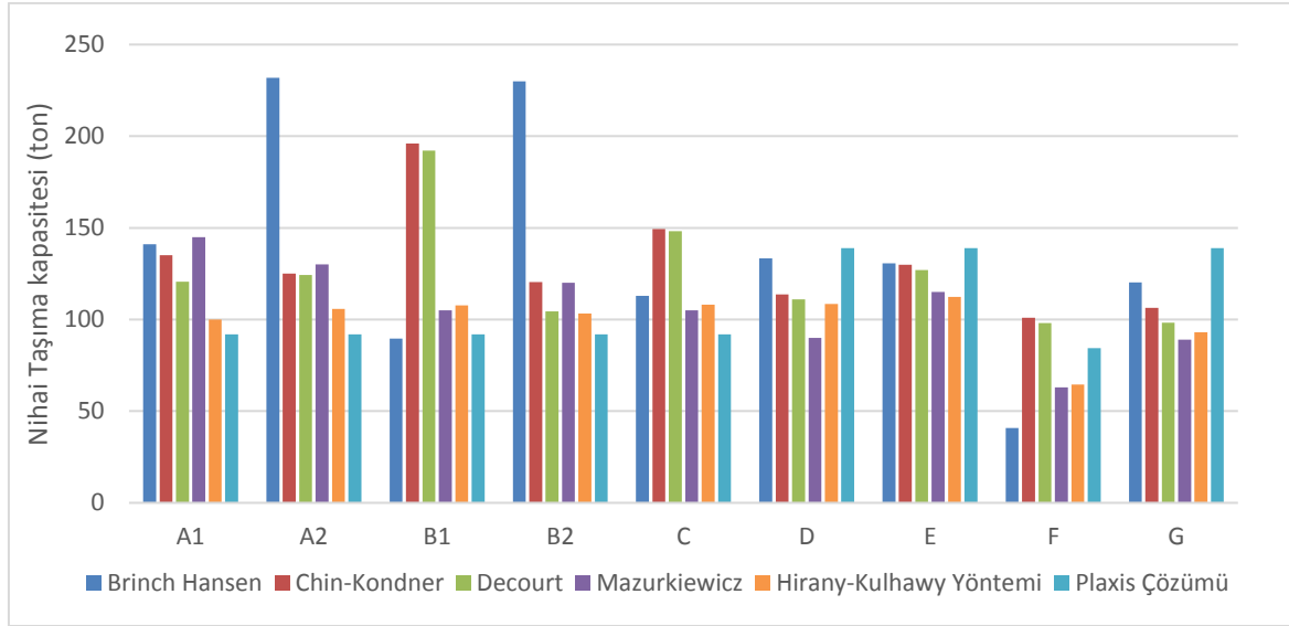
Şekil 6.12. Nihai taşıma kapasitesi hesaplarının karşılaştırılması
