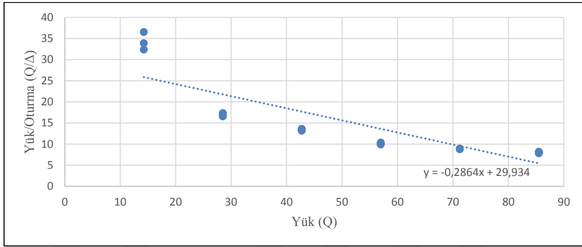
Şekil 25. B2 kolonu Decourt grafiği
