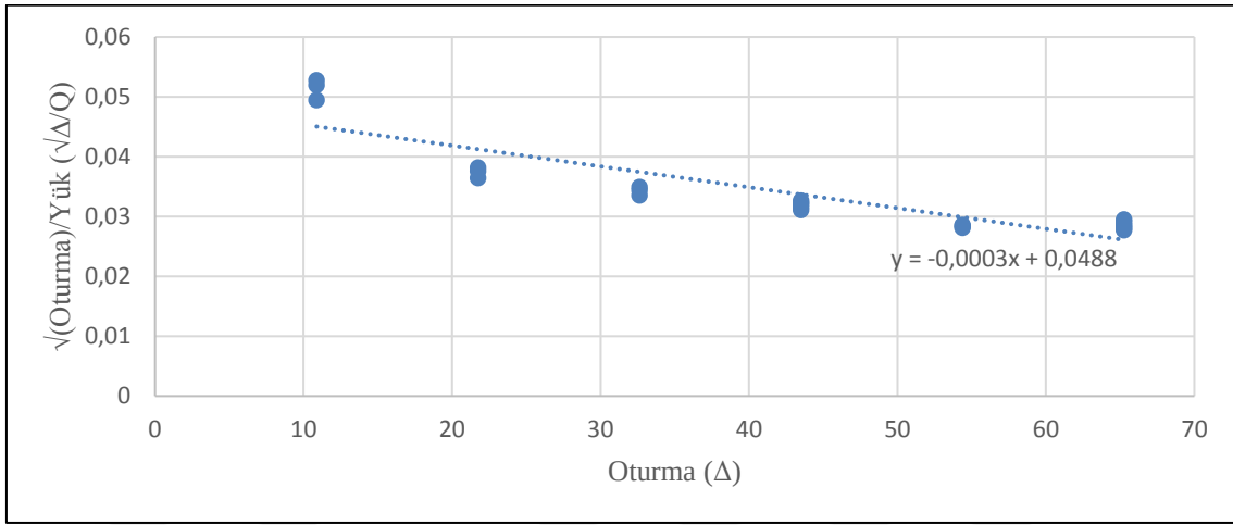
Şekil 10. E kolonu Brinch Hansen grafiği
