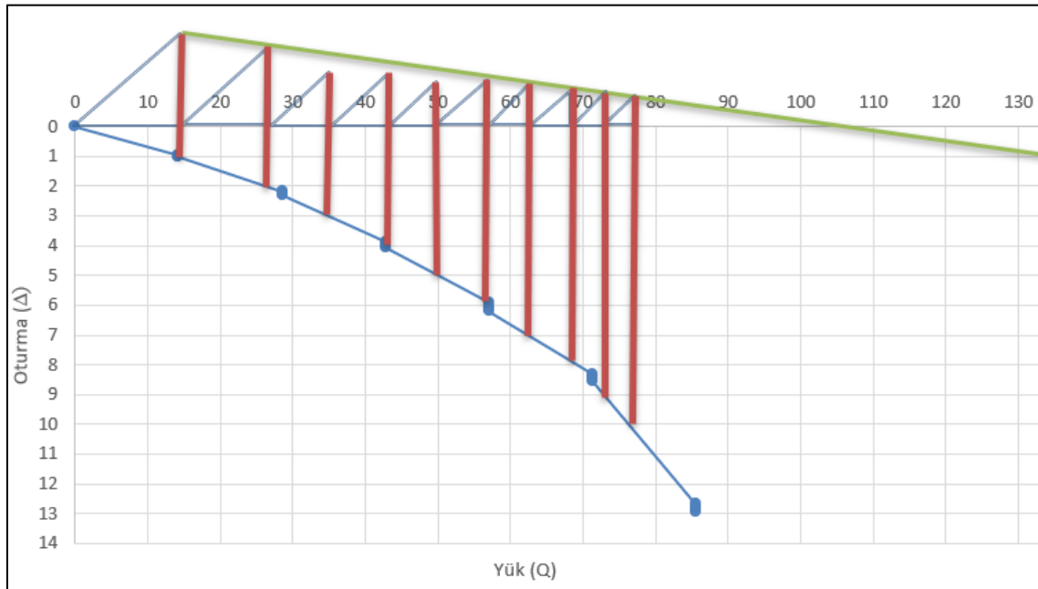
Şekil 35. C kolonu Mazurkiewicz grafiği
