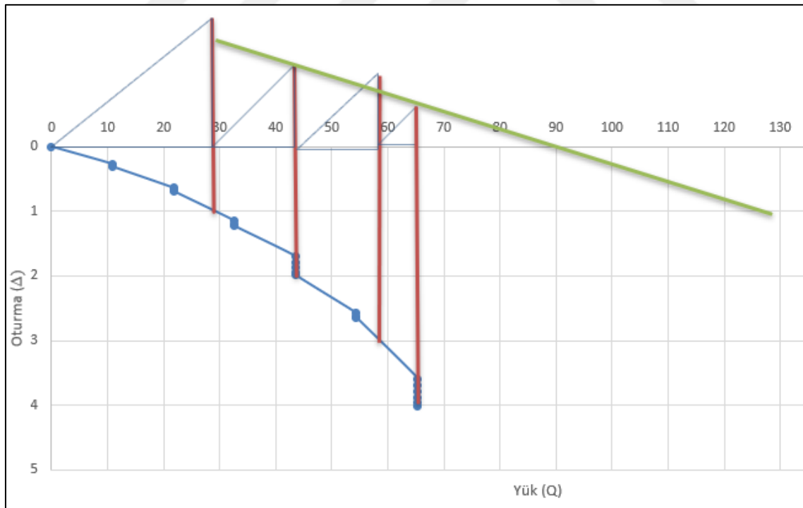
Şekil 36. D kolonu Mazurkiewicz grafiği
