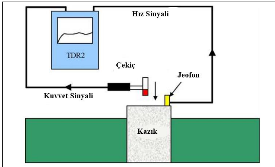
Şekil 2.10. Süreklilik deneyi düzeneği
