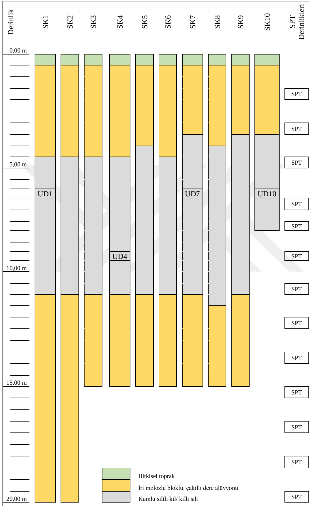
Şekil 5.2. Sondaj logları
