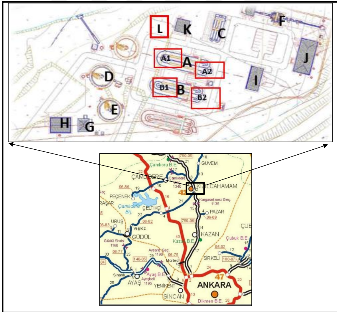
Harita 5.1. Kızılcahamam bölgesi haritası ve tesis yerleşim planı
