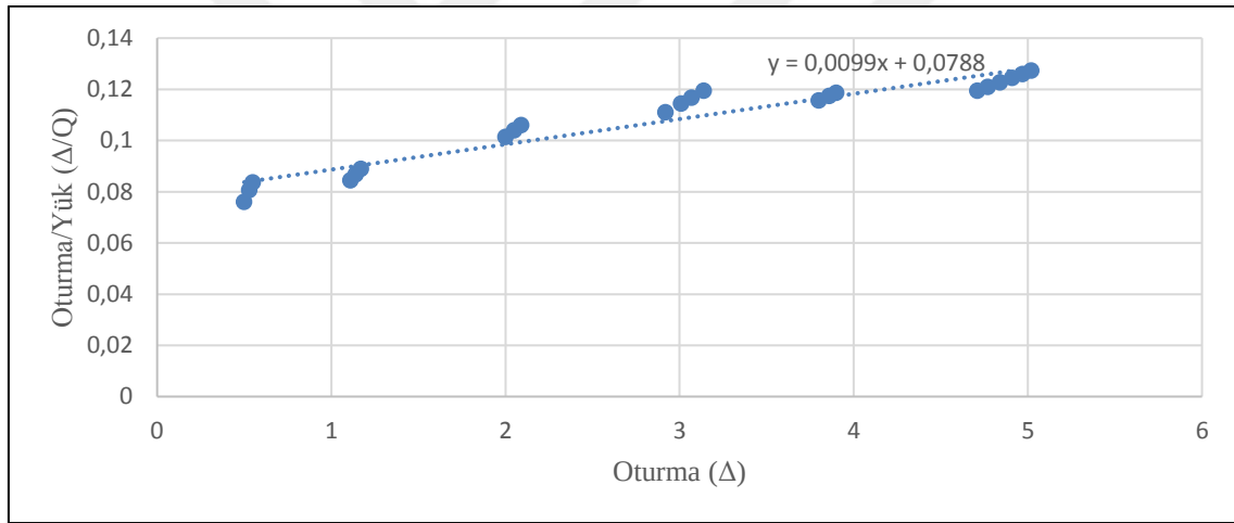
Şekil 20. F kolonu Chin Kondner grafiği
