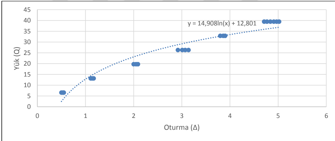
Şekil 47. F kolonu Hirany-Kulhawy grafiği
