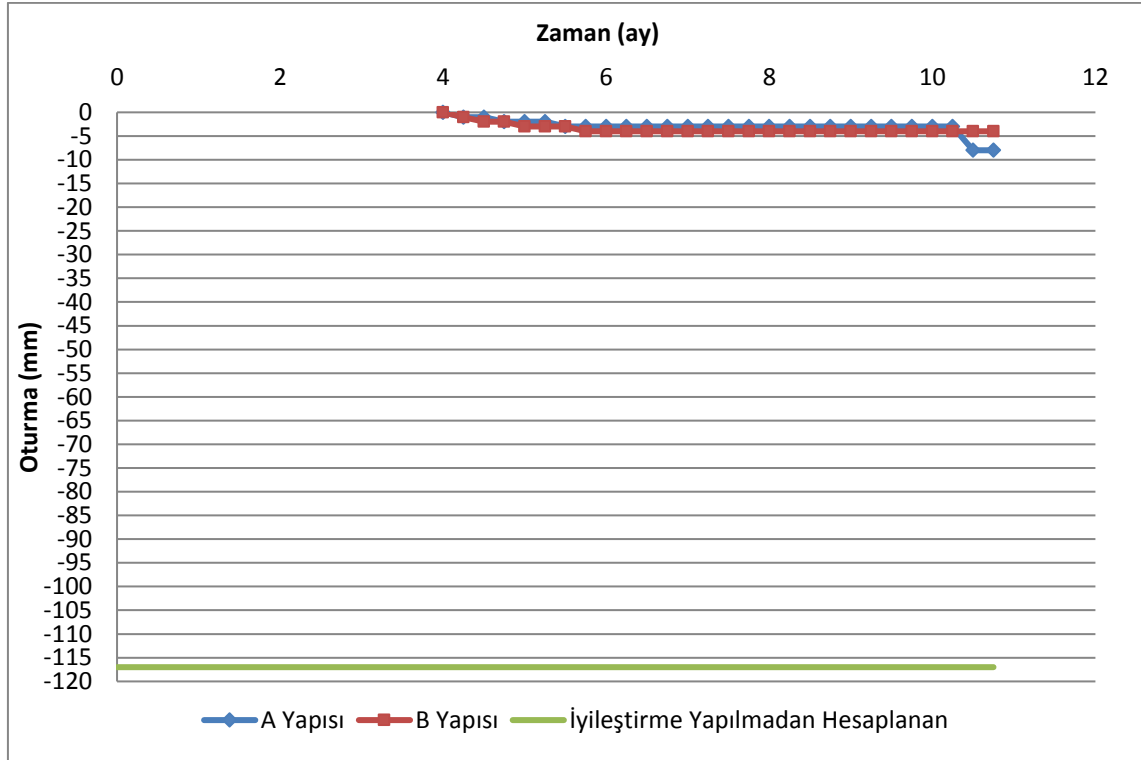
Şekil 6.17. Yapı oturması – zaman ilişkisi
