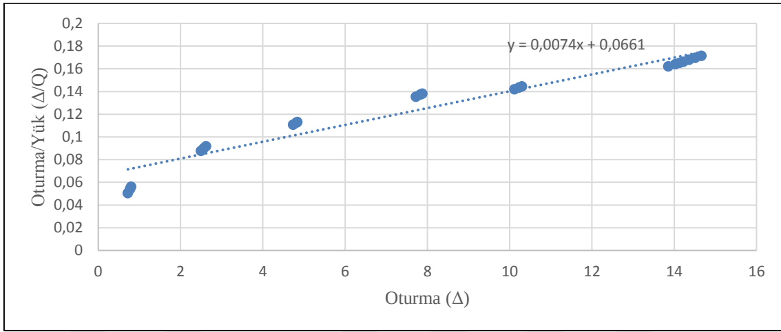
Şekil 13. A1 kolonu Chin Kondner grafiği
