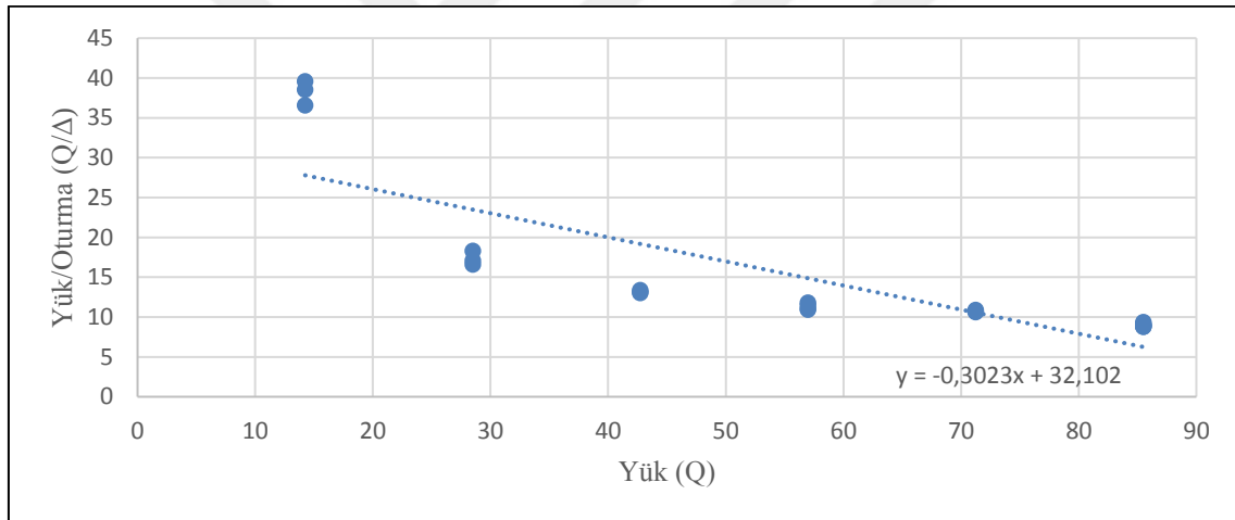
Şekil 23. A2 kolonu Decourt grafiği
