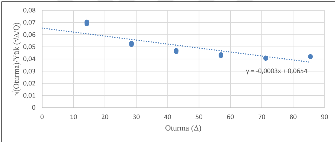
Şekil 8. C kolonu Brinch Hansen grafiği
