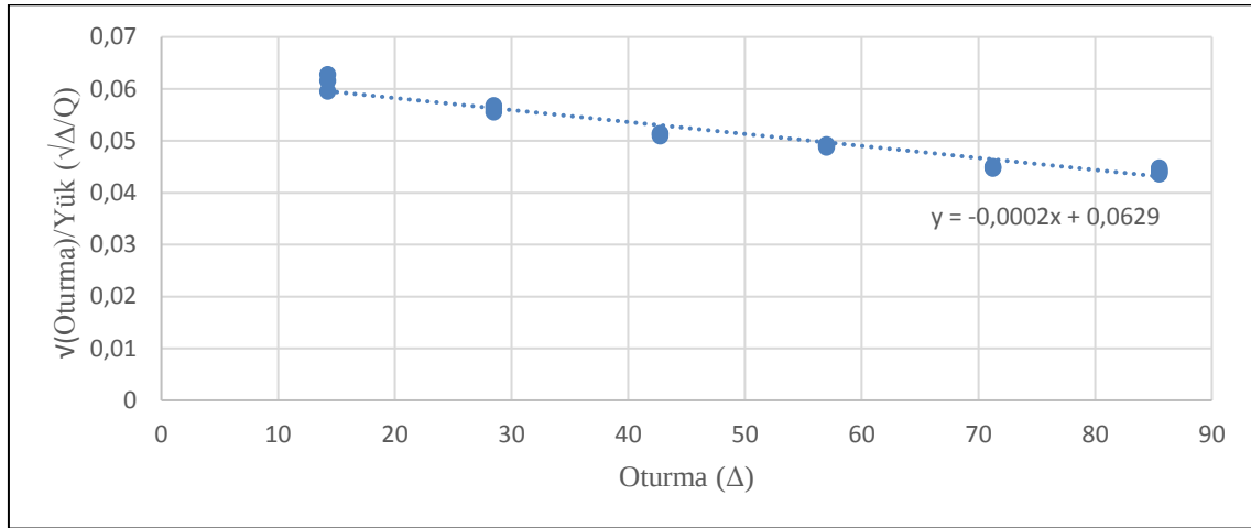
Şekil 4. A1 kolonu Brinch Hansen grafiği
