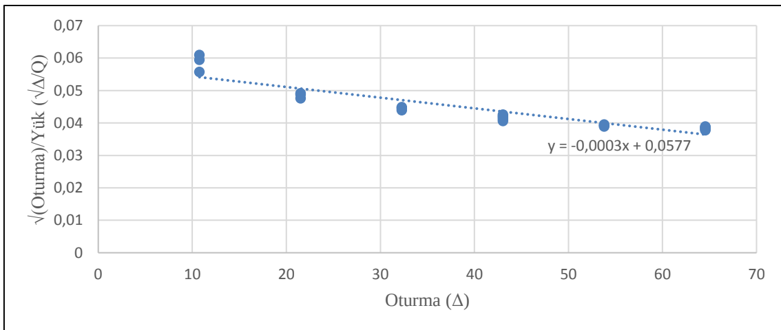
Şekil 12. G kolonu Brinch Hansen grafiği
