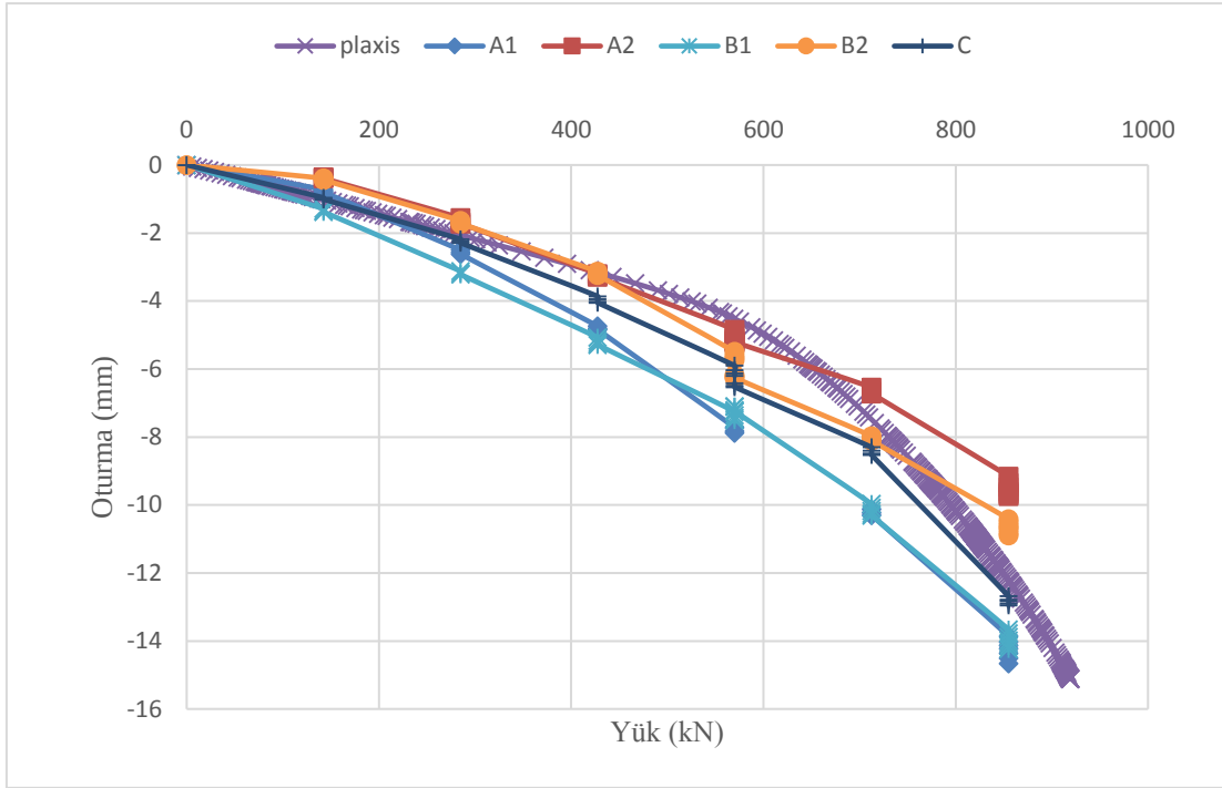
Şekil 49. A1, A2, B1, B2, C kazık yükleme deneyleri ve Plaxis 3D Foundation yük-oturma grafiklerinin karşılaştırılması
