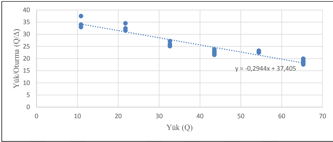
Şekil 28. E kolonu Decourt grafiği
