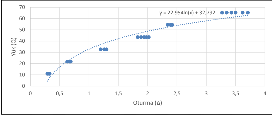
Şekil 46. E kolonu Hirany-Kulhawy grafiği
