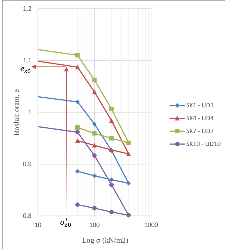
Şekil 5.4. Konsolidasyon deneyleri sonuçları
