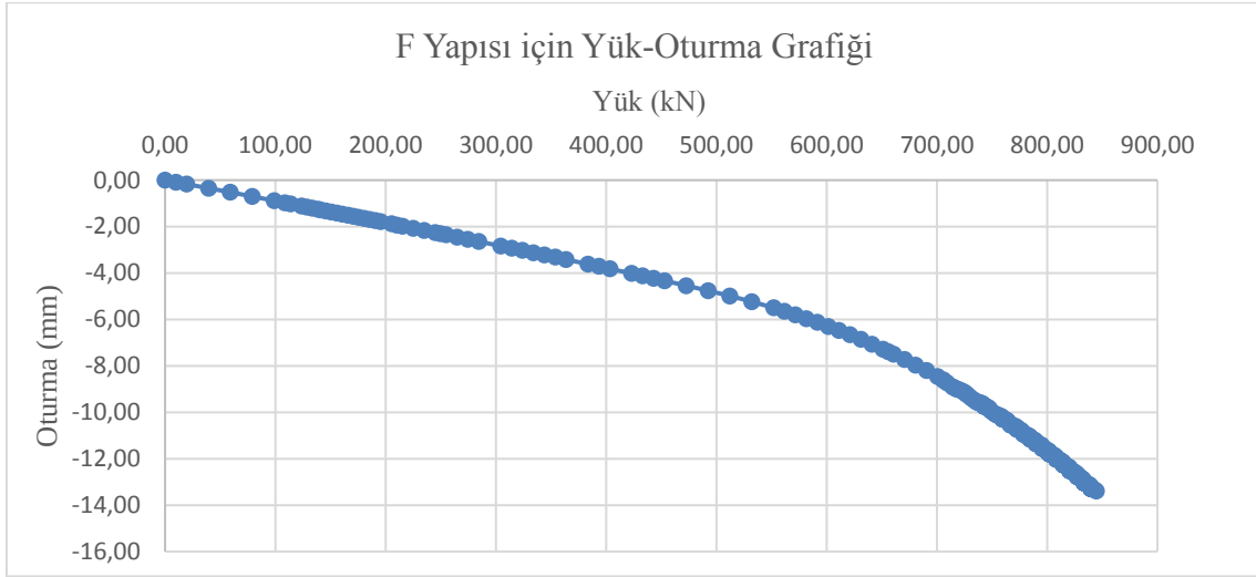
Şekil 6.6. F yapısı altındaki jet grout modeli için yük-oturma ilişkisi
