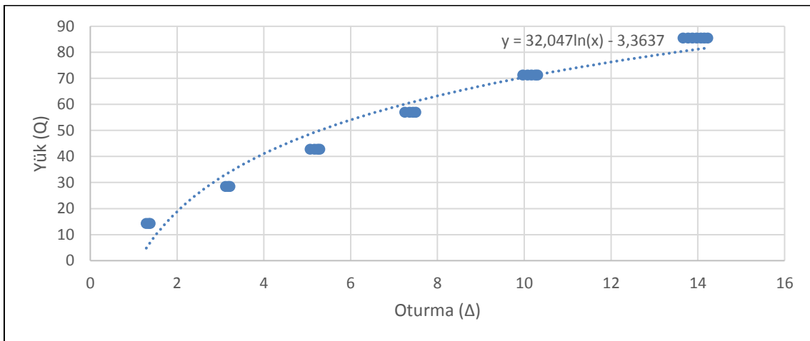
Şekil 42. B1 kolonu Hirany-Kulhawy grafiği
