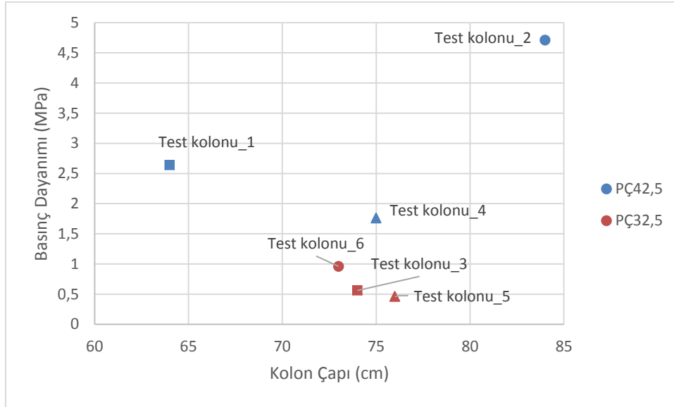
Şekil 6.7. Çimento tipinin jet grout kolon çapı ve dayanımına etkisi
