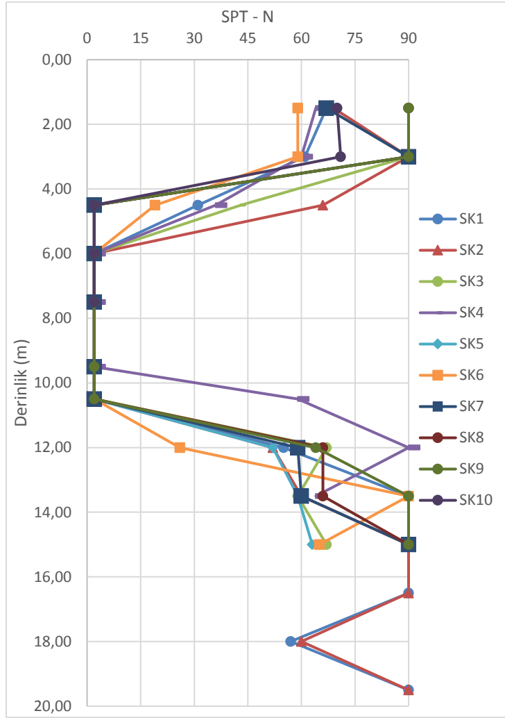
Şekil 5.3. Arazide elde edilmiş SPT N değerleri
