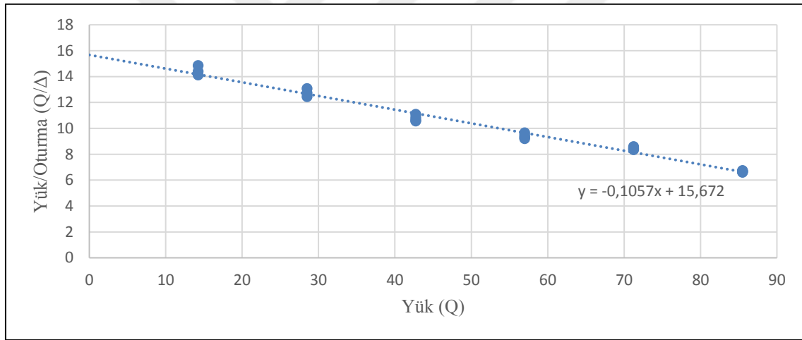
Şekil 26. C kolonu Decourt grafiği
