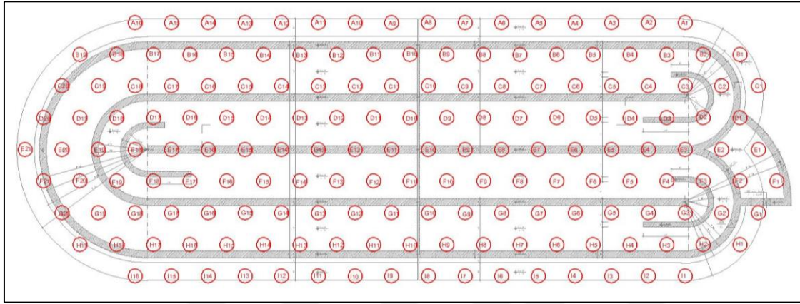
Şekil 6.1. A ve B yapıları altındaki jet grout yerleşim planı
