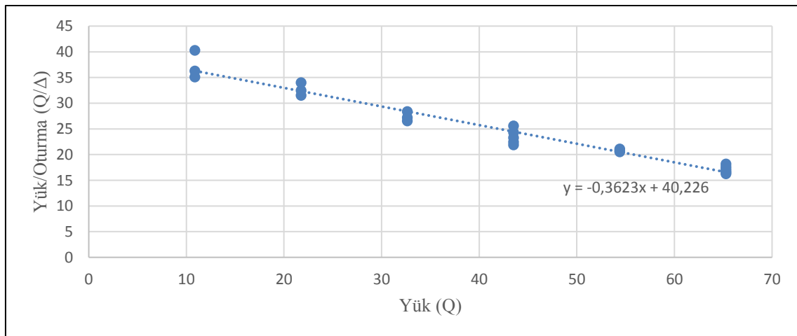
Şekil 27. D kolonu Decourt grafiği
