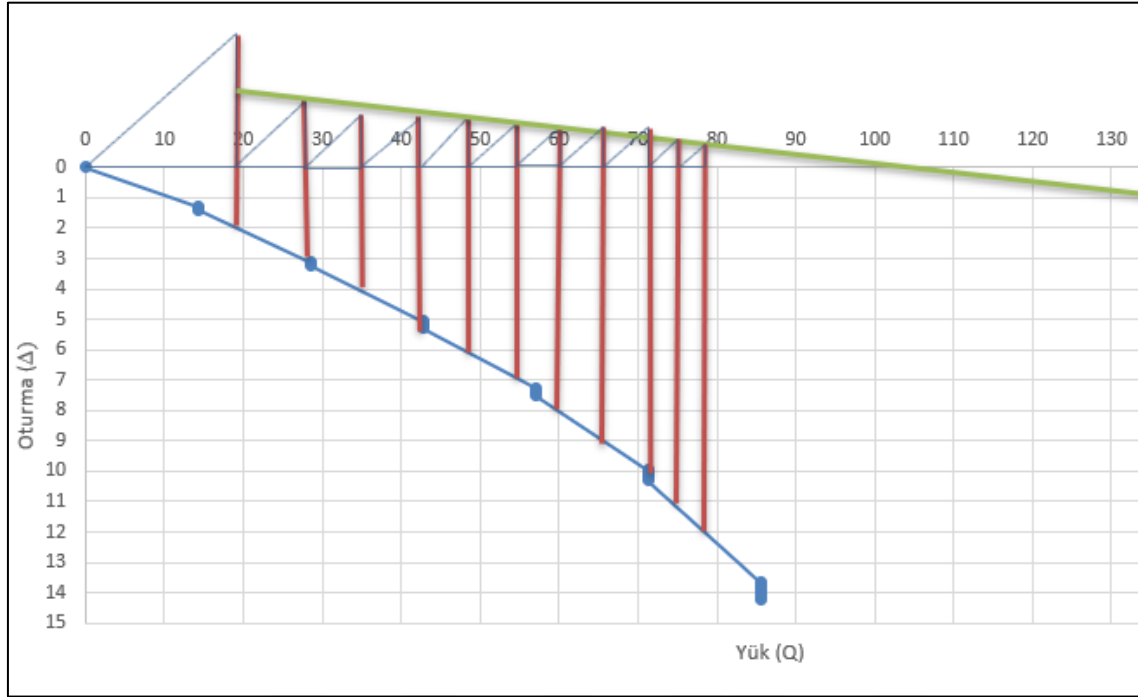
Şekil 33. B1 kolonu Mazurkiewicz grafiği
