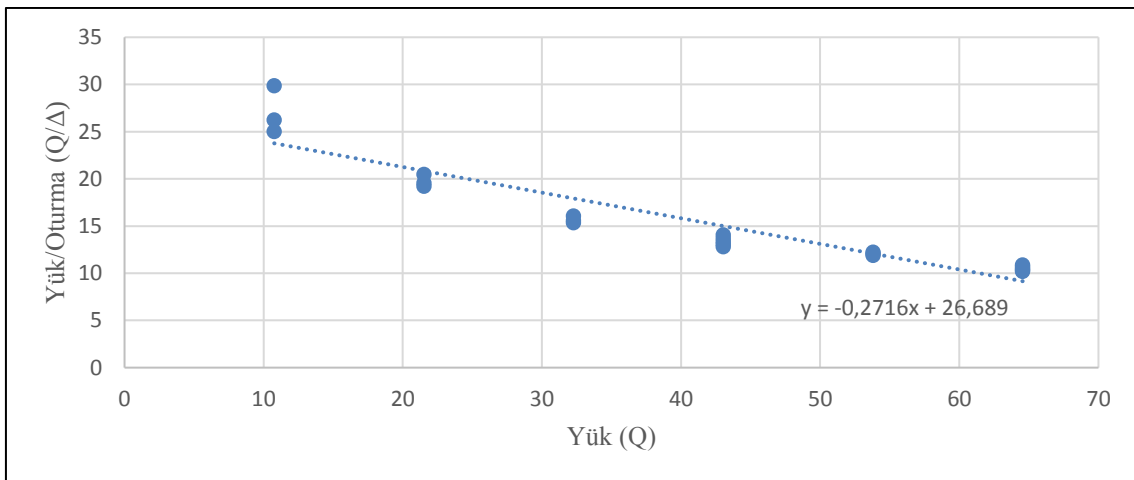
Şekil 30. G kolonu Decourt grafiği
