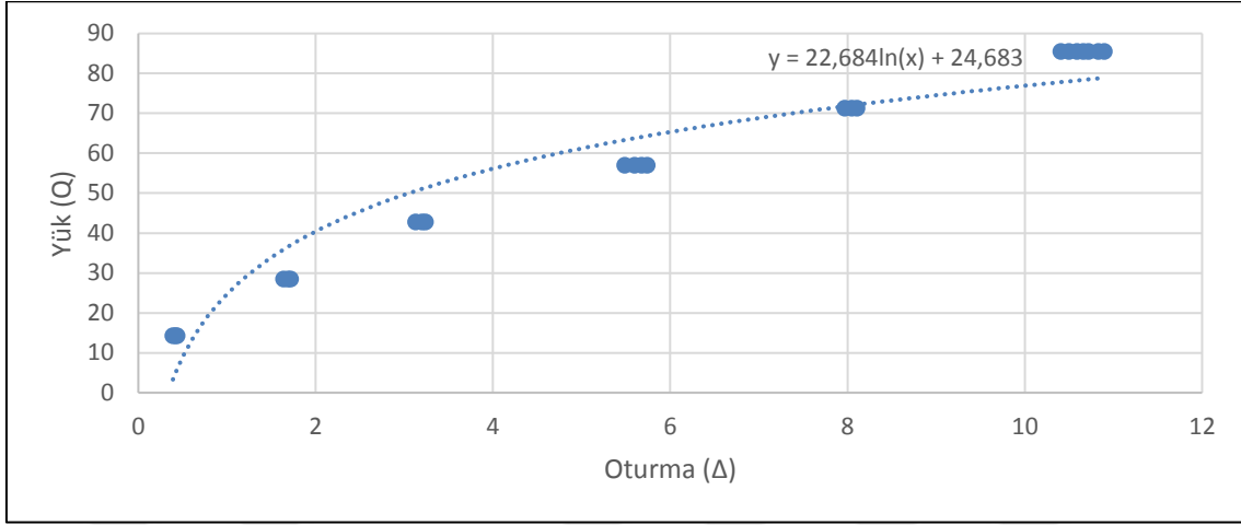
Şekil 43. B2 kolonu Hirany-Kulhawy grafiği
