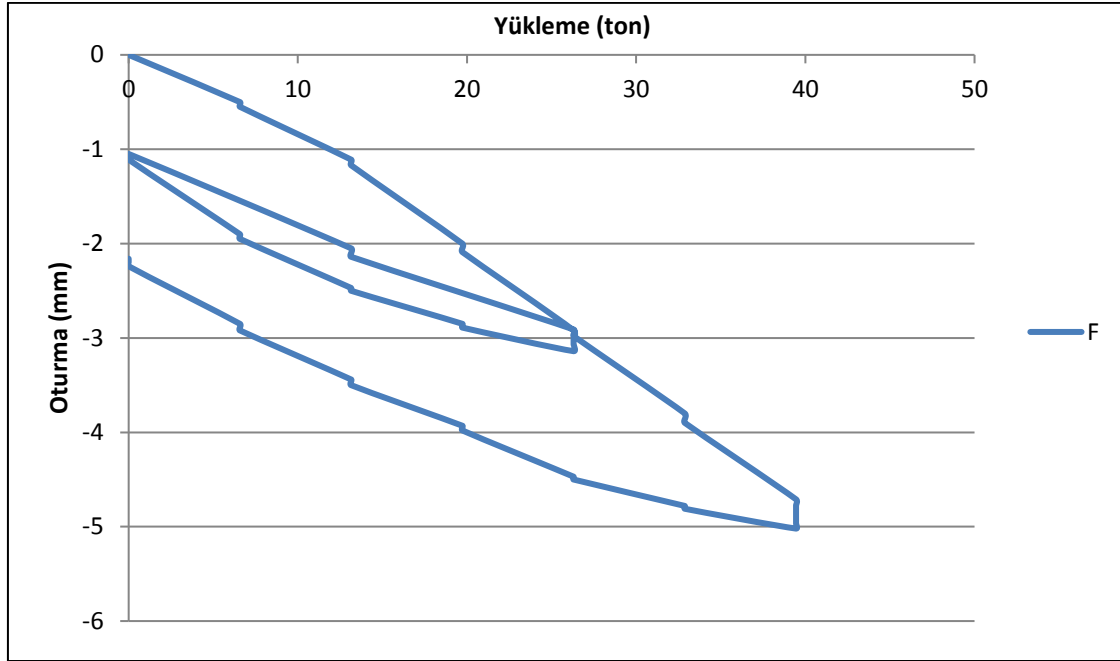
Şekil 6.11. F yapısında gerçekleştirilen kolon yükleme deneyi sonucu [41]
