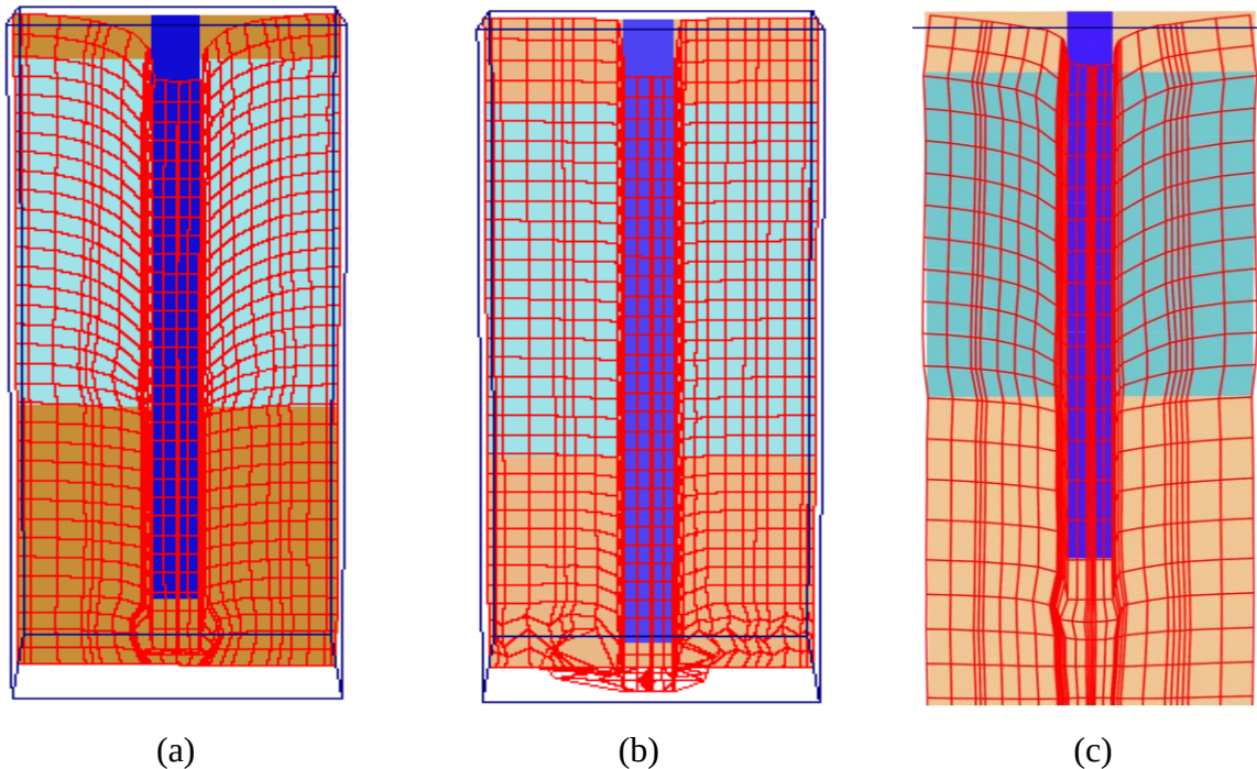
Şekil 6.3. Uygulanan yükler altında deforme olmuş mesh görüntüleri a) Model 1, b) Model 2, c) Model 3
