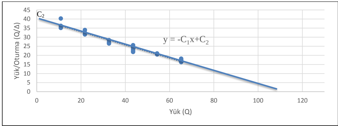
Şekil 3.4. Decourt (1999) yöntemi örneğı
