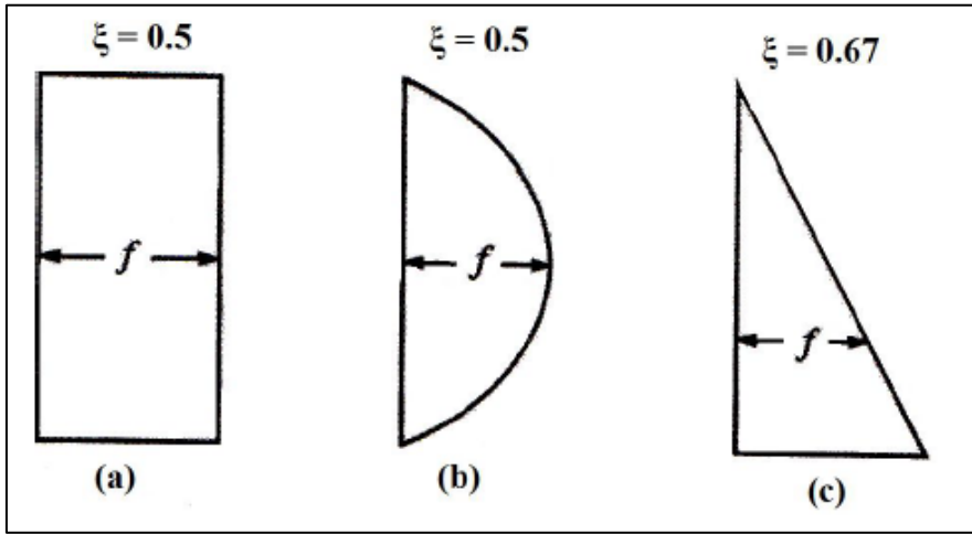
Şekil 4.1. Kazık boyunca birim sürtünme direnci uniform (a), parabolik (b), üçgen (c) dağılımı [36]
