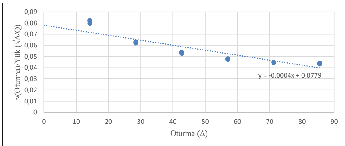
Şekil 6. B1 kolonu Brinch Hansen grafiği
