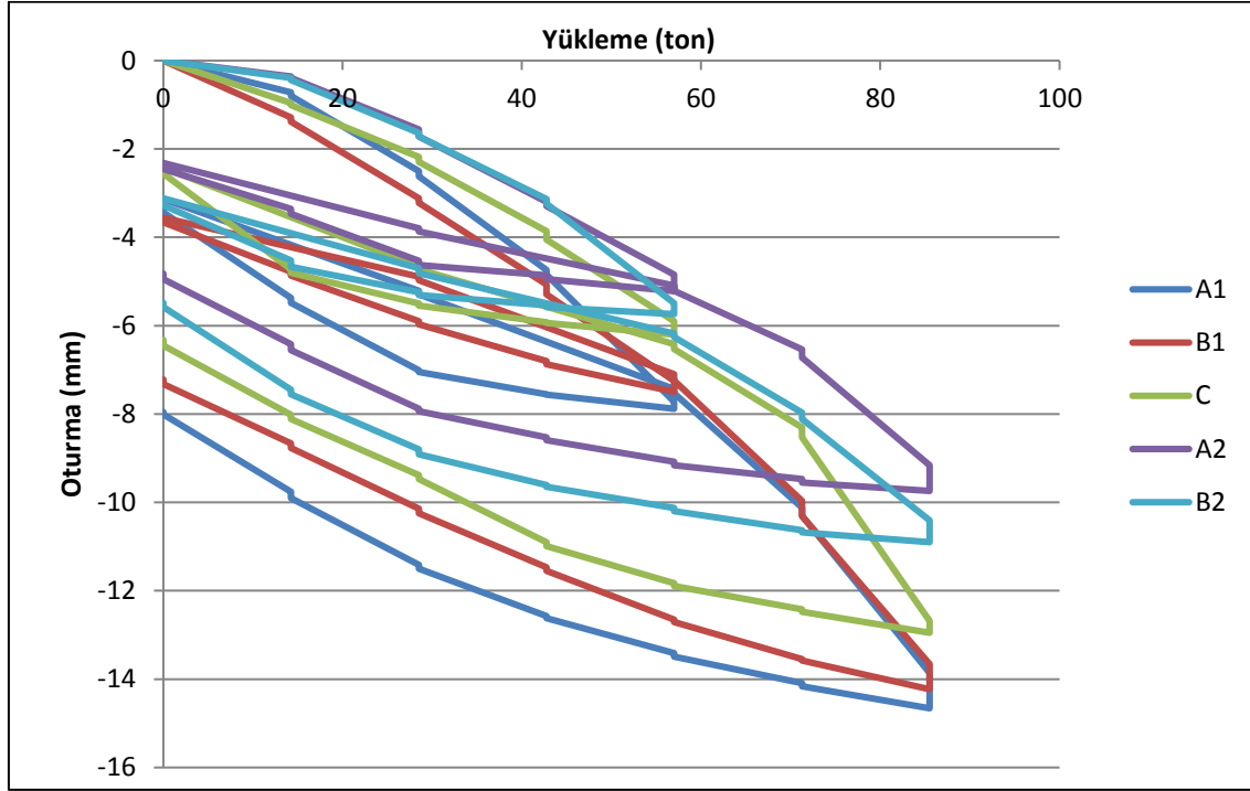
Şekil 6.9. A-B-C yapılarında gerçekleştirilen kolon yükleme deneyi sonuçları [41]
