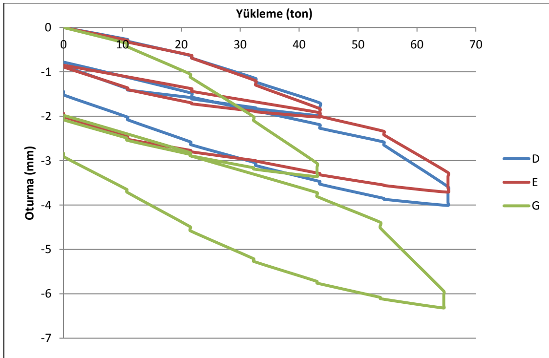
Şekil 6.10. D-E-G yapılarında gerçekleştirilen kolon yükleme deneyi sonuçları [41]
