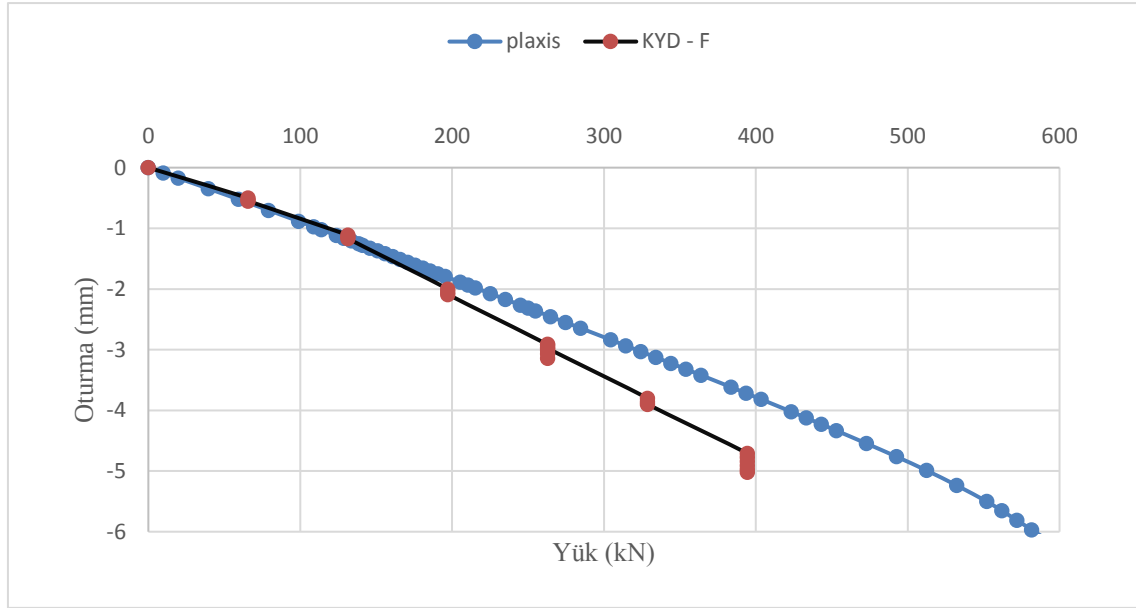
Şekil 51. F kazık yükleme deneyleri ve Plaxis 3D Foundation yük-oturma grafiklerinin karşılaştırılması
