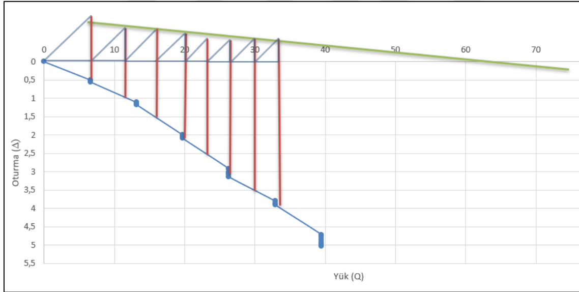
Şekil 38. F kolonu Mazurkiewicz grafiği
