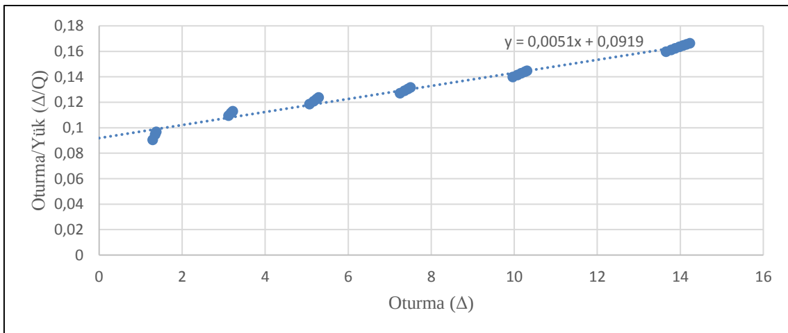
Şekil 15. B1 kolonu Chin Kondner grafiği
