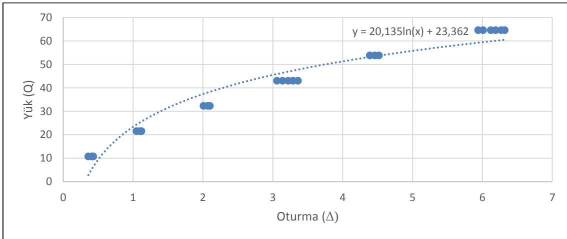
Şekil 48. G kolonu Hirany-Kulhawy grafiği
