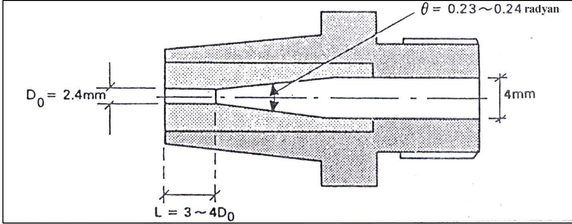
Şekil 2.8. Shizabaki ve Ohta'nın önerdiği ideal püskürtme ağızlığı [15]
