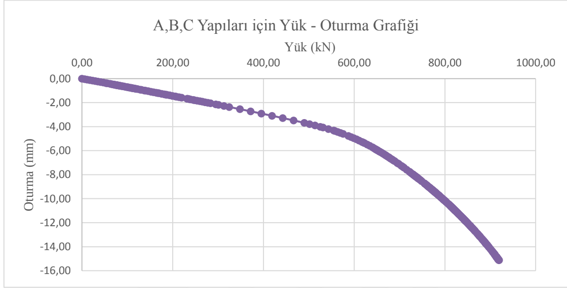
Şekil 6.4. A,B,C yapıları altındaki jet grout modeli için yük-oturma ilişkisi
