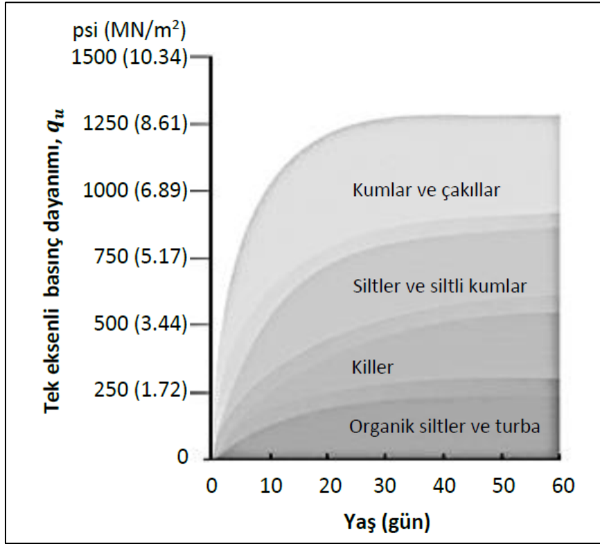
Şekil 2.13. Değişik zeminlerdeki jet grout kolonlarında elde edilebilecek tek eksenli karot basınç dayanımları [21]
