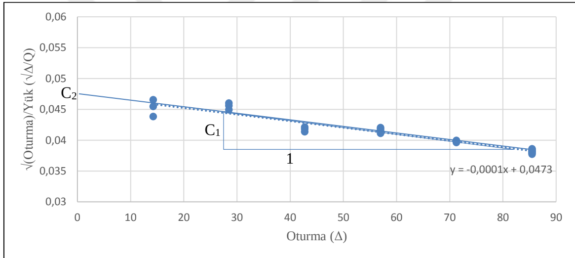
Şekil 3.1. Brinch Hansen %80 yöntemi örneği
