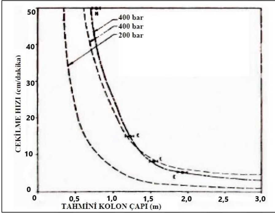
Şekil 2.7. Tahmini kolon çapı - tij çekme hızı arasındaki ilişki [13]
