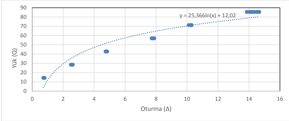
Şekil 40. A1 kolonu Hirany-Kulhawy grafiği
