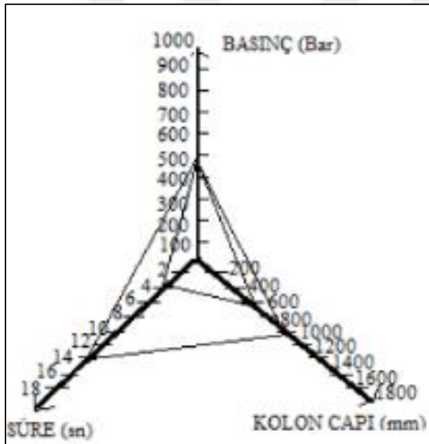
Şekil 2.4. Enjeksiyon basıncı – bekleme süresi ve kolon çapı arasındaki ilişki [11]
