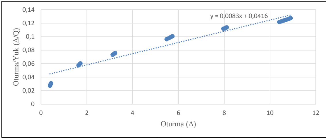
Şekil 16. B2 kolonu Chin Kondner grafiği
