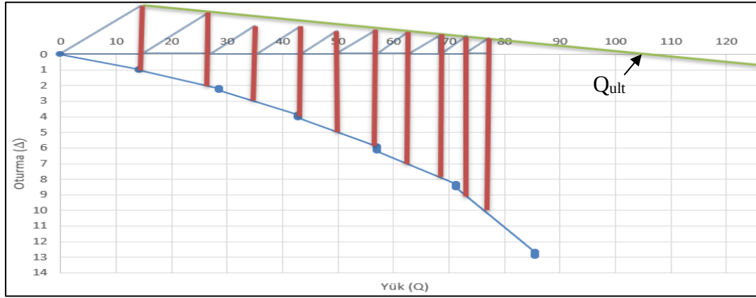
Şekil 3.2. Mazurkiewicz (1972) yöntemi örneği
