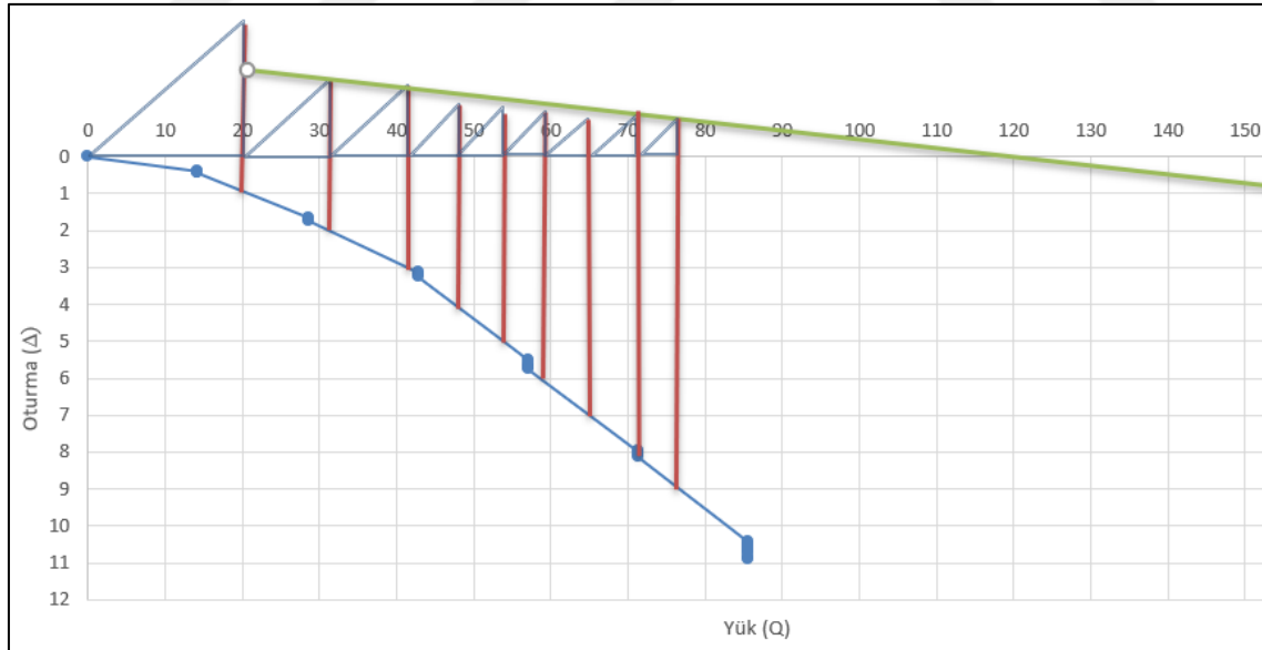
Şekil 34. B2 kolonu Mazurkiewicz grafiği
