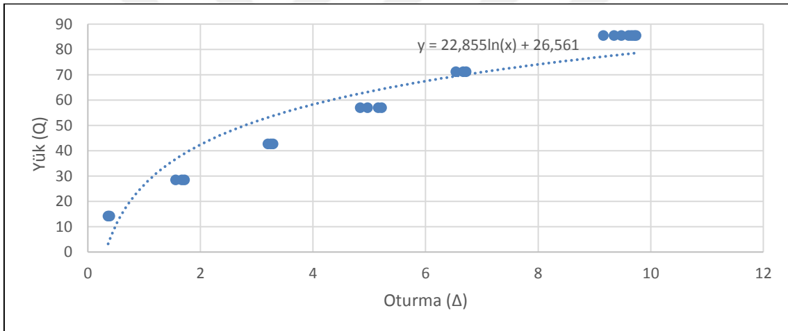
Şekil 41. A2 kolonu Hirany-Kulhawy grafiği
