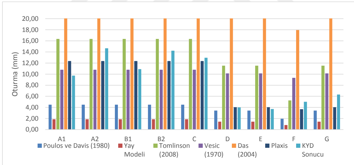
Şekil 6.13. Teorik ve KYD oturma karşılaştırılması
