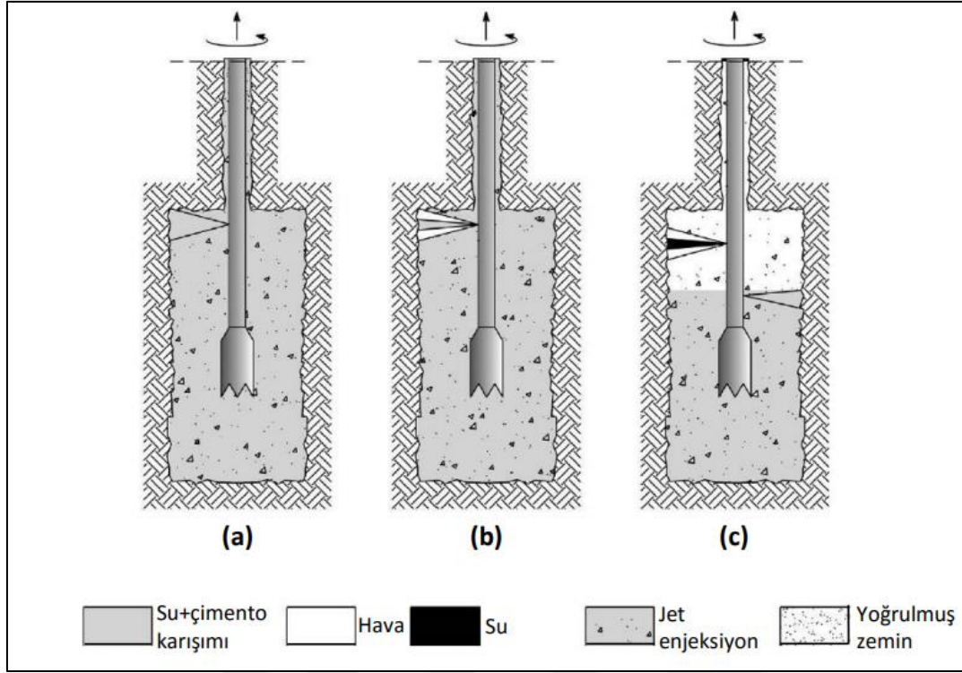
Şekil 2.2. (a) JET1 yöntemi – (b) JET2 yöntemi – (c) JET3 yöntemi [9]
