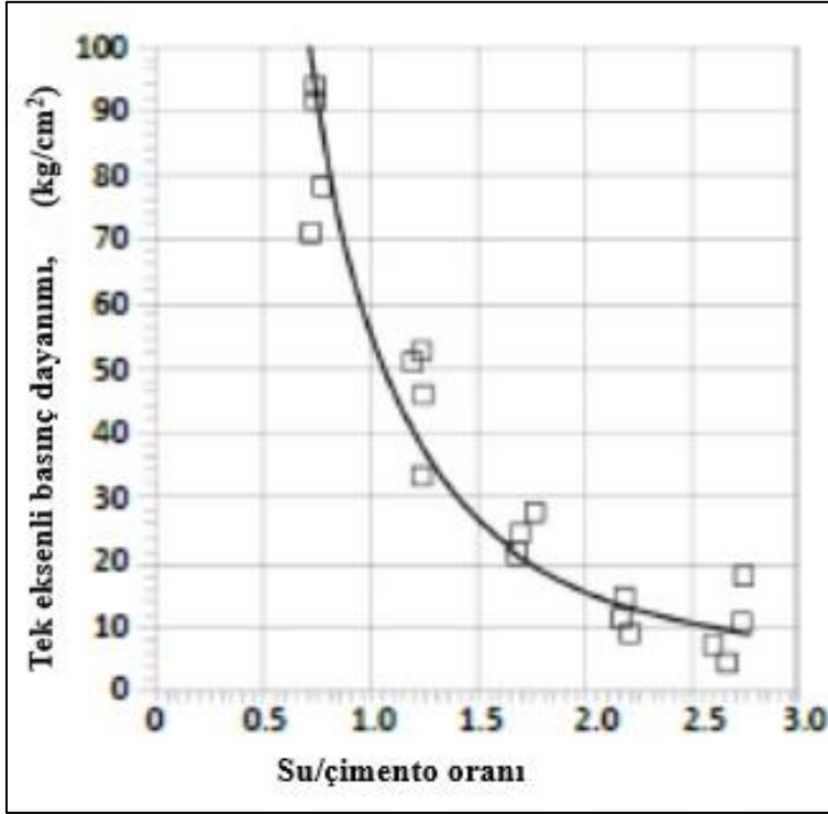
Şekil 2.11. Boston Mavi Killeri'nde su/çimento oranı ile karot basıncı ilişkisi [20]
