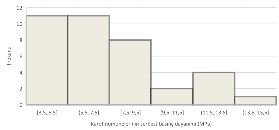
Şekil 6.15. Karot numunelerinin serbest basınç dayanım histogramı [41]
