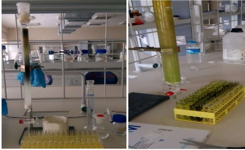
Şekil 3.5. Silika jel kolon kromatografisi
