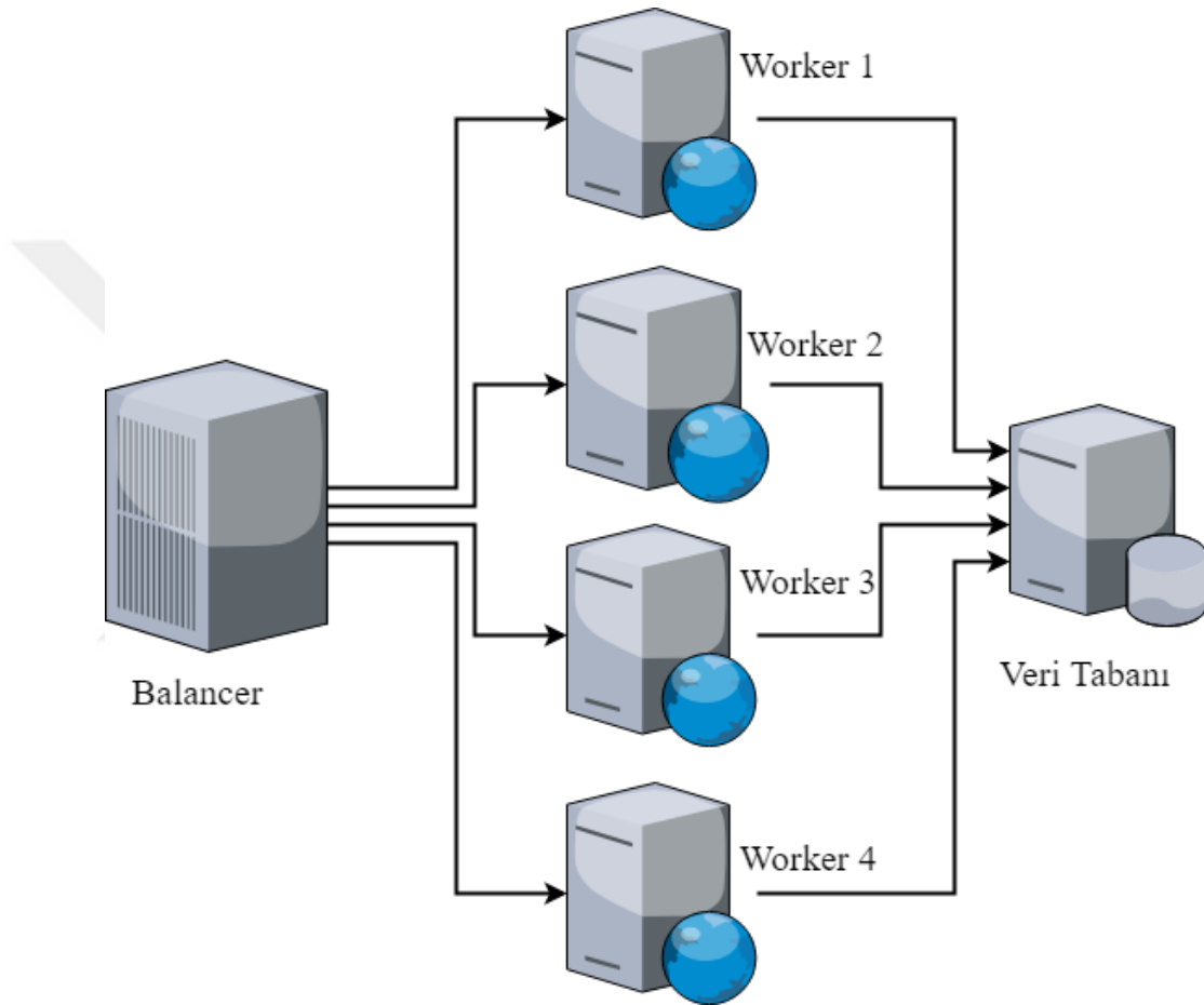
Şekil 4.3. Load balance sunucu yapısı.
