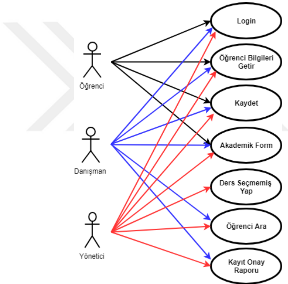
Şekil 4.6. Use Case diyagramı.
