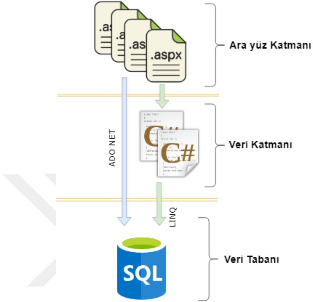
Şekil 2.2. Mevcut sistemin mimarisi.
