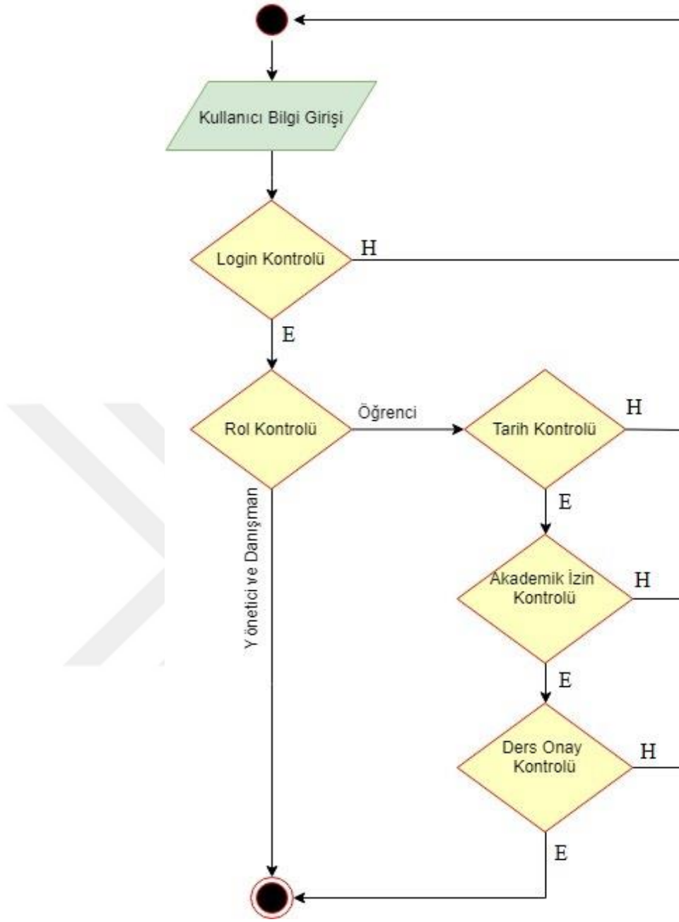
Şekil 4.7. Login aktivite diyagramı.
