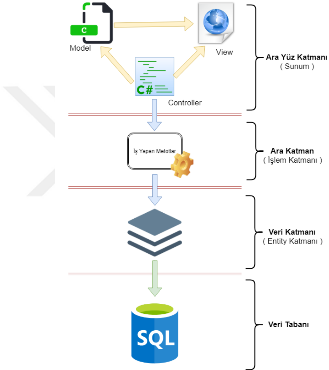
Şekil 4.2. Yeni uygulamanın yazılım mimarisi.
