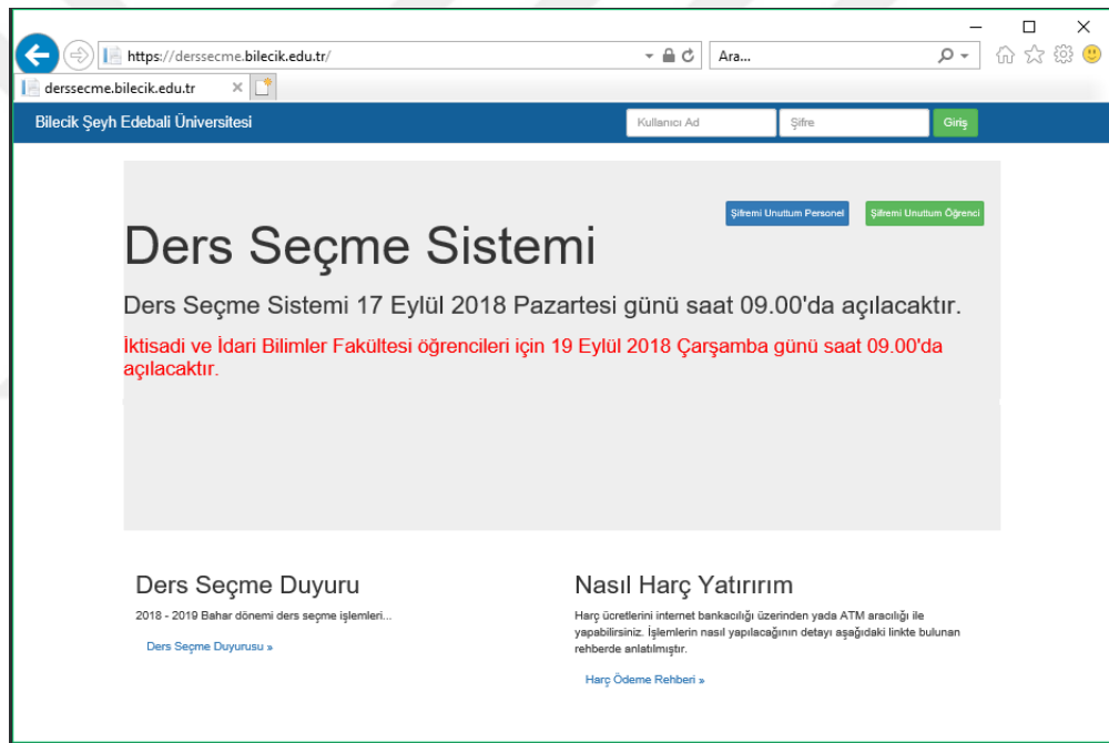
Şekil 4.20. Login ekranı.
