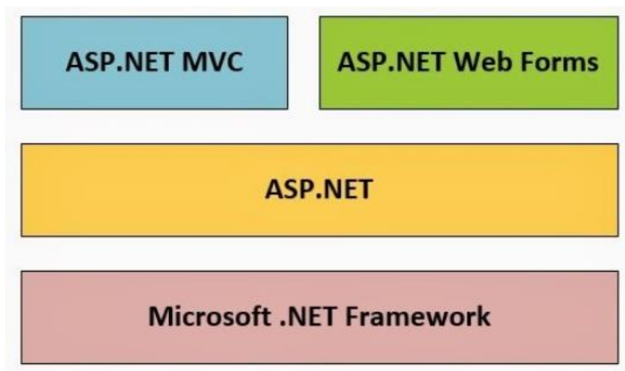
Şekil 3.2. ASP.NET bileşenleri.
