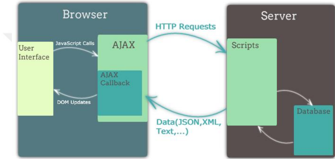
Şekil 3.8. AJAX çalışma yapısı ( http://javascript-coder.com/tutorials/re-introduction-to-ajax.phtml ).
