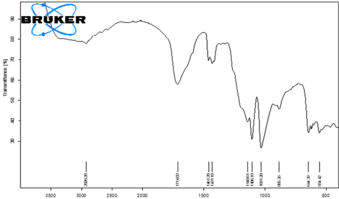
Şekil 4.8. (4)' nolu bileşiğin FTIR (ATR) spektrumu
