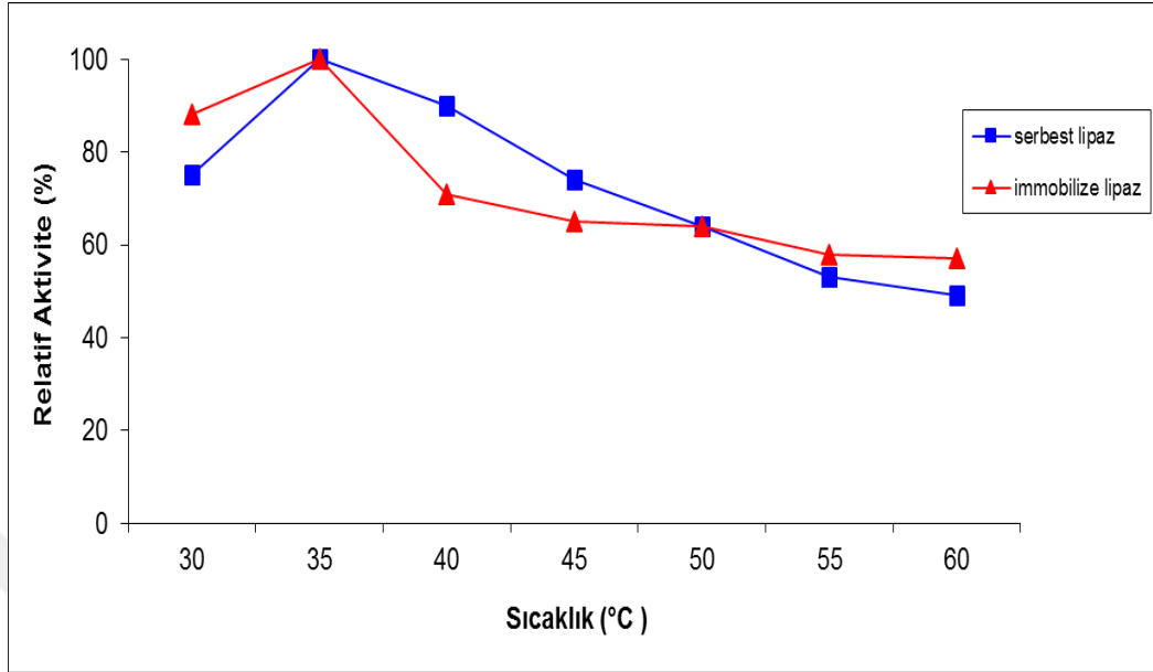
Şekil 4.14. Serbest ve \text{Fe}_3\text{O}_4@\text{Cal8S-E} nanopartiküllerin lipaz aktivitesi üzerine sıcaklık etkisi
