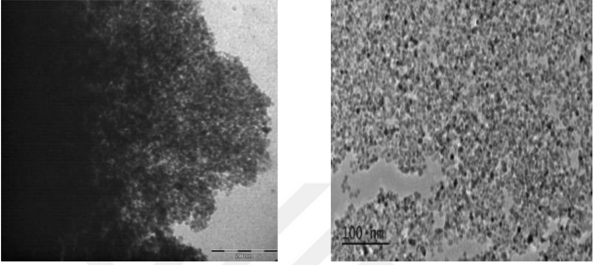
Şekil 4.10. Sırasıyla Saf \text{Fe}_3\text{O}_4 -nanopartiküllerinin ve \text{F}_3\text{O}_4@\text{Cal8S} nanopartüküllerin TEM görüntüleri
