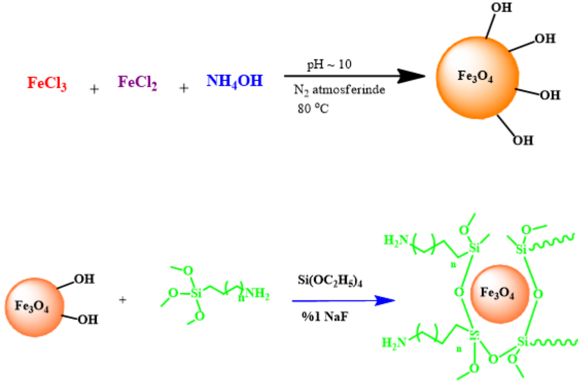
Şekil 2.1. \text{Fe}_3\text{O}_4 manyetik nanopartiküllerin hazırlanması
