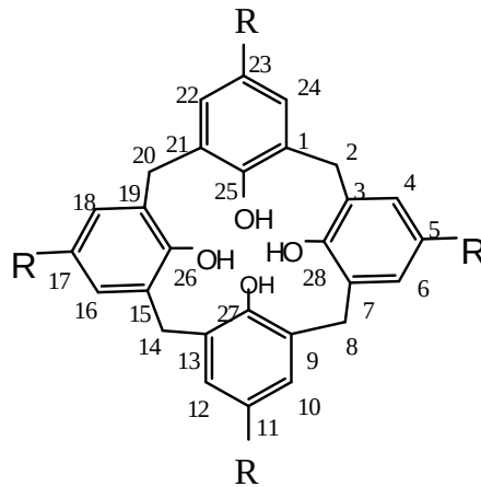
5,11,17,23-tetraalkil-25,26,27,28-tetrahidroksi-kaliks[4]aren
