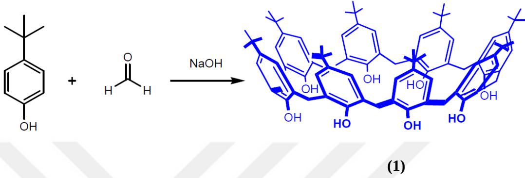
Şekil 4.1. p-ter -bütilkaliks[8]aren sentezi
