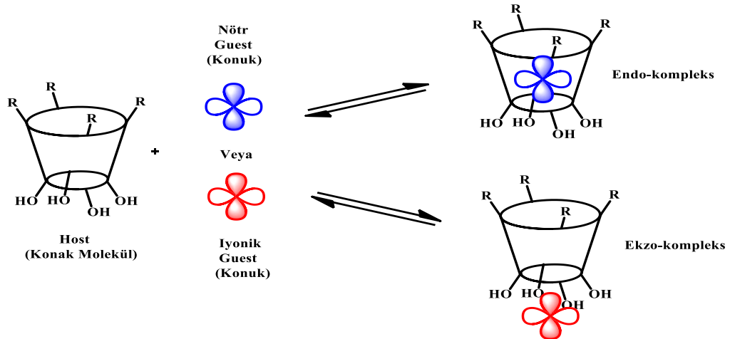
Şekil 1.14. Endo ve ekzo komplekslerin görünümü
