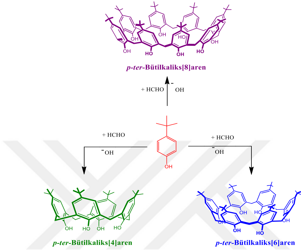
Şekil 1.4. p-ter -Bütil kaliks[4]aren, p-ter -Bütil kaliks[6]aren, p-ter -Bütil kaliks[8]arenlerin sentezi
