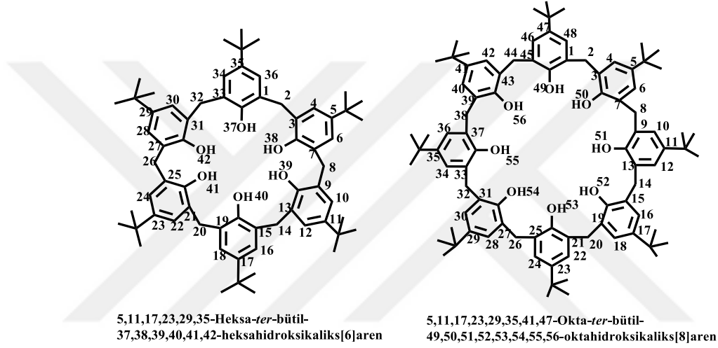
Şekil 1.3.1 Kaliks[6]aren ve Kaliks[8]arenlerin numaralandırması ve adlandırılması.
