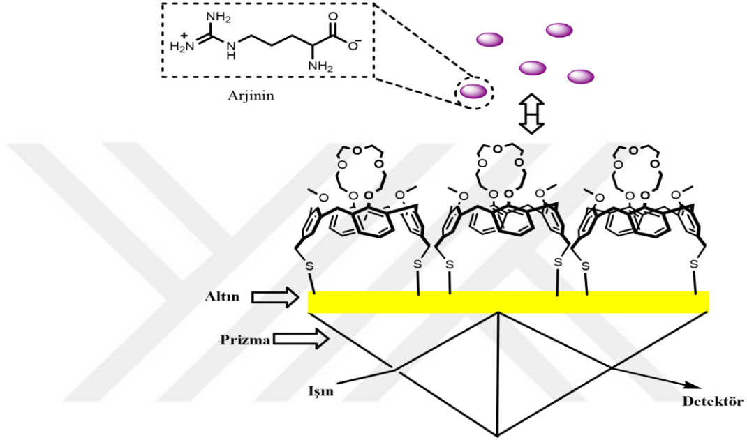
Şekil. 1.23. Arjinin sensörü
