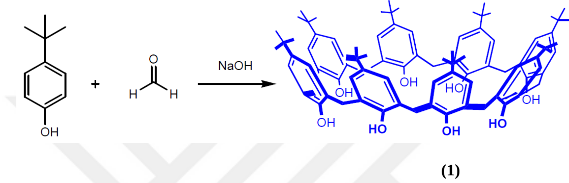
Şekil 3.1 p-ter-bütillikaliks[8]aren sentezi
