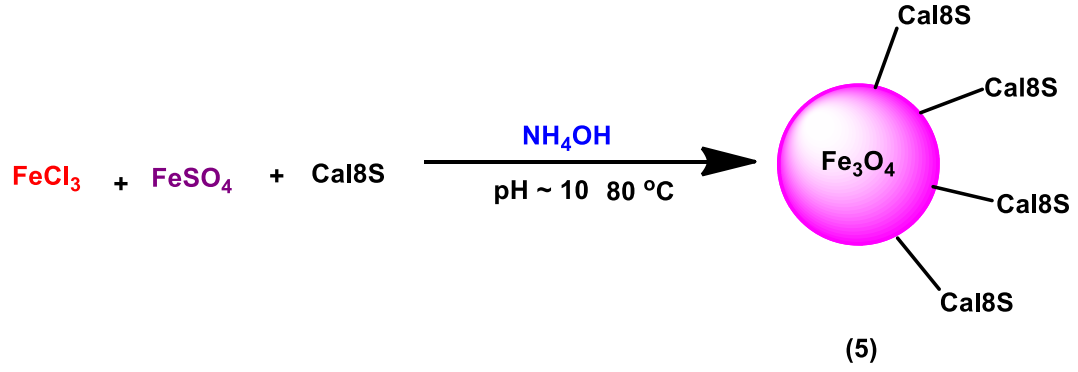
Şekil 3.5. Cal8S varlığında \text{Fe}_3\text{O}_4 nanopartiküllerin sentezi
