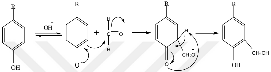
Şekil 1.7. Hidroksimetilfenolün oluşumu
