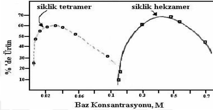
Şekil 1.5. Kaliks[n]aren sentezinde baz konsantrasyonunun reaksiyon verimine etkisi
