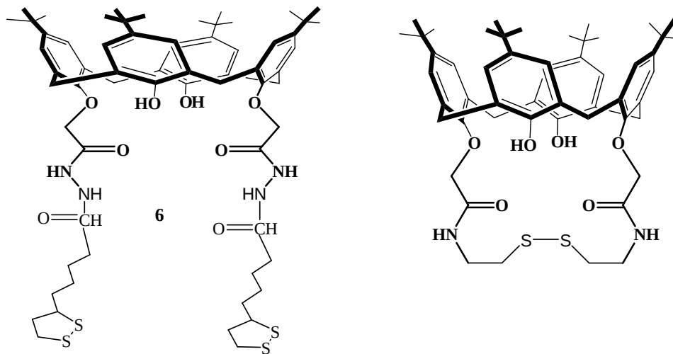
Şekil 2.7. Lipaz immobilizasyonunda kullanılan p-ter-Butilkaliks[4]arenin tiyol türevlerini
