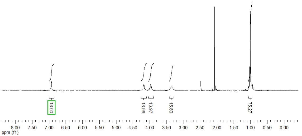
Şekil 4.6. p -ter-bütikaliks[8]aren oktakarboksilikasid türevinin 1 H-NMR spektrumu
