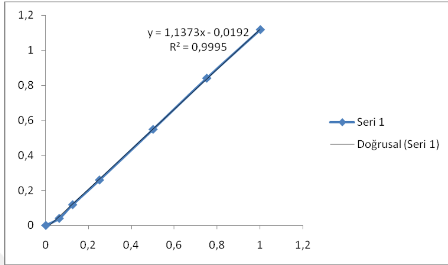
Şekil 3.8. Standart protein miktarı (mg/ml)- absorbans grafiği ( \lambda_{max} =595 nm)
