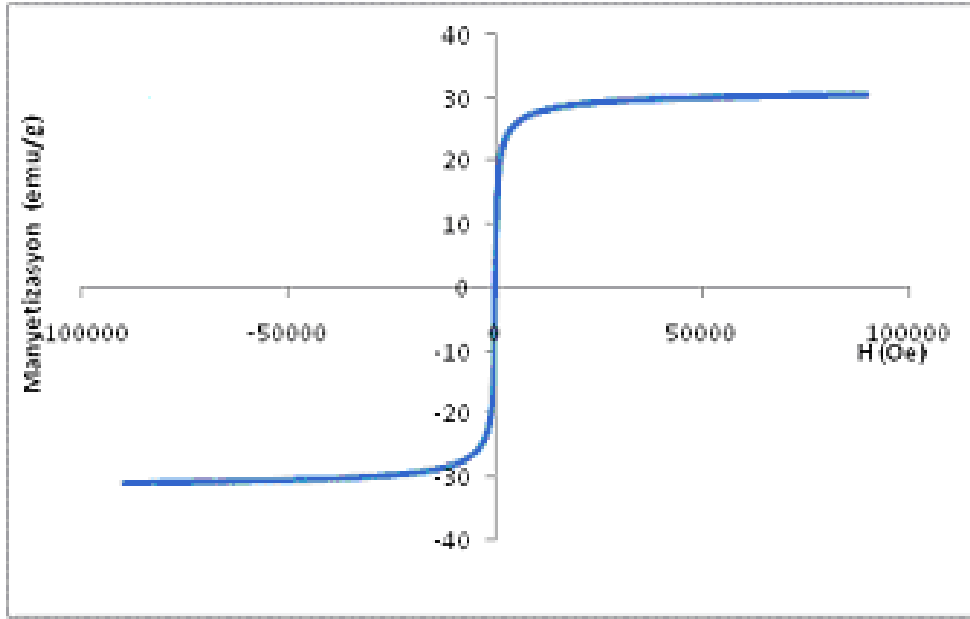
Şekil 4.11. F_3O_4@Cal8S nanopartüküllerin VSM'i
