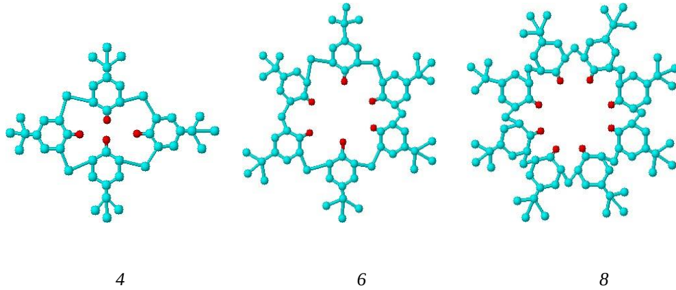
Şekil 1.2.1. p-ter-Bütılkaliks[n]arenlerin model yapıları
