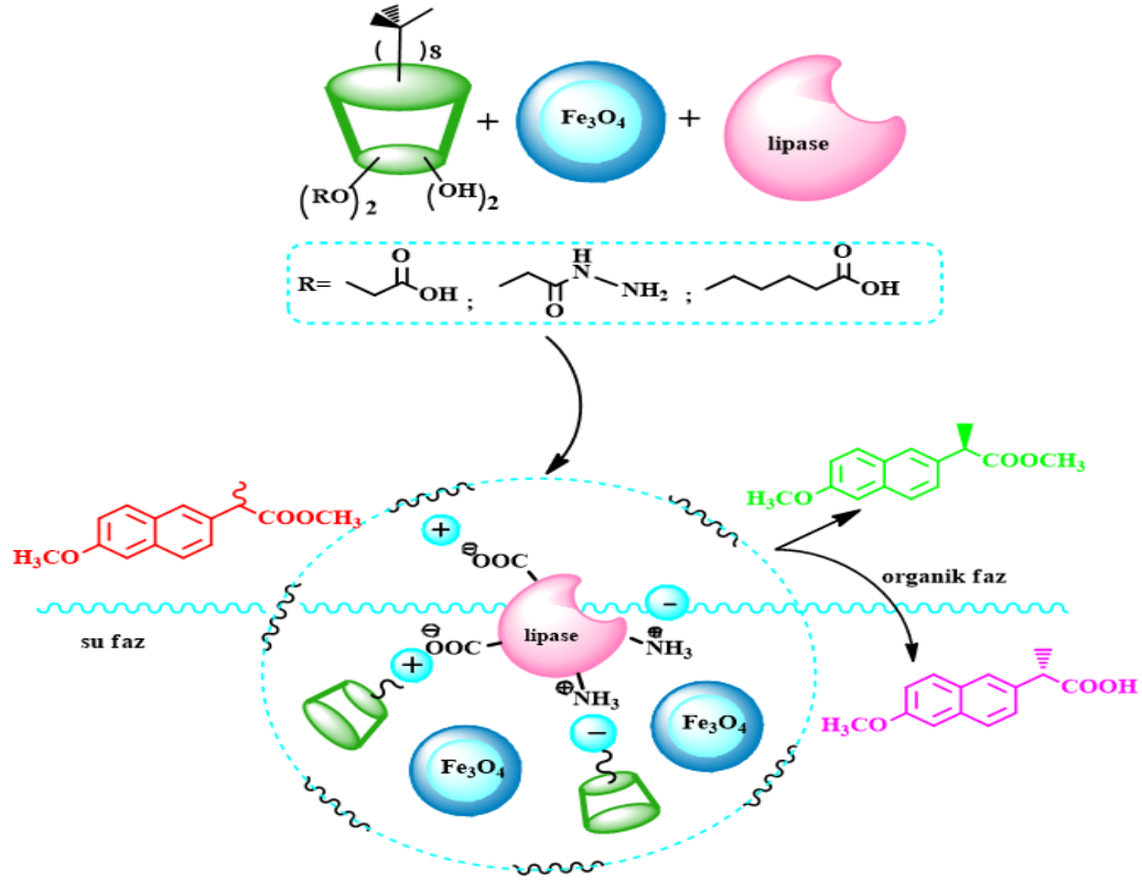
Şekil 2.5. Rasemik naproksen metil esterinin enantiyoseçimli reaksiyon çalışması
