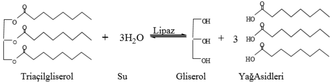
Şekil 1.26. Lipazların katalizlediği hidroliz reaksiyonu
