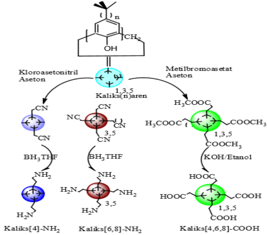
Şekil 2.2. Lipaz immobilizasyonunu ve rasemik naproksenin enantiyoseçimli çalışmalarında kullanılması
