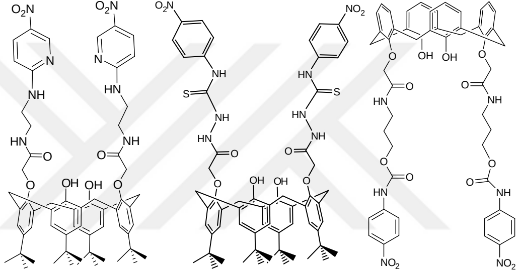
Şekil 2.8. Lipaz immobilizasyonunda kullanılan p-ter -butilkaliks[4]arenin nitro türevlerini
