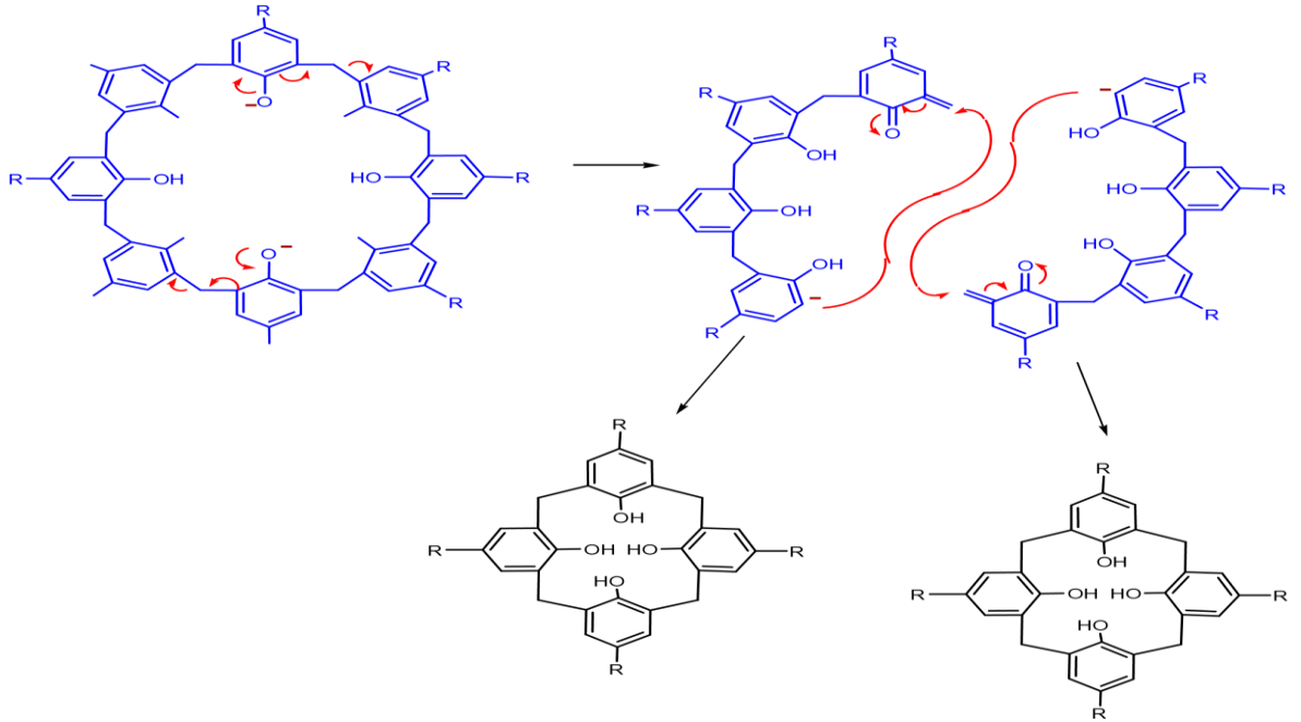
Şekil 1.10. Kaliks[8]aren' in parçalanarak kaliks[4]aren' e dönüşümü
