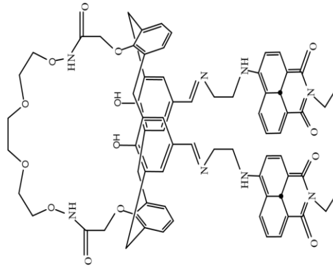
Şekil 1.19. Naftalimit kaliks[4]aren türevi
