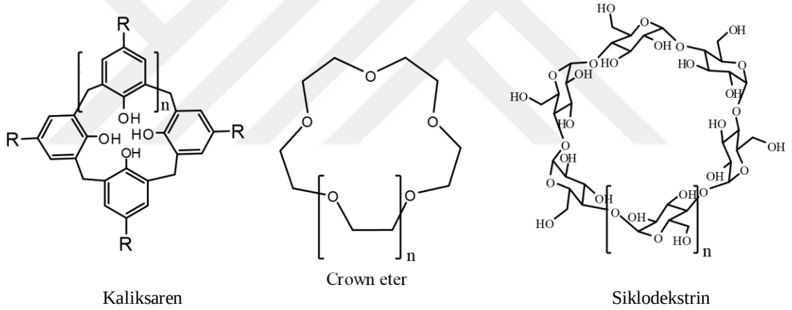
Şekil 1.1. Kaliks[n]aren, siklodekstrin ve crown eter supramoleküllerinin yapısı.
