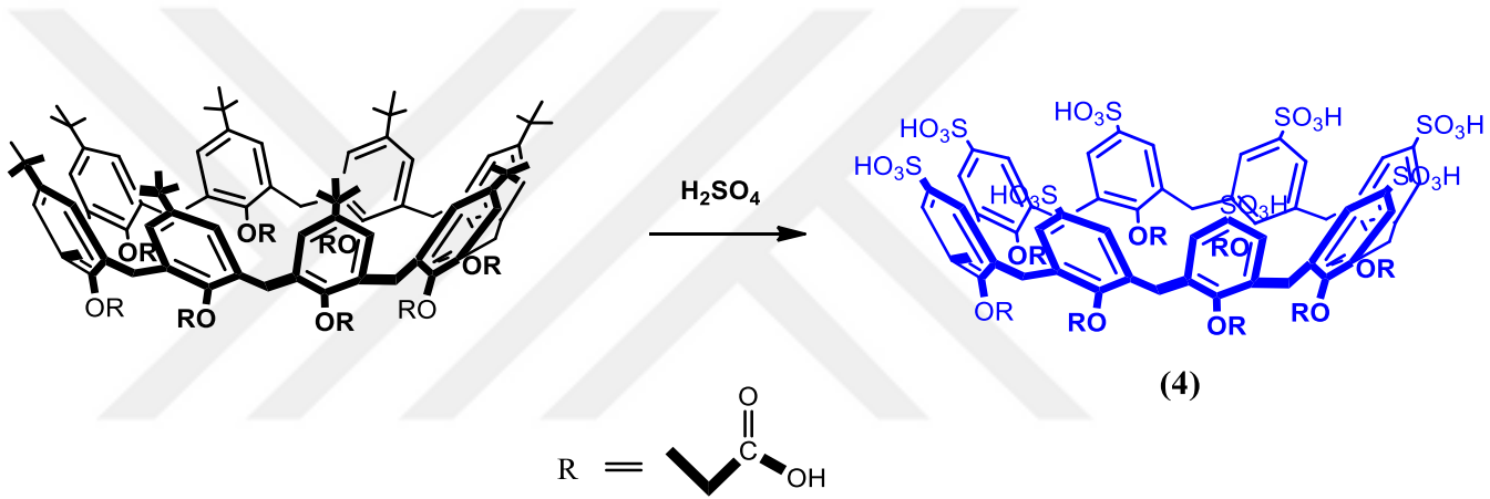
Şekil 3.4. p -Sulfokaliks[8]aren oktakarboksilik asid türevinin sentezi
