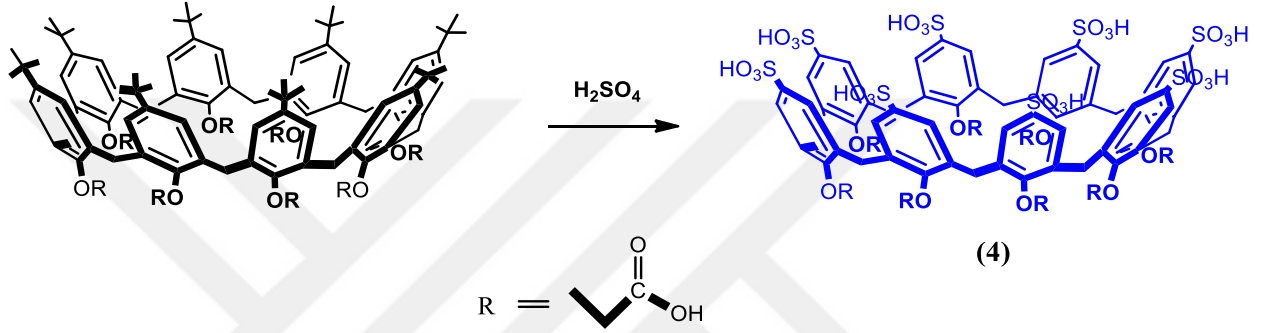
Şekil 4.7. p -Sulfokaliks[8]aren oktakarboksilikasid türevinin sentezi
