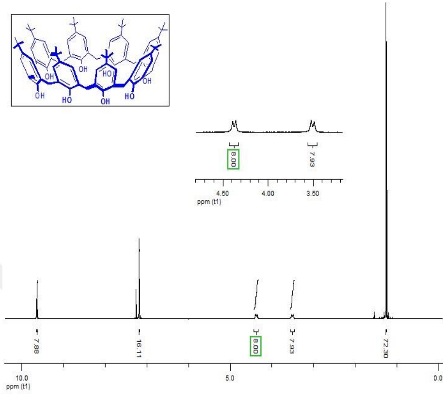
Şekil 4.2. p-ter -bütilkaliks[8]aren ^1\text{H} -NMR spektrumu
