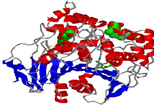
Şekil 1.30. X-ışını kristalografisi ile belirlenen Candida rugosa lipazının 3 boyutlu yapısı
