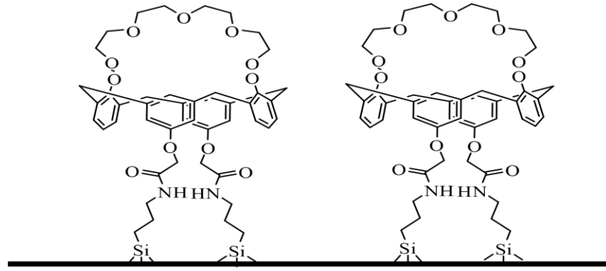
Şekil 1.21. Silikaya bağlı kaliks[4]crown-5
