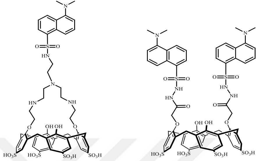
Şekil 1.16. Sülfo kaliks[4]aren dansil türevleri
