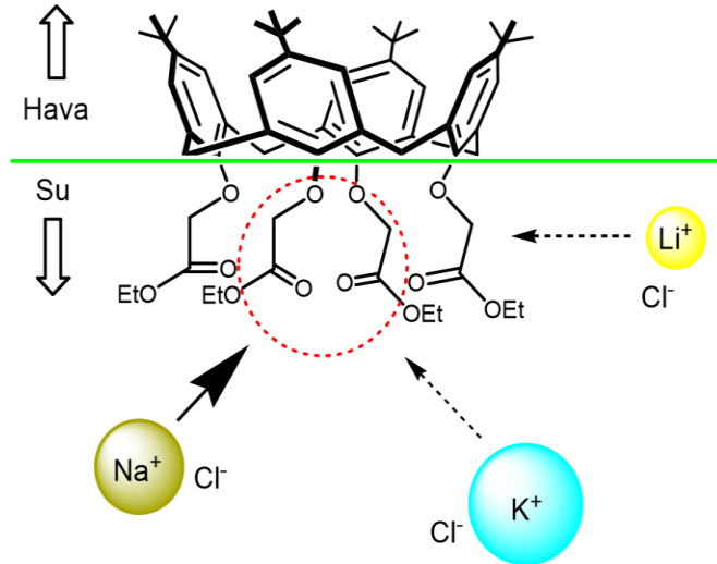
Şekil. 1.22. Su-hava arasında konumlanan kaliks[4]aren-tetraesterin \text{Na}^+ ile seçimli kompleks oluşturması
