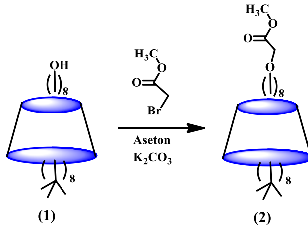
Şekil 4.3. p-ter -bütilkaliks[8]aren oktakarboksilik ester türevinin sentezi
