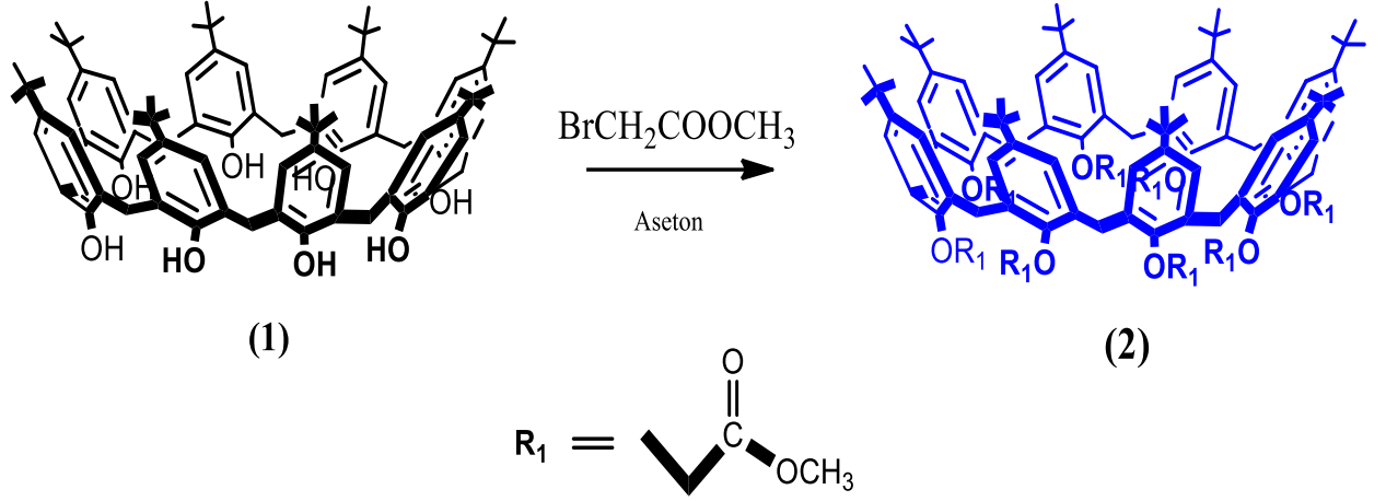
Şekil 3.2. p -terbütkaliks[8]aren oktakarboksilik ester türevinin sentezi
