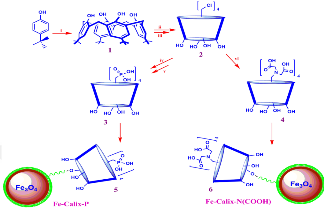
Şekil 2.6. Enantiyoseçimlilik çalışması
