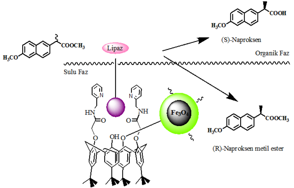
Şekil 2.4. \text{Fe}_3\text{O}_4 nanopartikülüne bağlı kaliks[4]aren'in dipridin türevinin lipaz ile immobilizasyonu
