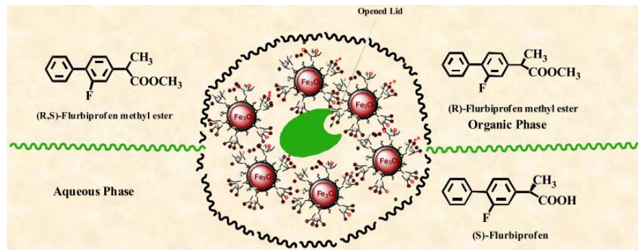
Şekil 2.9. Floresans kaliksaren türevlerinin enantiomer seçimli hidroliz
