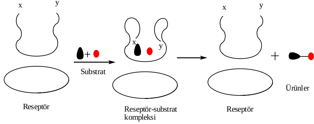
Şekil 1.13. Fonksiyonlandırılmış kaliksarenler üzerinde enzim modellerinin şematik gösterimi.
