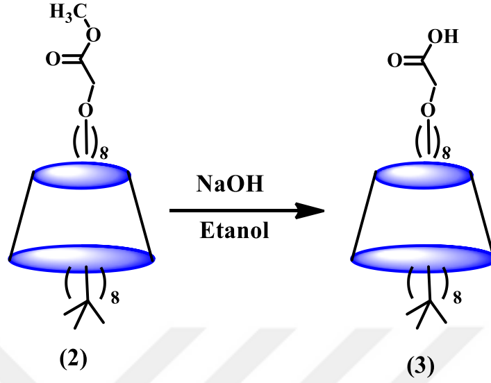
Şekil 4.5. p -ter-bütikaliks[8]aren oktakarboksilikasid türevinin sentezi
