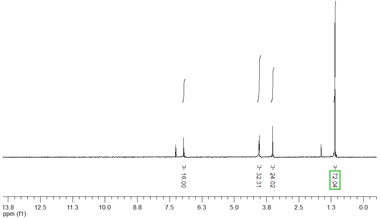
Şekil 4.4. (2) bileşiğinin 1 H-NMR spektrumu
