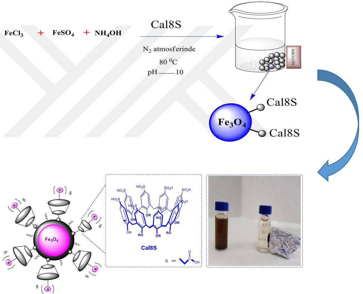
Şekil 4.9. Cal8S varlığında \text{Fe}_3\text{O}_4 nanopartiküllerin sentezi
