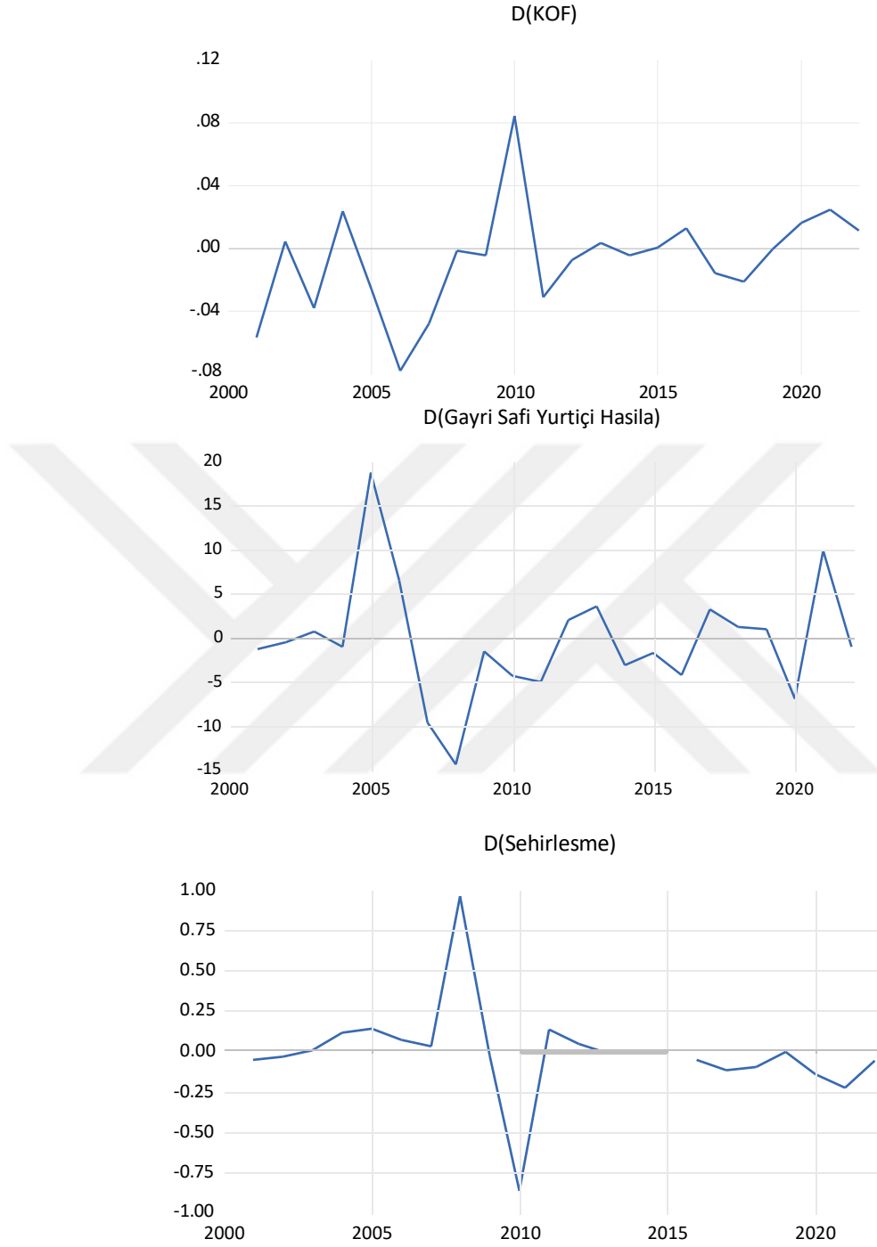
Şekil 3.3. Değişkenlerin Birinci Farklarının Grafikleri
