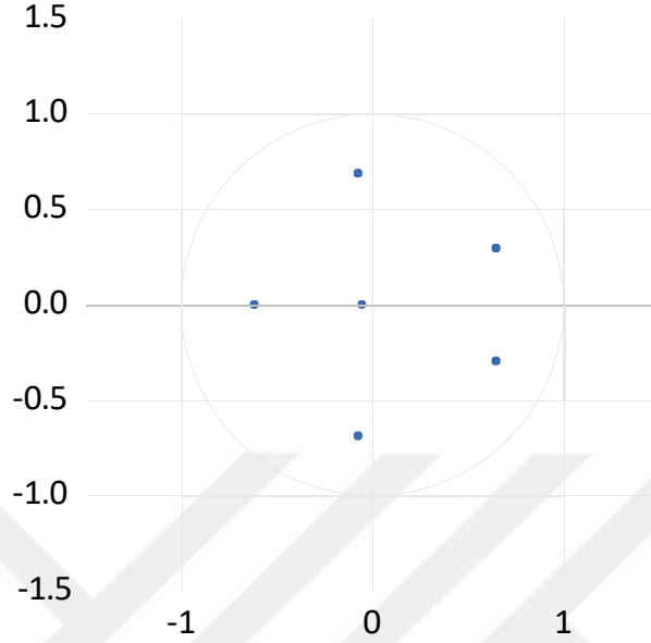
Şekil 3.4. VAR(4) Modeli için Birim Çember Grafiği
