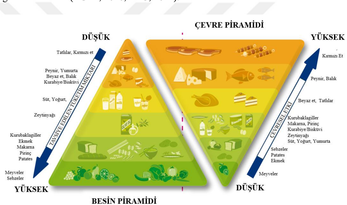
Şekil 2.4. Çift Piramit Beslenme Modeli (BCFN, 2010)
