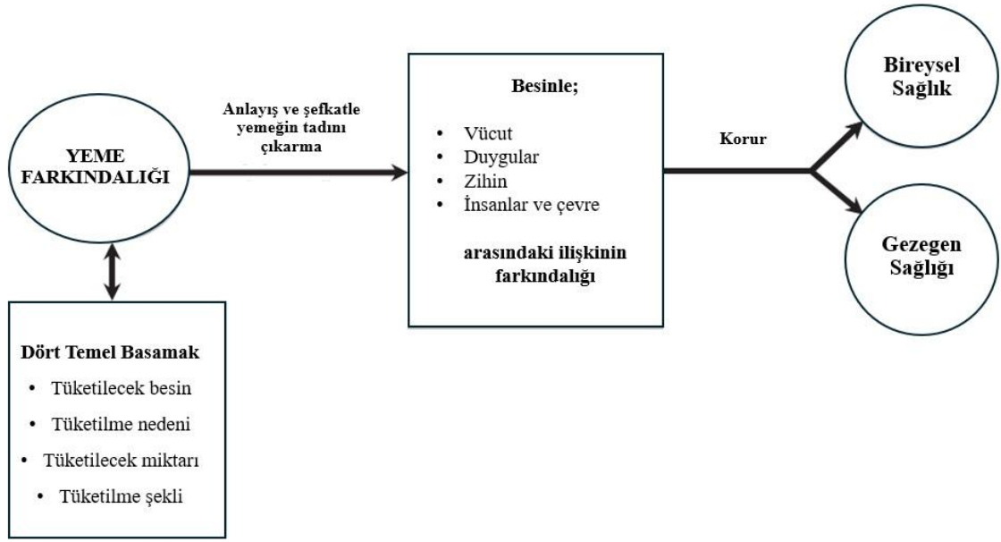
Şekil 2.5. Sürdürülebilir ve Sağlıklı Beslenme ile Yeme Farkındalığı İlişisinin Kavramsal Modeli (Fung vd., 2016)
