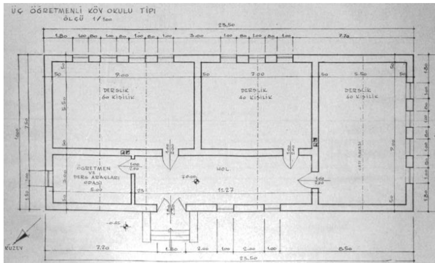
Şekil 2.45 Üç öğretmenli, üç derslikli köy okulu projesi (T.C. Maarif Vekâleti Tebliğler Dergisi,1949)
