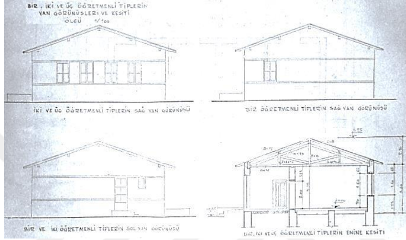
Şekil 2.46 Bir, iki ve üç öğretmenli köy okullarının batı ile doğu görünüşleri ve enine kesitleri (T.C. Maarif Vekâleti Tebliğler Dergisi,1949)
