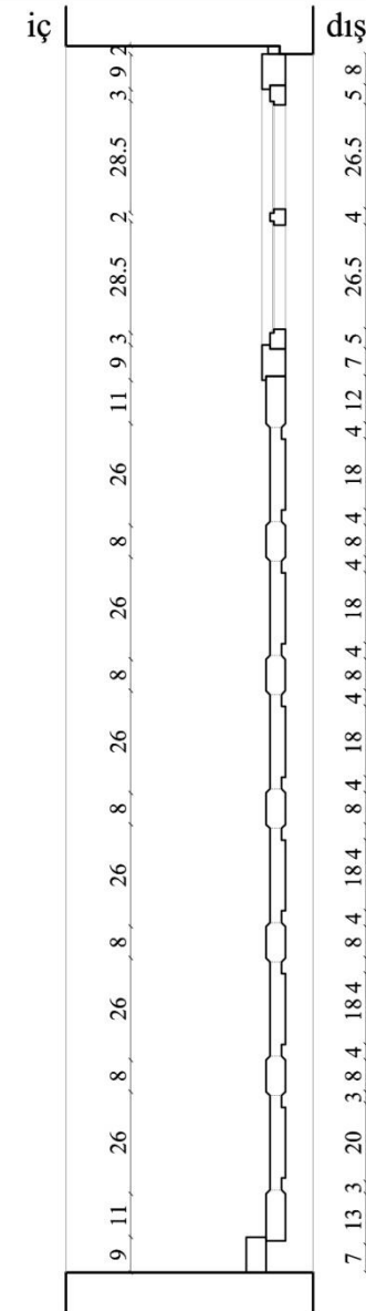
KESİT
