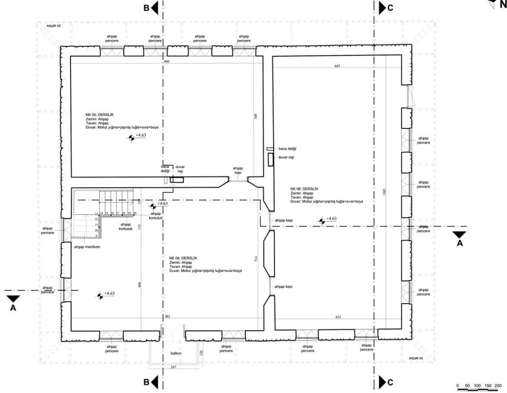
Şekil 5.77 Birinci kat planı restitüsyon çizimi (2024)
