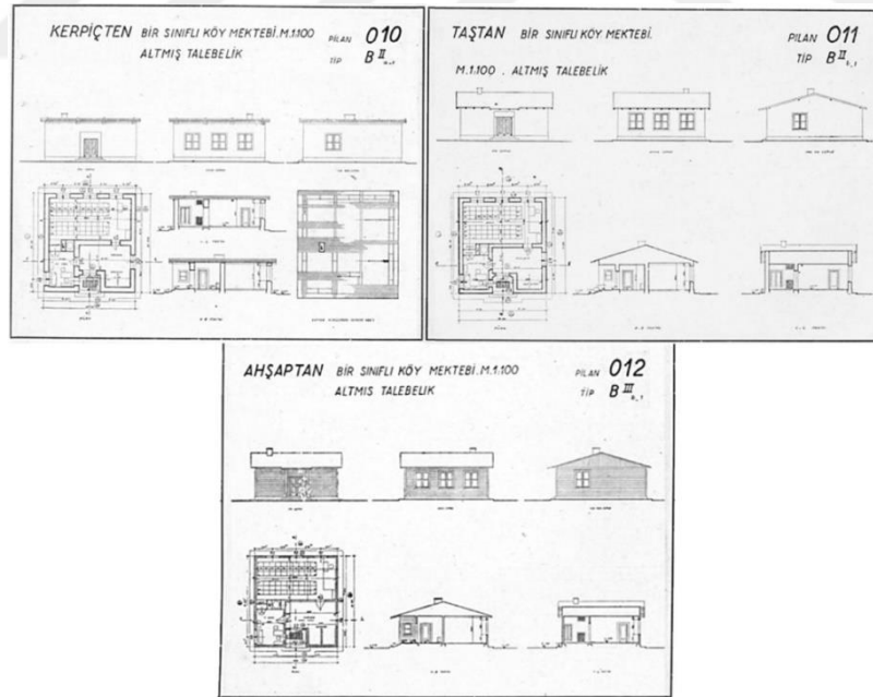
Şekil 2.17 Bir derslikli kerpiçten,taştan ve ahşaptan köy mektebi projesi (Maarif Vekâleti İlk Tedrisat Dairesi,1933; Dere ve Oral,2020, s.268-269)
