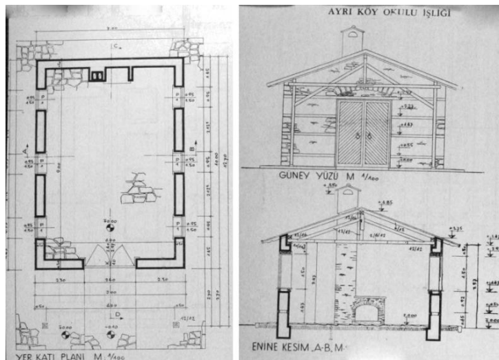
Şekil 2.37 Ayrı ışık planı (T.C. Maarif Vekâleti Tebliğler Dergisi,1945, sayı 337)
