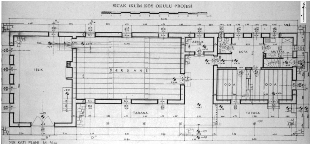
Şekil 2.35 Mutlu ve Yapanar tarafından tasarlanan sıcak iklim bölgesi köy okulu tip projesi (T.C. Maarif Vekâleti Tebliğler Dergisi,1946, s. 431-436)
