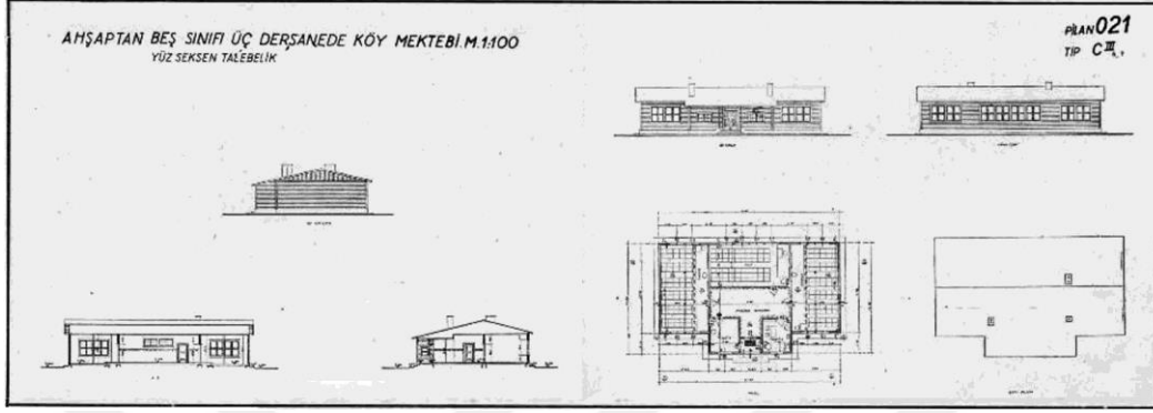
Şekil 2.23 Üç derslikli ahşaptan köy mektebi projesi (Maarif Vekâleti İlk Tedrisat Dairesi, 1933; Dere ve Oral, 2020: s.273)
