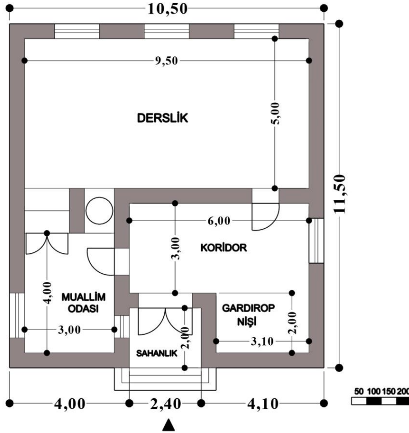
Şekil 2.18 Bir derslikli taştan yapılan köy mektebi projesinin planı (İdeli tarafından düzenlenmiştir)
