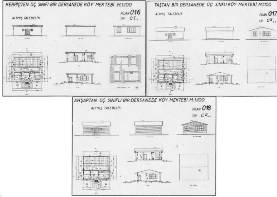
Şekil 2.19 Bir derslikli kerpiçten,taştan ve ahşaptan köy mektebi projesi (Maarif Vekâleti İlk Tedrisat Dairesi,1933; Dere ve Oral,2020, s.271-272)
