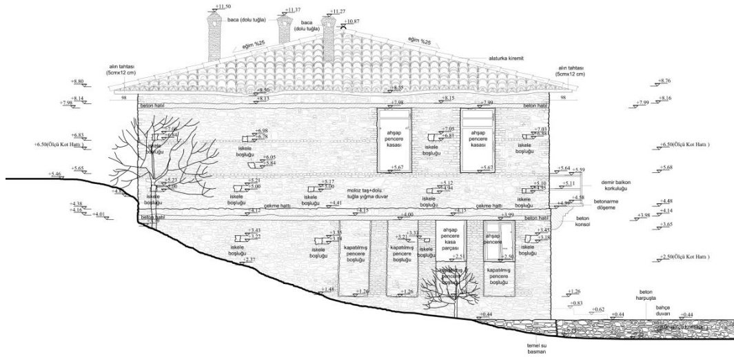
Şekil 5.34 Kuzey cephesi rölöve çizimi (2024)
