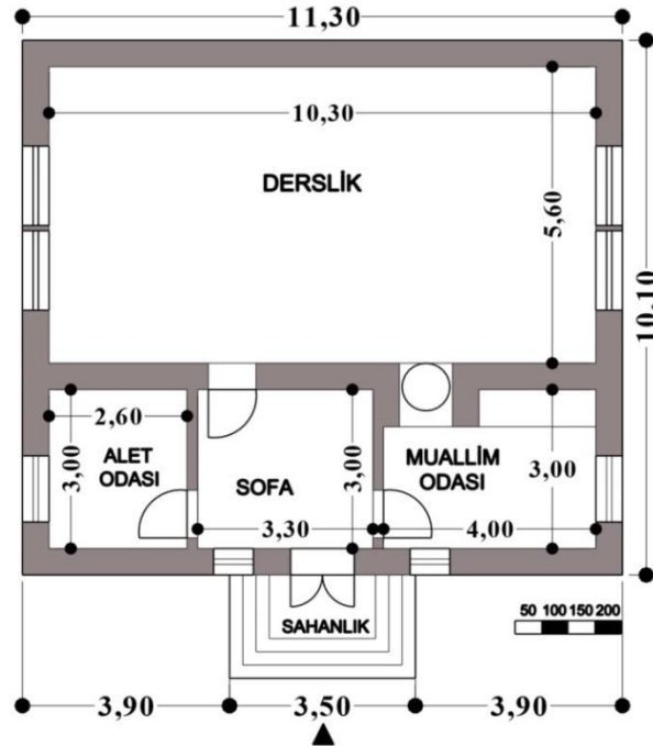
Şekil 2.20 Bir derslikli taştan yapılan köy mektebi projesinin planı (İdeli tarafından düzenlenmiştir)
