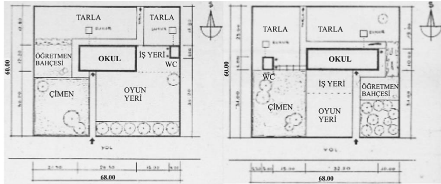
Köy Okulu Vaziyet Planı (Soğuk ve Mutedil İklim Bölgesi)
