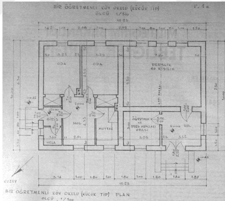
Şekil 2.41 Bir öğretmenli, bir derslikli küçük tip köy okulu projesi (T.C. Maarif Vekâleti Tebliğler Dergisi, 1949)
