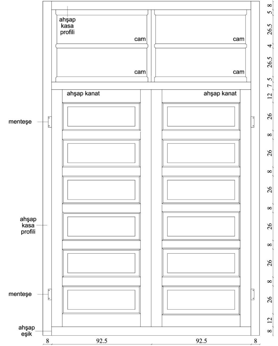
DİŞ GÖRÜNÜŞ
