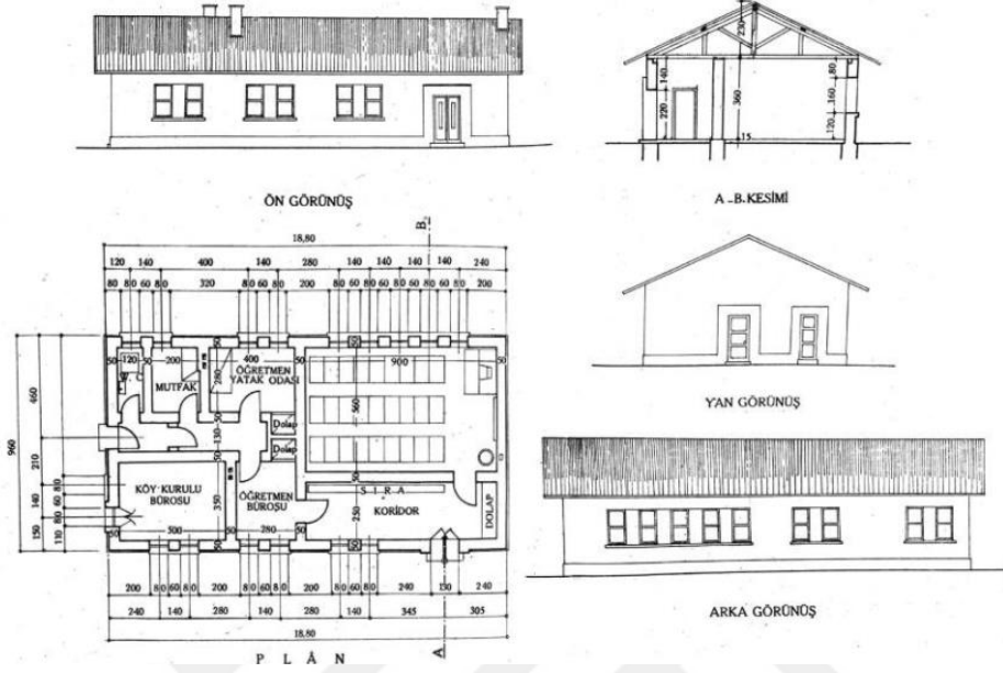
Şekil 2.27 Köy Okulu Binası adlı kitapçıktan alınan bir derslikli köy mektebi projesi (Aktürk, 2020, s. 21)
