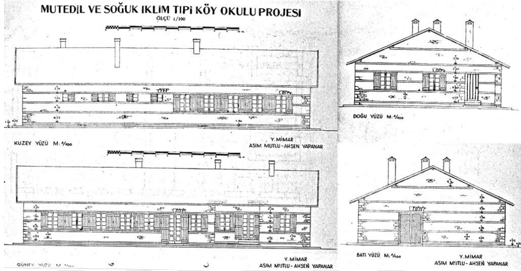
Şekil 2.34 Mutlu ve Yapanar tarafından tasarlanan soğuk ve ılıman iklim bölgesi köy okulu tip projesi (T.C. Maarif Vekâleti Tebliğler Dergisi,1945, s.152-155)
