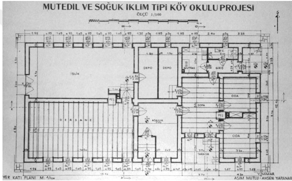
Şekil 2.33 Mutlu ve Yapanar tarafından tasarlanan soğuk ve ılıman iklim bölgesi köy okulu tip projesi (T.C. Maarif Vekâleti Tebliğler Dergisi,1945: s. 152-155)
