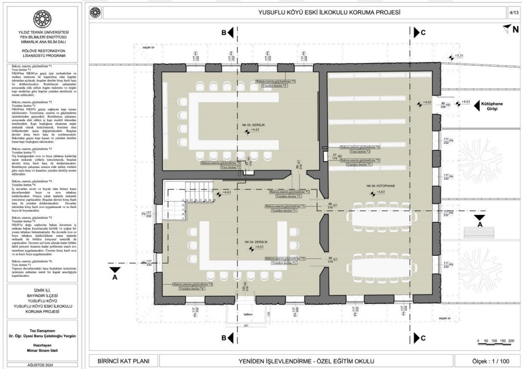
Şekil 6.5 Birinci kat planı restorasyon çizimi (2024)
