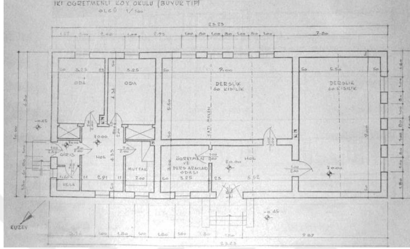
Şekil 2.44 İki öğretmenli, iki derslikli büyük tip köy okulu projesi (T.C. Maarif Vekâleti Tebliğler Dergisi,1949)
