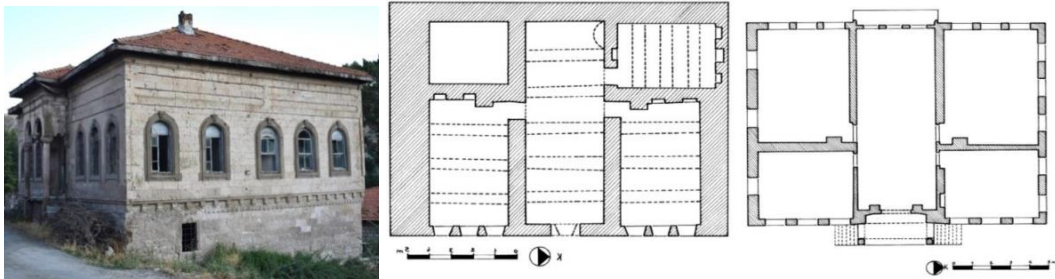
Şekil 2.8 Kayseri Başköy İptidai Mektebi görseli, zemin kat ve birinci kat planları (Kızılgın, 2024, s.4)
