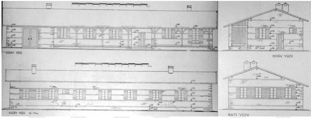
Şekil 2.36 Mutlu ve Yapanar tarafından tasarlanan sıcak iklim bölgesi köy okulu tip projesinin cepheleri (T.C. Maarif Vekâleti Tebliğler Dergisi,1946, s. 431-436)
