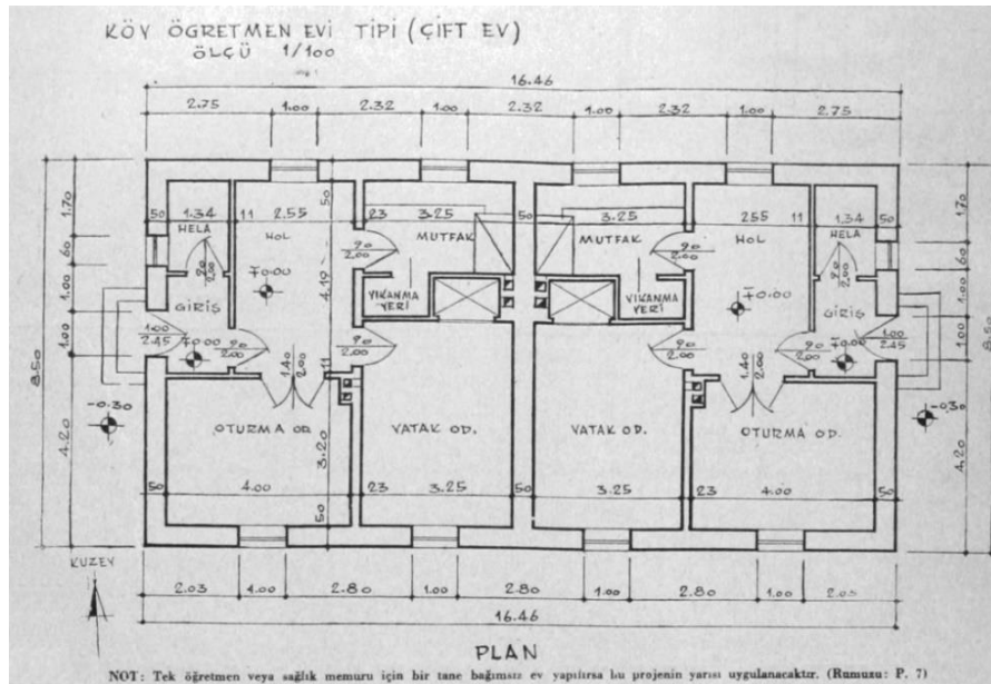
Şekil 2.47 Öğretmen evi bulunmayan köy okulları için inşa edilecek öğretmen ve sağlık memuru evi (T.C. Maarif Vekâleti Tebliğler Dergisi,1949)
