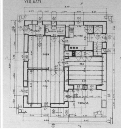
Plan 2. Sıcak iklim tipi ayrı öğretmen evi projesi
