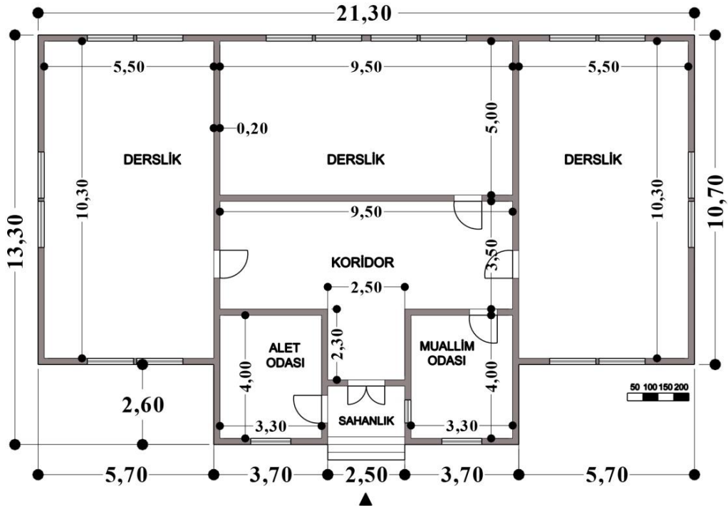
Şekil 2.24 Üç derslikli ahşaptan köy mektebi projesinin planı (İdeli tarafından düzenlenmiştir)
