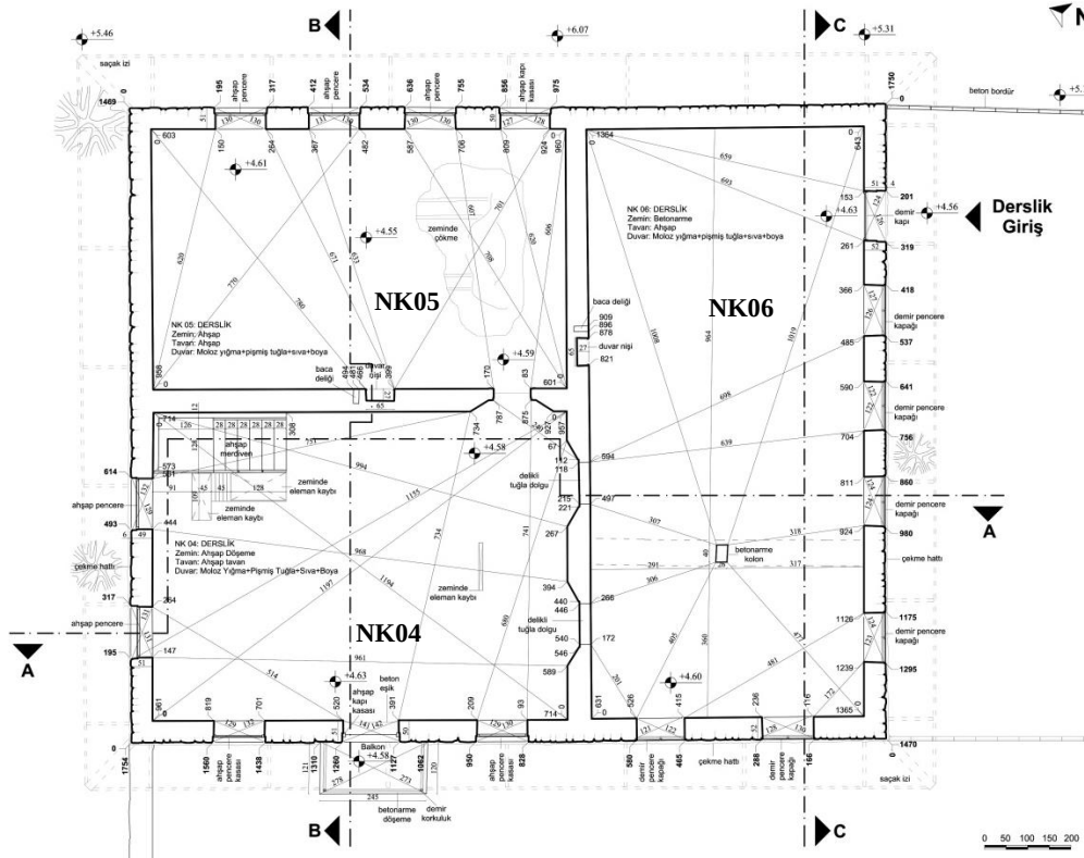
Şekil 5.24 Birinci kat planı rölöve çizimi (2024)
