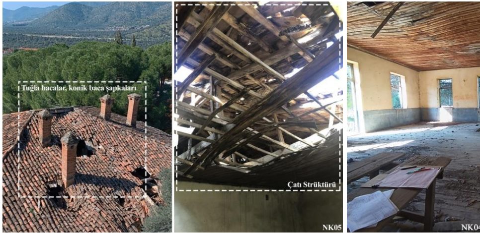
Şekil 5.64 Baca, çatı strüktürü ve döşeme detayları (İdeli Kişisel Arşivi, 2024)
