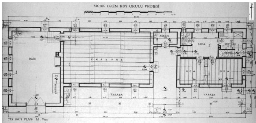
Şekil 4.47 Mutlu ve Yapanar tarafından tasarlanan sıcak iklim bölgesi köy okulu tip projesi (T.C. Maarif Vekâleti Tebliğler Dergisi, 1946, s. 431-436)
