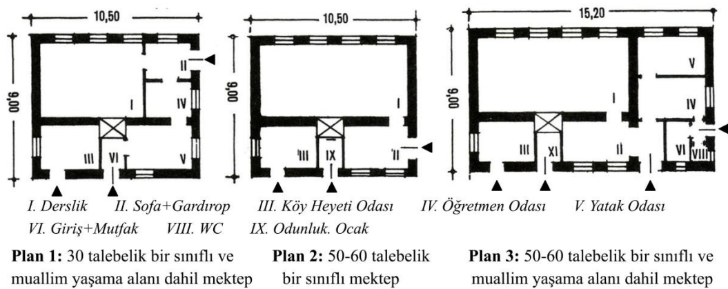
Şekil 2.29 ‘Yeni Köy Okulları Bina Tipleri Üzerinde Deneme’ kitapçığındaki tip projeler (Karain, 1996, s. 10; Lihotzky,1939)
