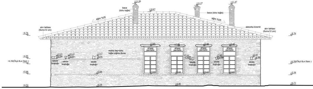
Şekil 5.85 Doğu cephesi restitüsyon çizimi (2024)
