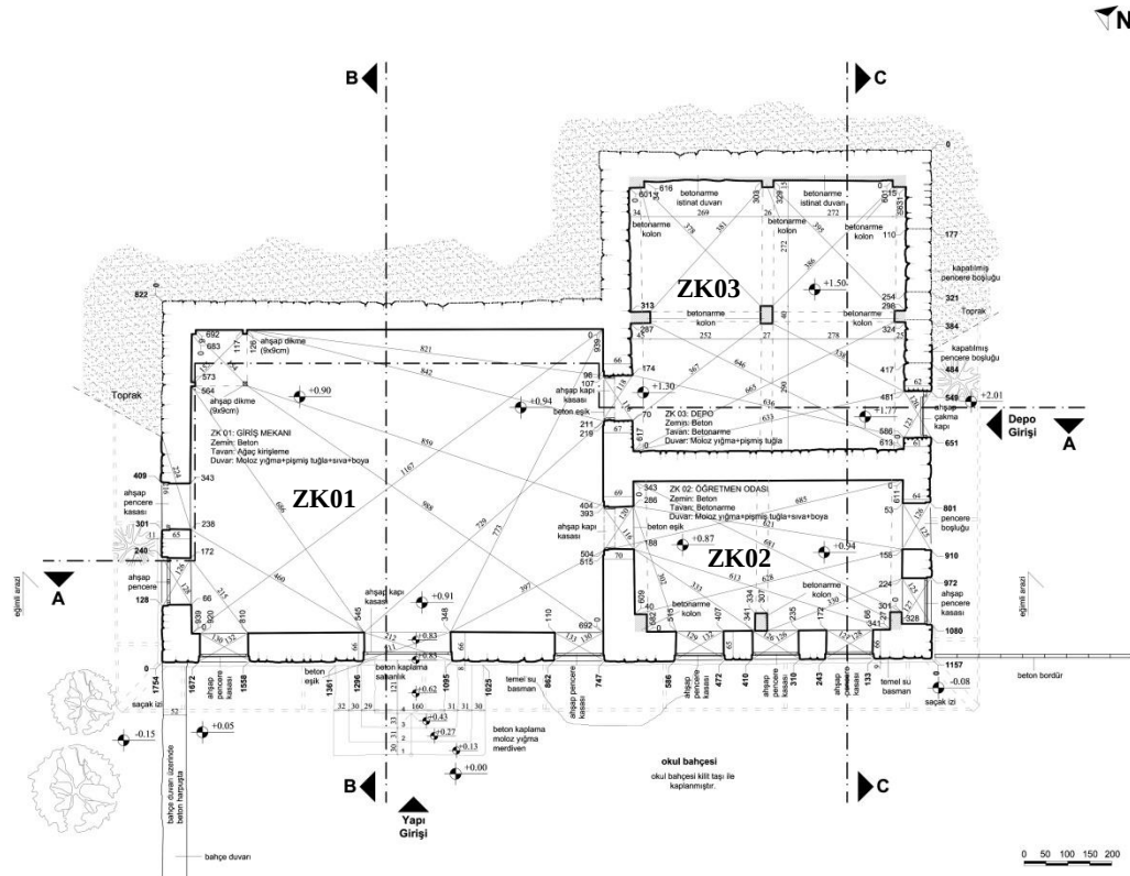
Şekil 5.14 Zemin kat planı rölöve çizimi (2024)
