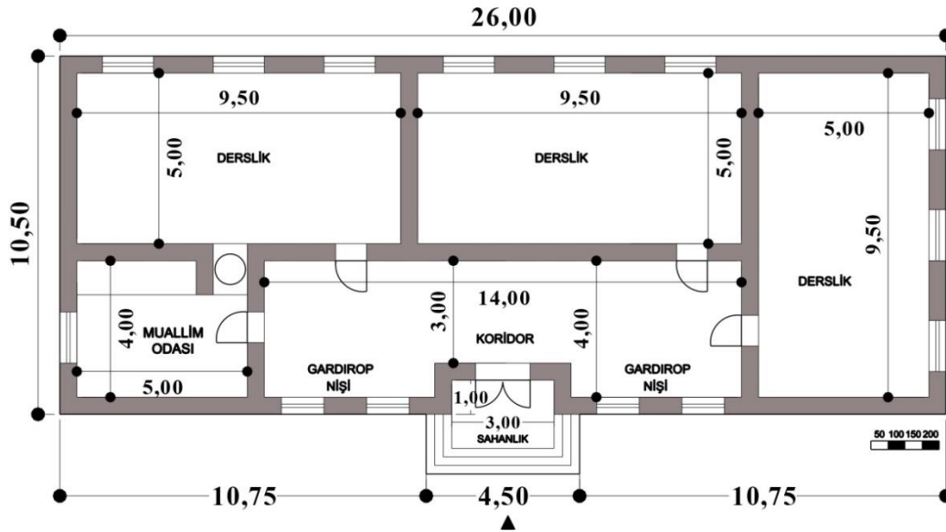
Şekil 2.22 Üç derslikli taştan yapılan köy mektebi projesinin planı (İdeli tarafından düzenlenmiştir.)
