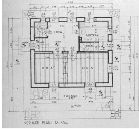
Plan 1. Mutedil ve soğuk iklim tipi ayrı öğretmen evi projesi
