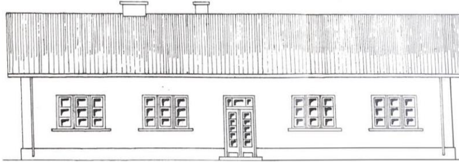
Şekil 2.26 Köy Okulu Binası adlı kitapçıkta yer alan bir derslikli köy mektebi projesinin cephesi (Aktürk, 2020, s.21)
