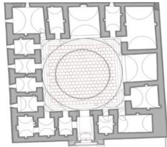
Şekil 2.3 Tokat Yağlıbasan Medresesi plan ve görünüşü (Korkmaz, Çarhoğlu, Usta, Gedik, 2013, s. 45)
