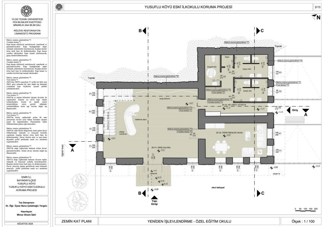
Şekil 6.2 Zemin kat planı restorasyon çizimi (2024)
