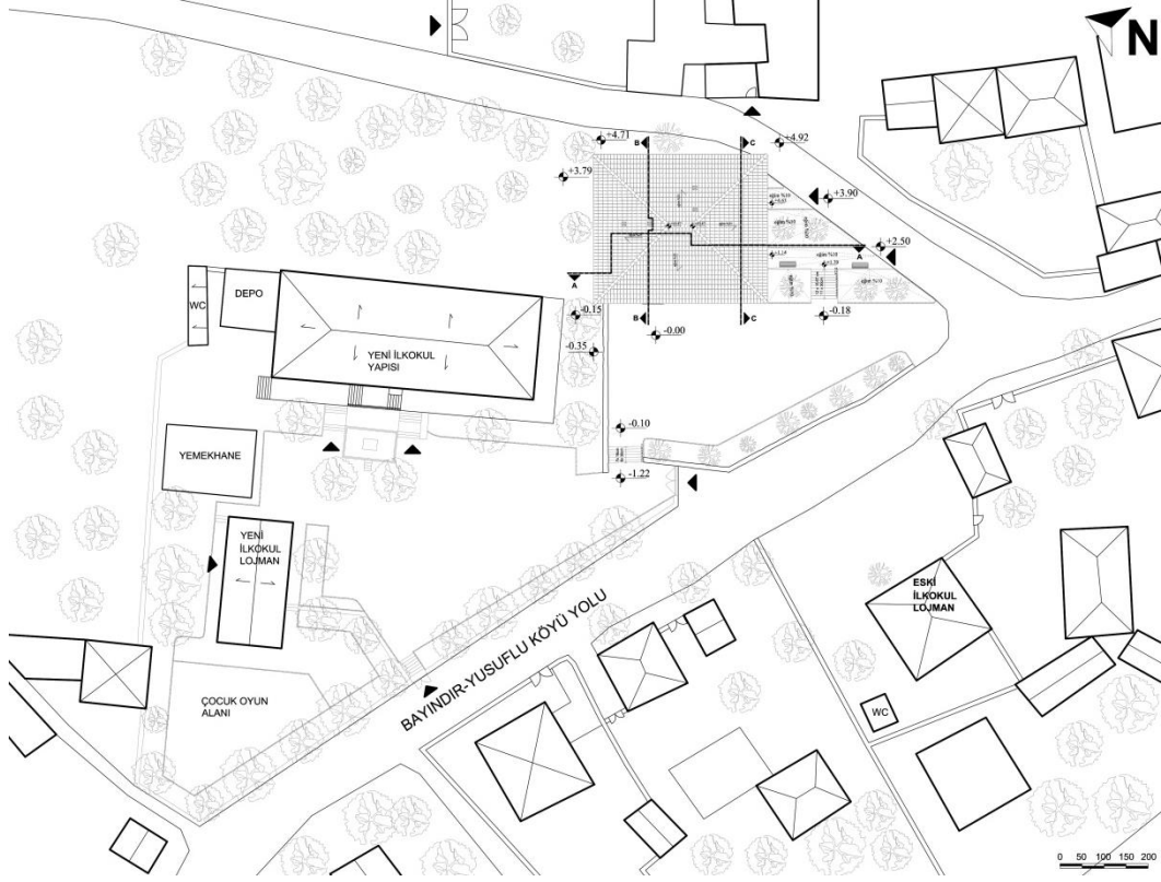
Şekil 6.1 Vaziyet planı restorasyon çizimi (2024)
