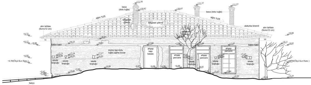
Şekil 5.43 Doğu cephesi rölöve çizimi (2024)
