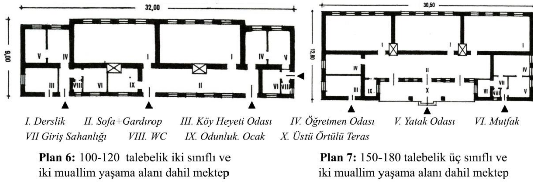
Şekil 2.31 Yeni Köy Okulları Bina Tipleri Üzerinde Deneme Kitapçığındaki tip projeler (Karain, 1996, s.10; Lihotzky,1939)
