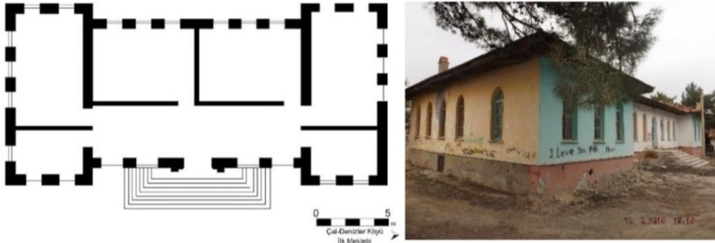
Şekil 2.15 Denizler Köyü Mektebi'nin plan ve cephesi (Türkmen, 2021, s.355-393)
