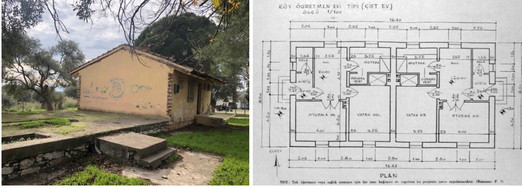
Şekil 4.53 Kızılcaova Köyü İlkokulu 3. öğretmenevi ve sağlık memuru evi temeli (Sol görsel: Öğretmenevi (İdeli Kişisel Arşivi, 2024), sağ görsel: Öğretmenevi ve sağlık memuru evi planı (T.C. Maarif Vekâleti Tebliğler Dergisi, 1949)
