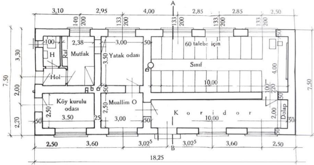
Şekil 2.25 Köy Okulu Binası adlı kitapçıkta yer alan bir derslikli köy mektebi projesinin planı (Aktürk, 2020, s.21)
