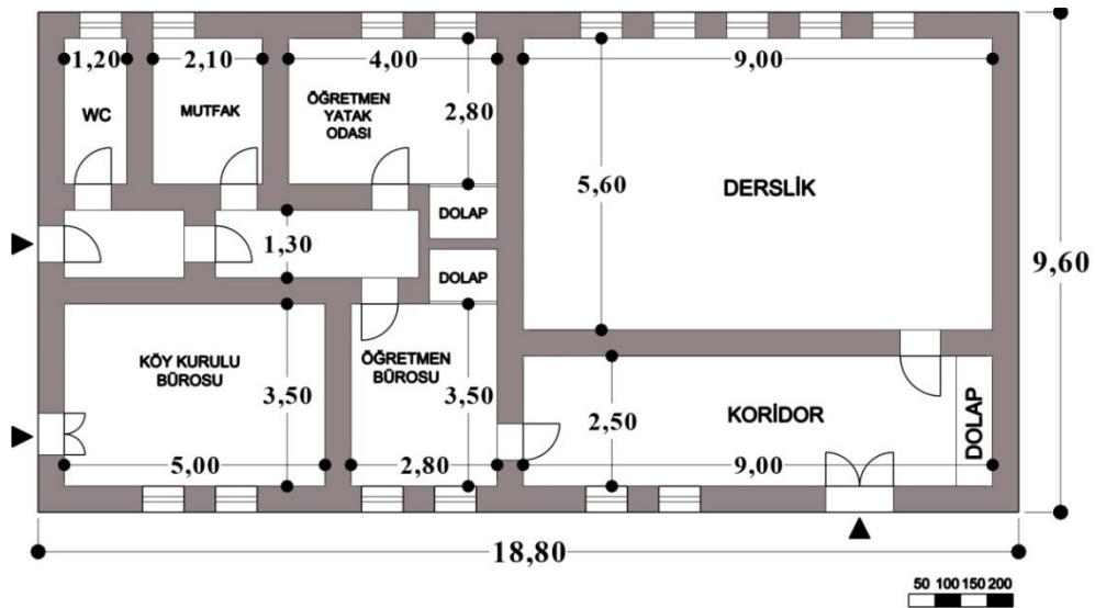
Şekil 2.28 Köy Okulu Binası kitapçığından alınan bir sınıflı bir projesinin planı (İdeli tarafından düzenlenmiştir)
