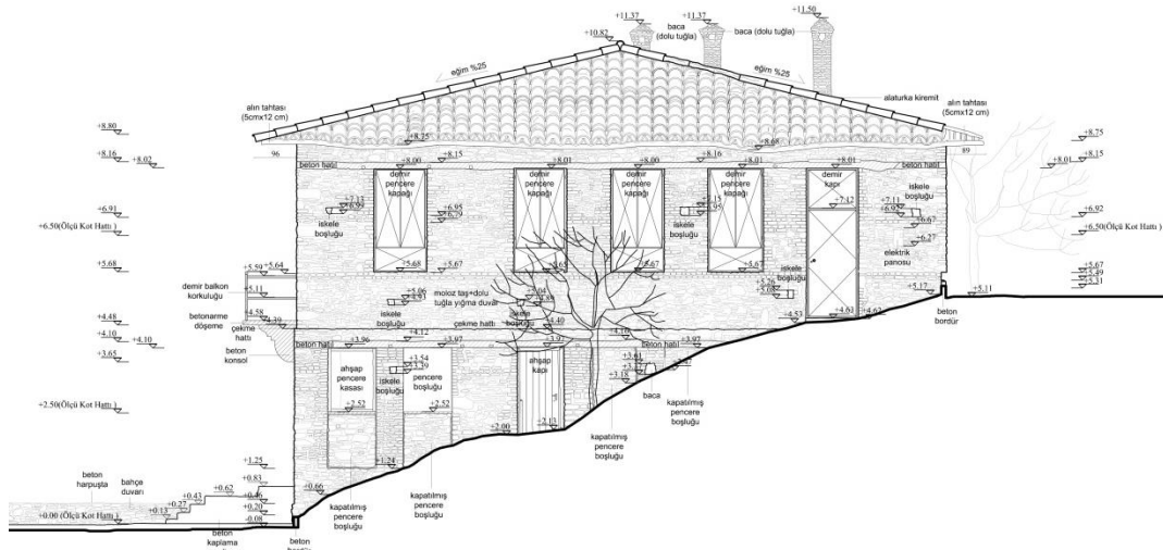
Şekil 5.37 Güney cephesi rölöve çizimi (2024)
