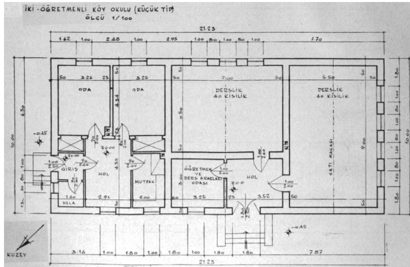
Şekil 2.43 İki öğretmenli, iki derslikli küçük tip köy okulu projesi (T.C. Maarif Vekâleti Tebliğler Dergisi,1949)
