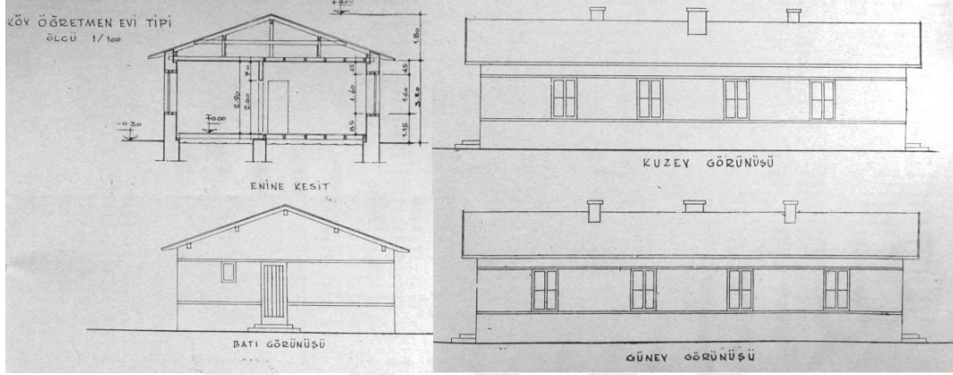
Şekil 2.48 Öğretmenevi bulunmayan köy okulları için inşa edilecek öğretmen ve sağlık memuru evinin cepheleri ve kesitleri (T.C. Maarif Vekâleti Tebliğler Dergisi,1949)
