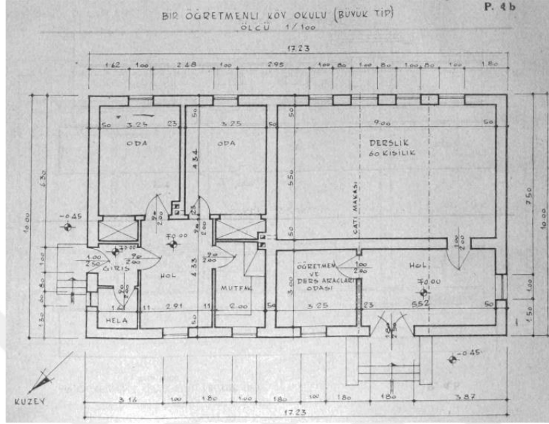
Şekil 2.42 Bir öğretmenli, bir derslikli büyük tip köy okulu projesi (T.C. Maarif Vekâleti Tebliğler Dergisi,1949)
