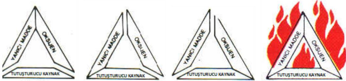
Şekil 1.1. Yangın Üçgeni
