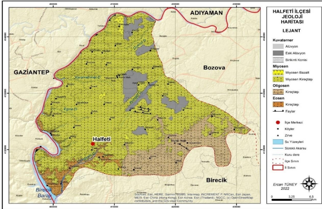
Şekil 2. 1. Halfeti İlçesi Jeoloji Haritası
