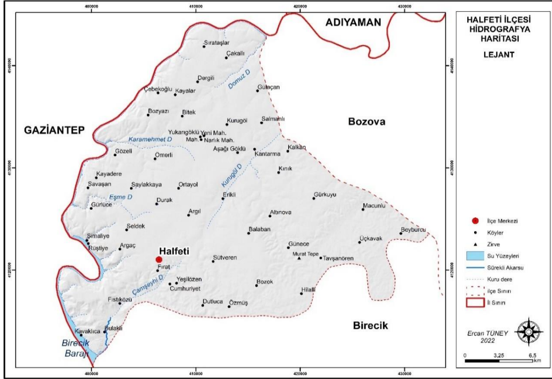
Şekil 2. 6. Halfeti İlçesi ve Yakın Çevresinin Hidrografya Haritası
