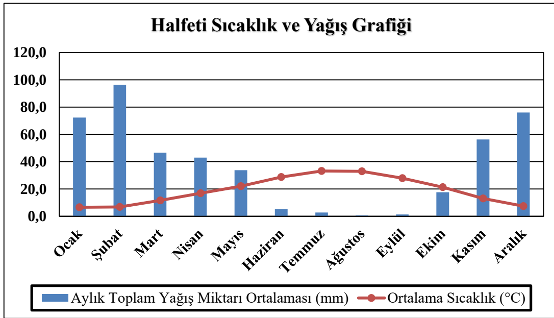
Şekil 2. 4. Halfeti Sıcaklık ve Yağış Grafiği
