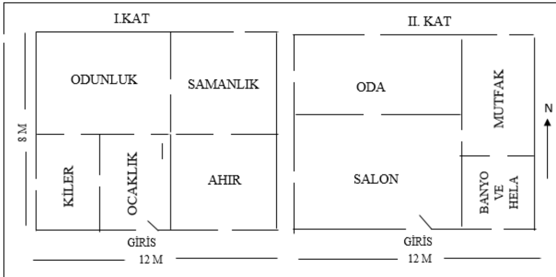
Şekil 3.35. Kırsal Sahadaki Geleneksel Halfeti Evlerinin Planı
