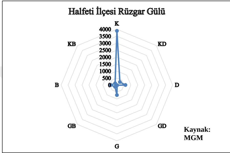
Şekil 2. 5. Halfeti İlçesinin 1985-2005 Yılları Arasına Ait Rüzgâr Frekans Gülü
