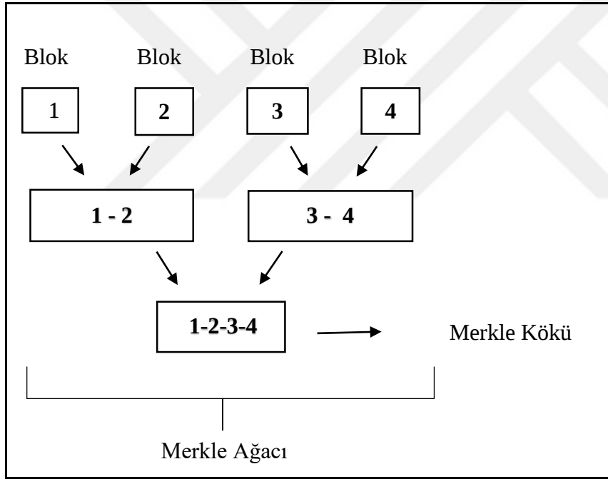
Şekil 7. Merkle Ağacı
