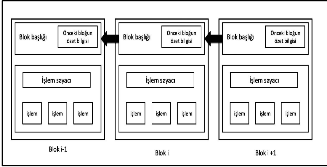
Şekil 4. Blokzincir 51
