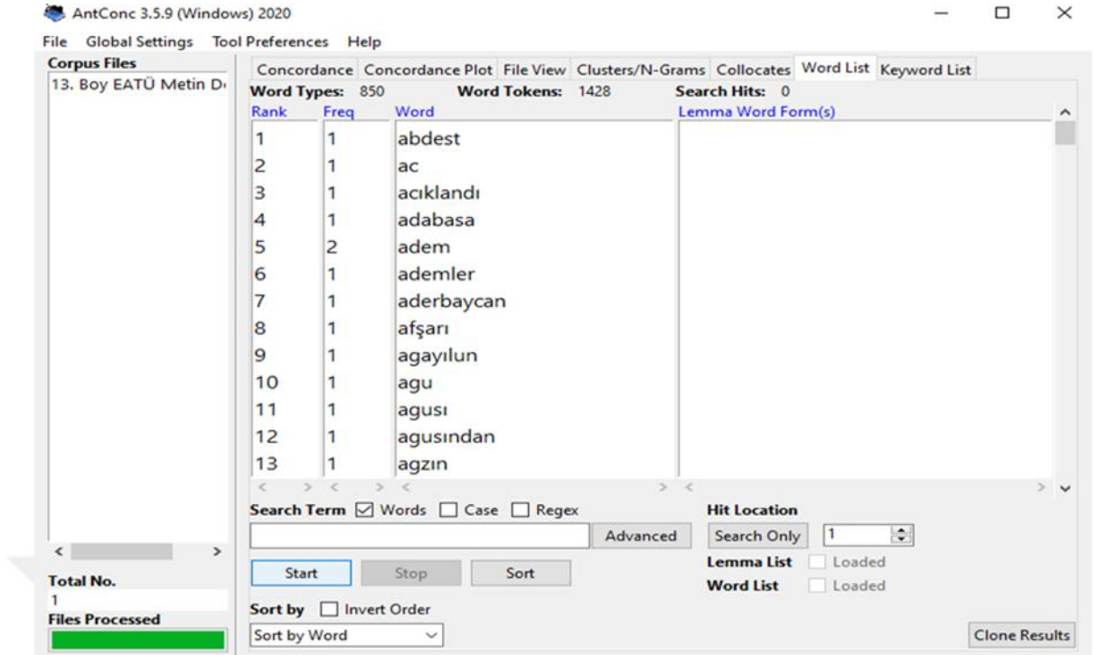
Şekil 8. AntConc 3.5.9 (Windows) 2020 Yazılımında Alfabetik Sıralı Kelime Listesi Ekran Görüntüsü
