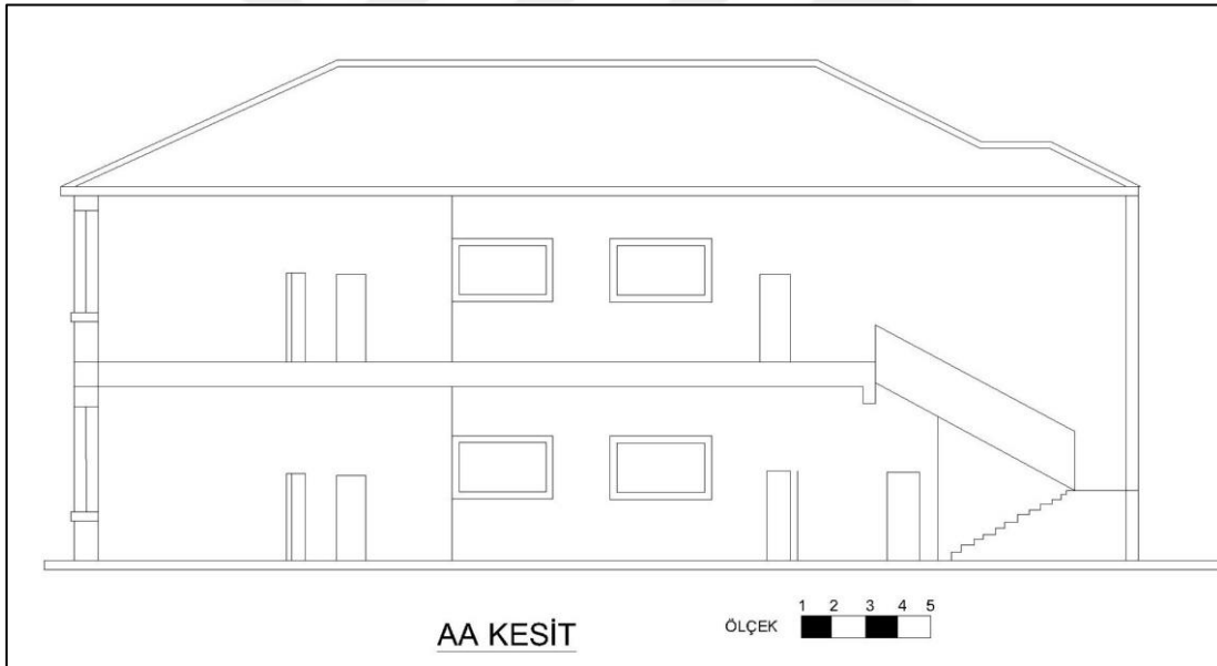
Çizim 3.5. Aksaray Gazi Mektebi AA kesiti
