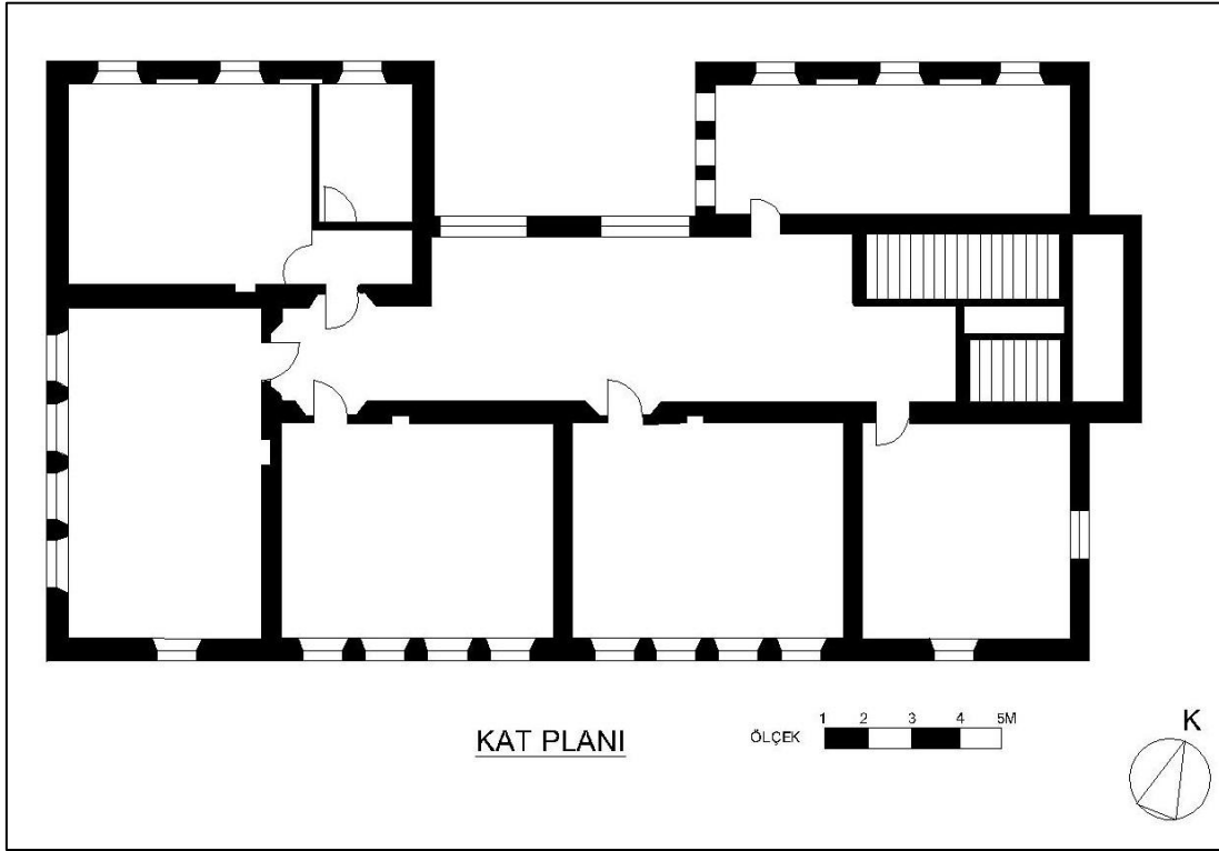
Plan 3.2. Aksaray Gazi Mektep Zemin Kat Planı
