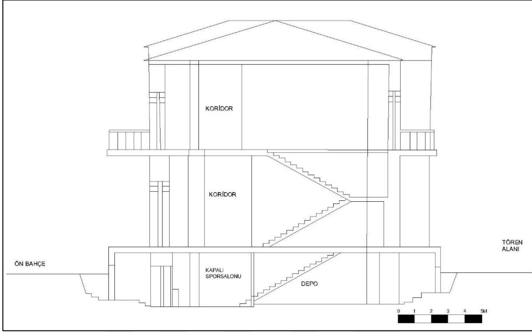
Çizim 3.3. Bodrum Kat Ve Üst Kata Geçişin Sağlandığı Merdivenler
