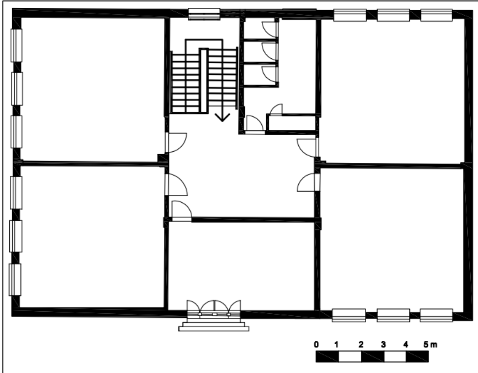
Plan 3.3. Zafer Mektebi Planı
