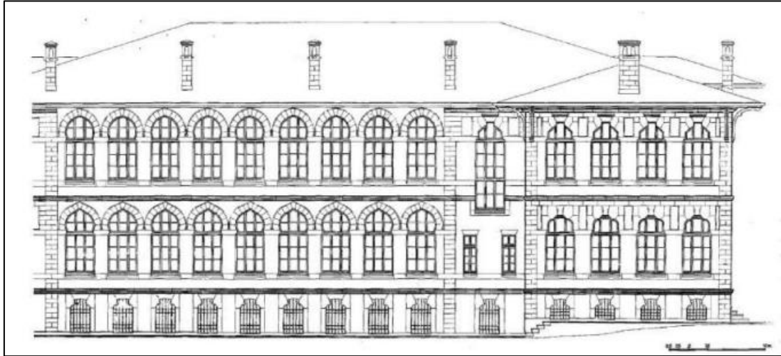
Çizim 4.1. Konya Öğretmen Lisesi Cephe Çizimi
