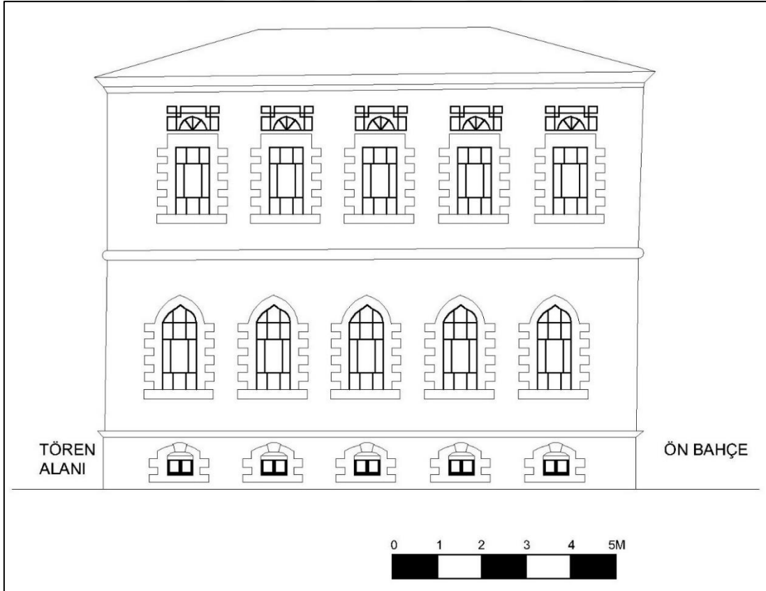
Çizim 3.1. Aksaray İdadi Mektep Güney Cehpe Görünüm
