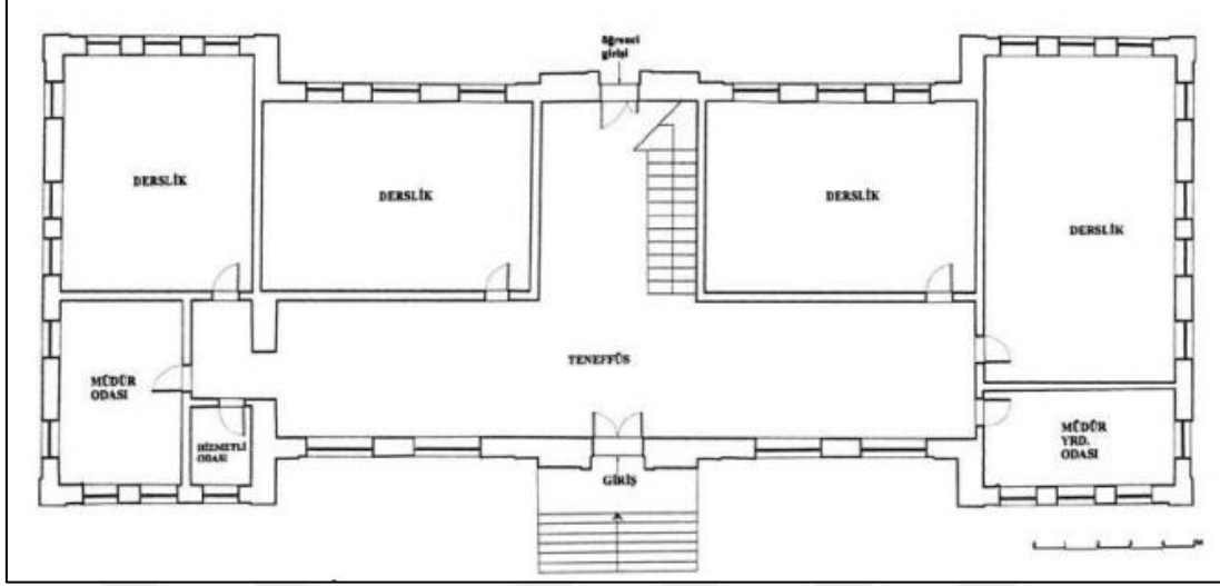
Plan 4.4. Kadınhanı İlköğretim Okulu Planı
