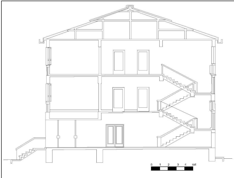
Çizim 3.7. Zafer Mektebi Kesiti
