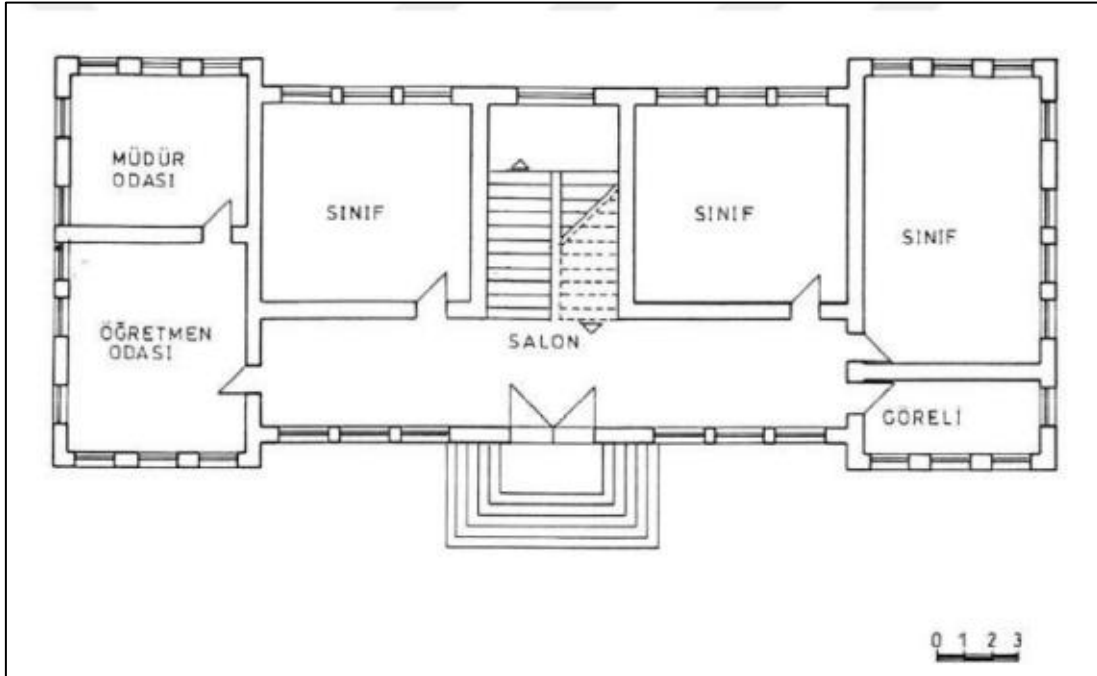
Plan 4.2. Akşehir Cumhuriyet İlkokulu Planı
