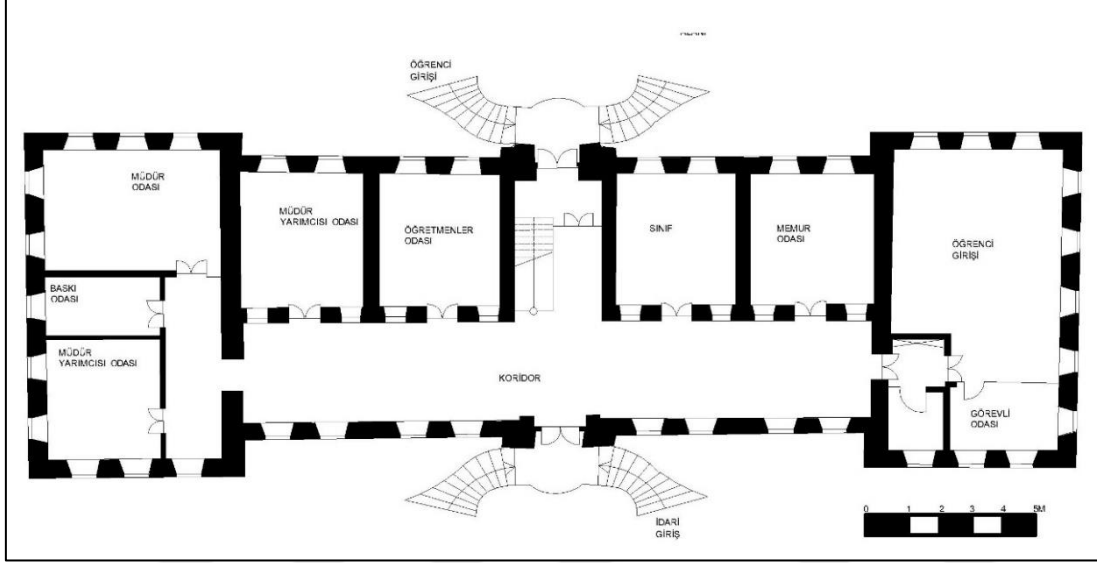
Plan 3.1. Aksaray İdadi Mektep Zemin Kat Planı
