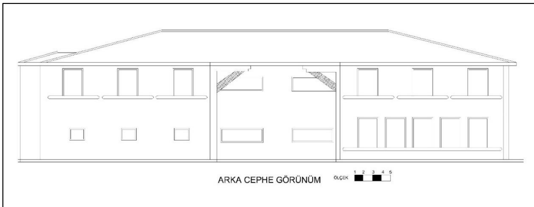
Çizim 3.4. Aksaray Gazi Mektebi Kuzey Batı Cephe Görünüm
