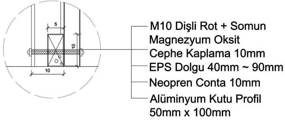
Şekil 5.15. Profil, taşıyıcı dikme, duvar bağlantı detayı (Kişisel Arşiv).
