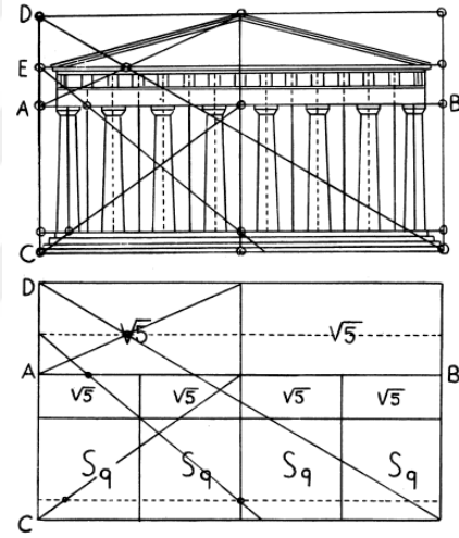
Şekil 4.3. Partenon için altın oran ölçümü, Ghyka(1977).
