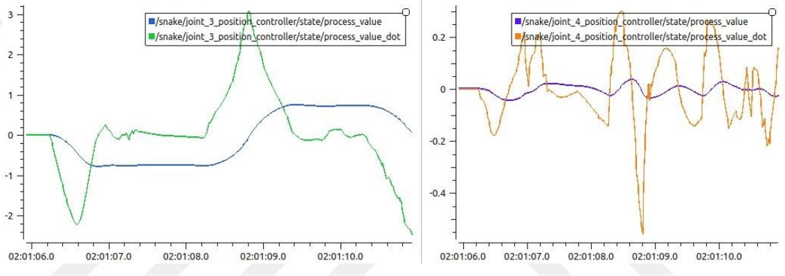
Şekil 5.22. Akordeon hareketi için process value ve dot grafiği,
