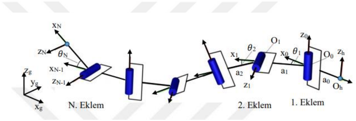
Şekil 3.12. N bileşenli yılanın kinematik gösterimi [15].
