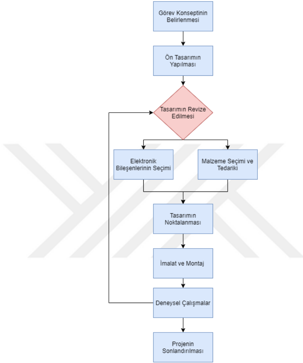
Çizelge 4.1. Biyomimetik yılansı robotun tasarım akış şeması
