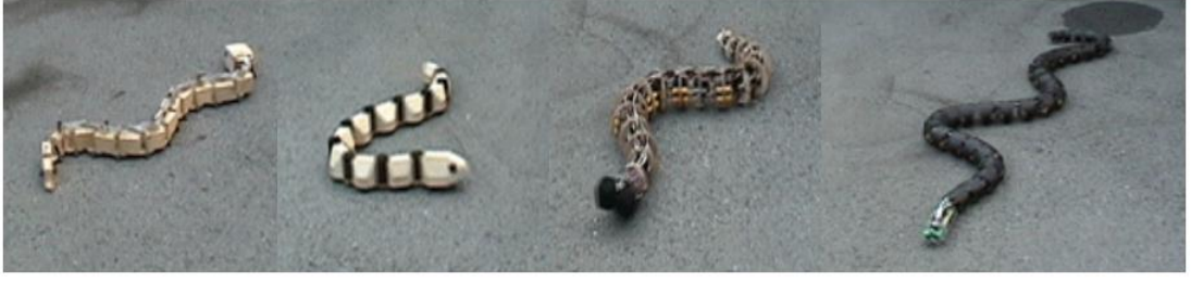
Şekil 2.6. Miller tarafından geliştirilen farklı tip yılan robotlar [12].
