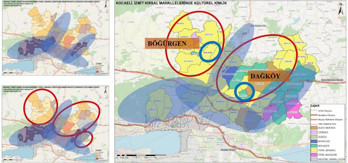
Şekil 4.20 Kocaeli, İzmit kırsal ve kısmen kırsal mahallelerinde karakter analizi ve alt bölgeleme sonucu yakından bakılacak kırsal yerleşmelerin belirlenmesi (Tez çalışması kapsamında hazırlanmıştır.)
